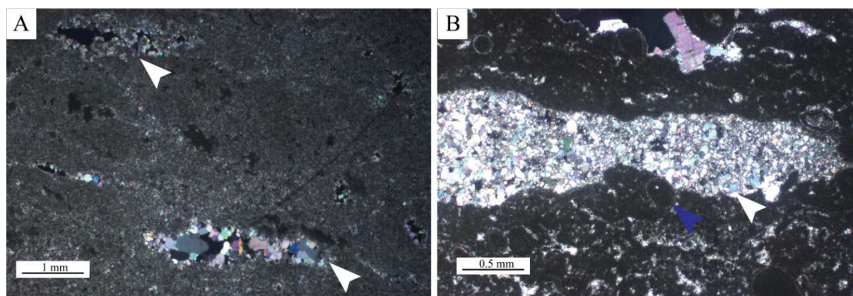
Figure 3.7: (A) [LPA] Faciès mudstone à fenestrées tabulaires, partiellement recristallisées par un ciment drusique (flèches blanches); (B) [LPA] Faciès wackestone à oïdes (flèche bleue) et fenestrées tabulaires, entièrement cimentées par un ciment microcristallin isométrique (flèche blanche).
