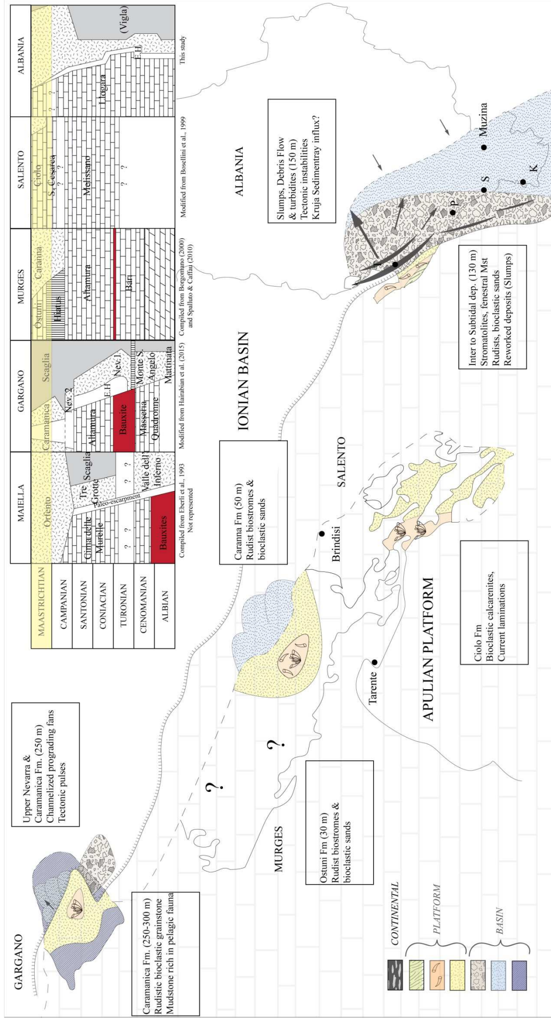
Figure 5.6: Représentation paléogéographique de la marge Apulienne au Maastrichtien. Les faciès de dépôts sont représentés depuis les plus externes (Bassin) vers les plus internes (continental émerse).
