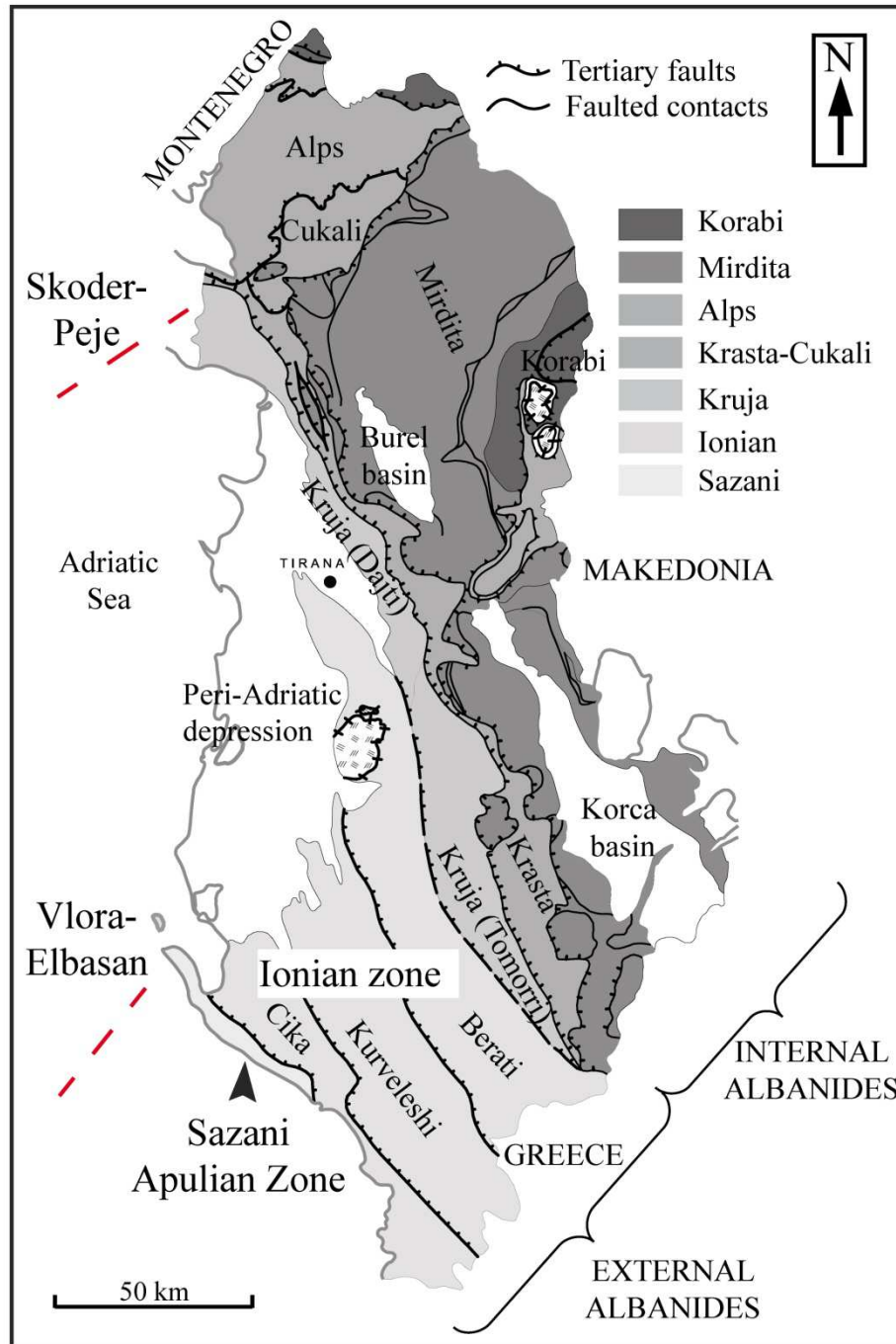
Figure 1.7: Carte litho-tectonique simplifiée de l'Albanie représentant les différentes zones litho-tectoniques. Les chevauchements et accidents tectoniques majeurs (Skoder-Peje et Vlora-Elbasan, en pointillés rouges) sont indiqués. Carte modifiée d'après Moisiu & Gurabardhi (2004) et Rubert et al. (2012).
