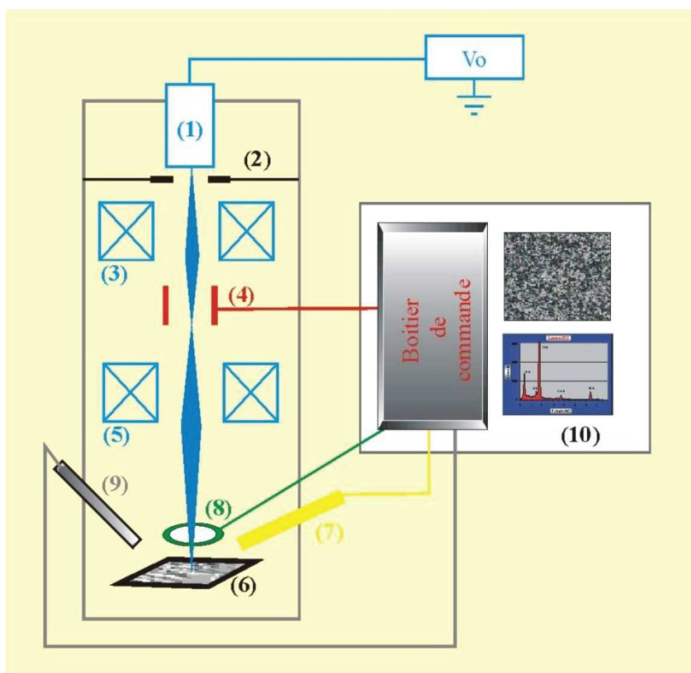
Figure 2.9: Représentation schématique d'un microscope électronique à balayage. (1) canon à électron ; (2) diaphragme ; (3) système de condensateurs ; (4) bobines de déflection reliées au boîtier de commande ; (5) lentille objectif ; (6) platine de support de l'échantillon ; (7) électrons secondaires ; (8) rayons X ; (9) électrons retrodiffusés ; (10) traitement et formation de l'image. D'après Galaup, communication personnelle.
