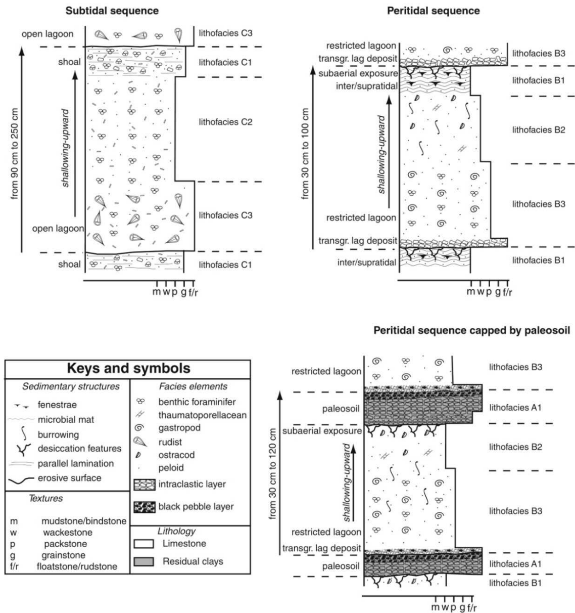
Figure 1.19: Représentation schématique de trois séquences de dépôt « type » identifiées dans les Murges (Albien-Cénomaniens), d'après Spalluto et al. (2012).
