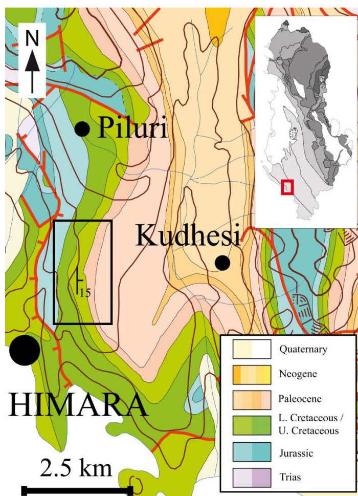
Figure 4.7: Cartographie de la zone n°3, modifié d'après Moisiu & Gurabardhi (2004).
