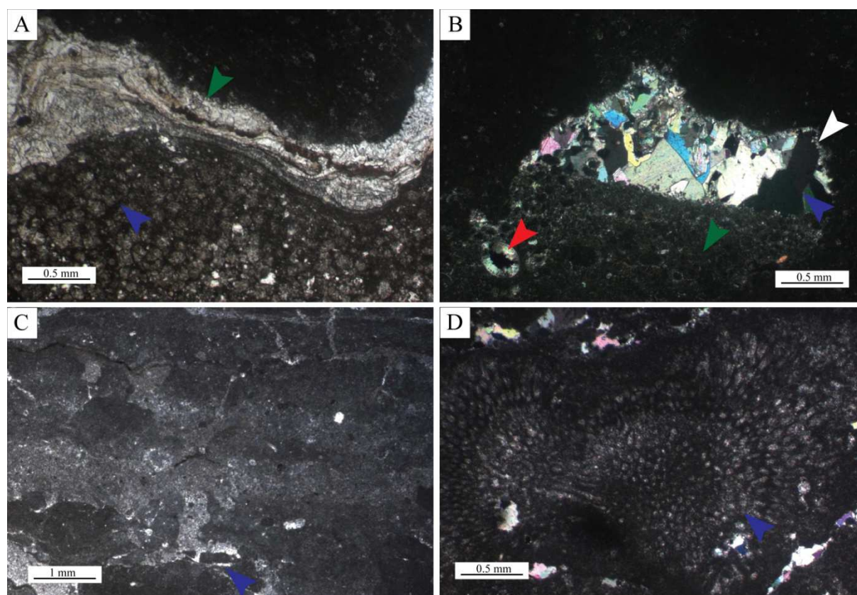
Figure 3.11: (A) [LN] Lamines microbiennes (flèche verte) et plage entièrement dolomitisée (flèche bleue), puis re-micritisée ; (B) [LPA] Faciès mudstone affecté de figures de dissolution partiellement remplies d'un sédiment plus jeune (flèche verte) constitué de peloïdes et ostracodes (flèche rouge). Une cimentation en scalénoèdre (flèche blanche) est attestée sur la bordure de la cavité, ainsi qu'une cimentation drusique occluant totalement la porosité ; (C) [LN] Indices de dessiccations dans un faciès micritique laminé ; (D) [LPA] Tissus algaires (flèche bleue) dans un faciès micritique.
