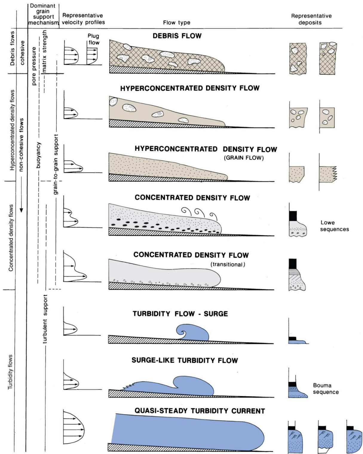
Figure 1.24: Classification des écoulements gravitaires, modifiée d'après Mulder & Alexander (2001).
