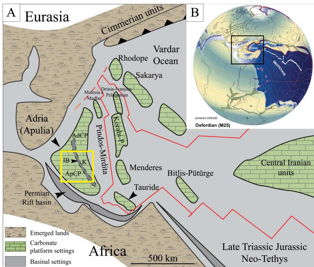
Figure 1.1: (A) Reconstitution paléogéographique de l'ensemble Téthysien au Jurassique Inférieur. La zone d'intérêt de cette étude est figurée dans le cadre jaune. Le développement du Jurassique au Crétacé du Bassin Ionien est indiqué en pointillés. Compilé d'après Degnan & Robertson (1998) et Robertson et al. (1991). (B) Modèle tectonique global au Jurassique Supérieur (Oxfordien) d'après Stampfli & Borel, 2002 avec l'emplacement de la zone représentée en (A) (cadre noir). Abréviations : Korabi P., Korabi – Pélagonien ; AdCP, Adriatic Carbonate Platform ; ApCP, Apulian Carbonate Platform ; IB, Ionian Basin ; K, Kruja.
