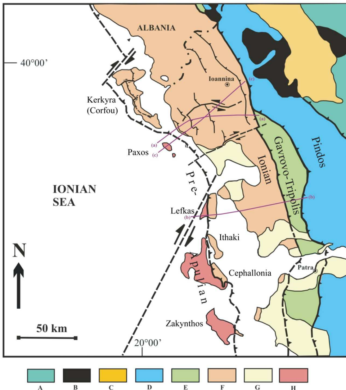
Figure 1.20: Carte géologique simplifiée de la Grèce occidentale. (A) Domaine Pelagonien, (B) Ophiolites, (C) Molasse Meso-hellénique, (D) Zone du Pinde, Italie Zone de Gavrovo-Tripolitza, (F) Zone Ionienne, (G) Néogène – Quaternaire, (H) Zone pre-Apulienne, d'après Karakitsios & Rigakis (2007).
