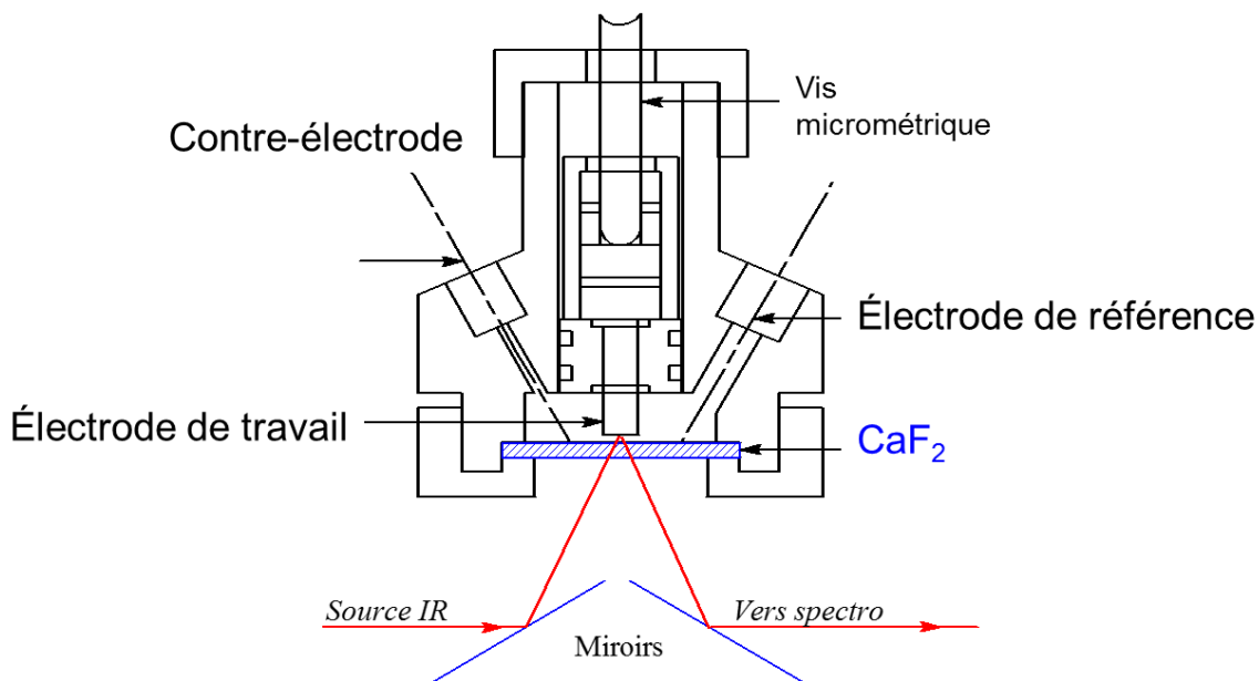
Figure 139 : Schéma d'une cellule de spectroélectrochimie.
