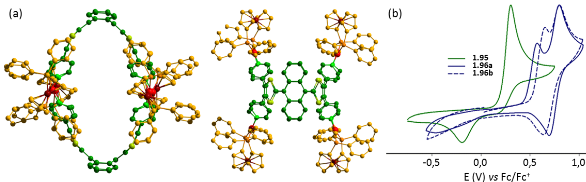
Figure 49 : (a) Structure RX de la cage M_4L_2 1.96a . Voltammogramme cyclique du ligand exTTF(4-Py)_4 1.95 ( C = 1 \text{ mM} , CH_3CN ( Bu_4NPF_6 ( 0,1 \text{ M} ), vitesse de balayage 100 \text{ mV}\cdot\text{s}^{-1} , Pt) et des cages M_4L_2 1.96a et 1.96b ( C = 1 \text{ mM} , CH_3CN ( n-Bu_4NPF_6 ( 0,1 \text{ M} ), vitesse de balayage 100 \text{ mV}\cdot\text{s}^{-1} , carbone vitreux). 225
