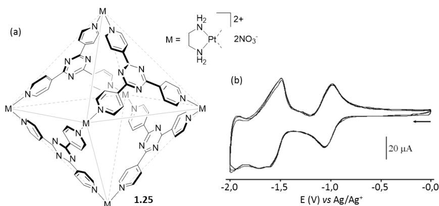
Figure 24 : (a) Structure de 1.25 et (b) voltammogramme cyclique de 1.25 : C = 0,5 mM, CH_3CN ( n-Bu_4NPF_6 (50 mM)), vitesse de balayage 100 mV.s^{-1} . 133
