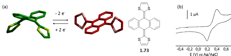
Figure 41 : Représentation schématique du changement de géométrie lors de l'oxydation à deux électrons de l'exTTF 1.73 . (b) Voltammogramme cyclique de 1.73 : CH_3CN ( n-Bu_4NClO_4 (0,1 M)), Pt, vitesse de balayage 100\text{ mV}\cdot\text{s}^{-1} . 204
