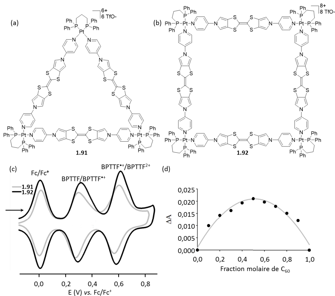
Figure 47 : (a) Triangle 1.91 et (b) carré 1.92 ; (c) Voltammogramme cyclique déconvolué de 1.91 et 1.92 en présence de ferrocène (3 et 4 éq. respectivement) : C = 0,5 mM dans CH 3 CN/CH 2 Cl 2 (Bu 4 NPF 6 (0,1 M)), Pt, vitesse de balayage 20 mV.s -1 , 221,222
