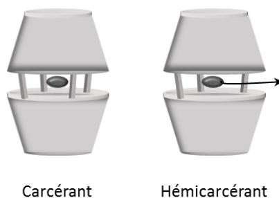
Figure 8 : Représentation schématique d'un carcérant et d'un hémicarcérant.
