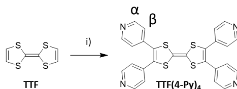
Schéma 19 : Synthèse du TTF(4-Py) 4 à partir de TTF. i) 4-iodopyridine, Pd(OAc) 2 , P( t -Bu) 3 ·HBF 4 , Cs 2 CO 3 , dioxane, reflux, 24h, 71%.
