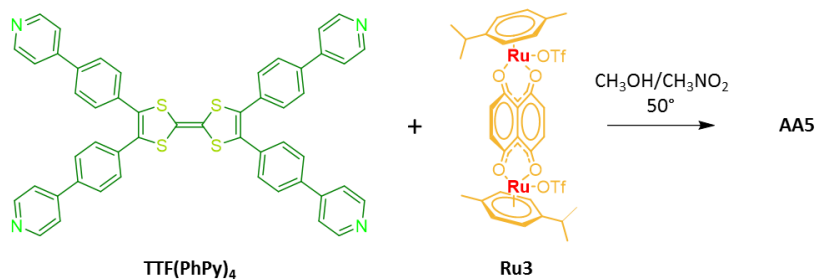
Schéma 23 : Assemblage entre le ligand TTF(PhPy) 4 et le complexe arène diruthénium Ru3 .
