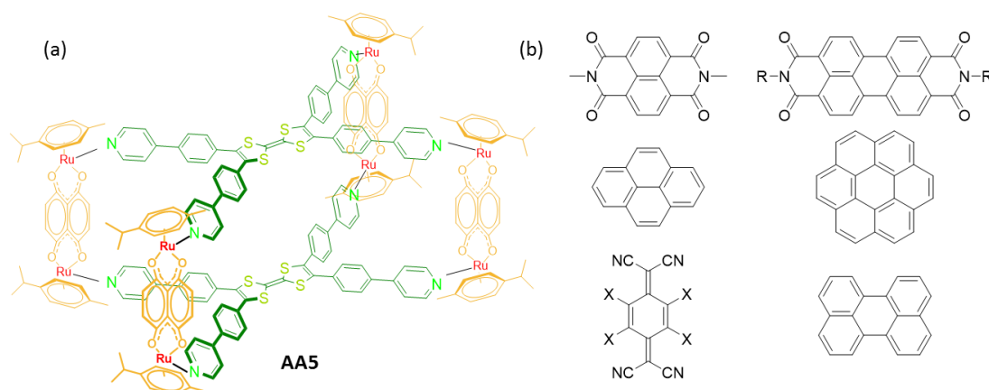
Figure 91 : (a) représentation de la cage AA5 ; (b) molécules planes testées : R = -\text{C}_5\text{H}_{11} ou 2,5-di- i Pr-benzène. X = \text{H} ou \text{F} .
