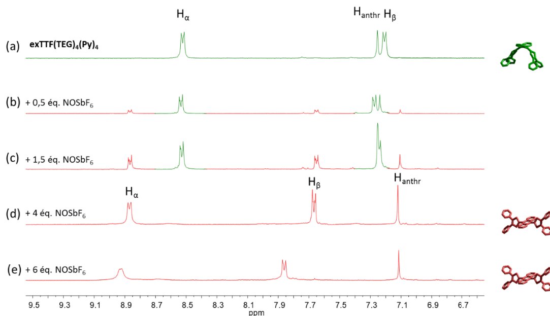
Figure 111 : Suivi RMN ^1\text{H} ( \text{CD}_3\text{CN} ) de l'oxydation progressive du ligand \text{exTTF(TEG)}_4(\text{Py})_4 ( C = 6,45 \cdot 10^{-3} \text{ mol}\cdot\text{L}^{-1} ) par une solution de \text{NOSbF}_6 ( C = 1,29 \text{ mol}\cdot\text{L}^{-1} ) : (a) ligand \text{exTTF(TEG)}_4(\text{Py})_4 , (b) 0,5 ; (c) 1,0 ; (d) 4,0 et (e) 6 équivalents de \text{NOSbF}_6 ajoutés.
