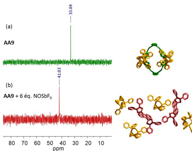
Figure 116 : Suivi RMN 31 P (CD 3 CN) de l'oxydation de la cage AA9 : (a) AA9 et (b) après ajout de 10 équivalents de NOSbF 6 .
