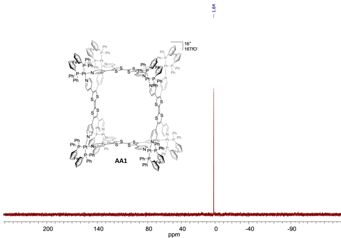
Figure 140 : RMN 31 P de AA1 (CD 3 NO 2 ).
