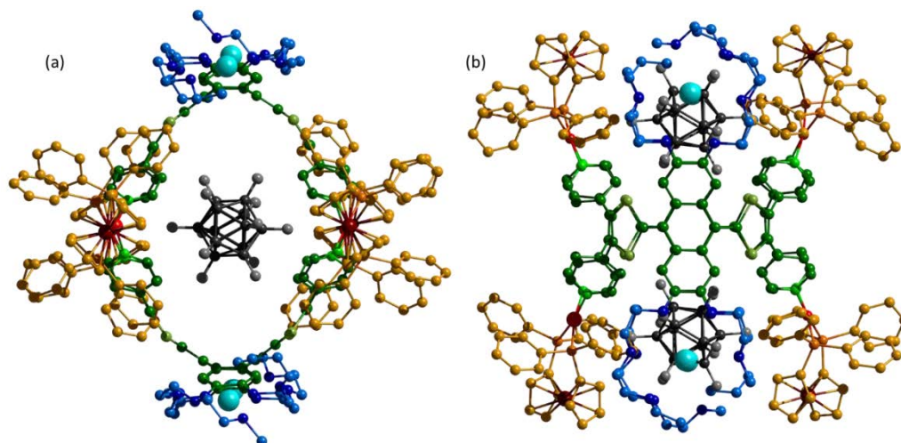
Figure 100 : Structure rayons-X de (B_{12}F_{12}^{2-})_2\text{-AA9} . (a) vue selon l'axe B_{12}F_{12} - B_{12}F_{12} et (b) vue de dessus.
