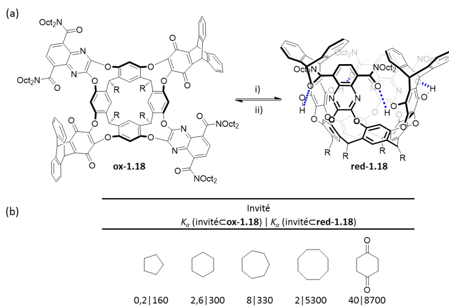
Figure 13 : (a) Changement de conformation d'un résorcin[4]arène-quinone, induit par réduction : i) H_2 , Pd/C, THF, 25°C, 3h, quantitatif ; ii) Air, CDCl_3 , quantitatif. (b) Constantes d'associations de ox-1.18 et red-1.18 envers différents invités. 45
