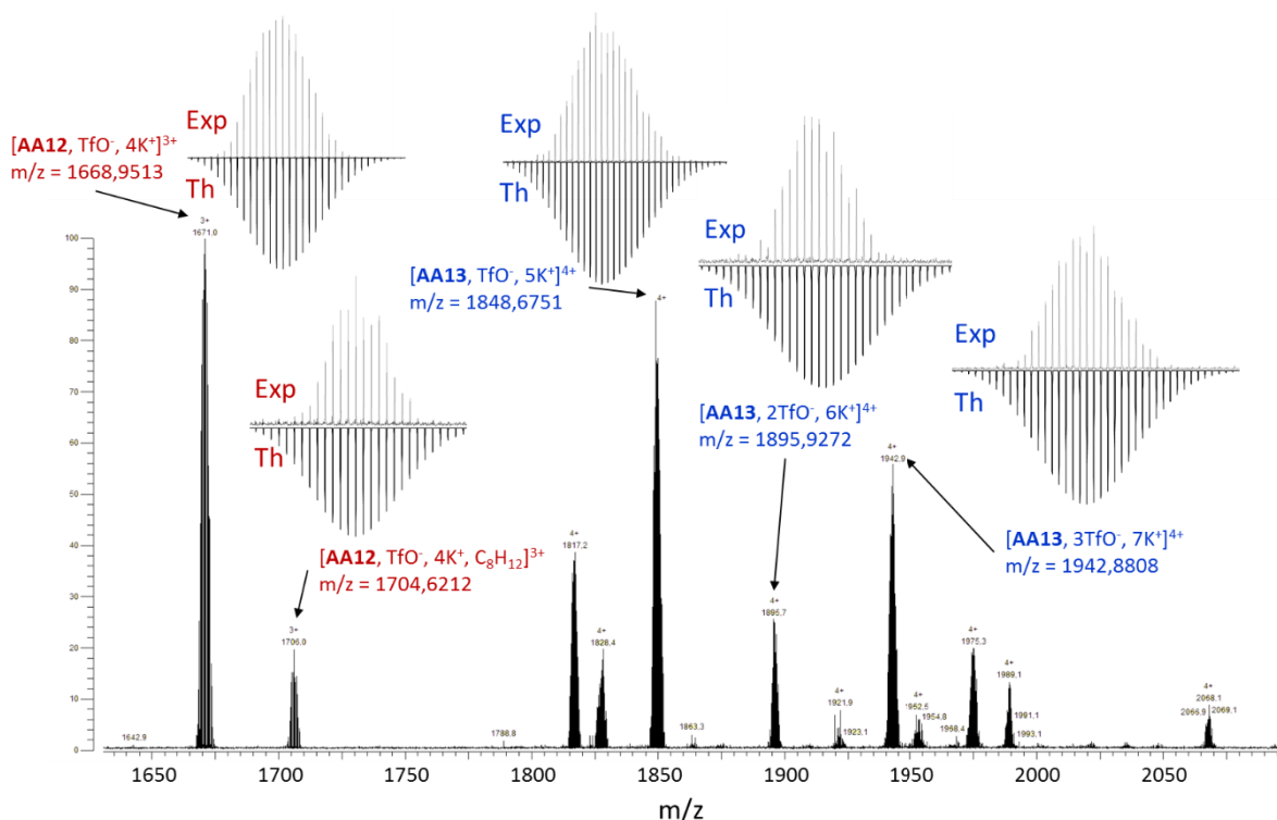
Figure 79 : Spectre de masse ESI-FTICR de AA12 et AA13 ( \text{CH}_2\text{Cl}_2/\text{CH}_3\text{CN} 5/2) en présence d'un excès de \text{KOTf} et les amas isotopiques théoriques et expérimentaux correspondants.
