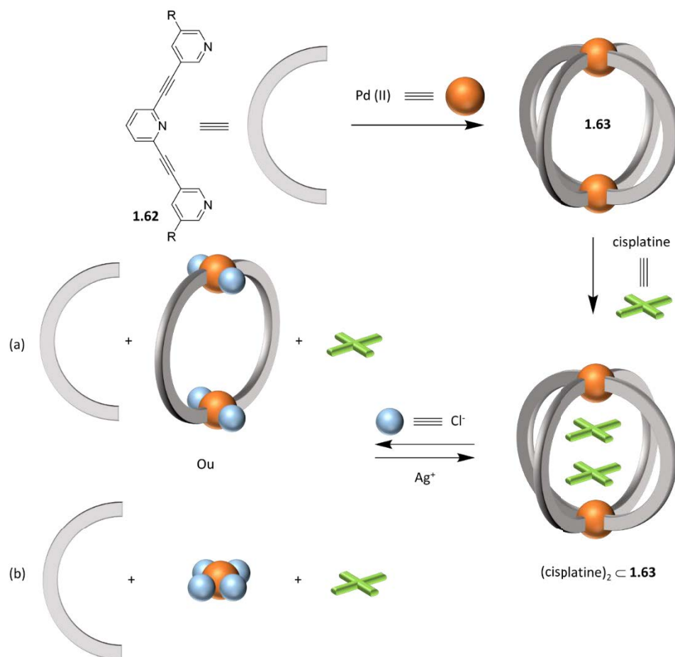
Figure 35 : Formation de la cage 1.63 à partir de Pd(II) et du ligand 1.62 ( R = H ou O(CH_2CH_2O)_2CH_3 ) puis libération de cisplatine par (a) désassemblage partiel ou (b) par désassemblage total. 165,166
