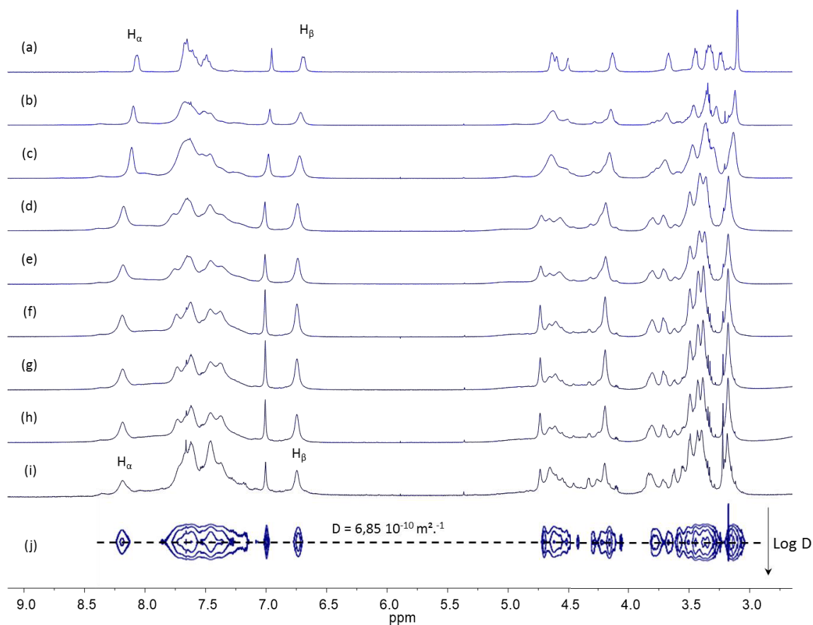
Figure 95 : Dosage de AA9 ( C = 8,4 \cdot 10^{-3} \text{ mol} \cdot \text{L}^{-1} ) par une solution de \text{K}_2\text{B}_{12}\text{F}_{12} , suivi par RMN ^1\text{H} ( \text{CD}_3\text{CN} ) : (a) cage AA9 ; (b) 0,5 ; (c) 1,0 ; (d) 1,5 ; (e) 2,0 ; (f) 2,5 ; (g) 3,0 ; (h) 3,5 ; (i) 4,0 équivalents de \text{K}_2\text{B}_{12}\text{F}_{12} ajoutés ; (j) RMN DOSY ^1\text{H} après l'ajout de 4 équivalents de \text{K}_2\text{B}_{12}\text{F}_{12} .
