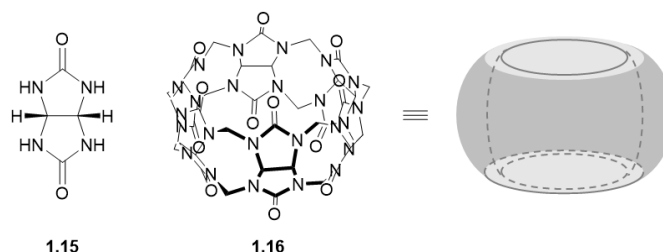
Figure 10 : Groupement glycolurile 1.15 permettant la synthèse des cucurbiturils CB[6] 1.16 .
