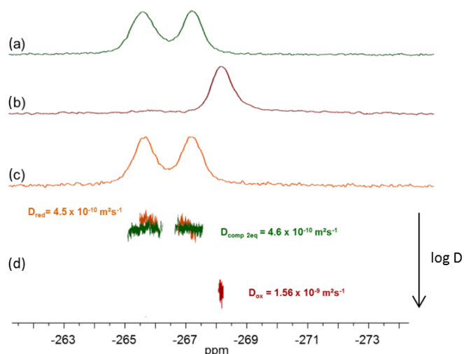
Figure 125 : Suivi RMN 19 F (CD 3 CN) de l'oxydation/réduction de B 12 F 12 2- - AA9 (C = 2,0 10 -3 mol.L -1 ) : (a) AA9 -(B 12 F 12 2- ) 2 , (b) après ajout de 4 équivalents de ThBF 4 , (c) après ajout de 2 équivalents de TDAE, et (d) RMN 19 F DOSY superposées correspondant à (a), (b) et (c).
