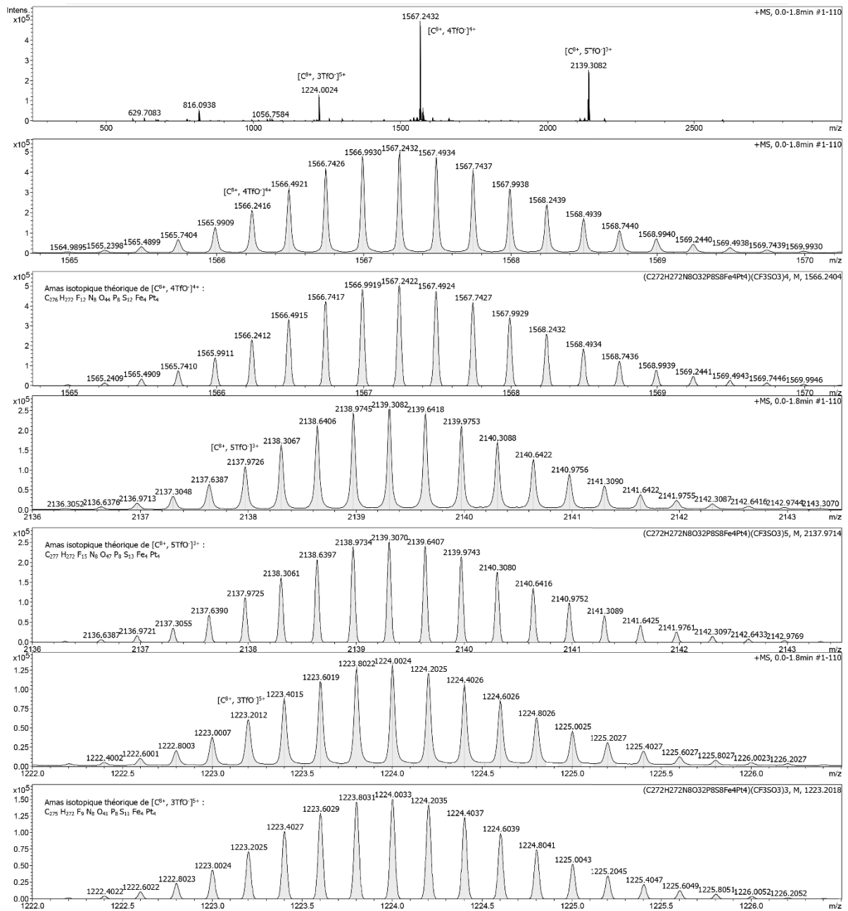
Figure 159 : Spectre de masse haute résolution ESI (Philippe Jéhant, CRMPO, Université de Rennes) de AA8.
