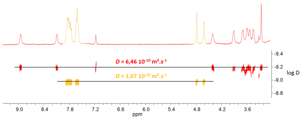
Figure 115 : RMN DOSY ^1\text{H} ( \text{CD}_3\text{CN} ) du mélange obtenu après l'ajout de 10 équivalents de \text{NOSbF}_6 sur AA9 .
