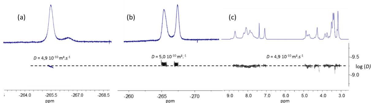
Figure 98 : (a) RMN DOSY ^{19}\text{F} ( \text{CD}_3\text{CN} ) d'un mélange AA9 / \text{K}_2\text{B}_{12}\text{F}_{12} 1/1, (b) RMN DOSY ^{19}\text{F} d'un mélange AA9 / \text{K}_2\text{B}_{12}\text{F}_{12} 1/2, RMN DOSY ^1\text{H} d'un mélange AA9 / \text{K}_2\text{B}_{12}\text{F}_{12} 1/2.
