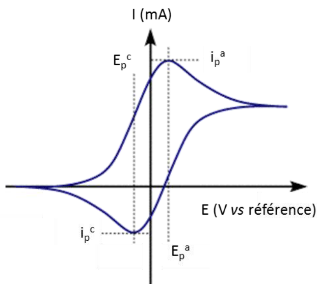
Figure 135 : Voltammogramme cyclique réversible.
