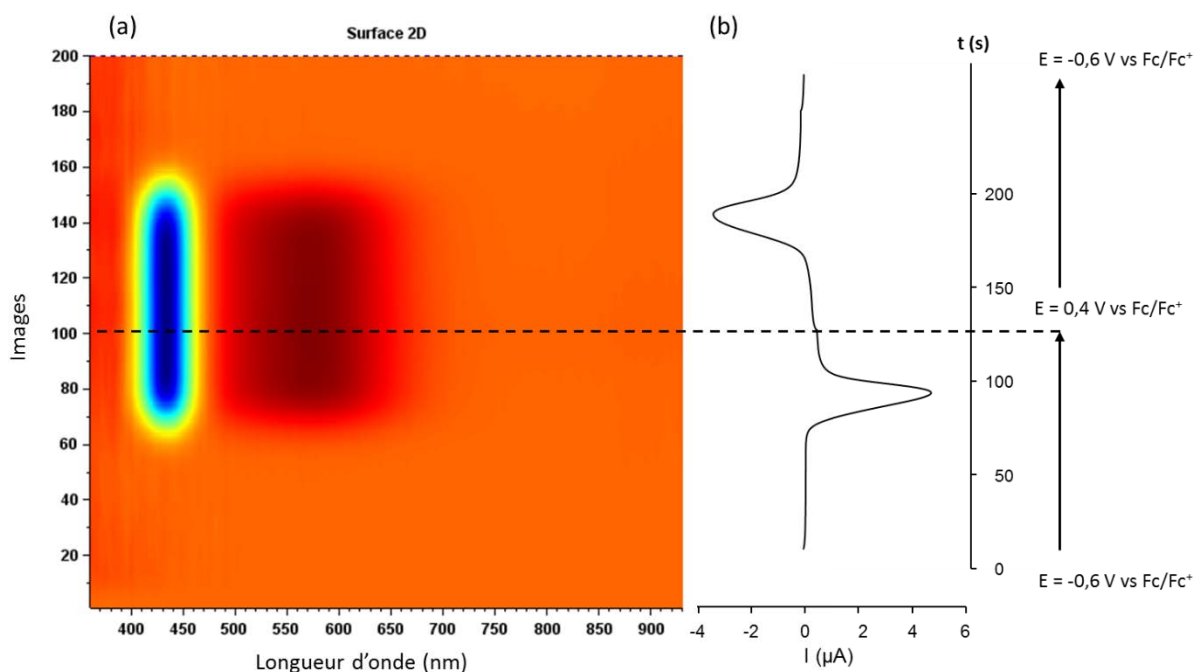
Figure 105 : Études spectroélectrochimiques du ligand \text{exTTF(TEG)}_4(\text{Py})_4 : (a) Représentation 2D des images collectées au cours du temps ; (b) Voltammogramme cyclique résolu dans le temps, C = 10^{-3} \text{ M} , \text{CH}_3\text{CN} ( n\text{-Bu}_4\text{NPF}_6 C = 0,1 \text{ M} ), 10 \text{ mV}\cdot\text{s}^{-1} , carbone vitreux, vs \text{Fc}/\text{Fc}^+ . La ligne en tirets noirs représente l'inversion du potentiel.
