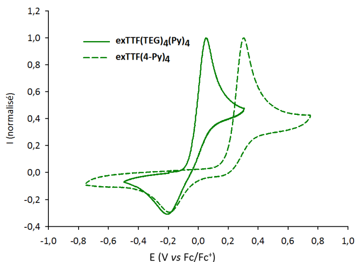
Figure 73 : Voltammogrammes cycliques de exTTF(TEG)_4(Py)_4 ( CH_3CN ) et de exTTF(4-Py)_4 ( CH_3CN/CH_2Cl_2 , 1/1) ; C = 1 mM, ( n-Bu_4NPF_6 (0,1 M)), 100 mV \cdot s^{-1} , carbone vitreux, V vs. Fc/Fc + .
