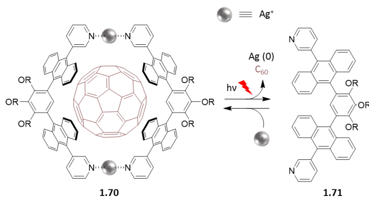
Schéma 15 : Relargage de C_{60} par désassemblage de la cage 1.70 ( R = -CH_2CH_2OCH_3 ) par irradiation UV-vis, puis réassemblage par ajout de sel de Ag(I) . 173
