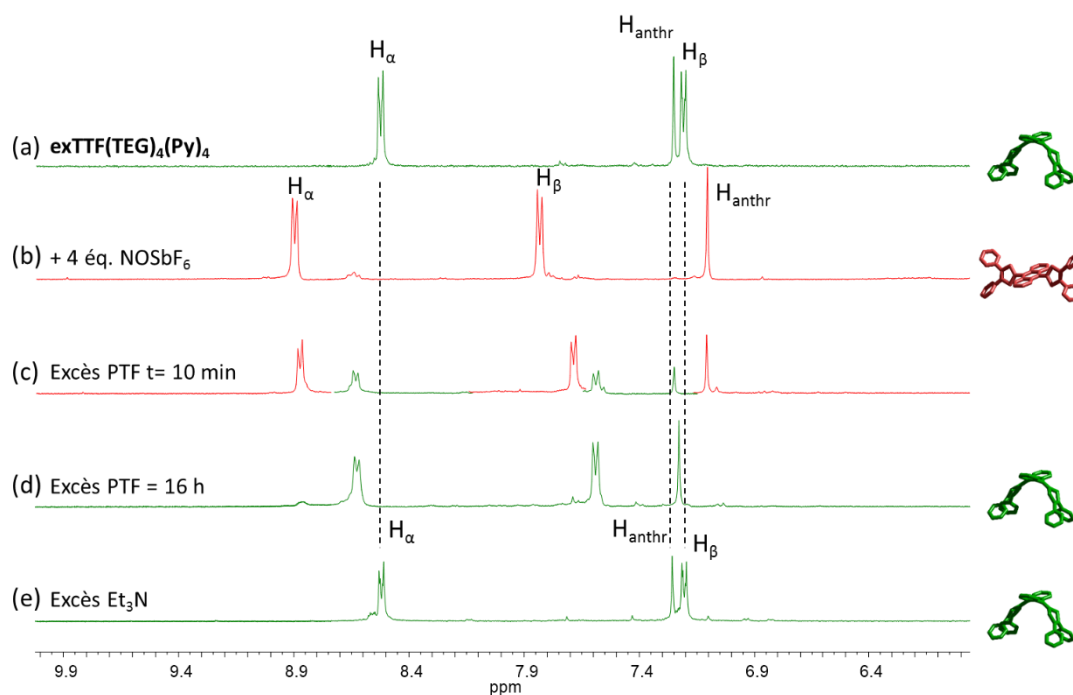
Figure 113 : Suivi RMN ^1\text{H} ( \text{CD}_3\text{CN} ) de l'oxydation puis réduction du ligand \text{exTTF(TEG)}_4(\text{Py})_4 : (a) \text{exTTF(TEG)}_4(\text{Py})_4 , (b) 4 équivalents de \text{NOSbF}_6 ajoutés, (c) 10 minutes après l'ajout d'un large excès de PTF ajouté, (d) après 16h à TA et (e) après l'ajout d'un excès de triéthylamine.
