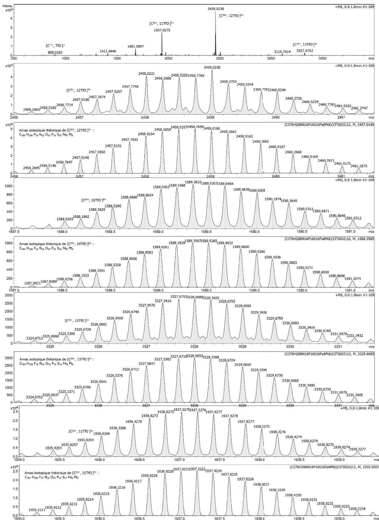
Figure 154 : Spectre de masse haute résolution ESI (Philippe Jéhan, CRMPO, Université de Rennes) de AA1.
