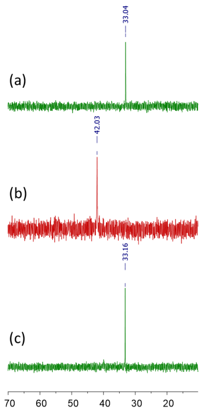
Figure 150 : Suivi RMN ^{31}\text{P} de l'oxydation et de la réduction de la cage AA9. (a) AA9, (b) après l'ajout de 4 éq. de \text{NOSbF}_6 et (c) après l'ajout d'un excès de PTF.
