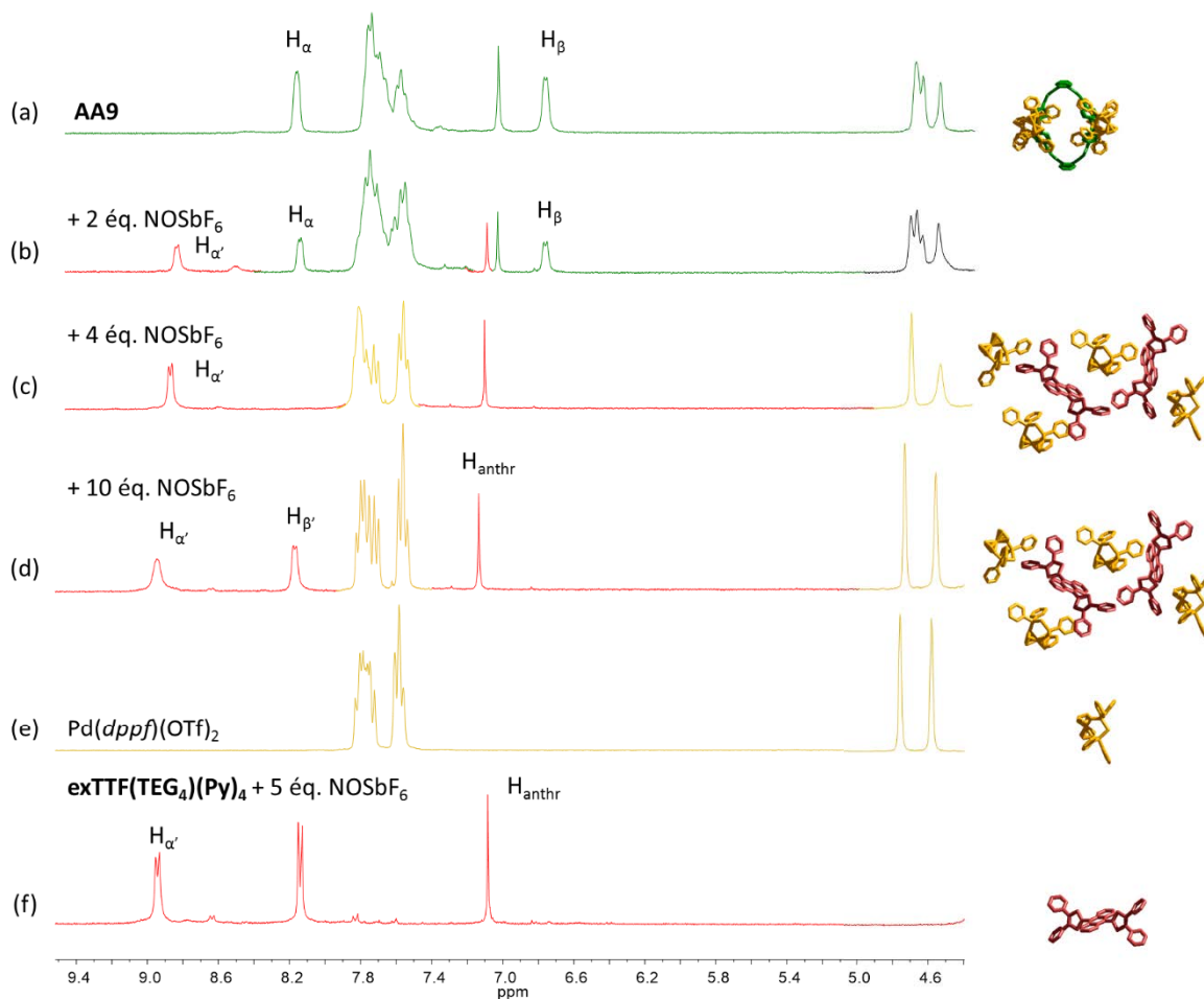
Figure 114 : Suivi RMN ^1\text{H} ( \text{CD}_3\text{CN} ) de l'oxydation de la cage AA9 ( C = 3,19 \cdot 10^{-3} \text{ mol.L}^{-1} ) par une solution de \text{NOSbF}_6 ( C = 1,28 \text{ mol.L}^{-1} ) : (a) AA9 , (b) 2 ; (c) 4 ; (d) 10 équivalents de \text{NOSbF}_6 ajoutés (e) \text{Pd}(\text{dppf})(\text{OTf})_2 et (f) exTTF(TEG) _4 (Py) _4 après ajout de 5 équivalents de \text{NOSbF}_6 .
