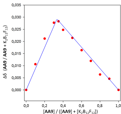
Figure 97 : Analyse de la courbe de Job de AA9 en présence de K_2B_{12}F_{12} déterminé par RMN ^1H ( AA9 H_\beta ) dans CD_3CN à 298 K, [AA9] + [K_2B_{12}F_{12}] = 5,0 \cdot 10^{-4} \text{ mol.L}^{-1} .
