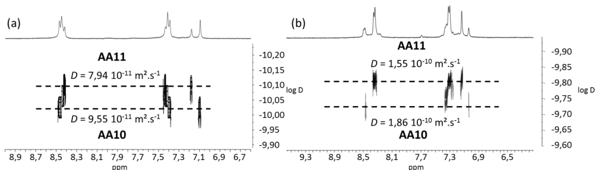
Figure 76 : RMN DOSY des assemblages formés dans (a) CD_3OD/D_2O 1 : 1 et (b) CD_3CN/D_2O 1 : 1 ; \delta (ppm, abscisse) vs. \log D (ordonnée).
