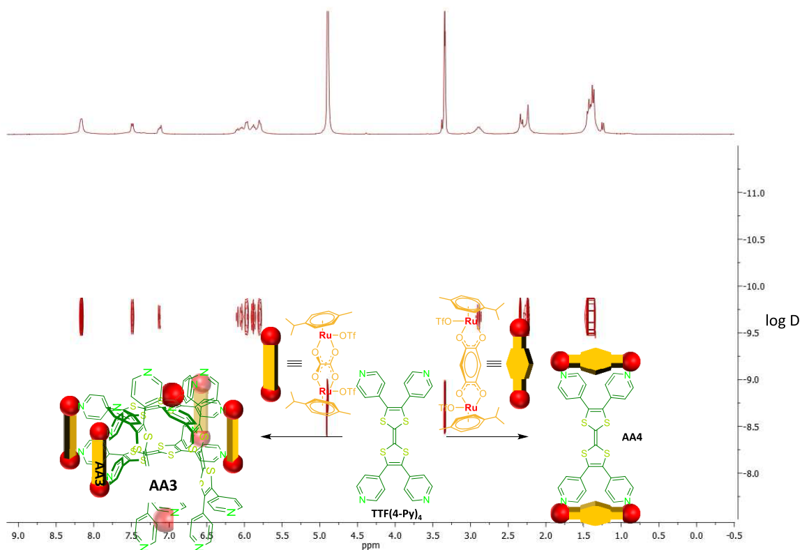
Figure 142 : RMN DOSY de AA3 (MeOD) : D = 2,14 \cdot 10^{-10} \text{ m}^2 \cdot \text{s}^{-1} .
