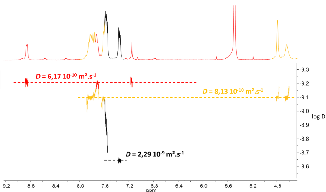
Figure 122 : RMN DOSY ^1\text{H} ( \text{CD}_3\text{CN} ) du mélange après oxydation de la cage AA9 avec 4 éq. de \text{Th}^{*\cdot} .
