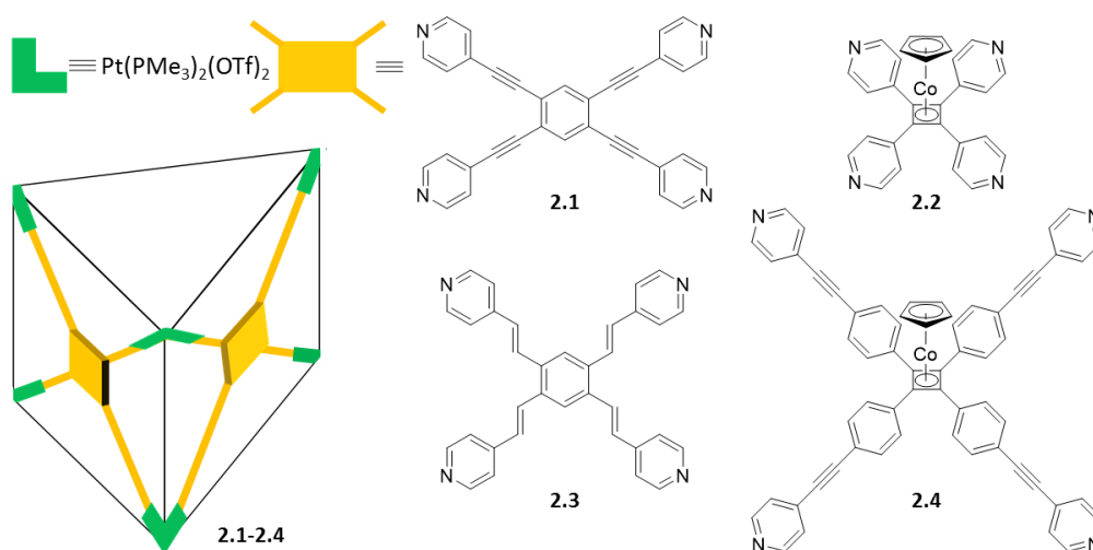
Figure 52 : Exemples de cages auto-assemblées 2.1-2.4 synthétisées à partir de ligands tétrapyridyles. 1,2
