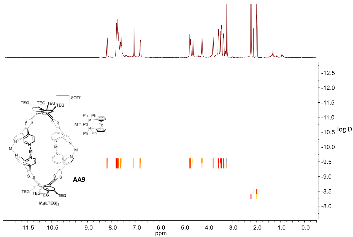
Figure 147 : RMN DOSY de AA9 ( CD_3CN ) : D = 4,9.10^{-10} m^2.s^{-1} .
