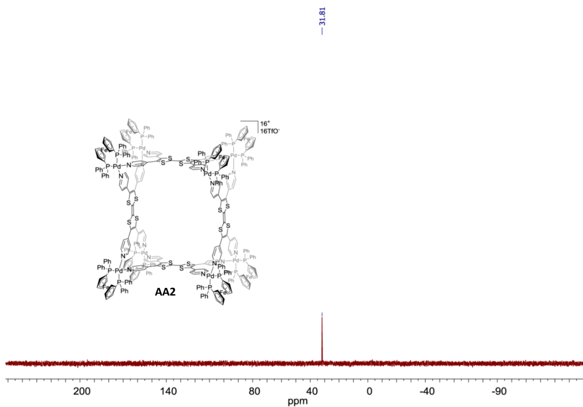
Figure 141 : RMN 31 P de AA2 (CD 3 NO 2 ).
