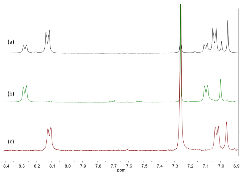
Figure 81 : Spectres RMN 1 H (CDCl 3 ) : (a) du mélange AA12 et AA13 ; (b) de AA13 (préparé dans le DMSO) et (c) AA12 (préparé dans l'acétone).
