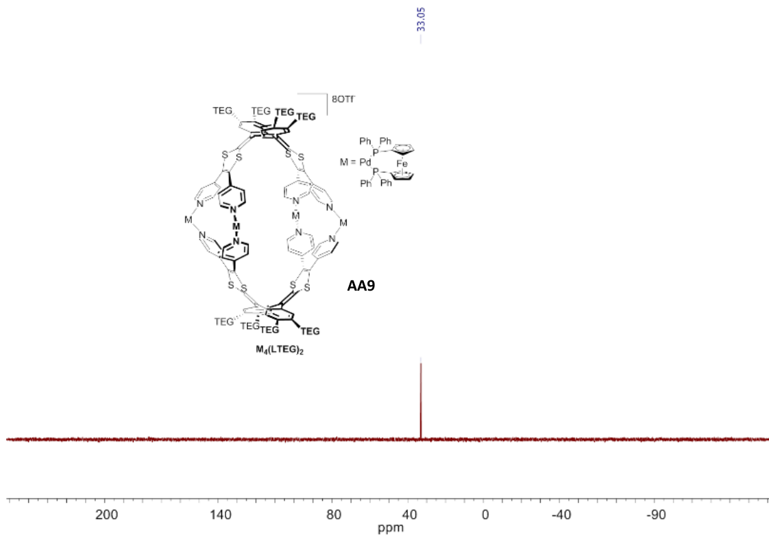
Figure 146 : RMN ^{31}P de AA9 ( CD_3CN ).
