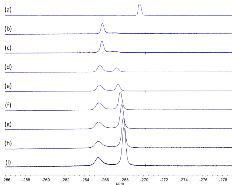
Figure 96 : Dosage de AA9 ( C = 8,4 \cdot 10^{-3} \text{ mol.L}^{-1} ) par une solution de K_2B_{12}F_{12} , suivi par RMN ^{19}F ( CD_3CN ) : (a) K_2B_{12}F_{12} libre ; (b) 0,5 ; (c) 1,0 ; (d) 1,5 ; (e) 2,0 ; (f) 2,5 ; (g) 3,0 ; (h) 3,5 ; (i) 4,0 équivalents de K_2B_{12}F_{12} ajoutés.
