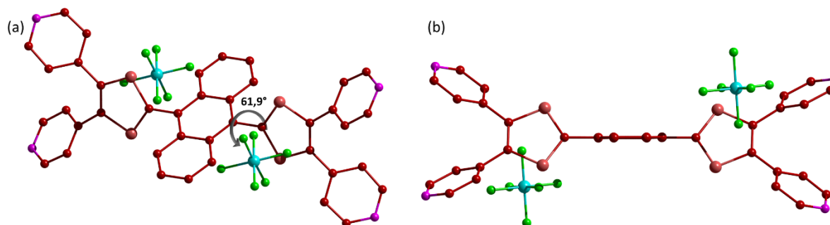
Figure 103 : Structure rayons X du ligand oxydé \text{exTTF(4-Py)}_4^{2+}(\text{PF}_6^-)_2 . (a) Vue en perspective (b) Vue perpendiculaire au plan de l'anthracène.
