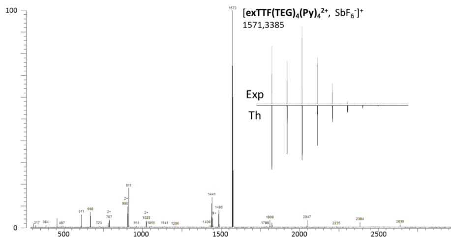
Figure 112 : Spectre de masse ESI-FTICR du ligand en présence de 10 équivalents de \text{NO}^+\text{SbF}_6^- ( \text{CH}_3\text{CN} , C = 10^{-3} \text{ mol.L}^{-1} ). Comparaison de l'amas isotopique expérimental (Exp) et théorique (Th).
