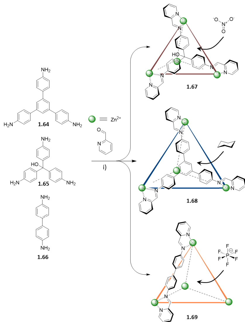
Schéma 14 : Auto-assemblages sélectifs de trois cages à partir de 5 composés. i) \text{CH}_3\text{CN} , 70^\circ\text{C} , 16h. 172
