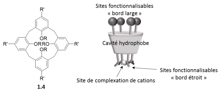
Figure 3 : Structure du calix[4]arène ( R=R'=H ) et représentation schématique de dérivés du du calix[4]arène (cas de la conformation cône).
