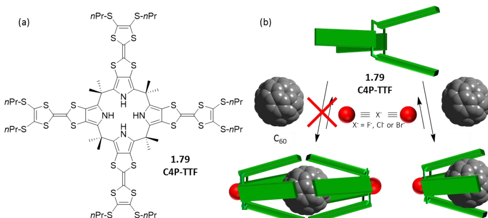
Figure 40 : (a) structure du TTF-C4P 1.79 et (b) représentation schématique de la complexation du \text{C}_{60} dans la cavité formée par \text{X}^- . 1.79 . 201, 202, 203
