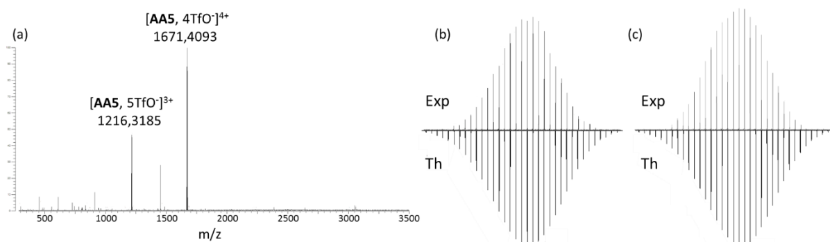
Figure 63 : (a) Spectre de masse FTICR de \text{AA5} correspondant à une stœchiométrie \text{M}_8\text{L}_2 ; Corrélation entre les massifs isotopiques expérimentaux et théoriques de (b) [\text{AA5}, 5\text{TfO}]^{3+} et (c) [\text{AA5}, 4\text{TfO}]^{4+} .
