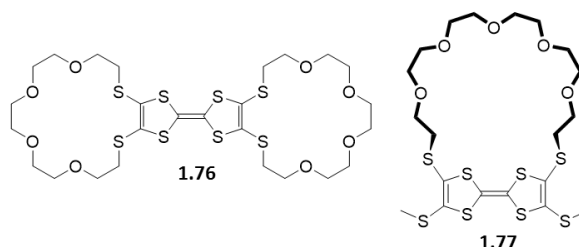
Figure 38 : Exemples de dérivés TTF éthers couronnes, 1.76 197 et 1.77 . 198,199
