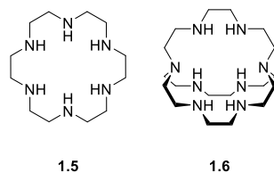
Figure 4 : Structure de l'hexacyclène 1.5 et du octaazacryptant 1.6 .
