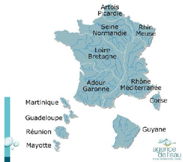
Figure 4 : Les 12 bassins hydrographiques en France.
