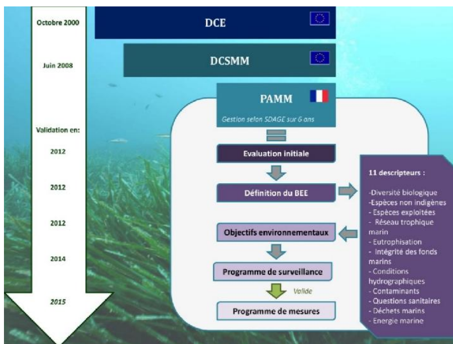
Figure 6 : Schéma récapitulatif des cinq étapes du PAMM (Plan d'Action pour le Milieu Marin).
