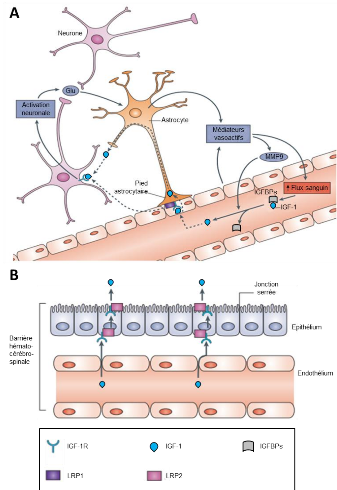
Figure 16 : Mécanismes d'entrée de l'IGF-1 périphérique dans le cerveau. A : Représentation de l'entrée d'IGF-1 par la BHE. L'activité neuronale induit la libération de médiateurs vasoactifs qui activent la MMP9. Cette protéase clive les IGFBPs sanguines, libérant localement l'IGF-1. En se fixant à son récepteur, l'IGF-1 est internalisé et mis à disposition des cellules neuronales. B : Représentation de l'entrée d'IGF-1 par la barrière hémato-cérébro-spinale. L'IGF-1 en se fixant sur son récepteur induit l'activation de la LRP2 qui permet la transcytose de l'IGF-1 et sa diffusion dans le LCR. Adapté de Fernandez et Torres-Alemán 2012.
