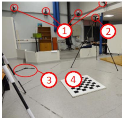
Figure 11 Système de Motion Capture jumelé à un capteur RGBD.
