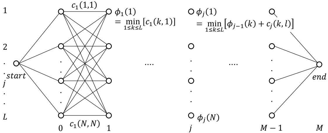
Figure 19 Treillis entièrement connecté de N Etats.
