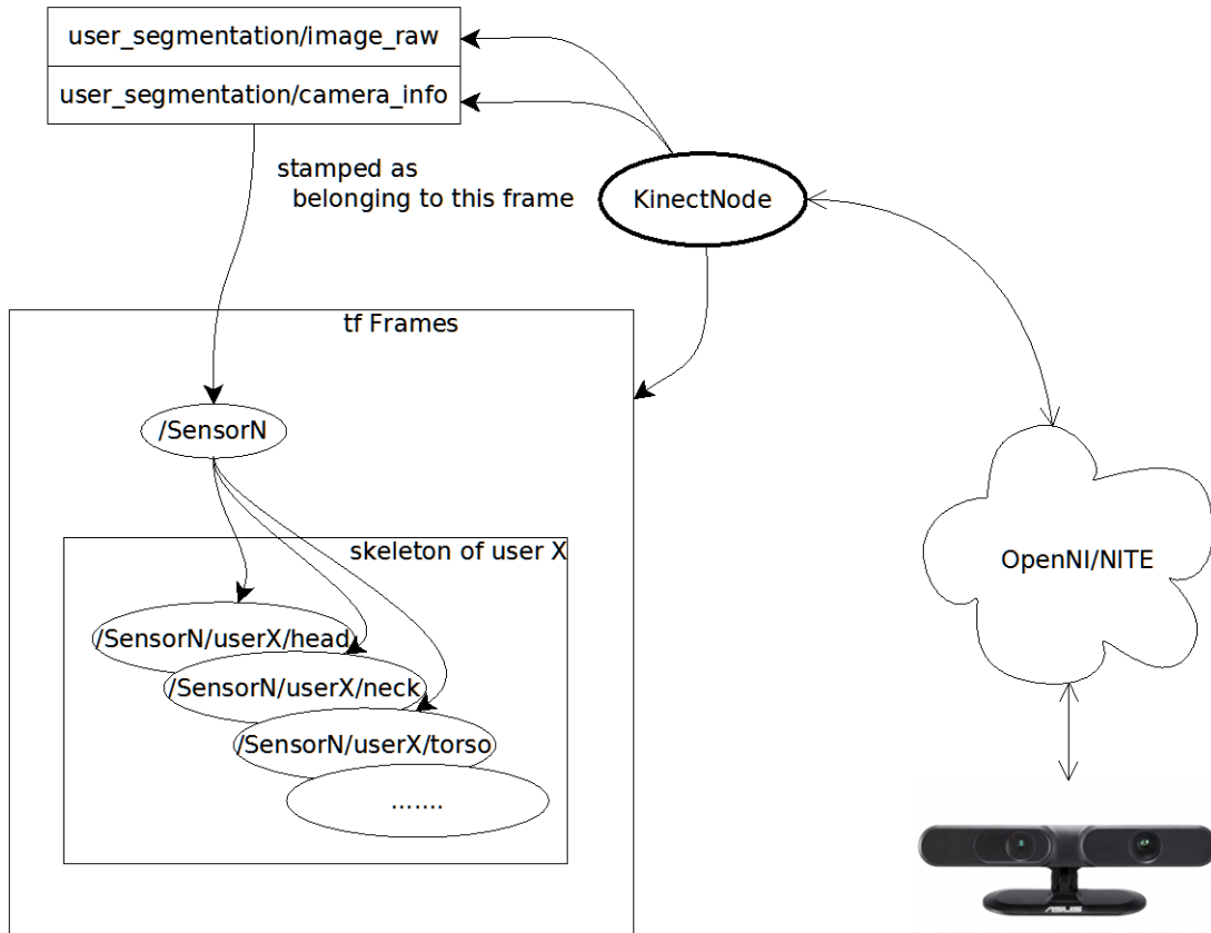
Figure 45 Schéma de communication de KinectNode .
