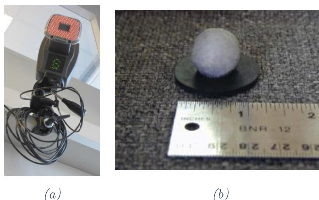
Figure 13 Gros plan sur une caméra infrarouge et le réseau de LEDs de la Motion Capture (a), et d'un marqueur (b).
