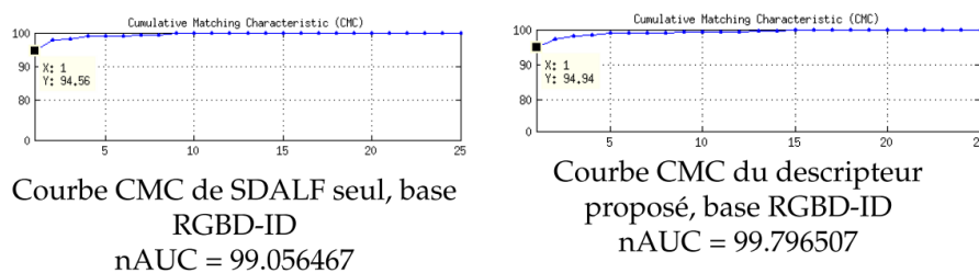
Figure 47 Courbes Cumulative Matching Curve sur dataset ETHZ1 (Leibe, Schindler, & Van Gool, 2007) de méthode de réidentification proposé par G. Marion (Stage 2014).
