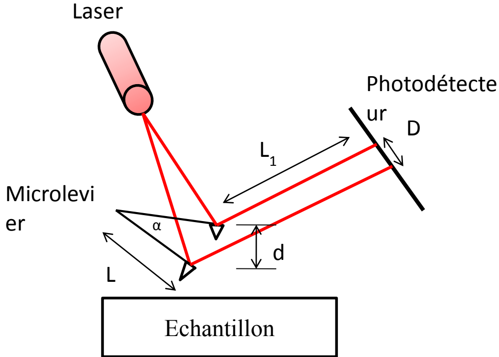
Figure 8 : Schéma représentant la relation entre la déflexion du miroir suivant la direction z et le déplacement D du faisceau laser sur le photodétecteur
