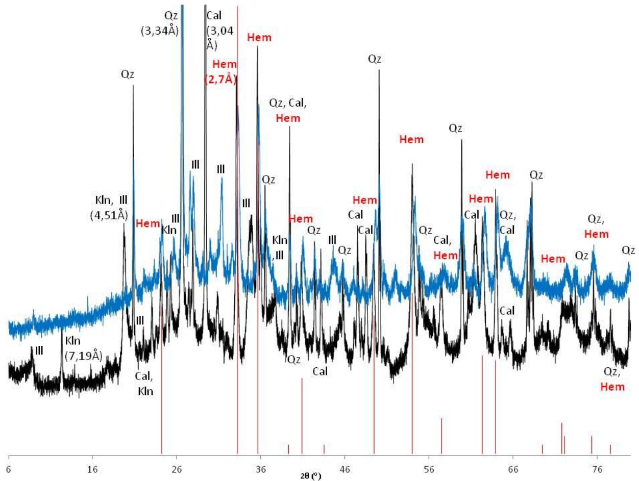
Figure 40 : Diffractogrammes de rayons X du résidu de thermo-analyse de l'échantillon 317. La courbe noire représente la poudre utilisée avant les travaux d'analyse et la courbe bleue représente le résidu de la chauffe (1000°C) effectuée sous une atmosphère d'argon. Les mêmes phases minéralogiques sont présentes sur les deux diffractogrammes : Quartz (Qz) et hématite (Hem), sauf pour la kaolinite (Kln), calcite (Cal) et l'illite (Ill). Les traits verticaux rouges représentent l'hématite standard.
