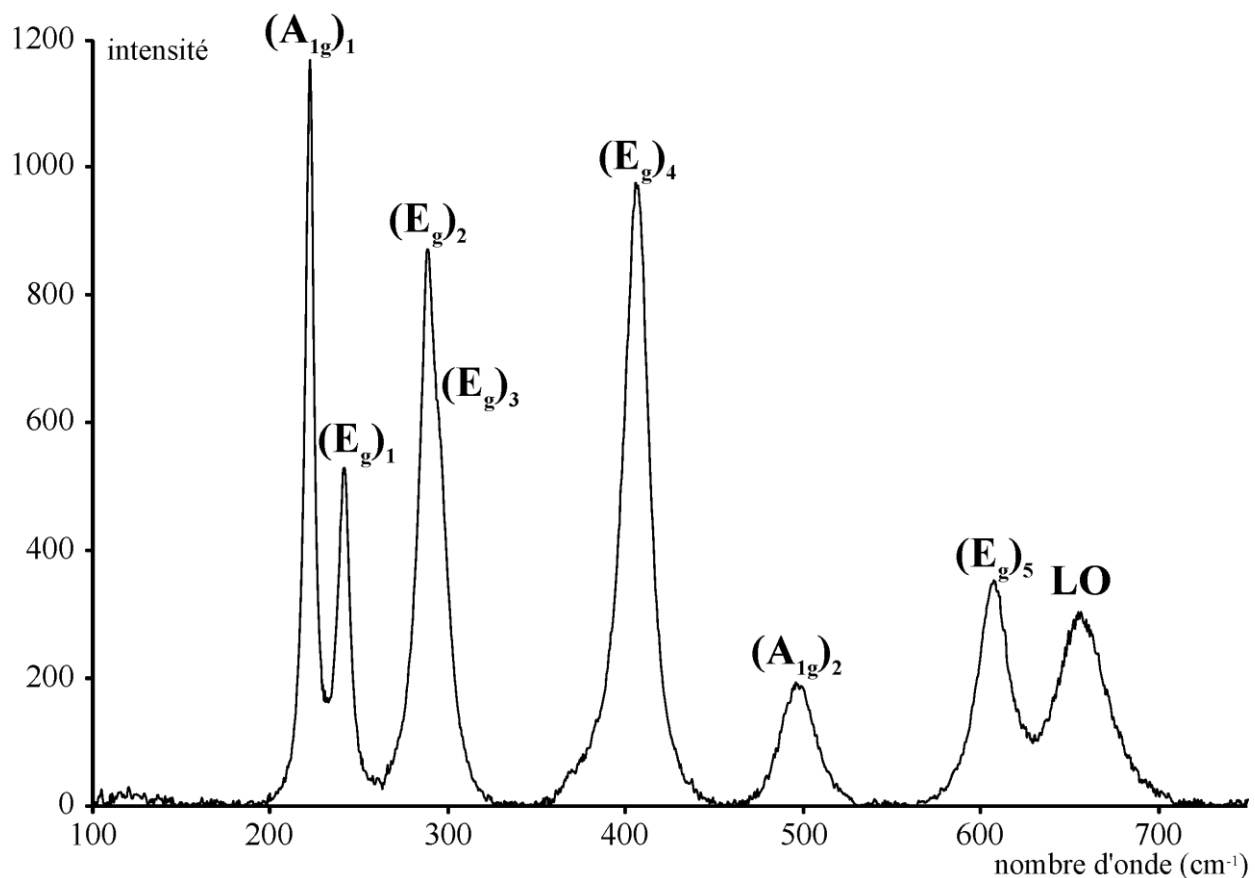
Figure 18 : spectre Raman d'une hématisation (spéculaire) avec l'attribution des pics (échantillon E09_05_10, Kiggavik).
