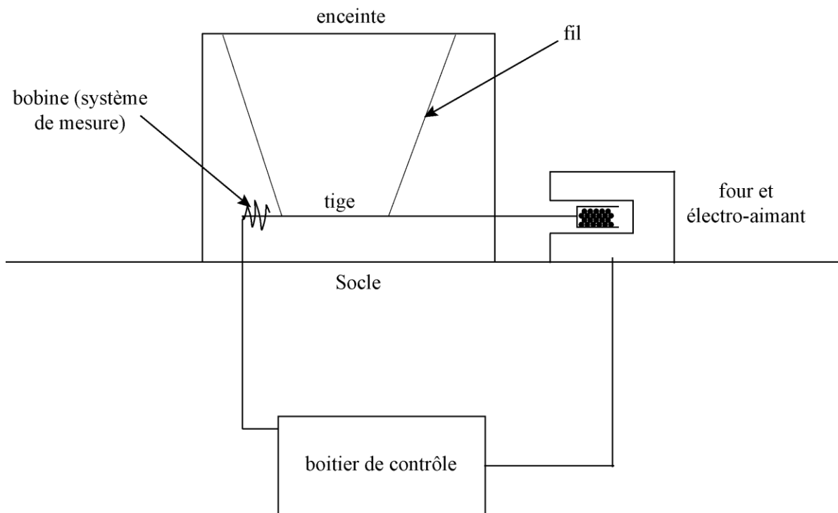
Figure 6 : Schéma de la balance de Curie.
