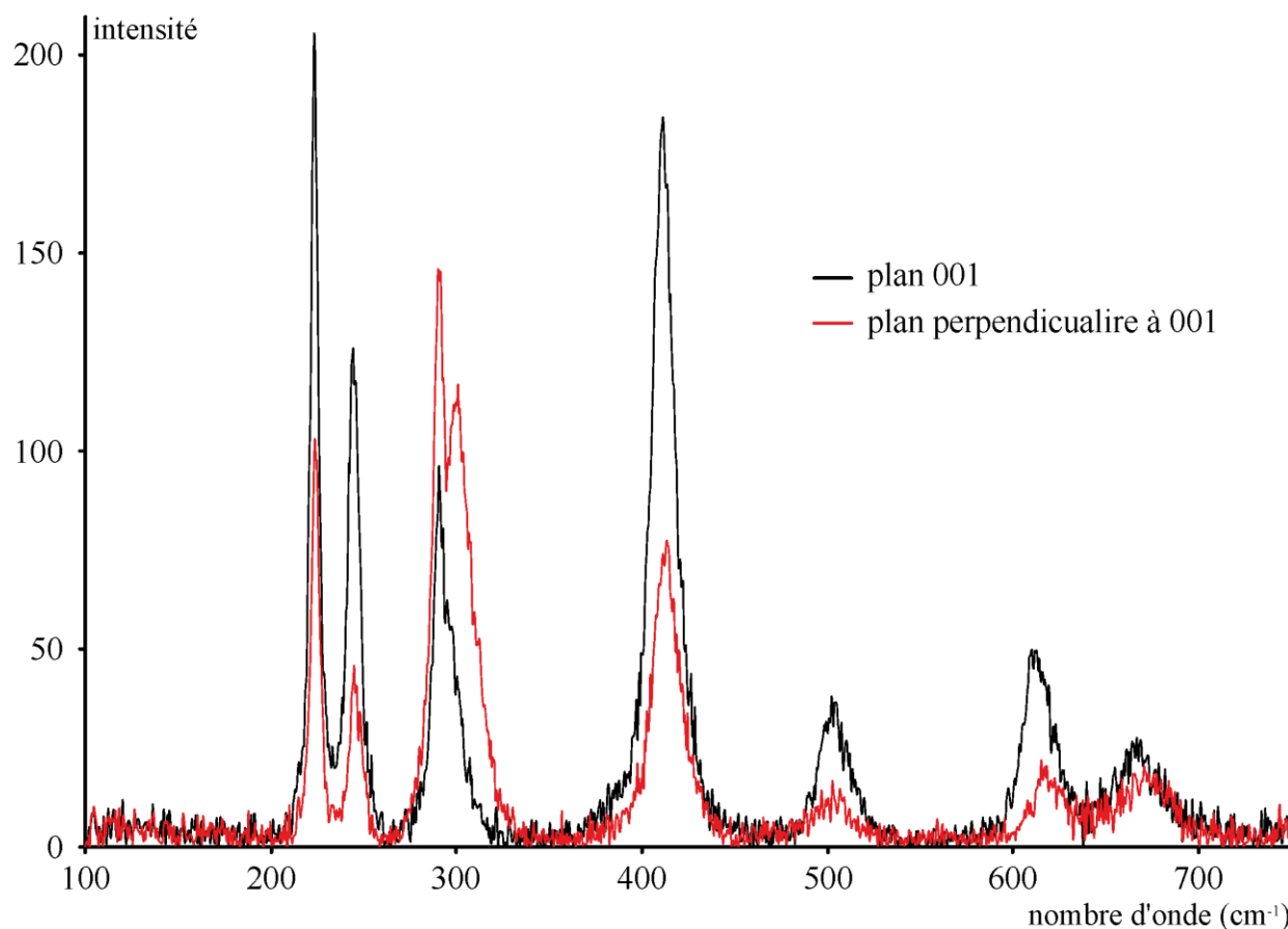
Figure 21 : exemple de spectres Raman sur l'hématite spéculaire (Kiggavik), le spectre noir représente une analyse sur le plan 001 d'une hématite et le spectre rouge sur un plan perpendiculaire a un plan 001.
