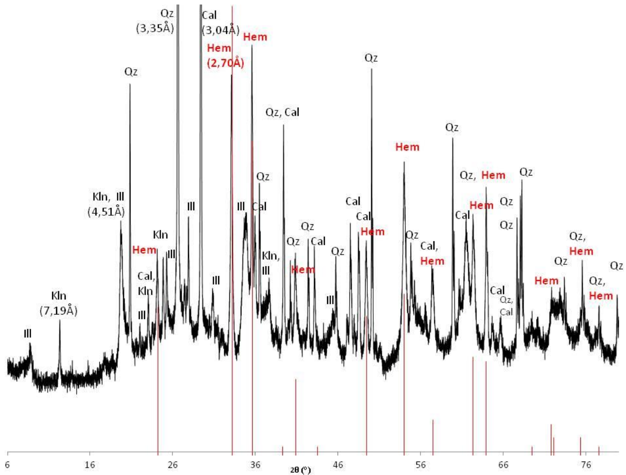
Figure 36 : Diffractogramme de rayons X de l'échantillon 317. La courbe noire représente le résultat de la diffraction de rayons X sur la partie rouge de l'échantillon, préalablement trié de manière granulométrique (entre 100 et 200 \mu\text{m} ) et magnétique (partie magnétique). Cette courbe indique la présence de quartz (Qz), calcite (Cal), kaolinite (Kln), illite (Ill) et d'hématite (Hem). Les traits verticaux rouges représentent l'hématite standard.
