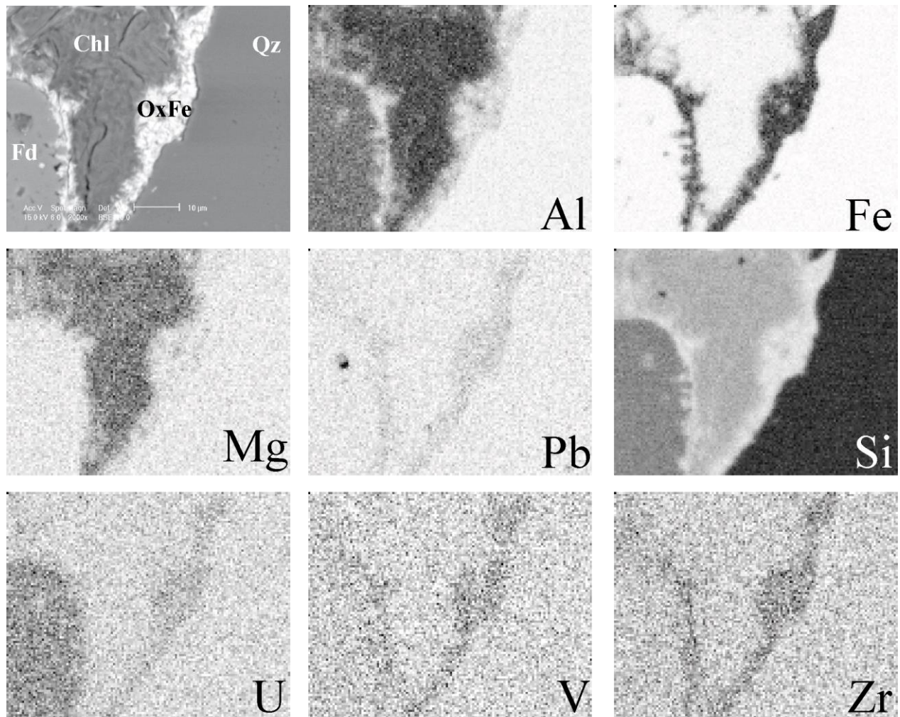
Figure 12 : Cartographie élémentaire de la zone à oxy-hydroxyde de fer de l'échantillon 105 composée de quartz (Qz), feldspath (Fd), chlorite (Chl) et d'oxy-hydroxyde de fer (OxFe) au MEB EDS. Image MEB (en électrons rétrodiffusées) et répartition de l'aluminium (Al), fer (Fe), magnésium (Mg), plomb (Pb), silice (Si), uranium (U) vanadium (V) et zirconium (Zr). Remarque le feldspath ne contient pas d'uranium, c'est le potassium qui une raie à la même place que l'uranium.
