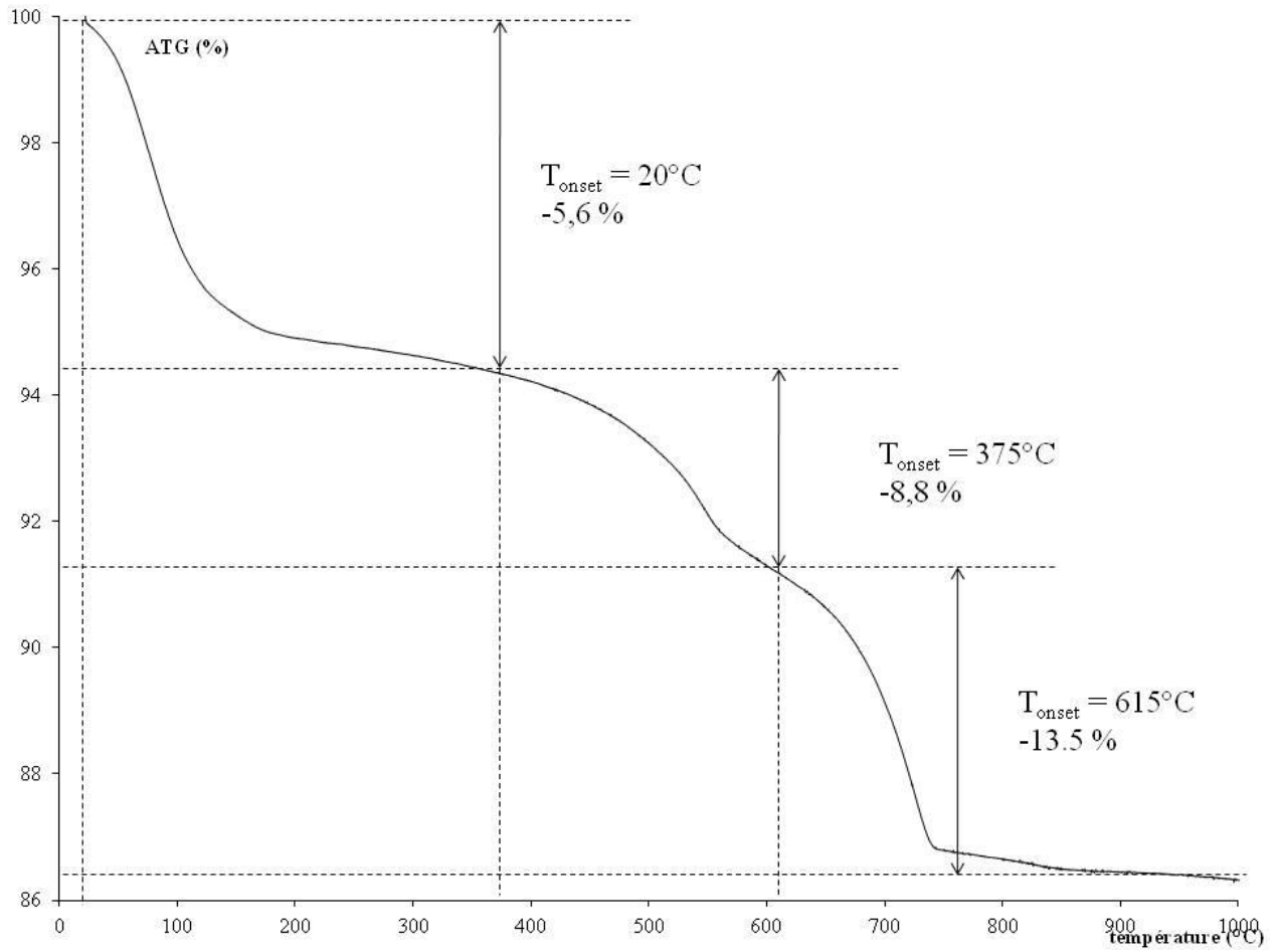
Figure 30 : Thermogramme ATG de l'échantillon 317 sous une atmosphère d'Ar, avec les températures de début de perte de poids ( T_{onset} ) et les pertes de masse associées (en %).
