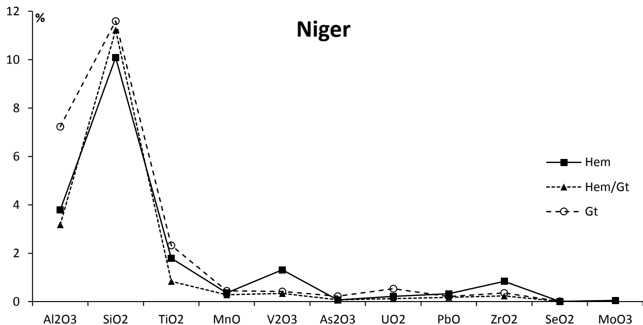
Figure 23 : Diagramme des moyennes des éléments en traces dans les goethites et hématites des fronts rédox minéralisés du gisement d'Ebba.
