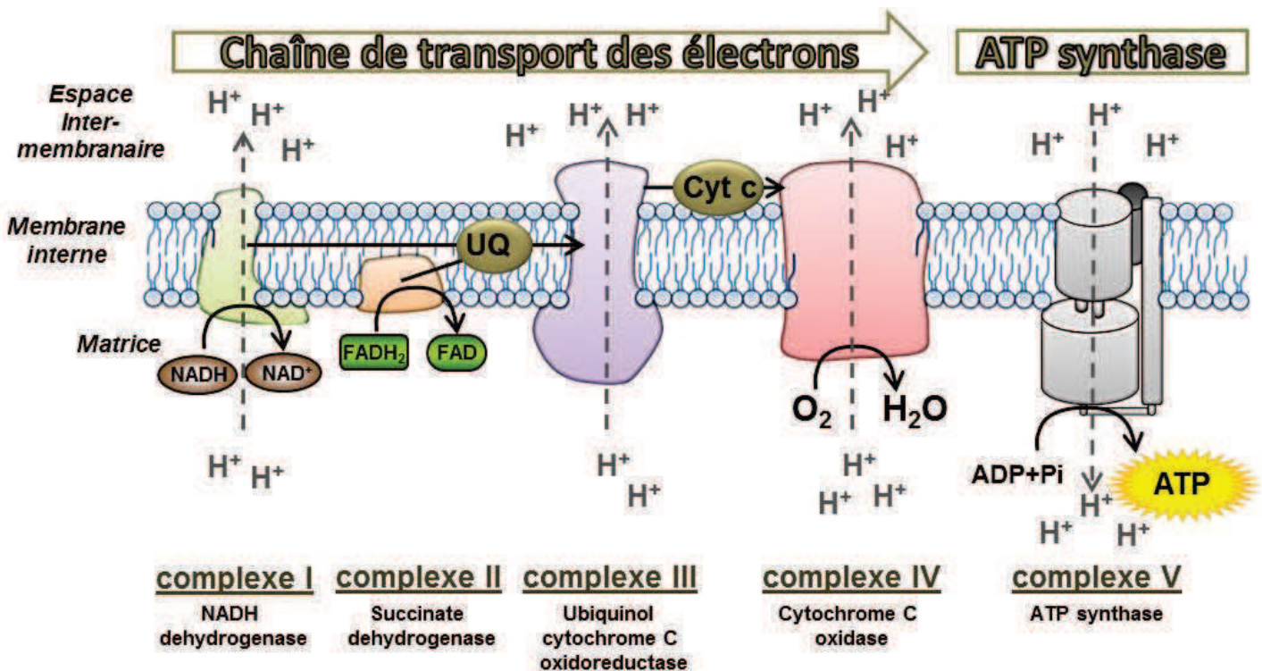
Fig. 2: Bioénergétique de la chaîne de transport d'électrons. Après le cycle de Krebs, le NADH généré est transféré au complexe I et converti en NAD + . Le transfert d'électrons à travers la chaîne maintient le potentiel de membrane mitochondriale en pompant des protons de la matrice vers l'espace intermembranaire. Au final, l'ADP est phosphorylée pour former l'ATP par le complexe V (ATP synthase). UQ; coenzyme Q, Cyt c; cytochrome c (adapté de (5) et (6)).
