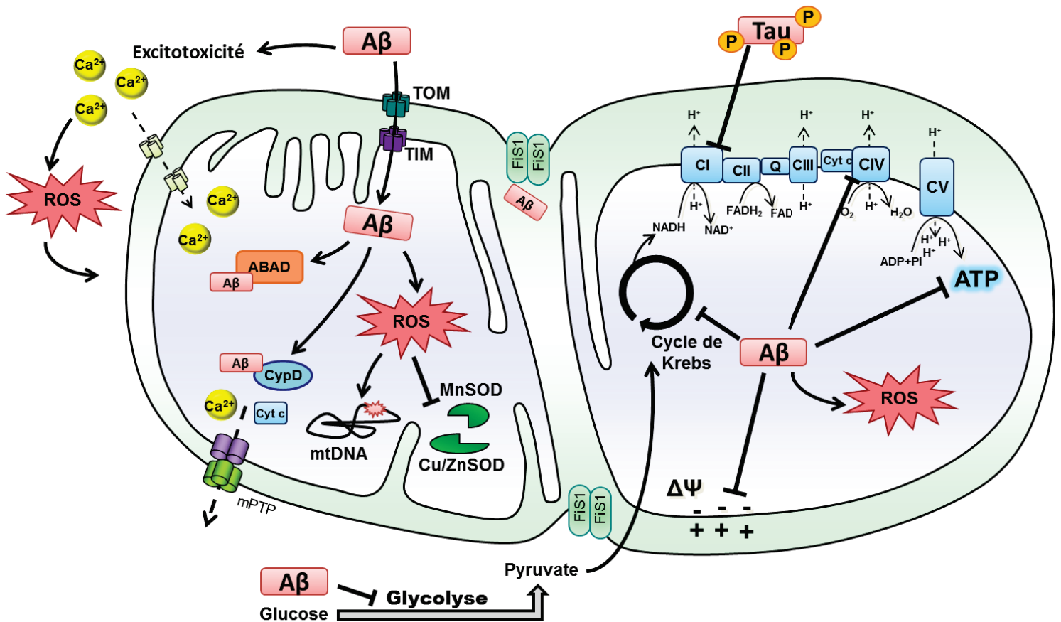
Fig. 3 : Convergence pathogène de la protéine tau hyperphosphorylée et le peptide A \beta sur les mitochondries. A \beta et la protéine tau sont capables d'altérer la respiration mitochondriale en inhibant le complexe IV et complexe I respectivement. Ceci induit une diminution de la consommation d'oxygène, de la production d'ATP et une augmentation des niveaux de ROS. Le stress oxydant induit par le dysfonctionnement de la chaîne de transport des électrons peut surpasser les défenses antioxydantes des cellules (MnSOD, Cu/ZnSOD) et impacter le potentiel de membrane ( \Delta\Psi ) ainsi que l'ADN mitochondrial (mtDNA). Dans les mitochondries, le peptide A \beta peut se lier à des protéines comme l'ABAD et CypD, ce qui génère plus de ROS et mène à l'ouverture des pores de transition de perméabilité mitochondriale (mPTP), déclenchant les voies apoptotiques par la libération de Cyt C dans le cytosol. En parallèle, le peptide A \beta peut également être responsable des altérations métaboliques en inhibant les enzymes impliquées dans la glycolyse et du cycle de Krebs, de même que l'excitotoxicité induite par le calcium dans les neurones. Enfin, l'A \beta et la protéine tau peuvent perturber l'activité de fusion / fission mitochondriale, conduisant à une mauvaise répartition des mitochondries dans les neurones. C1 complexe I, CII complexe II, CIII complexe III, CIV complexe IV, CV complexe V, cyt c cytochrome c, Cu/Zn SOD cuivre/zinc superoxyde dismutase, MnSOD manganèse superoxyde dismutase, ROS espèces réactives de l'oxygène, mtDNA ADN mitochondrial, TOM / TIM translocases des membranes mitochondriales interne / externe, ABAD A \beta binding alcohol dehydrogenase, FIS, protéine fission 1, CypD cyclophiline D (adapté de (26) et (22)).
