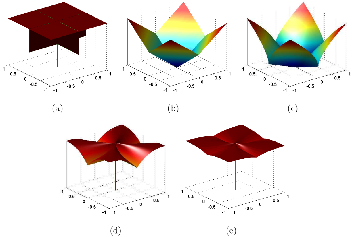
Figure 6.11 – (a) Fonction \ell_0 . (b) Fonction \ell_1 . (c) Fonction \ell_{1/2} . (d) Fonction \ell_{1,\alpha}/\ell_{2,\eta} . (e) Fonction h_2 = \log\left(\frac{\ell_{1,\alpha} + \beta}{\ell_{2,\eta}}\right) .
