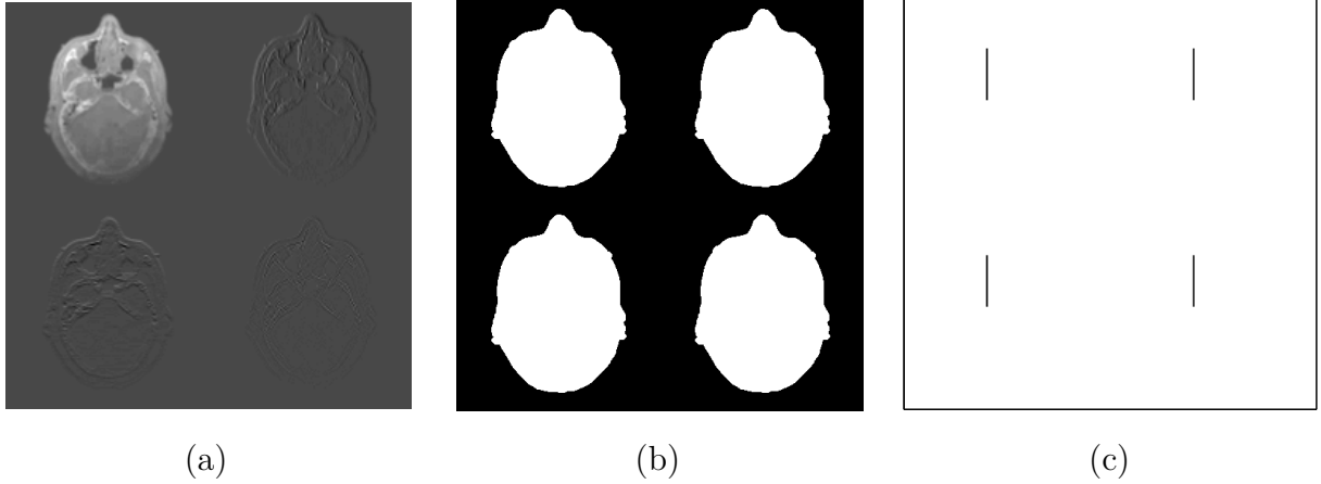
Figure 6.7 – Seuls les coefficients de trame correspondants à la partie réelle de l'image \overline{\mathbf{y}}_{\mathcal{R}} sont représentés dans les trois figures. (a) Exemple de décomposition de trame de \overline{\mathbf{y}}_{\mathcal{R}} . (b) Masque \mathbb{E} permettant de forcer les coefficients de l'arrière plan de l'objet à être égaux à 0. (c) Indices d'un bloc \mathbf{x}^{(j)} pour Q = 32 .
