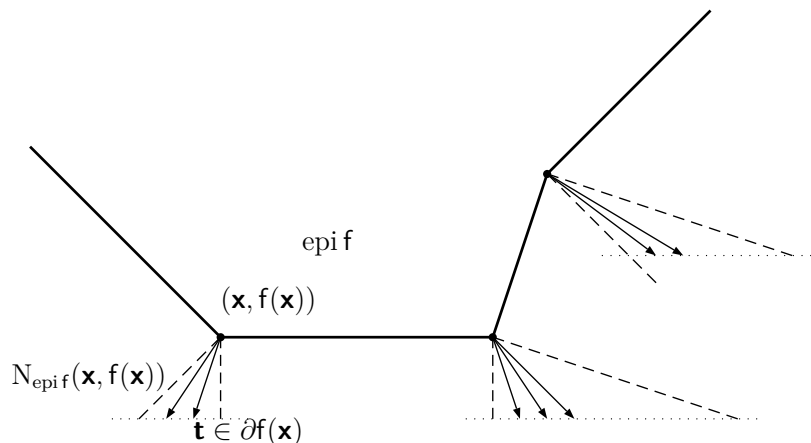
Figure 2.9 – Cônes normaux de l'épigraphe d'une fonction f: \mathbb{R} \rightarrow ]-\infty, +\infty] .
