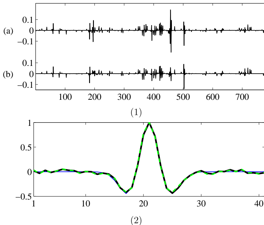
Figure 6.13 – (1) Erreur résiduelle \bar{\mathbf{x}} - \hat{\mathbf{x}} pour le signal estimé \hat{\mathbf{x}} obtenu en utilisant [Krishnan et al. , 2011] (a) et l’algorithme 6.2 (b). (2) Noyau original \bar{\mathbf{k}} (ligne fine continue bleue), estimé \hat{\mathbf{k}} par l’algorithme 6.2 (ligne épaisse continue noire) et par [Krishnan et al. , 2011] (ligne discontinue épaisse verte).
