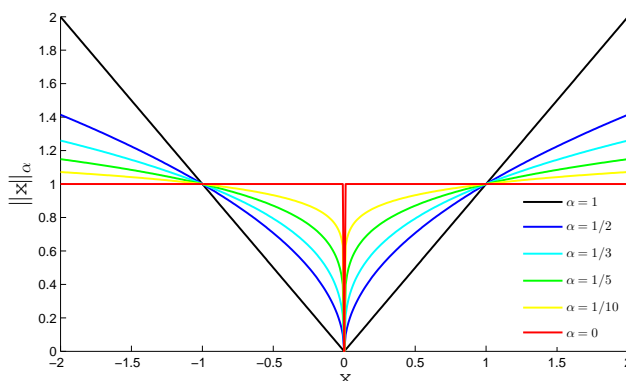
Figure 2.3 – Fonctions \ell_\alpha pour \alpha \in \{0, 1/10, 1/5, 1/3, 1/2, 1\} .
