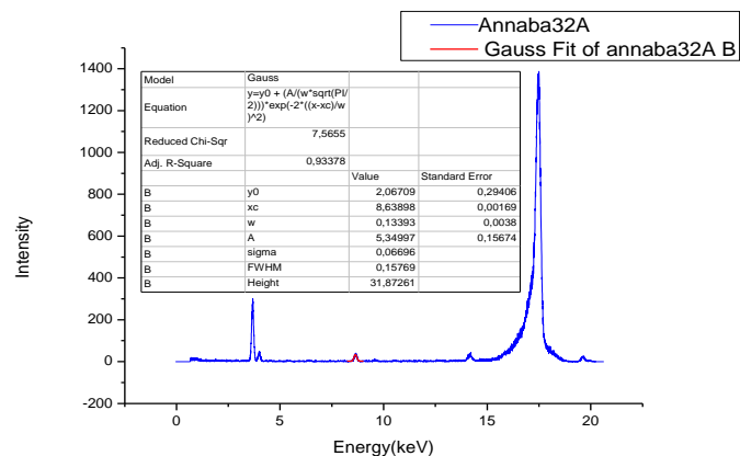
Figure 9. Montage classique pour la fluorescence X localisé au LPS et spectre de fluorescence X tracé sous le logiciel Origine
