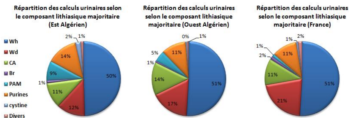
Figure 1: la répartition des calculs urinaires selon le composant lithiasique majoritaire, Wh : whewellite ; Wd : weddellite ; CA : carbapatite ; Br : brushite ; PAM : phosphate ammoniaco-magnésien ; Purines : acides uriques et urates.
