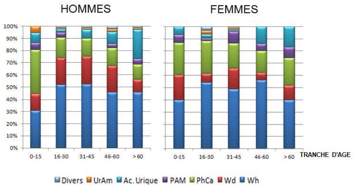
Figure 2. Composition des calculs en fonction de l'âge, sur une série de 1354 calculs provenant des services d'urologie de l'Ouest Algérien [56].
