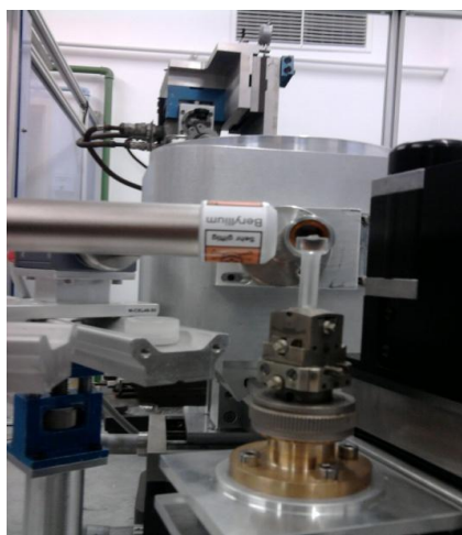
Figure 9. Montage classique pour la fluorescence X localisé au LPS et spectre de fluorescence X tracé sous le logiciel Origine
