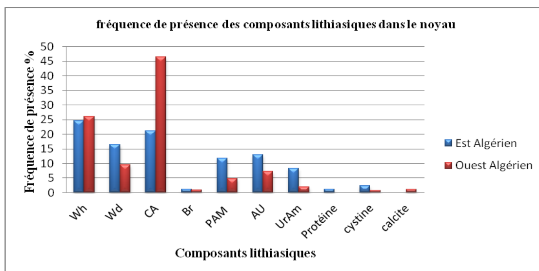
Figure 3. Fréquence des composants lithiasiques dans le noyau pour des calculs urinaires provenant de l'Est et de l'Ouest Algérien.
