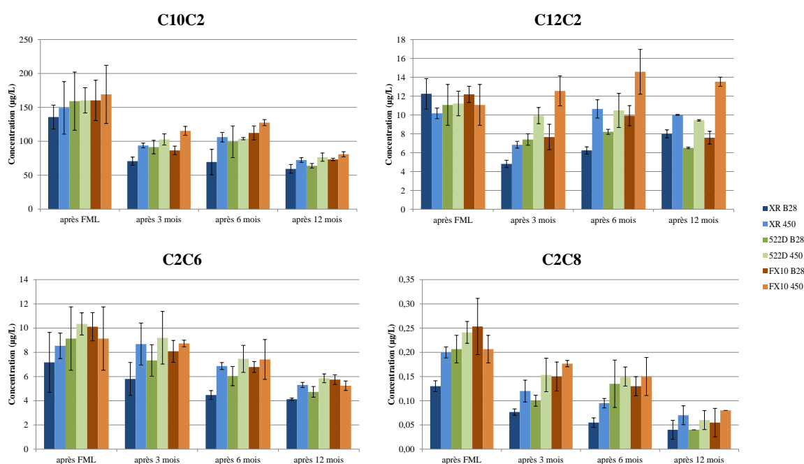
Figure 18. Teneurs moyennes en décanoate et dodécanoate d'éthyle ( C_{10}C_2 et C_{12}C_2 ) et en acétate d'hexyle et d'octyle ( C_2C_6 et C_2C_8 ) (exprimées en \mu\text{g/L} ) \pm intervalle de confiance à 5 % entre les répliquats observées dans les vins WEC 11 après FML et au cours de l'élevage.
