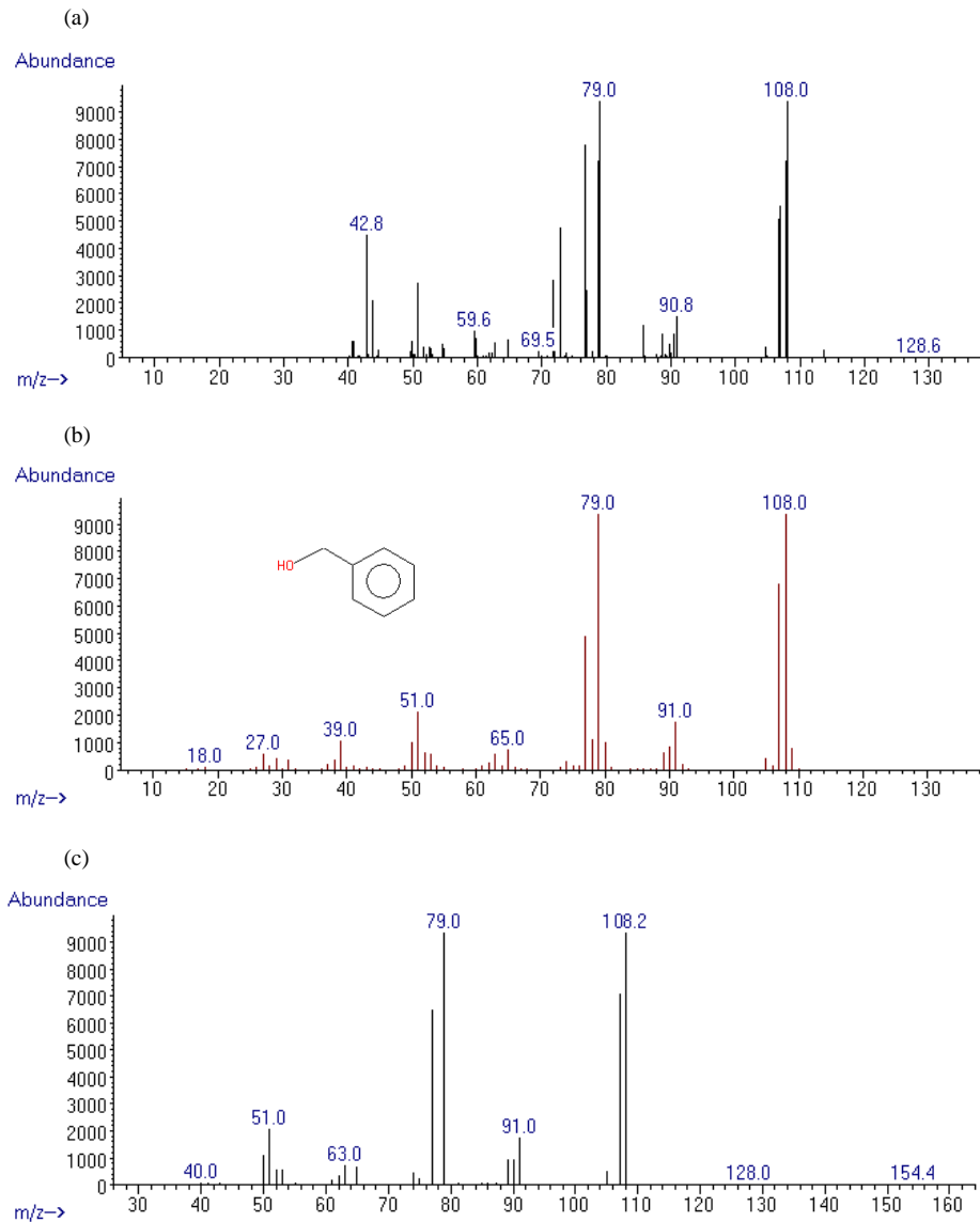
Figure 33. (a) Spectre de masse du pic C. (b) Spectre de masse de l'alcool benzylique selon NIST 2008 (NIST register number : 151560 ; CAS number : 100-51-6). (c) Spectre de masse de l'alcool benzylique en solution pure.
