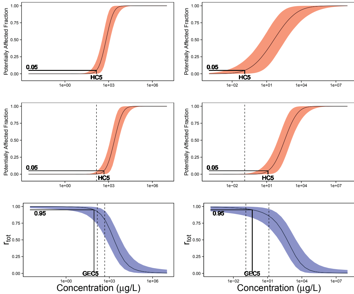
Figure I.3: SSD et réponse globale de la communauté à l'atrazine (gauche) et au diuron (droite). Haut : SSD classique, ajustée sur les EC_{10} avec la bande de confiance à 95% calculée par bootstrap et la HC_5 . Milieu : SSD classique, ajustée sur les EC_{50} avec la bande de confiance à 95% calculée par bootstrap et la HC_5 . Bas : réponse globale de la communauté avec la bande de crédibilité à 95% et la concentration correspondant à une réduction de 5% de la réponse globale ( GEC_5 ). Les lignes pointillées horizontales permettent de comparer la HC_{5,EC_{10}} , la HC_{5,EC_{50}} et la GEC_5
