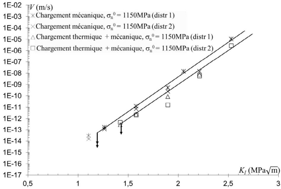
Figure III.27 Influence des contraintes initiales thermiques sur la prédiction de la fissuration lente à \sigma_n^0 = 1150\text{MPa} pour deux distributions d'orientations de grains du polycristal de zircon anisotrope.
