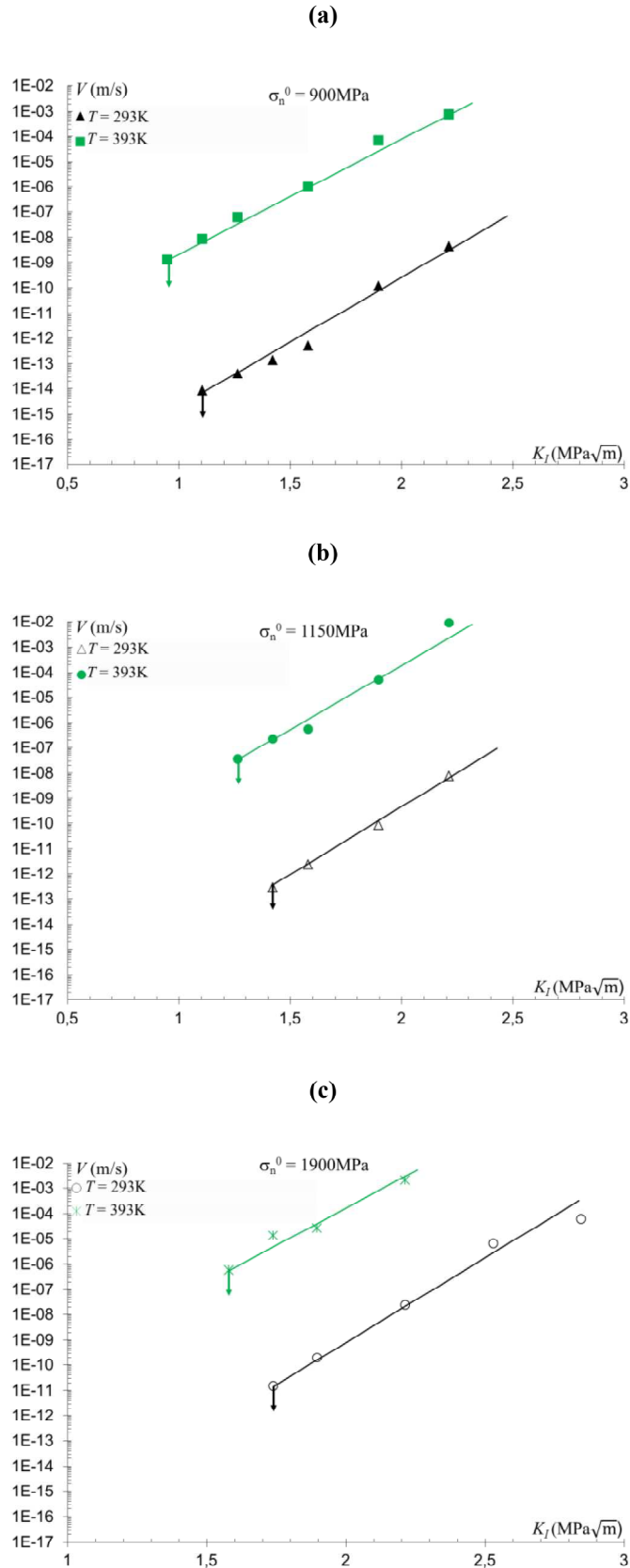
Figure IV.5 Influence de la température sur la fissuration lente intergranulaire de polycristal de zircone de \Phi_G = 0.8\mu\text{m} , (a) \sigma_n^0 = 900\text{MPa} , (b) \sigma_n^0 = 1150\text{MPa} et (c) \sigma_n^0 = 1900\text{MPa} . Le seuil de chargement K_0 diminue et la vitesse de fissuration augmente avec la température.
