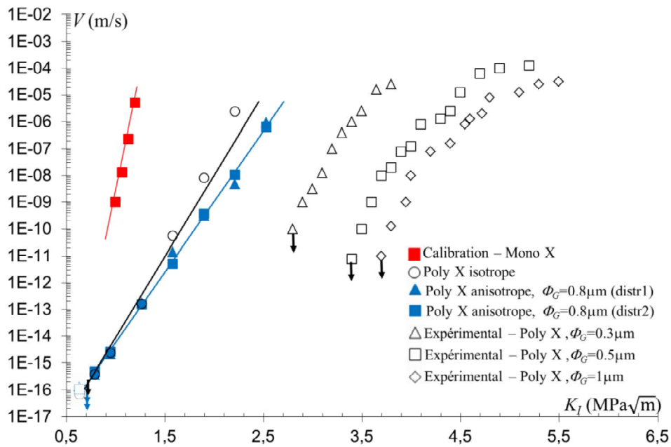
Figure III.16 Courbes V - K_I de fissuration lente avec la calibration des paramètres cohésifs de la zirconie, le polycristal de zirconie isotrope, le polycristal constitué de grains élastiques anisotropes vierge de contrainte initiale avec \Phi_G = 0.8\mu\text{m} avec deux distributions d'orientation de grains différentes et les résultats expérimentaux de propagation pour différentes tailles de grains [5].
