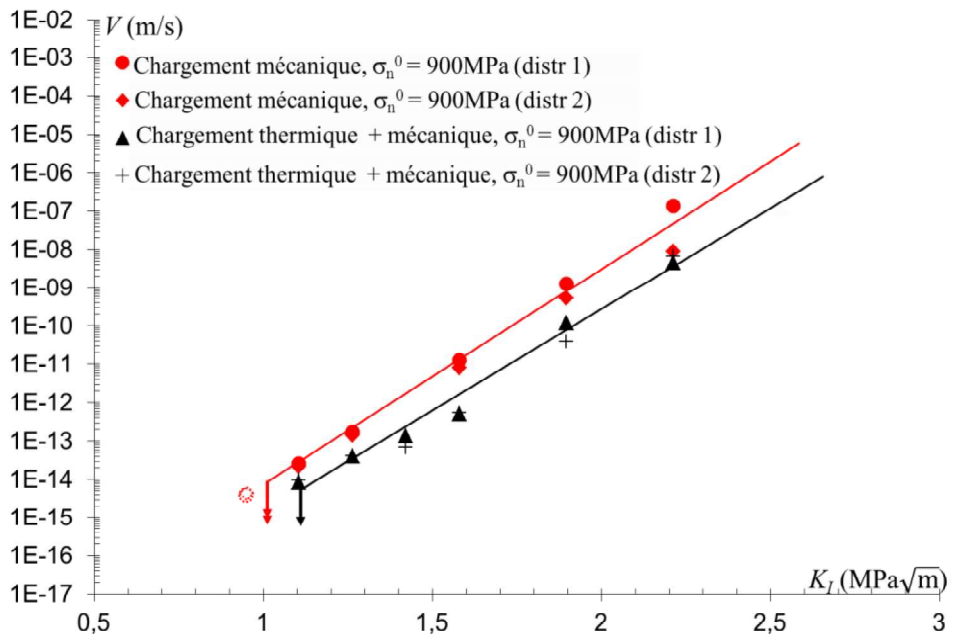
Figure III.26 Influence des contraintes initiales thermiques sur la prédiction de la fissuration lente à \sigma_n^0 = 900 MPa pour deux distributions d'orientations de grains du polycristal de zircon anisotrope.
