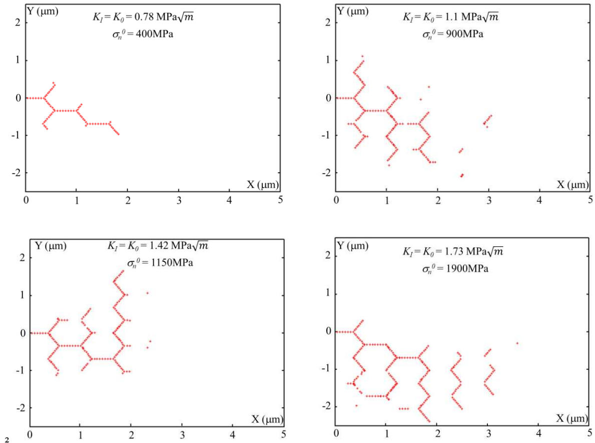
Figure III.29 Chemins des fissures jusqu'à l'arrêt de la propagation dans un polycristal de zirconium en tenant compte de contraintes initiales thermiques pour différentes valeurs de \sigma_n^0 = 400\text{MPa} , 900\text{MPa} , 1150\text{MPa} et 1900\text{MPa} .
