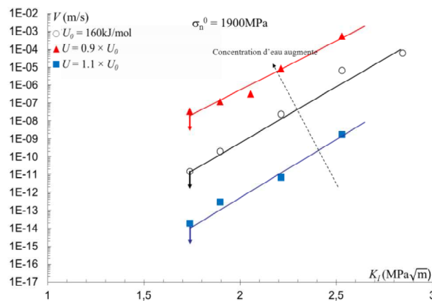
Figure IV.2 Influence de l'humidité avec une dépendance à l'énergie d'activation U sur la prédiction de la courbe V - K_I et le seuil K_0 dans un polycristal de zircon de \Phi_G = 0,8\mu\text{m} et une énergie d'activation référence U_0 = 160 kJ/mol à l'air ambiant, (a) \sigma_n^0 = 900 MPa, (b) \sigma_n^0 = 1150 MPa, (c) \sigma_n^0 = 1900 MPa. La vitesse de fissuration augmente avec la concentration d'eau sans affecter le niveau de chargement seuil K_0 .
