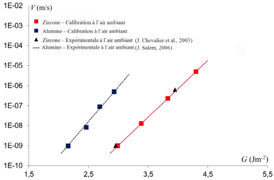
Figure II.11 Vitesse de fissuration V en fonction de taux de restitution G pour les monocristaux de zirconium et de saphir à l'air ambiant.
