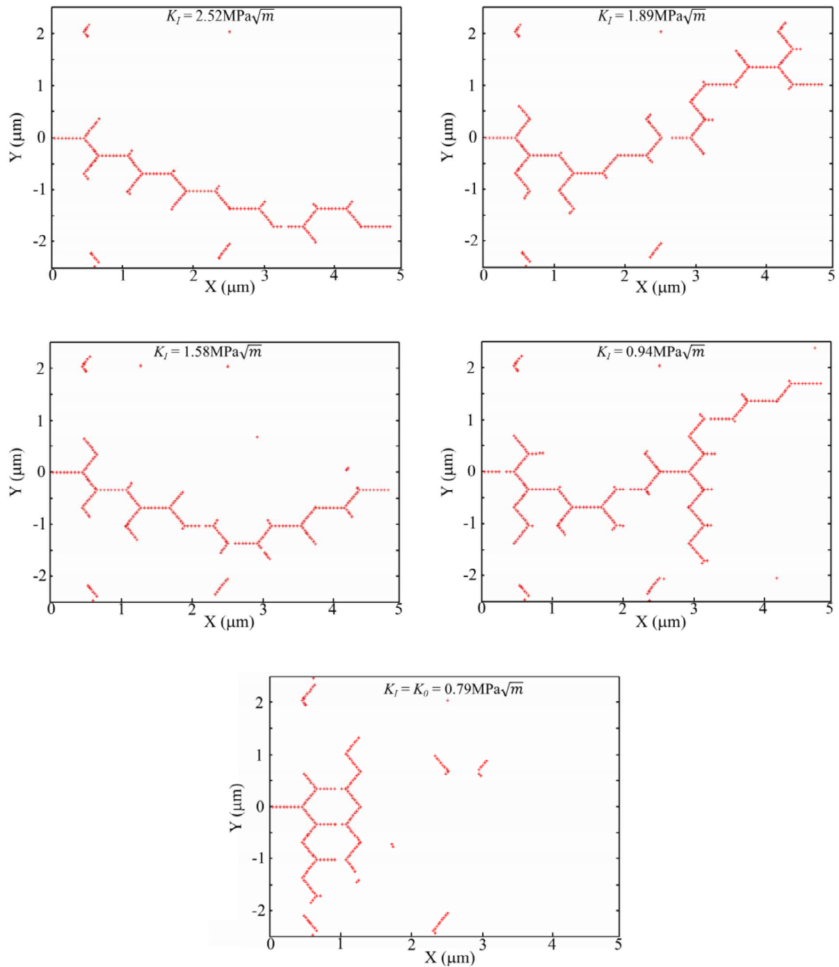
Figure IV.9 Chemins de fissuration intra-splat obtenus pour le polycristal de zircon ( \Phi_G = 0.8 \mu\text{m} ) anisotrope après relaxation des contraintes thermiques initiales et soumis à un chargement de fatigue statique pour différentes valeurs de K_I . Pour K_I = K_0 = 0.79 \text{ MPa}\sqrt{\text{m}} , la fissure est stoppée.
