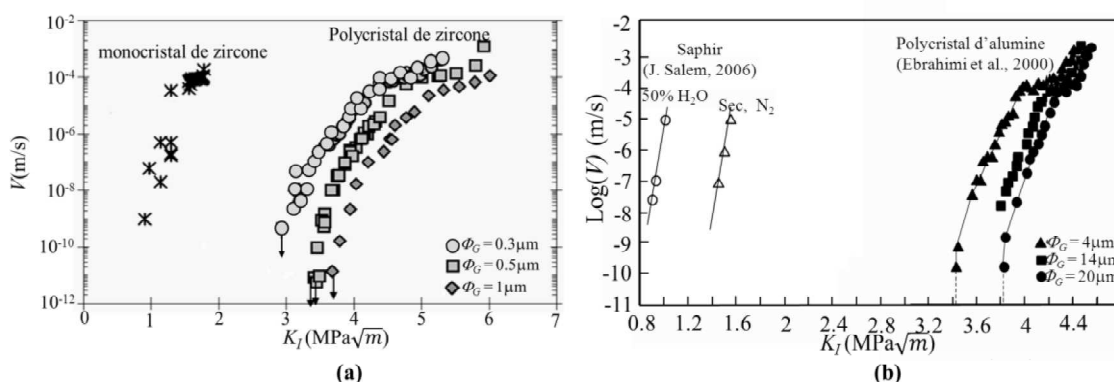
Figure I.10 (a) Courbes V-K_I d'un monocristal de zircon et de polycristaux de zircon frittés avec différentes tailles de grain (Chevalier et al. [34]), (b) Courbes V-K_I d'un saphir [35] et d'un polycristal d'alumine fritté avec différentes tailles de grain (Ebrahimi et al. [36]). La microstructure polycristalline augmente la résistance à la fissuration lente comparée à celle des monocristaux. Cette résistance augmente également avec la taille de grains.
