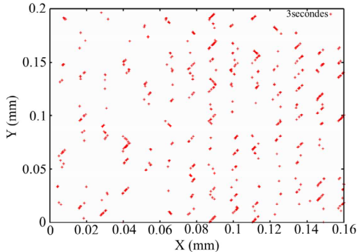
Figure V.15 Influence de la température sur la fissuration inter-splat de la zircono projetée plasma. Les taux de fissuration inter-splat à T = 393\text{K} est notablement supérieur à celui en conditions ambiantes (cf. Figure IV.13b).
