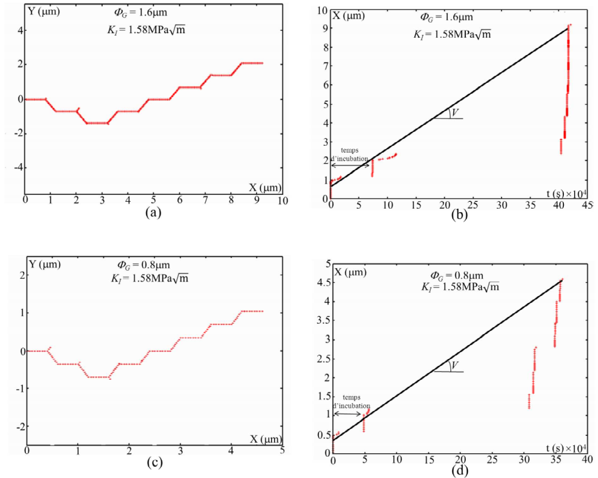
Figure III.19 Graphes X-t et X-Y pour une zone granulaire composée de (8 \times 8) grains de taille variable sous un niveau de chargement K_I = 1.58 \text{ MPa}\sqrt{\text{m}} . (a), (b) pour une taille de grain \Phi_G = 0.8 \mu\text{m} et (c), (d) pour une taille de grain \Phi_G = 1.6 \mu\text{m} . Le chemin de fissuration et l'avancée de la fissure au cours de temps sont identiques pour les deux tailles de grain considérées.
