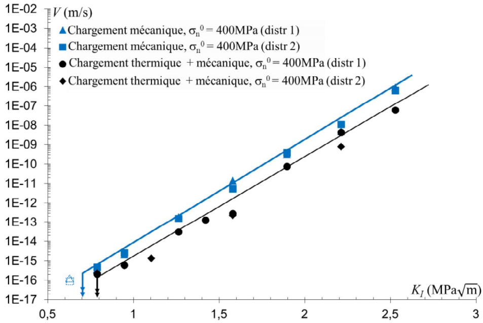
Figure III.25 Influence des contraintes initiales thermiques sur la prédiction de la fissuration lente à \sigma_n^0 = 400 MPa pour deux distributions d'orientations de grains du polycristal de zircon anisotrope.
