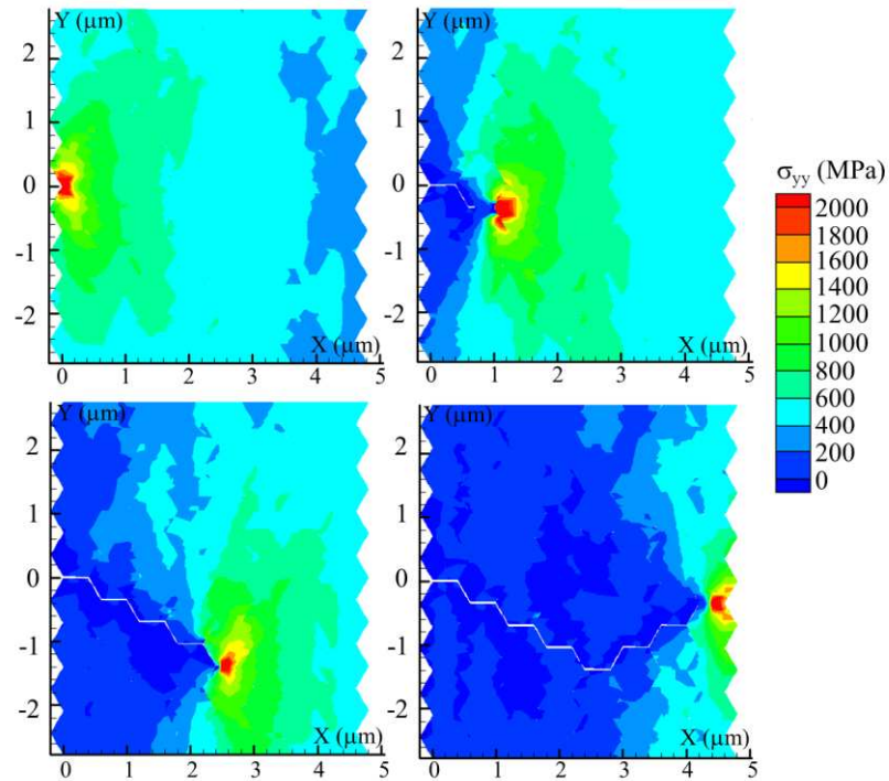
Figure III.11 Répartition de la composante \sigma_{yy} (MPa) de contrainte au cours de la propagation de la fissure au sein d'un polycristal constitué de grains élastiques anisotrope et vierge de contrainte initiale pour un chargement
