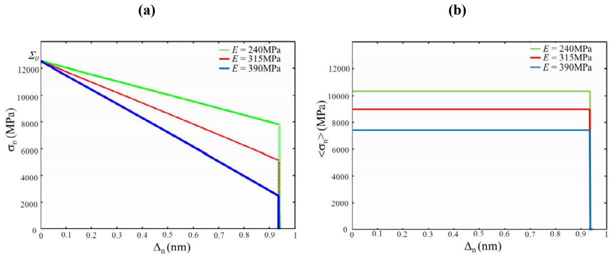
Figure II.15 (a) Courbes de la contrainte normale \sigma_n en fonction de l'ouverture normale \Delta_n de la surface cohésive insérée entre les deux blocs élastiques isotropes soumis à un chargement de relaxation avec une contrainte initiale \Sigma identique pour les différentes valeurs de module d'Young E considérées, (b) Courbes de contrainte moyenne \langle \sigma_n \rangle en fonction de déplacement \Delta_n au niveau de la surface cohésive.
