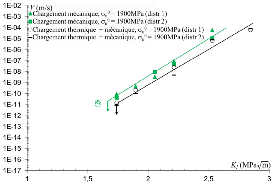
Figure III.28 Influence des contraintes initiales thermiques sur la prédiction de la fissuration lente à \sigma_n^0 = 1900\text{MPa} pour deux distributions d'orientations de grains du polycristal de zircon anisotrope.
