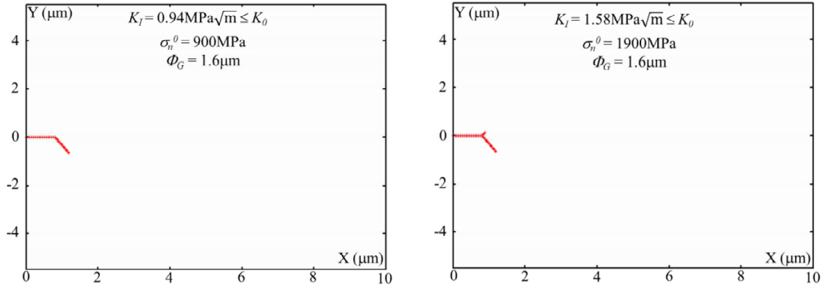
Figure III.21 Chemins de fissures jusqu'à l'arrêt lorsque l'obstacle P3 est atteint pour un polycristal de zircon avec \Phi_G = 1.6 \mu\text{m} et pour \sigma_n^0 = 900 MPa et 1900 MPa.
