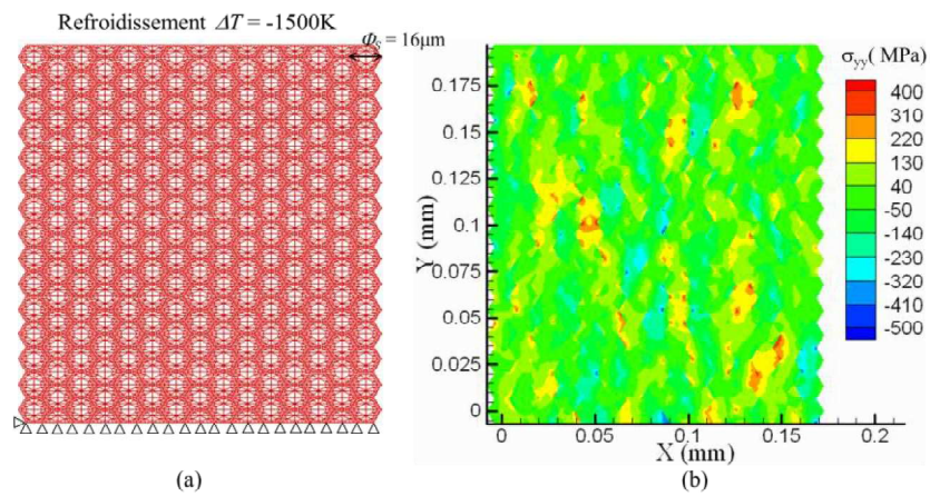
Figure IV.12 (a) Maillage et conditions aux limites appliquées pour le chargement thermique pour un polycristal de zircone projetée plasma à l'échelle des splats, le matériau est modélisé par de 15 \times 15 splats avec une taille \phi_s = 16\mu\text{m} , (b) Répartition de la contrainte \sigma_{yy} (MPa) refroidissement uniforme \Delta T = -1500\text{K} .
