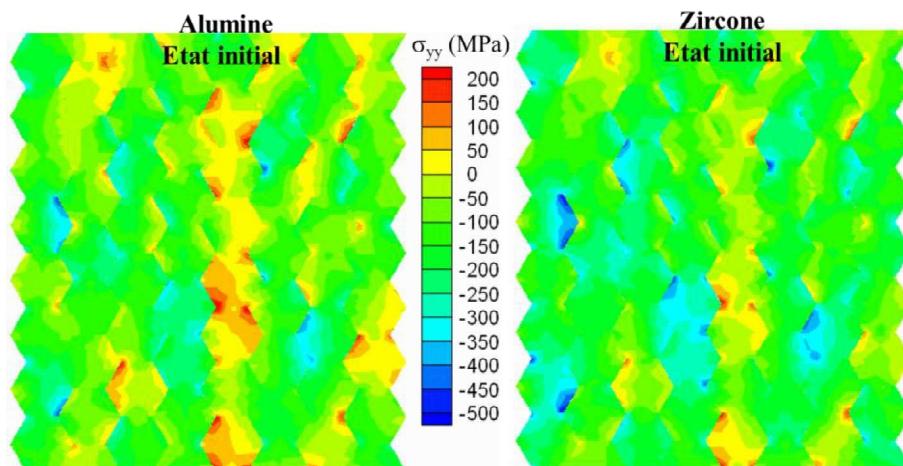
Figure III.35 Répartition de la composante \sigma_{yy} (MPa) dans les cellules granulaires des grains d'alumine et de zirconium après un chargement thermique de \Delta T = -1500\text{K} . La cellule granulaire des grains de zirconium présentent plus de zones en compression et moins de zone en traction en comparaison avec celle des grains d'alumine.
