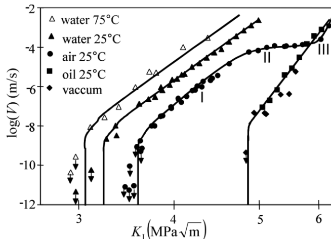
Figure IV.1 Courbes V-K_I d'un polycristal de zircono stabilisée (3% Yttrium) avec une taille de grain \Phi_G \approx 1\mu\text{m} sous différents environnements. La fissuration des céramiques polycristallines est, à l'image des verres et monocristaux, sensible au temps, à la contrainte, à la température et à l'eau (Chevalier et al. [1])
