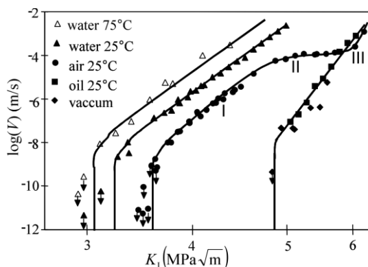
Figure I.11 Courbes V-K_I d'un polycristal de zircon stabilisée (3% Yttrium) avec une taille de grain \Phi_G \approx 1\mu m sous différents environnements. La fissuration des céramiques polycristallines est, à l'image des verres et des monocristaux, sensible au temps, au niveau de chargement mécanique appliqué, à la température et à l'eau (Chevalier et al. [37]).
