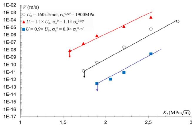
Figure IV.3 Influence de l'humidité avec une dépendance à l'énergie d'activation U et du seuil de réaction-rupture \sigma_n^0 sur la prédiction de la courbe V-K_I et le seuil K_0 dans un polycristal de zircone de \Phi_G = 0,8\mu\text{m} . La vitesse de fissuration augmente et le seuil K_0 diminue lorsque la concentration d'eau locale augmente.
