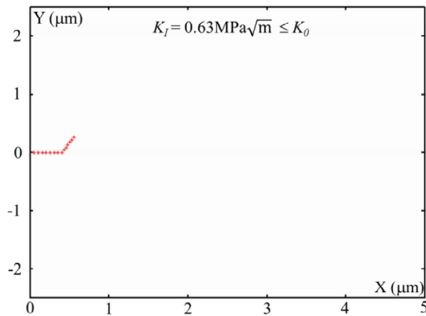
Figure III.6 Chemin de fissure et arrêt dès que la phase P3 est atteint pour un polycristal constitué de grains isotropes avec \Phi_G = 0,8\mu m . La fissure s'arrête après amorçage de sa propagation au niveau du point triple pour un chargement seuil K_I = 0,63 MPa\sqrt{m} \leq K_0 , K_0 étant le chargement seuil au-dessous duquel il n'y a plus propagation de la fissure.
