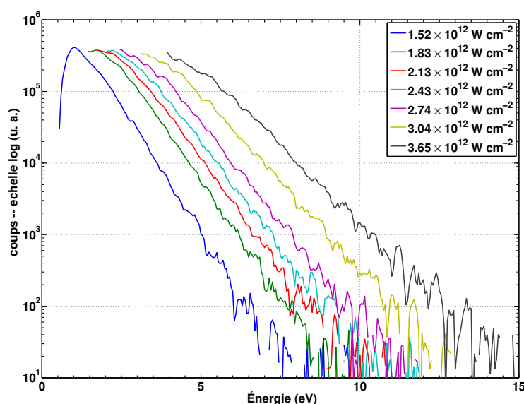
Figure D.9 – Spectres de photoélectrons pour des intensités laser de \{1,52, 1,83, 2,13, 2,43, 2,74, 3,04, 3,65\} \times 10^{12} \text{ W cm}^{-2} , avec V_{\text{tip}} = 20 \text{ V} . Les spectres sont plus étroits que ceux obtenus à partir de nanopointes de tungstène avec des intensités équivalentes, mais avec une émission beaucoup plus intense qui sature les MCPs. Ces effets de saturation ont été supprimés des spectres.
