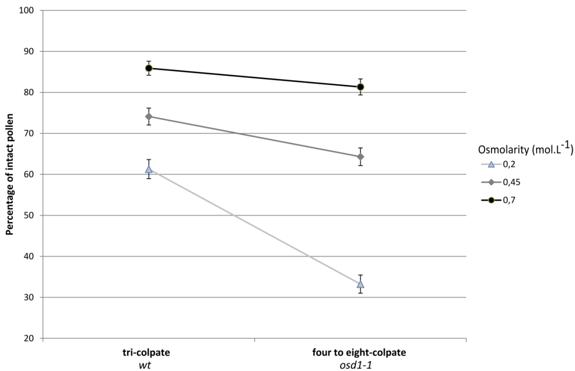
Figure 22 : Effet de l'osmolarité et du nombre d'apertures dans le fond génétique Nooséen. Les individus étudiés produisent du pollen à trois apertures, ou des pollens présentant de quatre à huit apertures.
