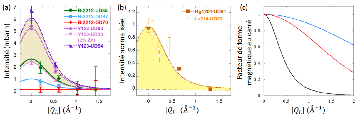
Figure 5.12: (a) Évolution de l'intensité magnétique en fonction de |Q_L| = \frac{2\pi}{c}L dans deux systèmes bicouches Y123 et Bi2212. (b) Évolution de l'intensité magnétique normalisée en fonction de |Q_L| dans deux systèmes monocouches Hg1201 et La214. (c) Facteur de forme magnétique au carré du cuivre (ligne bleue) et de l'oxygène (ligne rouge) en comparaison à l'évolution de l'intensité de l'ordre à q=0 (ligne noire) en fonction de |Q_L| . Cette dépendance suit la forme d'une fonction lorentzienne au carré. Il s'agit d'une fonction d'essai, sans signification physique particulière. Les trois courbes sont normalisées à |Q_L|=0 .
