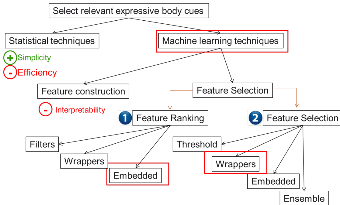
Figure 13: Résumé des méthodes de sélection de paramètres dans proposées dans la littérature.
