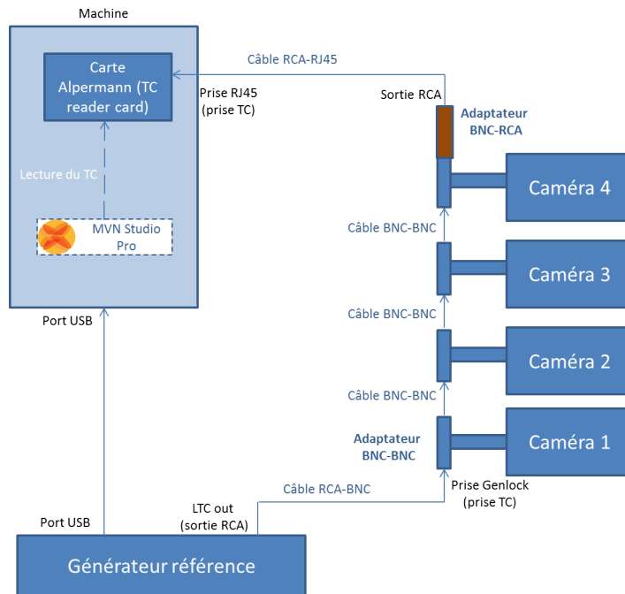
Figure 4: Le protocole de synchronisation des données de capture de mouvement et les données audio-visuelles que nous avons utilisé pour enregistrer les expressions corporelles dans la base de données Emilya.
