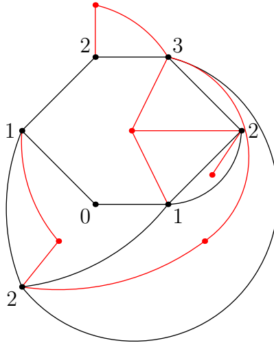
Figure 1.1.5 – Exemple de la construction de la bijection BDG en partant d'une carte bipartie pour arriver à un arbre.
