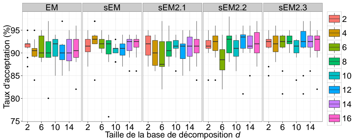
FIGURE 2.25 – Cas analytique : boxplots du critère C_3^e , taux d'acceptation du test de Kolmogorov-Smirnov sur la covariable, en fonction de la taille d de la base de décomposition.
