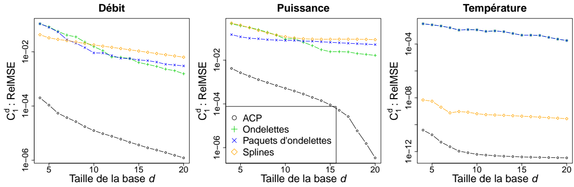
FIGURE 2.15 – Cas LiPoSo : critère C_1^d (RelMSE) pour le débit (à gauche), la puissance (au milieu) et la température (à droite) pour les décompositions ACP, splines, décomposition en ondelettes et en paquet d'ondelettes (échelle logarithmique).
