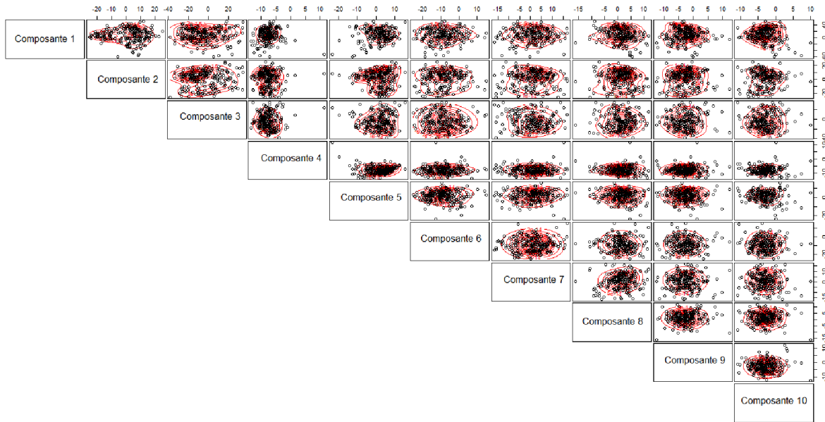
FIGURE 2.26 – Cas analytique : les 200 coefficients de la base d’apprentissage en dimension 10 (en noir) et le contour de la densité de probabilité estimée avec l’algorithme sEM2.2 (en rouge).
