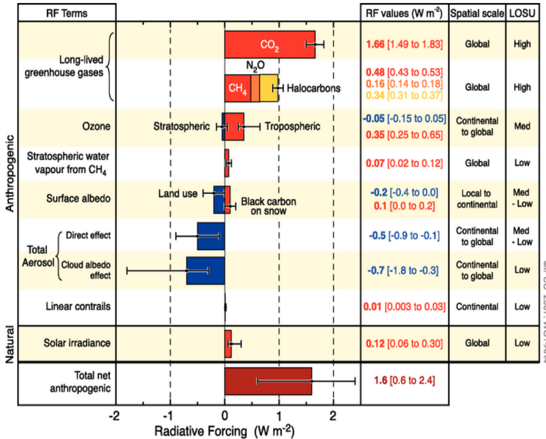
Figure 3.3. Forçage radiatif des différents constituants de l'atmosphère (Source : IPCC)
