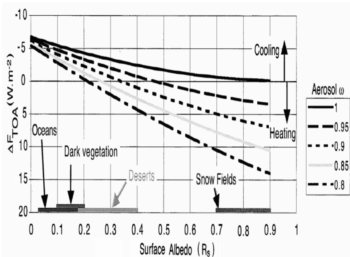
Figure 3.5. Variation du forçage radiatif au sommet de l'atmosphère pour différentes valeurs de SSA et d'albedo de surface (Sources : Russell et al., 2002).
