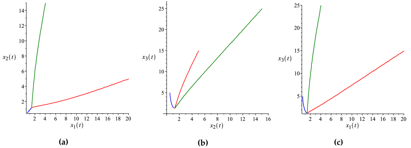
FIGURE 4.3 – Trajectoires avec les conditions initiales indiquées dans le texte : (a) l'espace (x_1, x_2) . (b) l'espace (x_2, x_3) . (c) l'espace (x_1, x_3) .
