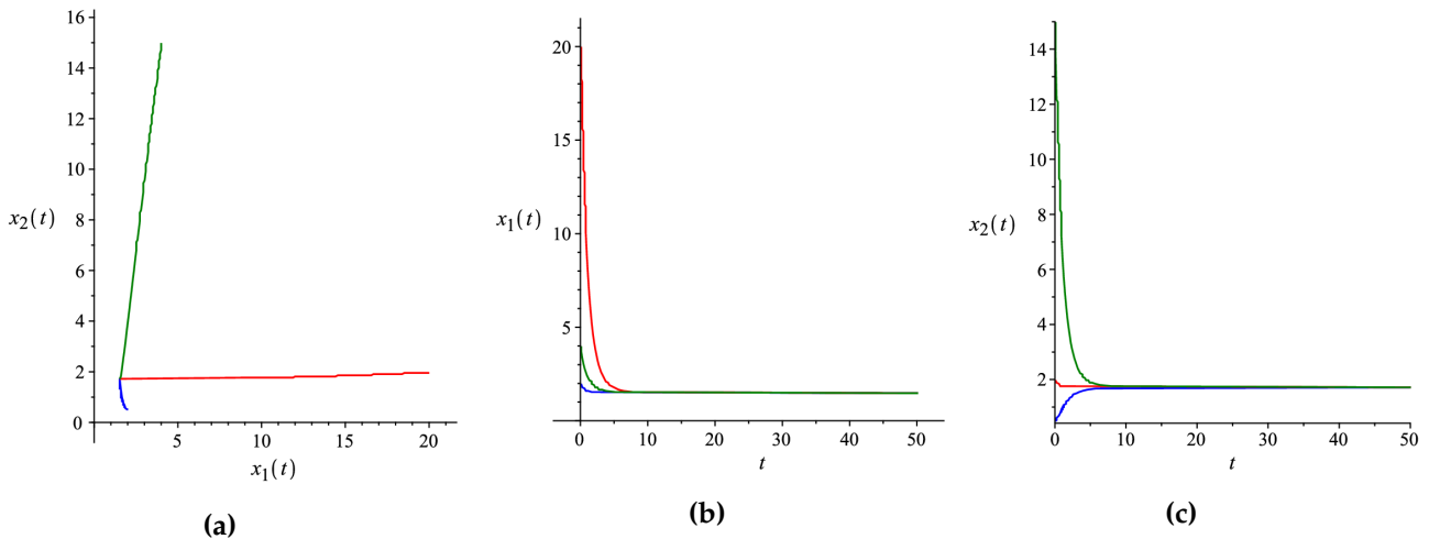
FIGURE 3.3 – (a) Trajectoires dans l'espace (x_1, x_2) avec les conditions initiales indiquées dans le texte. (b)-(c) La convergence des composantes x_1(t) et x_2(t) vers un point d'équilibre intérieur.
