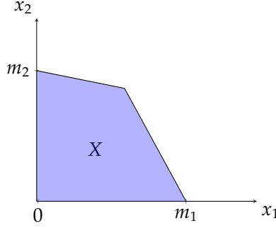
FIGURE 3.1 – Domaine de définition du système (3.4) avec m_i := \min(\gamma_{si}s^\circ, \gamma_{ri}r^\circ) .
