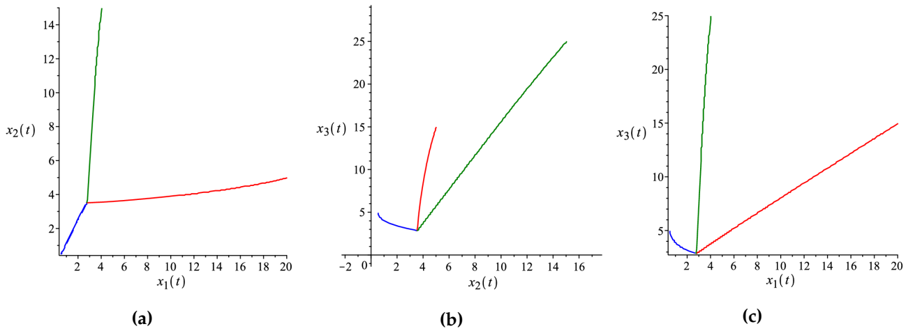
FIGURE 4.1 – Trajectoires avec les conditions initiales indiquées dans le texte : (a) l'espace (x_1, x_2) . (b) l'espace (x_2, x_3) . (c) l'espace (x_1, x_3) .
