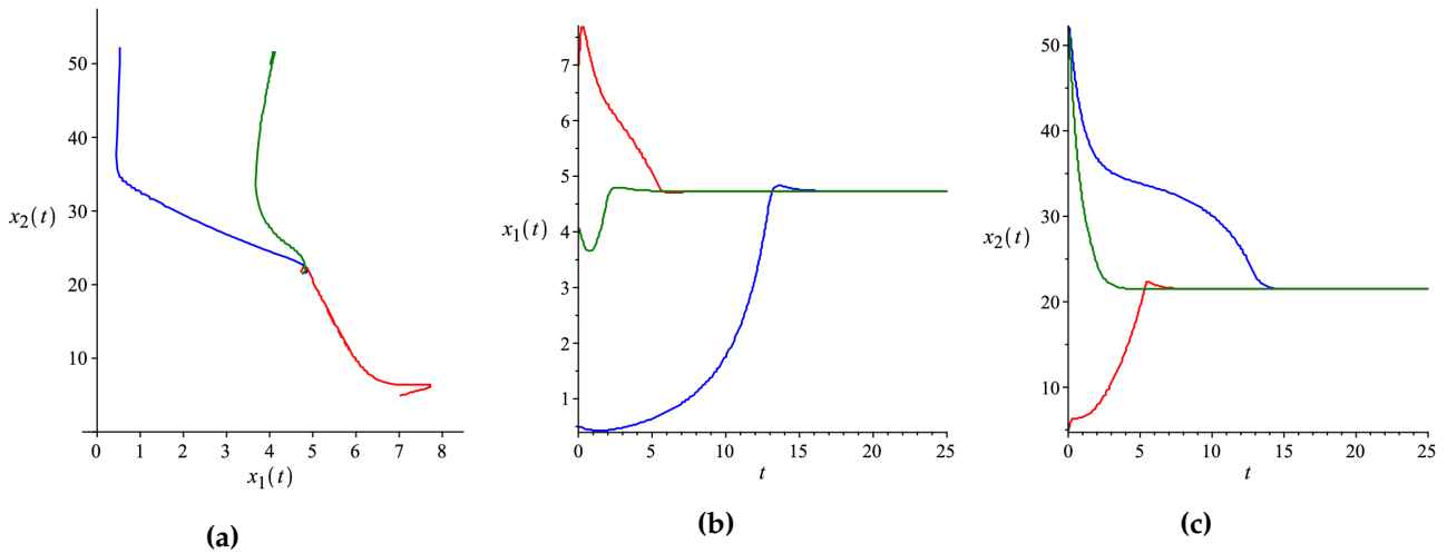
FIGURE 2.1 – (a) Trajectoires dans l'espace (x_1, x_2) avec les conditions initiales indiquées dans le texte. (b)-(c) La convergence des composantes x_1(t) et x_2(t) vers un point d'équilibre intérieur.
