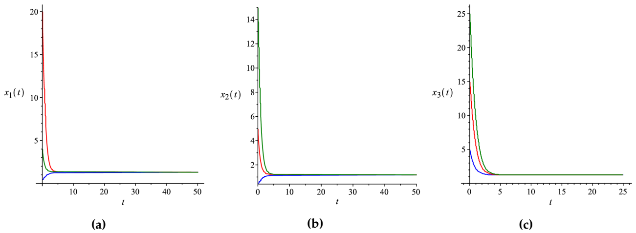
FIGURE 4.4 – La convergence vers un point d'équilibre intérieur de la composante : (a) x_1(t) . (b) x_2(t) . (c) x_3(t) .
