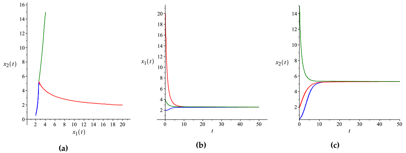
FIGURE 3.4 – (a) Trajectoires dans l'espace (x_1, x_2) avec les conditions initiales indiquées dans le texte. (b)-(c) La convergence des composantes x_1(t) et x_2(t) vers un point d'équilibre intérieur.
