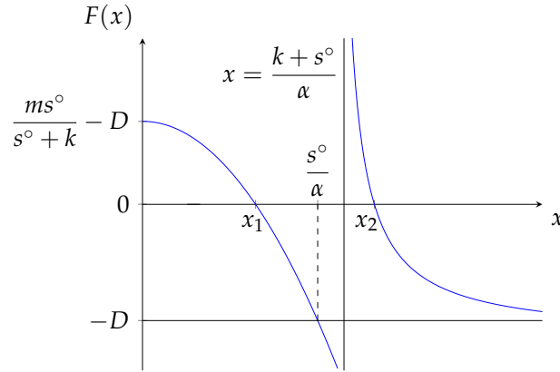
FIGURE 3.2 – Allure de la courbe de F .
