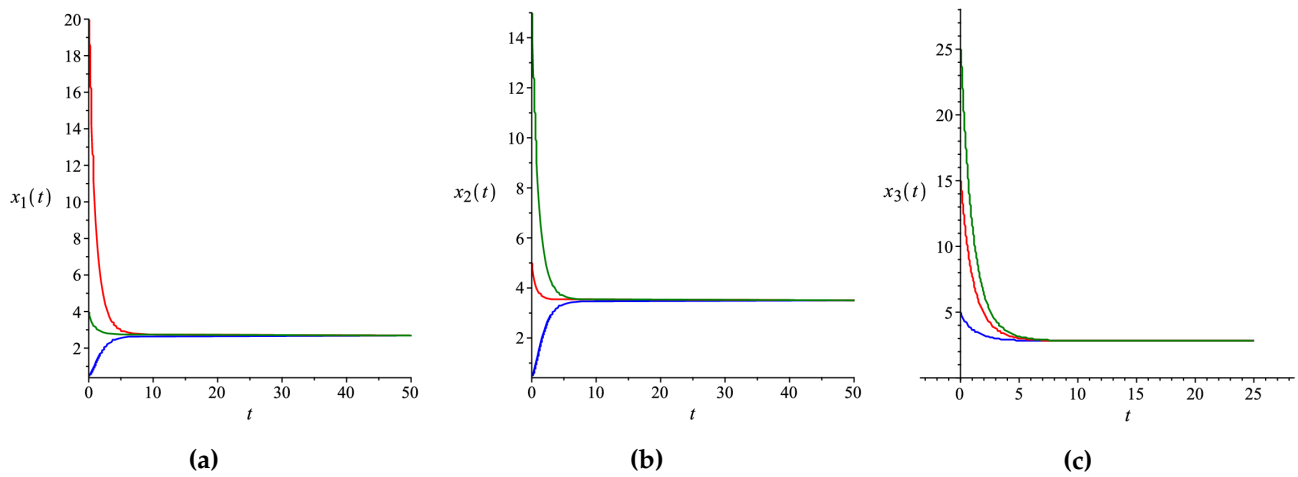
FIGURE 4.2 – La convergence vers un point d'équilibre intérieur de la composante : (a) x_1(t) . (b) x_2(t) . (c) x_3(t) .
