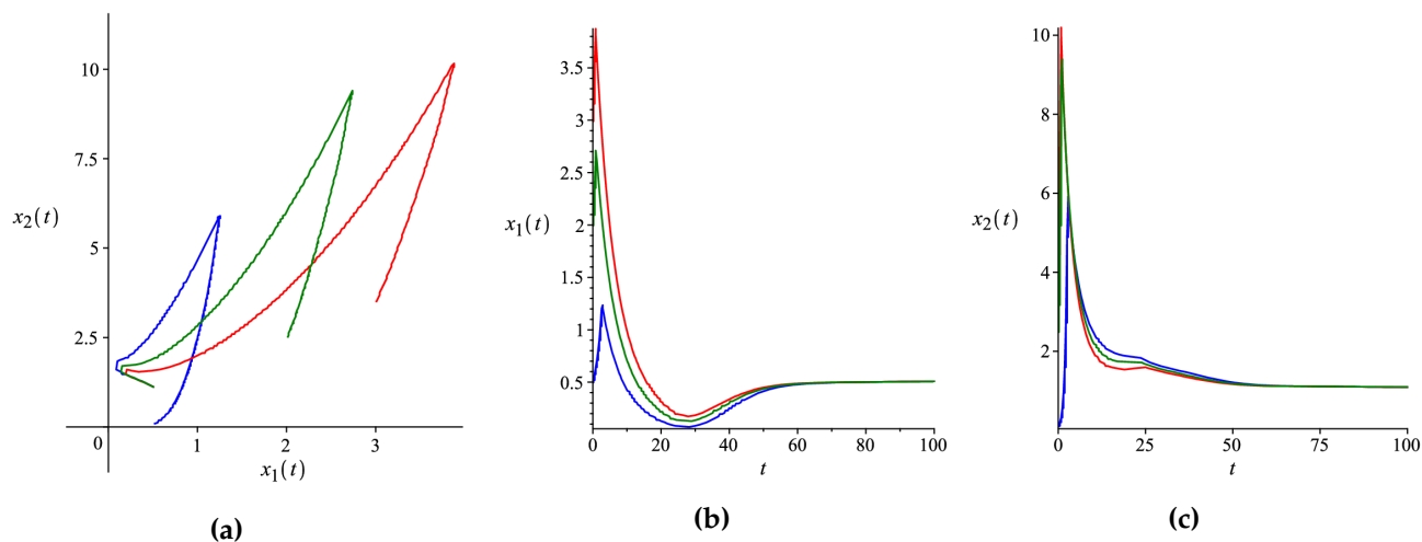
FIGURE 2.2 – (a) Trajectoires dans l'espace (x_1, x_2) avec les conditions initiales indiquées dans le texte. (b)-(c) La convergence des composantes x_1(t) et x_2(t) vers un point d'équilibre intérieur.
