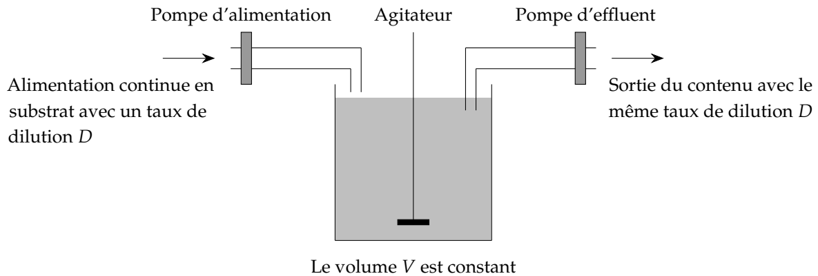
FIGURE 1.1 – Schéma d'un chemostat.
