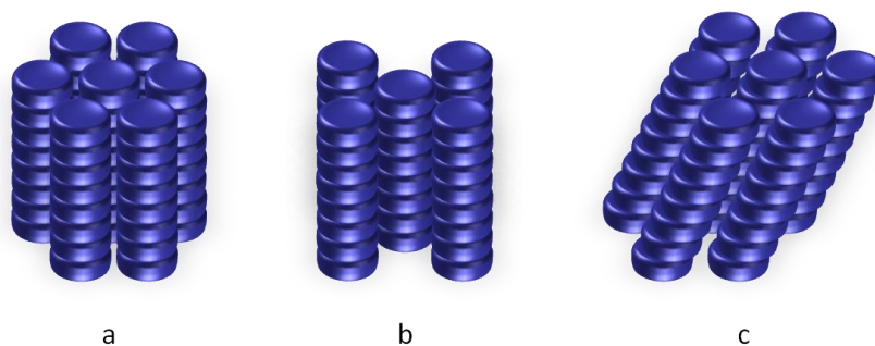
Figure III-4 : Représentation schématique des phases colonnaire hexagonale (a), rectangulaire (b), et obliques (c). Les disques bleus représentent les mésogènes discotiques.
