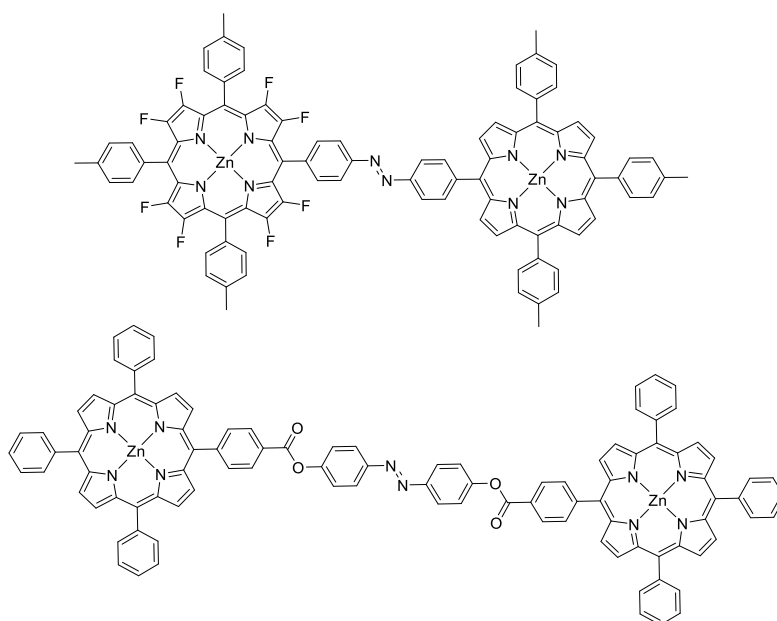
Figure II-49 : Représentations des dimères de porphyrines développés par Tsuchiya ( en haut ) et Arai ( en bas ).
