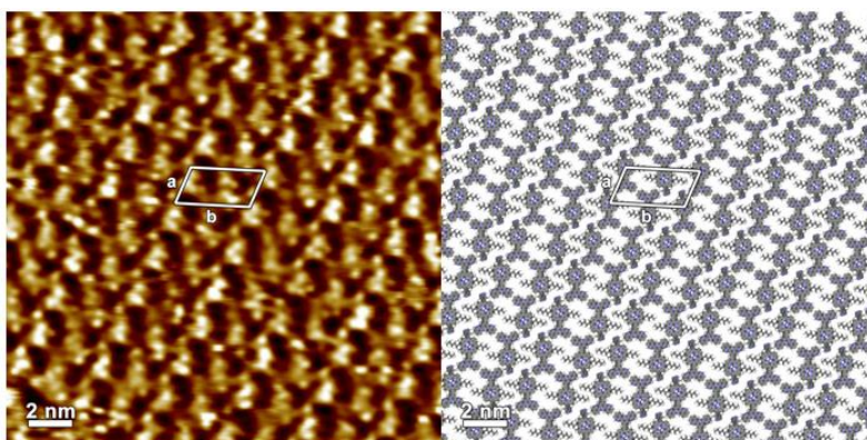
Figure I-32 : Image STM (a) et représentation de l'arrangement des molécules T3 sur une surface HOPG (b). L'unité asymétrique est indiquée en blanc (rhombique ; a = 1.86 \text{ nm} , b = 3.44 \text{ nm} , \alpha = 70^\circ ).
