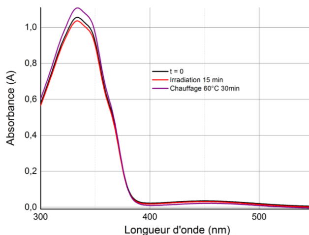
Figure II-47 : Spectre d'absorption du suivi de l'isomérisation de 22 par chauffage.
