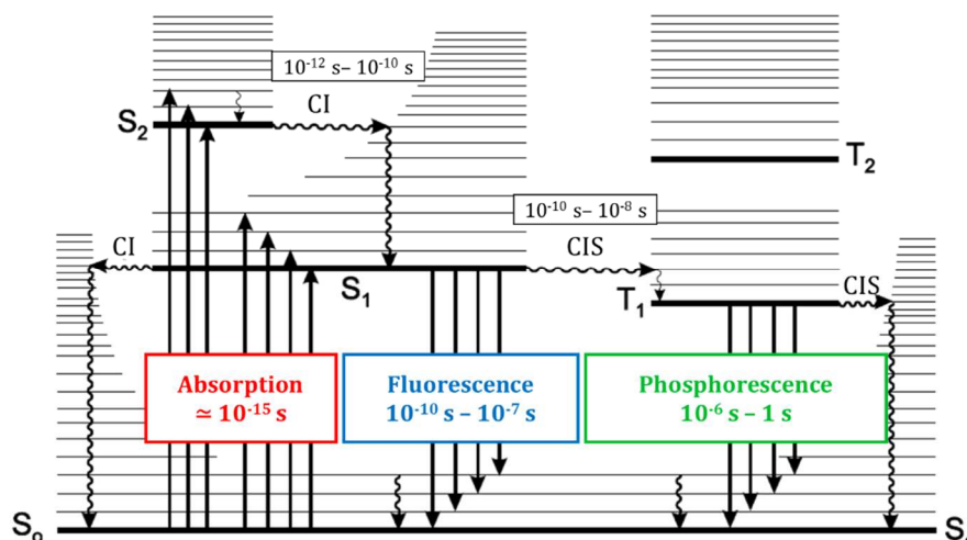
Figure 1.42. Diagramme de Perrin-Jablonski.
