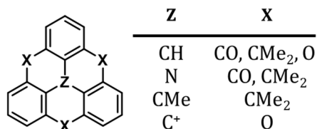
Figure 2.4. Formule générale des triangulènes.
