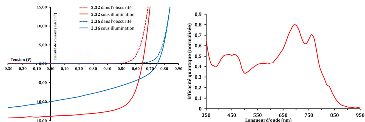
Figure 2.68. À gauche : Courbes J(V) dans l'obscurité et sous illumination des dispositifs basés sur les mélanges 2.32 /PC 70 BM et 2.36 /PC 70 BM. À droite : spectre d'efficacité quantique externe mesuré sur la cellule du mélange 2.32 /PC 70 BM ayant donné le résultat précédent.
