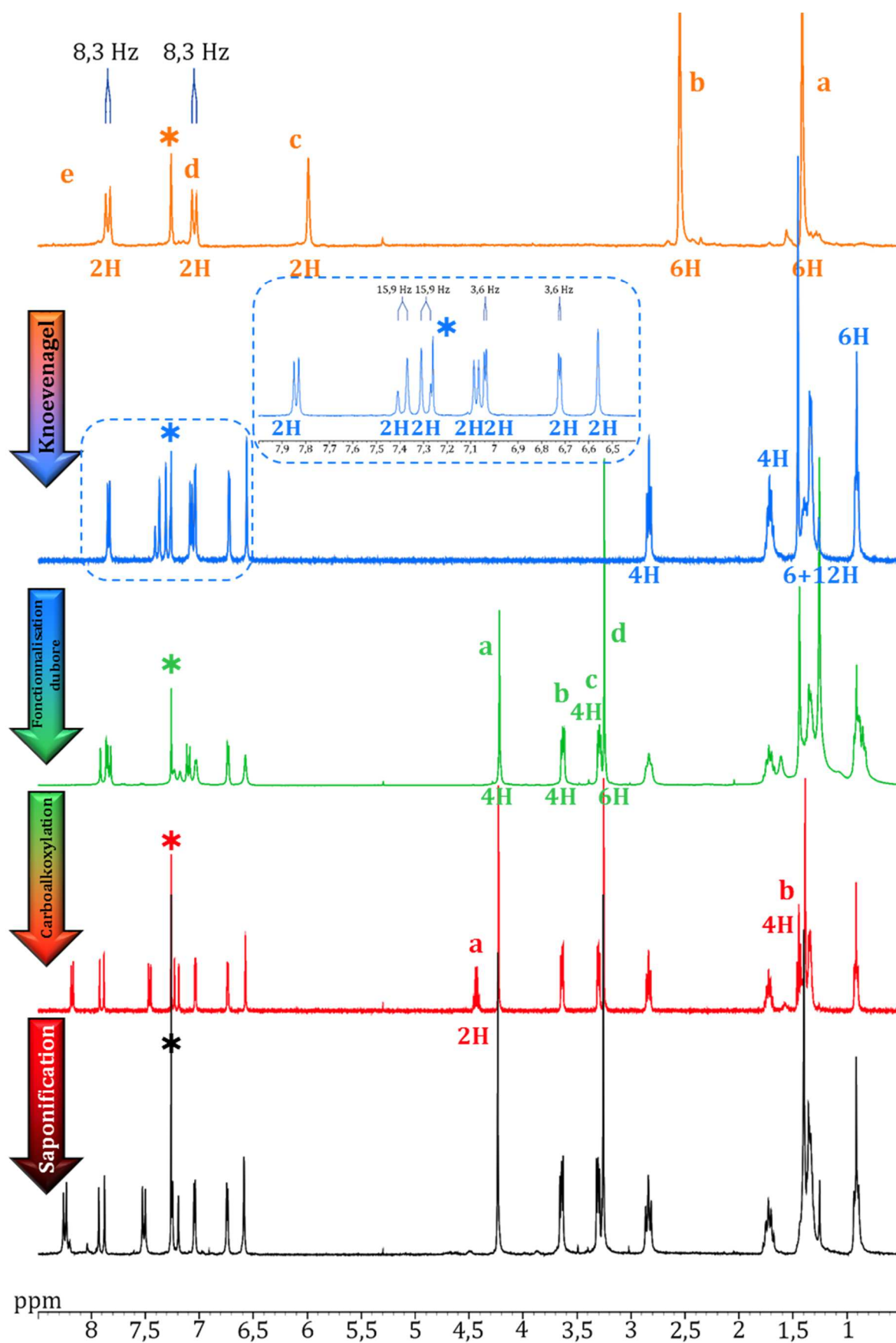
Figure 4.18. Spectres RMN du ^1\text{H} de chaque étape menant à la formation de S 2 TPA . 4.0 ( \text{CDCl}_3 , 200 MHz), 4.1 ( \text{CDCl}_3 , 300 MHz), 4.4 ( \text{CDCl}_3 , 300 MHz), 4.7 ( \text{CDCl}_3 , 300 MHz) et S 2 TPA ( \text{CDCl}_3 , 300 MHz) à 298 K ; * = \text{CHCl}_3 .
