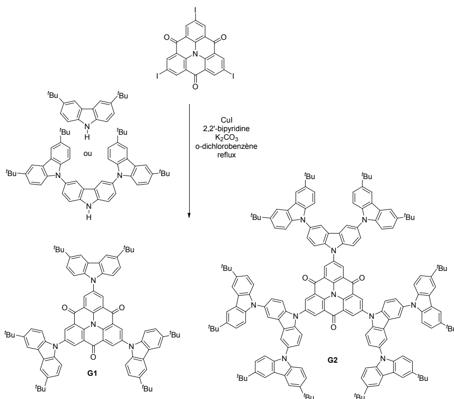
Figure 2.10. Synthèses proposée par Chen et al. des dendrimères possédant un cœur central à base de triangulène utilisés dans des dispositifs OLED. 140
