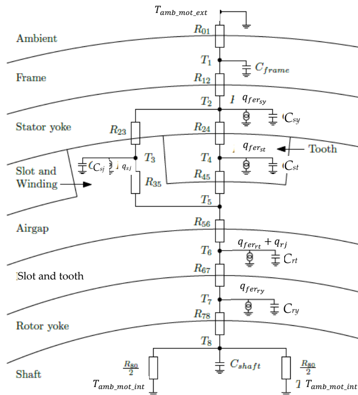
Figure 2.23 : Schéma du modèle thermique [KREU08] adapté
