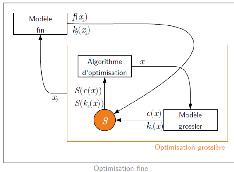
Figure 3.5 : Schéma de principe de l'OSM [PIER14]
