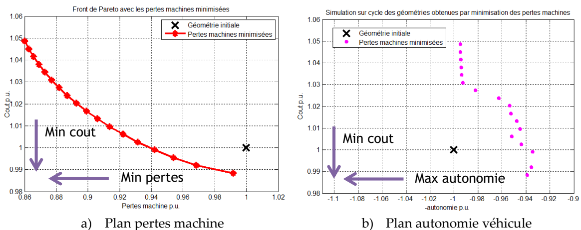
Figure 4.6 : Front de Pareto de la minimisation des pertes machine
