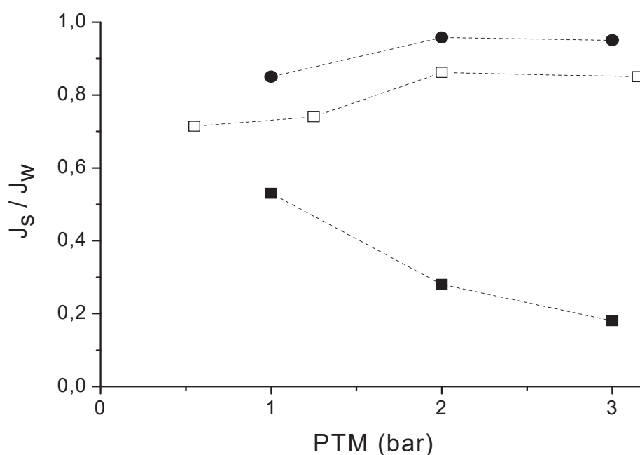
Figure 41 : Influence de la nature de la solution filtrée et de la pression PTM sur le rapport J_s/J_w ; pH = 7 ; [PAANa] = [BPEI] = 5 \cdot 10^{-3} mol.L -1 ; [M]_{\text{tot}} = 1,67 \times 10^{-3} mol.L -1 ; SC : 150 kDa ; membrane d'UF en TiO 2 ; M_{\text{tot}} = \text{Ag}^+ , \text{Ni}^{2+} et \text{Zn}^{2+} ; vitesse tangentielle = 6,1 m.s -1 ; Cations métalliques libres (●) PAANa-M-BPEI (■) Surnageant de PAANa-M-BPEI (□).
