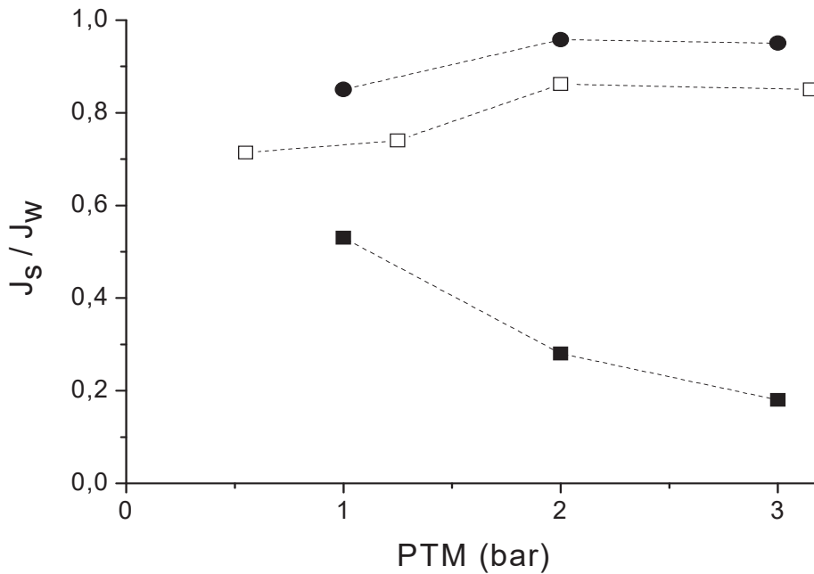
Figure 41 : Influence de la nature de la solution filtrée et de la pression PTM sur le rapport J_s/J_w ; pH = 7 ; [PAANa] = [BPEI] = 5 \cdot 10^{-3} mol.L -1 ; [M]_{\text{tot}} = 1,67 \cdot 10^{-3} mol.L -1 ; SC : 150 kDa ; membrane d'UF en TiO 2 ; M_{\text{tot}} = \text{Ag}^+ , Ni 2+ et Zn 2+ ; vitesse tangentielle = 6,1 m.s -1 ; Cations métalliques libres (●) PAANa-M-BPEI (■) Surnageant de PAANa-M-BPEI (□).
