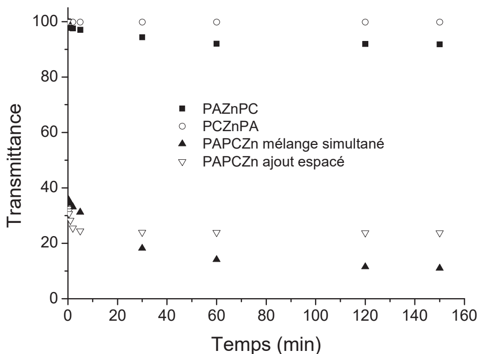
Figure 30 : Evolution de la transmittance pour les solutions contenant polyélectrolytes et Zn^{2+} à pH= 6,5 ; [PAANa]_0 = [BPEI]_0 = 5 \times 10^{-3} \text{ mol.L}^{-1} ; [Zn^{2+}]_0 = 1/6 [\text{polymère}]_{\text{tot}} = 1,67 \times 10^{-3} \text{ mol.L}^{-1} .
