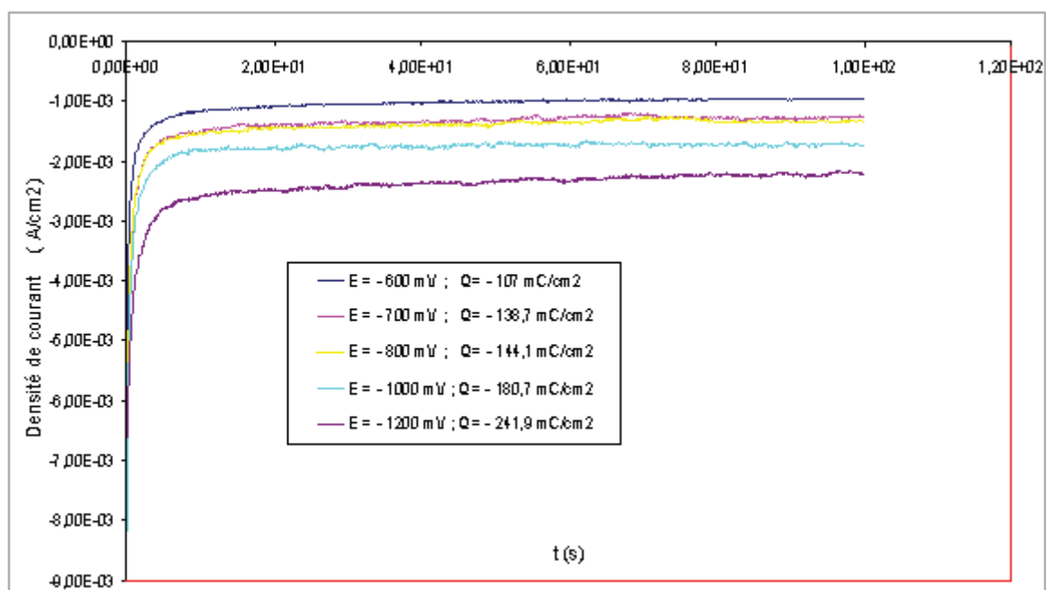
Figure 48 : Courbes de chronoampérométrie de la solution PAANa-Cu-BPEI à pH = 4, [PAANa] = [BPEI] = 5 \cdot 10^{-3} mol.L -1 , [Cu 2+ ] = 1,67 \cdot 10^{-3} mol.L -1 .
