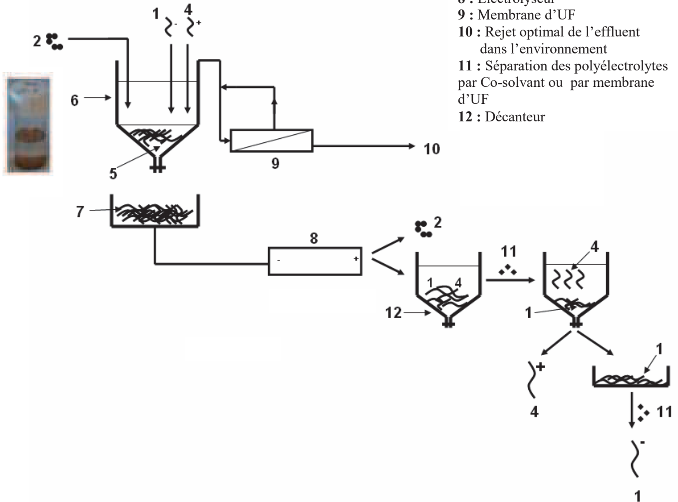
Figure 27 : Schéma de principe du procédé développé.
