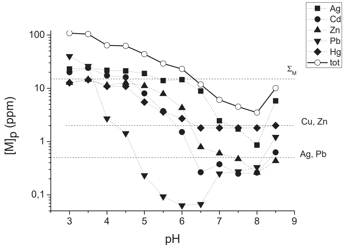
Figure 35 : Effet du pH sur la concentration résiduelle en ions métalliques libres dans l'assemblage PAANa-M-BPEI. Membrane en PES (SC : 3 kDa) ; [PAANa]_0 = [BPEI]_0 = 5 \times 10^{-3} \text{ mol.L}^{-1} ; [M]_{\text{tot}} = 1,67 \times 10^{-3} \text{ mol.L}^{-1} ; PTM = 3 bars ; M_{\text{tot}} = \text{Ag}^+, \text{Cd}^{2+}, \text{Zn}^{2+}, \text{Pb}^{2+} \text{ et } \text{Hg}^{2+} .
