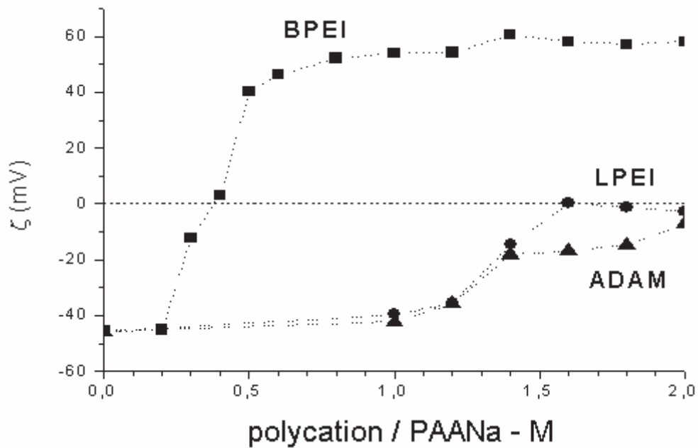
Figure 39 : Courbe du potentiel zêta en fonction du rapport de quantité de polyelectrolytes ; [M]_{\text{tot}} = 8,33 \times 10^{-4} \text{ mol.L}^{-1} ; \text{pH} = 7 ; [\text{PAANa}]_0 = 5 \times 10^{-5} \text{ mol.L}^{-1} ; M_{\text{tot}} = \text{Cd}^{2+}, \text{Ni}^{2+}, \text{Zn}^{2+} et \text{Pb}^{2+} ; BPEI (-■-) ; LPEI (-●-) et ADAM (-▲-).
