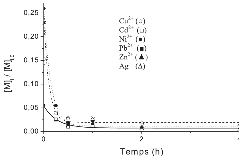
Figure 33 : Courbe de cinétique de la fixation des ions métalliques par le PAANa. Membrane en PES (SC : 3kDa) ; pH = 6,5 ; [M]_{0,\text{tot}} = 2 \times 10^{-4} \text{ mol.L}^{-1} = 1/50 [PAANa]_0 ; [PAANa]_0 = 10^{-2} \text{ mol.L}^{-1} ; PTM = 3 bar ; [M]_0 = 3,3 \times 10^{-5} \text{ mol.L}^{-1} .
