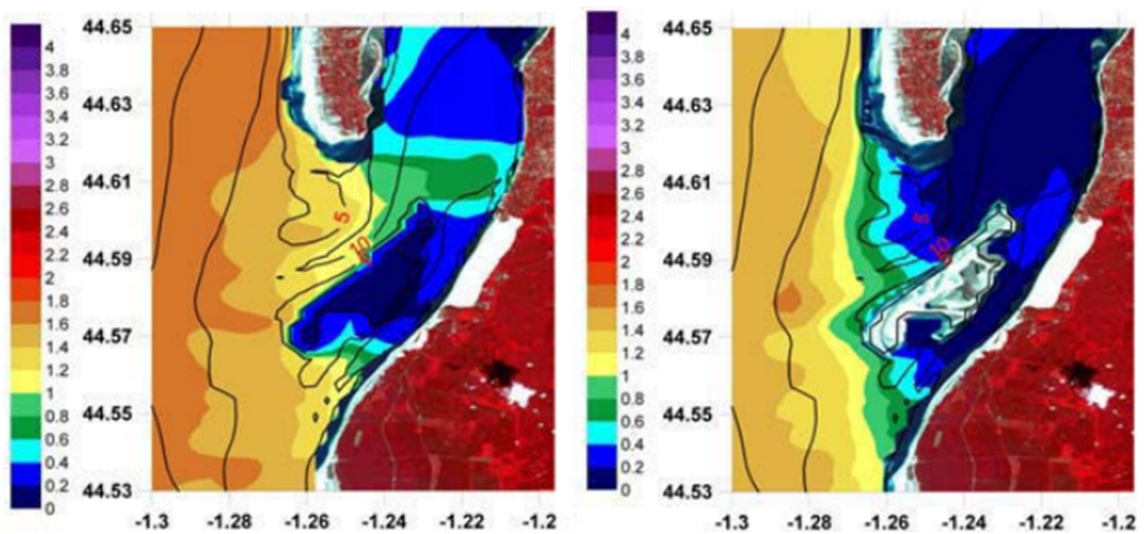
FIGURE 6.3 – Hauteur significative de la houle H_s à l'entrée des passes du Bassin d'Arcachon à marée haute et à marée basse. D'après Pedrerros et al. (2008).
