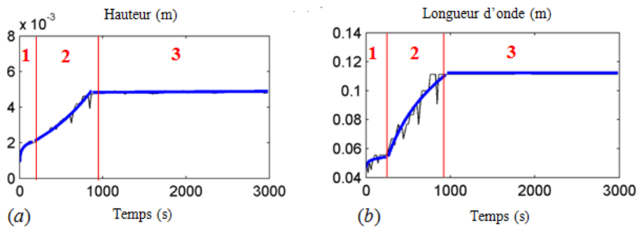
FIGURE B.2 – Évolution temporelle de (a) la moyenne des hauteurs du champ de dunes et (b) de leurs longueurs d'onde. Le trait noir montre le résultat brut et le trait bleu sa courbe de régression.
