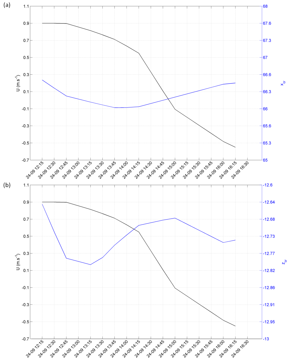
FIGURE 6.33 – Évolution temporelle de la vitesse et du déplacement horizontal de la crête (a) et du déplacement vertical de la crête (b) lors de la campagne du 24 Septembre 2013.
