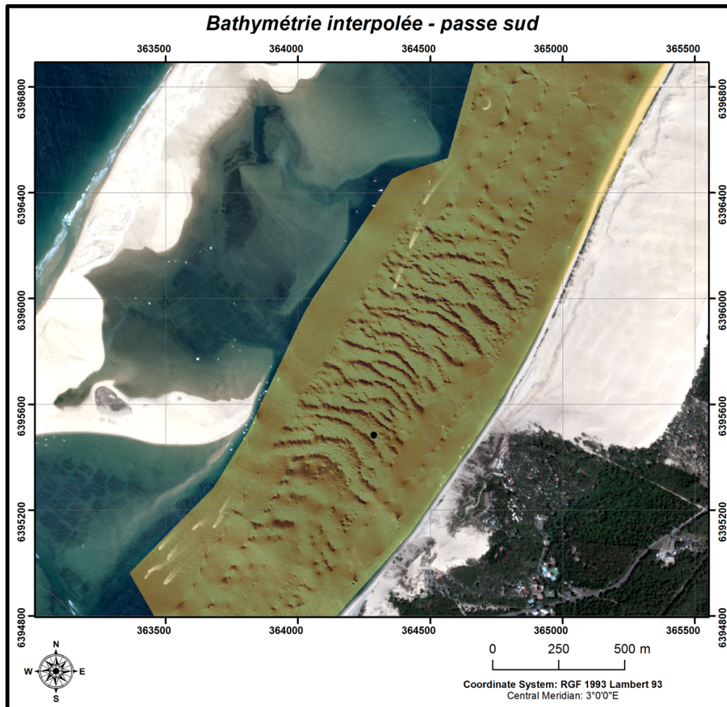
FIGURE 6.7 – Bathymétrie interpolée à partir des campagnes de mesure réalisées entre le 22 Avril et le 08 Juillet 2013. L'interpolation est réalisée sous ARCGIS avec une méthode des voisins naturels. La point noir représente la position des mesures sur le cycle de vives-eaux mortes-eaux (ADCP et ADV).
