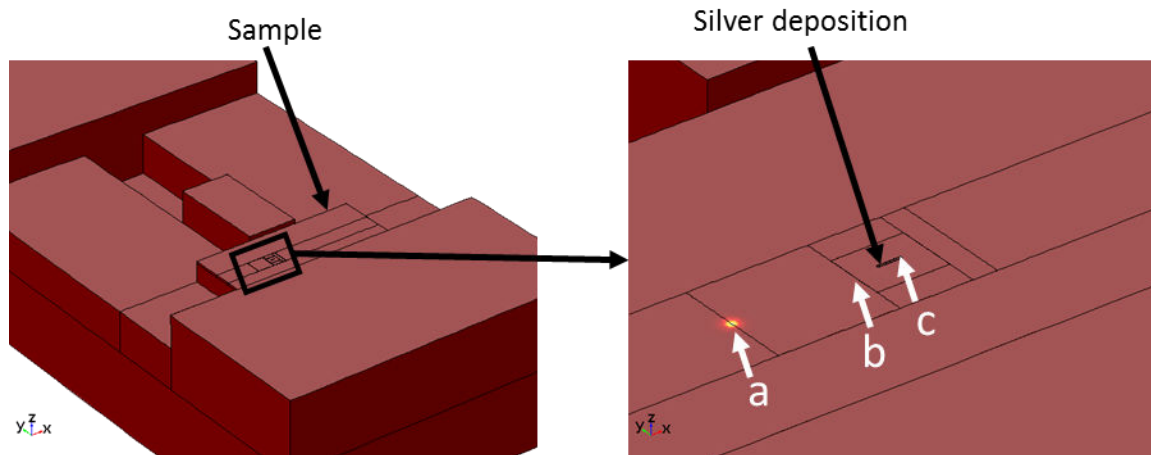
Figure 13 : (a) Représentation 3-D du système « porte échantillon / échantillon / déposition d'Ag » et (b) un grossissement sur le trajet du laser : une ligne droite entre les points « a » et « c ».
