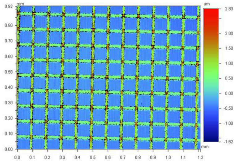
Figure 8 : Observation profilométrique d'un échantillon après dépôt d'un pattern de nanoparticules d'argent.
