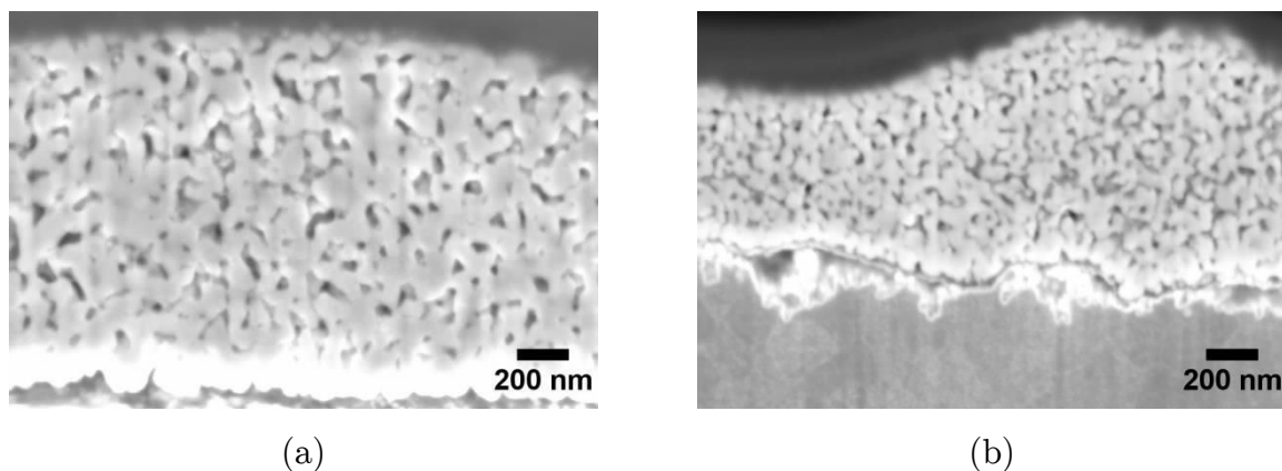
Figure 10 : Images MEB d'une section transverse d'une déposition de nano-particules d'argent après traitement thermique au laser avec une puissance de 8 W, une taille du spot de 85 µm et une vitesse de (a) 0.1 mm.s -1 et (b) 0.7 mm.s -1 .
