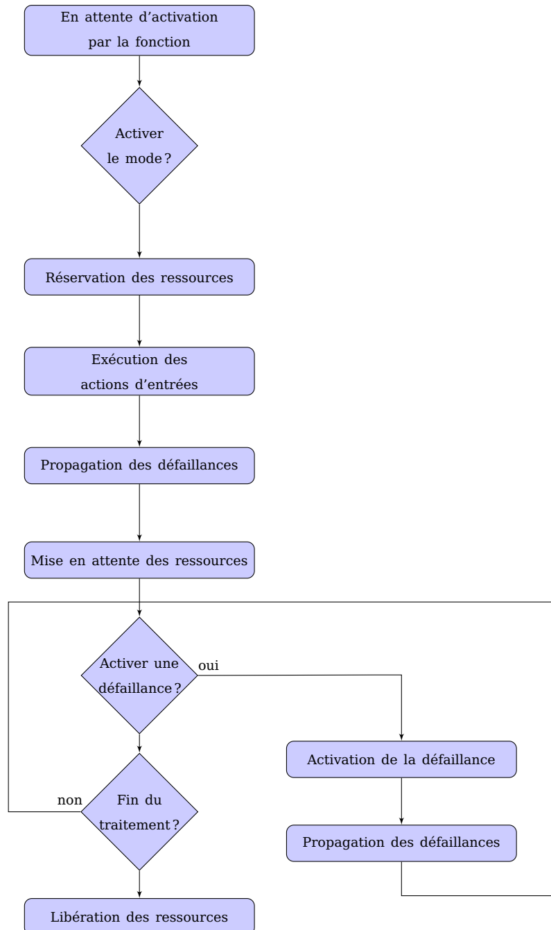
Figure 4.15: Fonctionnement des modes et interactions avec les ressources selon FIS
