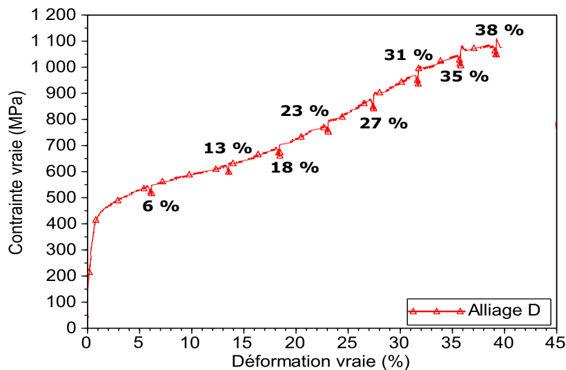
FIGURE 3.22 – Courbe de traction contrainte en fonction de la déformation vraie pour l'alliage D
