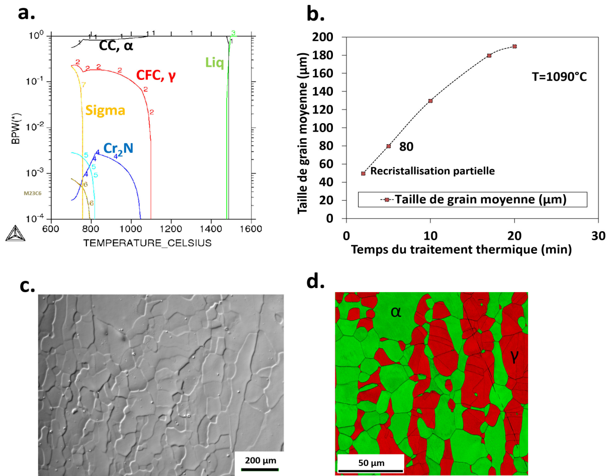
FIGURE 4.3 – Optimisation de la microstructure de la nuance ferritique a. fraction massique des phases en fonction de la température de recuit, calculs d'équilibre effectué avec Thermo-Calc ® b. taille de grains en fonction de la durée du traitement thermique c. micrographie optique suivant la direction normale de la nuance ferritique à l'issue du traitement de recristallisation. d. cartographie EBSD des phases suivant le sens normal pour la nuance duplex.
