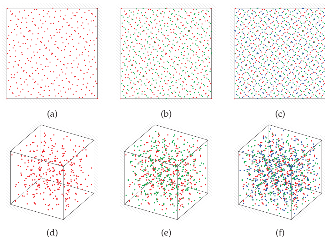
FIGURE 4.9 – Échantillonnage par séquences à basse discrétance dans différentes dimensions. (a), (b) et (c) : Les 340, 640 et 1024 premiers points de la séquence de Sobol dans l'espace \mathcal{U}^2 . (d), (e) et (f) : Les 340, 640 et 1024 premiers points de la séquence de Halton dans l'espace \mathcal{U}^3 . Les couleurs permettent de voir que les points déjà ajoutés ne sont pas déplacés lorsque le nombre de points augmente.
