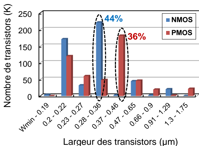
Figure 3-5 : Répartition du nombre de transistors en fonction de leur taille de la partie logique d'un circuit
