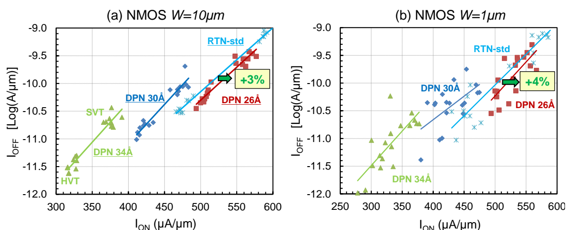
Figure 2-14 : Courbes de mérite I_{OFF}/I_{ON} d'un transistor NMOS de dimension W=10\mu\text{m} (a) et W=1\mu\text{m} (b)
