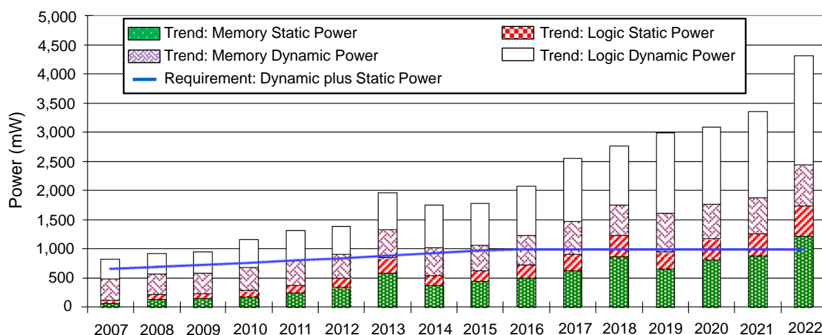
Figure 0-2 : Courbe montrant l'évolution de la consommation des systèmes complets sur puce (« Système On Chip » - SOC) en fonction des années de production pour des applications portables [ITRS'08]
