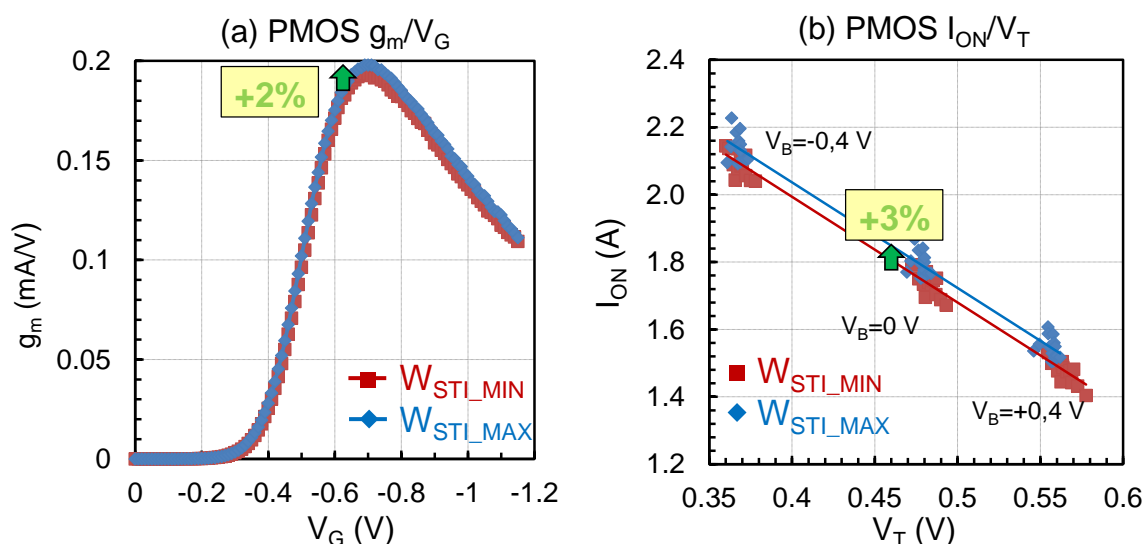
Figure 4-32 : Transconductance g_m en fonction de la tension de grille (a) et courant I_{ON} en fonction de la tension de seuil (b) d'un transistor PMOS dessiné avec différentes largeurs de STI
