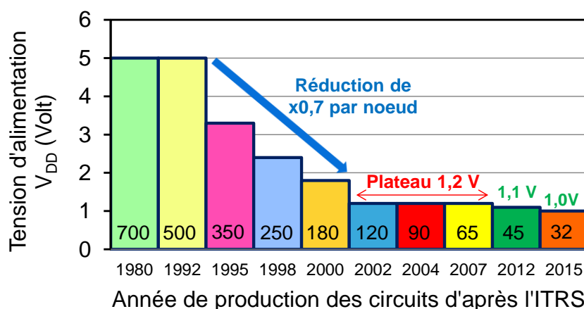
Figure 0-3 : Tension d'alimentation V_{DD} en fonction de l'année de production des circuits intégrés CMOS et du nœud technologique [Skotnicki'08]
