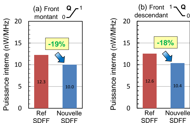
Figure 4-20 : Différence entre la puissance interne consommée par la cellule SDFF de référence et la nouvelle cellule SDFF lors d'un front montant (a) ou descendant (b) sur le signal de sortie
