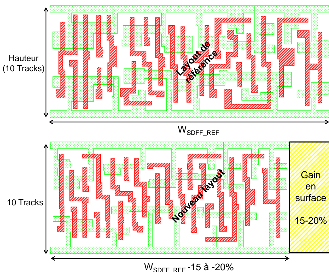
Figure 4-19 : Vue layout de la cellule SCAN de référence (a) et de la nouvelle cellule SCAN conçue avec les largeurs d'active réduites et l'utilisation des nouvelles règles de dessin (b)
