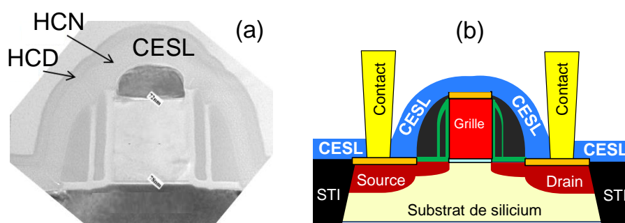
Figure 2-28 : Coupe TEM (a) et représentation schématique (b) d'un transistor GO1 montrant la couche d'arrêt de gravure des contacts (CESL) utilisée dans le procédé de fabrication standard et formée d'une couche de nitrure HCN et HCD
