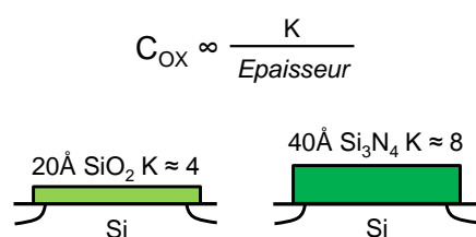
Figure 2-3 : Utilisation d'un oxyde « High-K » permettant d'augmenter l'épaisseur de l'oxyde sans impacter la valeur de C_{OX}
