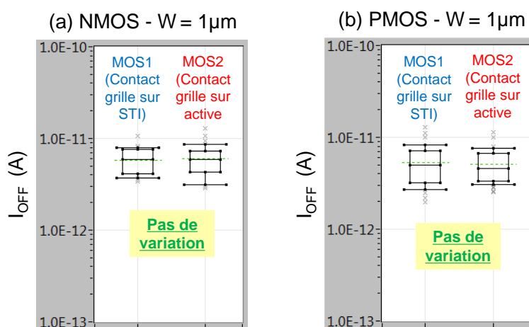
Figure 4-13 : Courant de fuite de drain ( I_{OFF} ) d'un transistor NMOS (a) et d'un transistor PMOS (b) de dimension W=1\mu\text{m} conçus avec le contact de grille sur STI (MOS1) ou sur active (MOS2)
