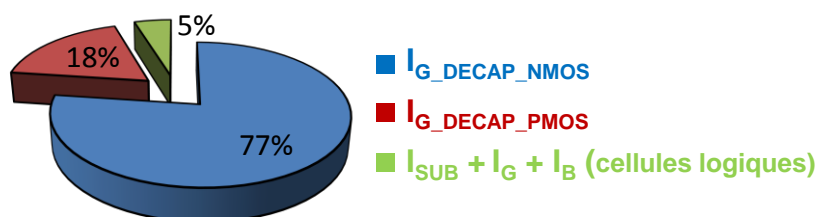
Figure 3-29 : Répartition des courants de fuite du DES1
