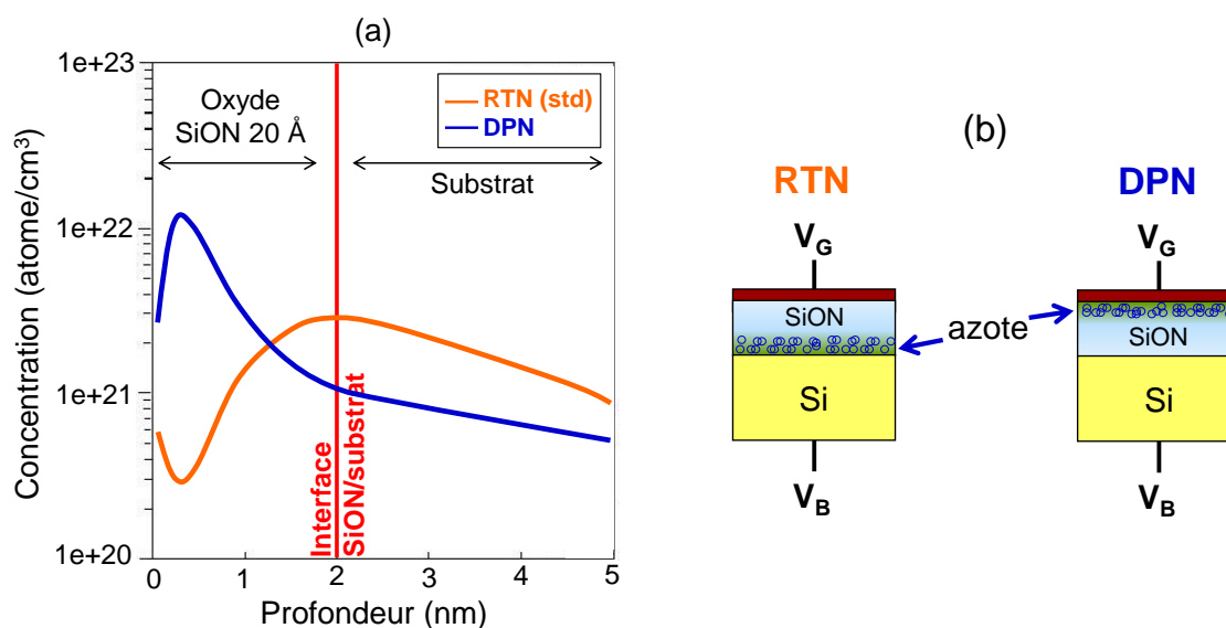
Figure 2-20 : Profils SIMS (a) et représentation graphique (b) montrant la concentration d'azote en fonction de la profondeur dans l'oxyde nitruré de type RTN et DPN. (b)
