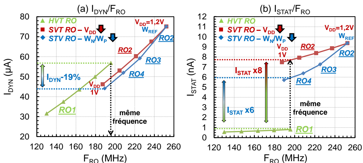
Figure 3-14 : Gains en courant dynamique (a) et dégradation du courant statique (b) obtenus entre un RO utilisant des transistors LVT et un RO utilisant des transistors HVT lors d'une réduction de la tension d'alimentation V_{DD} ou de la taille des transistors W_N/W_P
