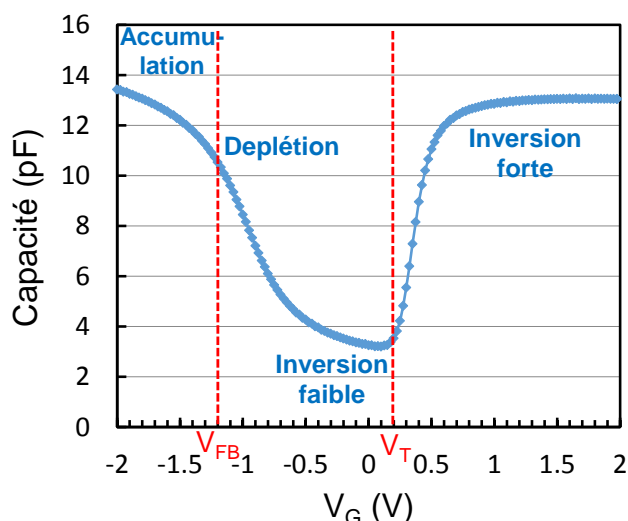
Figure 1-3 : Mesure d'une capacité MOS sur un substrat de type <p> en fonction de la tension de grille V_G (caractéristique C-V)
