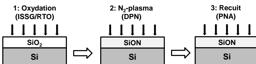
Figure 2-5 : Les trois différentes étapes du procédé DPN
