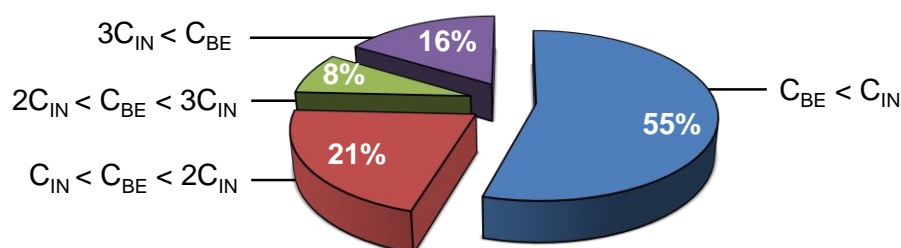
Figure 3-8 : Répartition des capacités C_{BE} et C_{IN} dans un circuit fabriqué en technologie e-NVM CMOS 80 nm
