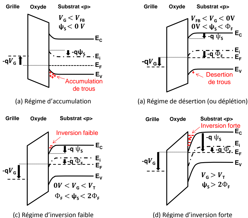
Figure 1-2 : Courbures de bande d'une structure MOS de type <p> dans les quatre différents régimes de fonctionnement
