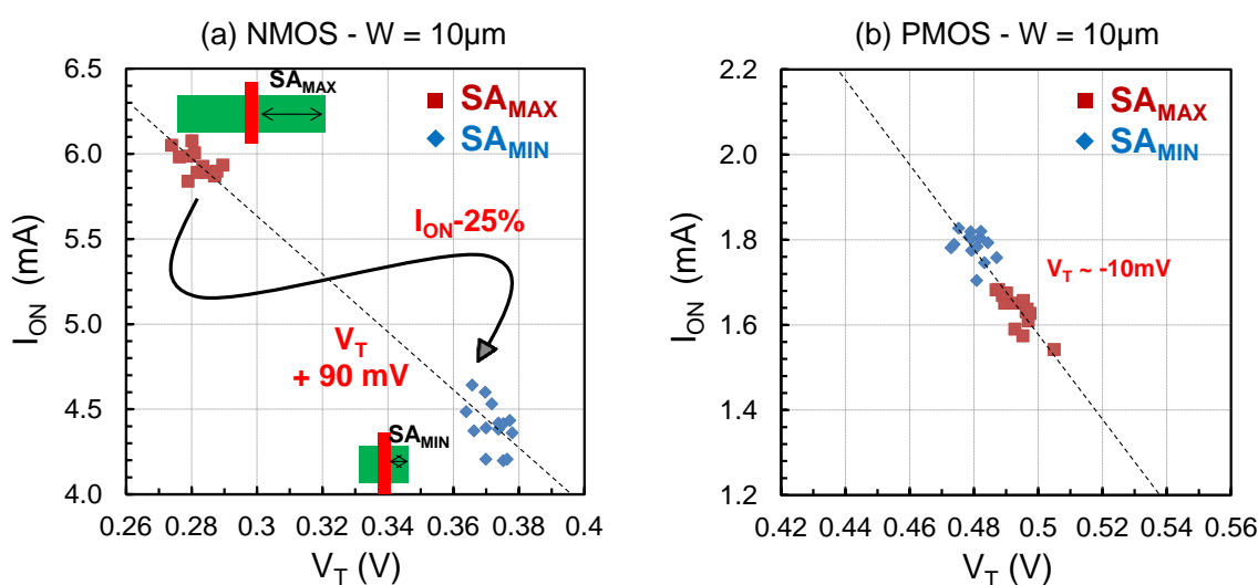
Figure 4-28 : Courbe de mérite I_{ON}/V_T d'un transistor NMOS (a) et d'un transistor PMOS (b) dessinés avec une distance grille/STI minimale ( SA_{MIN} ) et maximale ( SA_{MAX} )
