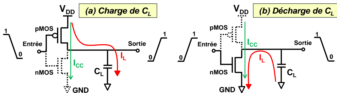
Figure 1-29 : Courant dynamique consommé lors d'une transition d'un état logique bas vers un état logique haut (a) et inversement (b) dans un inverseur CMOS chargeant une capacité C_L
