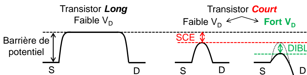
Figure 1-6 : Abaissement de la barrière de potentiel engendré par la réduction de la longueur de grille (SCE) et de la polarisation de drain (DIBL)
