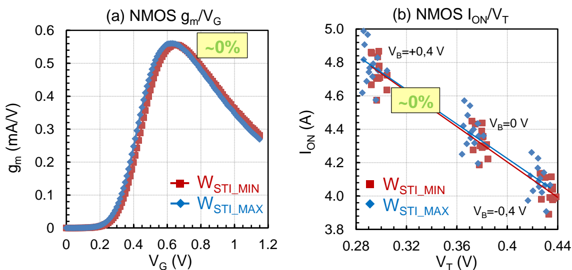
Figure 4-33 : Transconductance g_m en fonction de la tension de grille (a) et courant I_{ON} en fonction de la tension de seuil (b) d'un transistor NMOS dessiné avec différentes largeurs de STI
