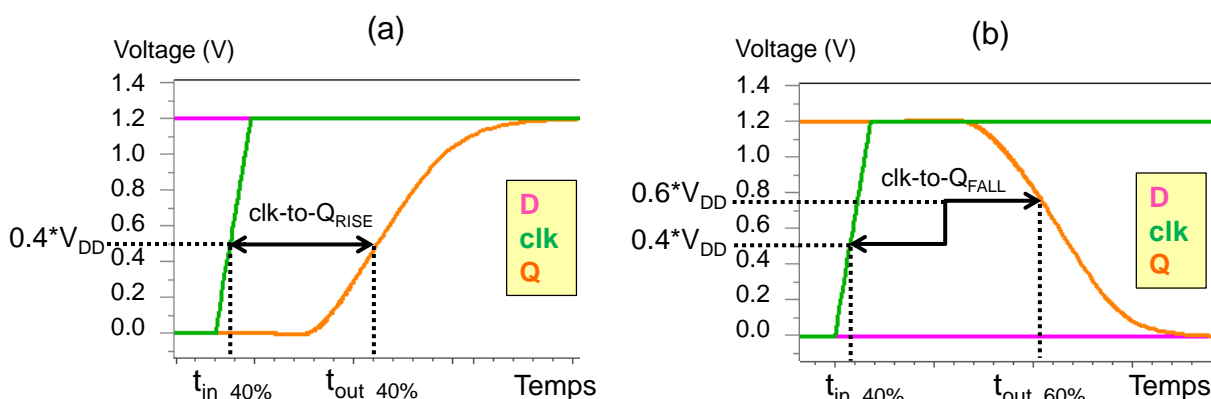
Figure 4-21 : Définition du temps de propagation « clock-to-Q » lors d'un front montant (a) et lors d'un front descendant (b) du signal de sortie Q
