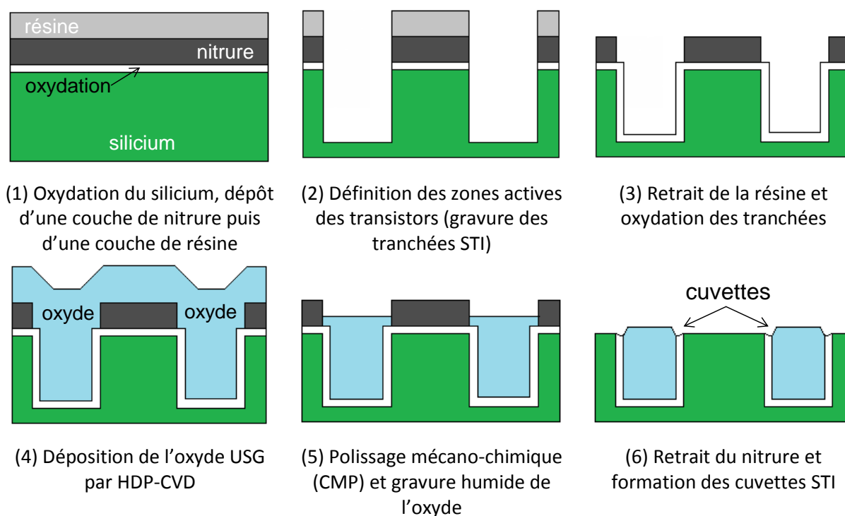
Figure 1-16 : Etapes de fabrication des tranchées d'isolation peu profondes (STI)
