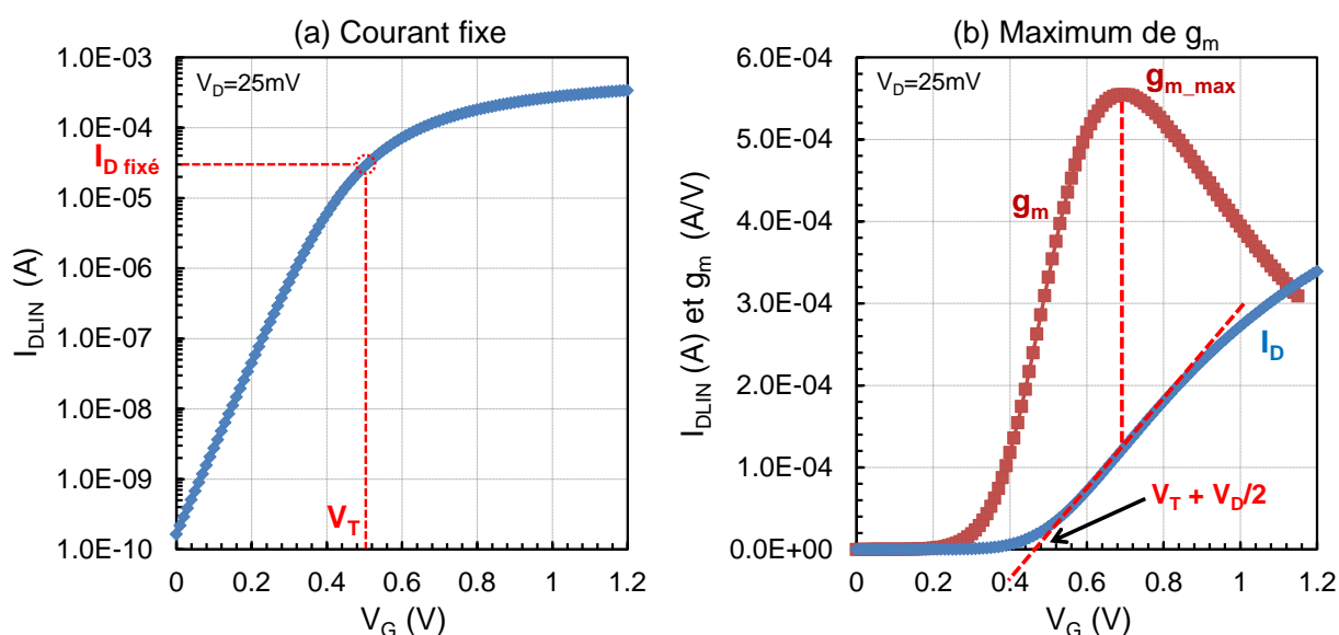
Figure 1-5 : Mesure de la tension de seuil des transistors par la méthode à courant fixe (a) ou par le maximum de la transconductance (b)
