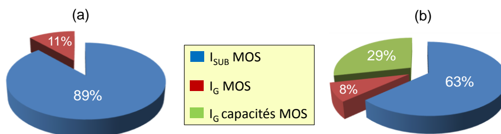
Figure 2-2 : Répartition du courant statique d'un circuit e-NVM fabriqué par STMicroelectronics Rousset sans (a) ou avec la contribution du courant de grille des capacités de découplage (b)
