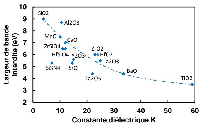
Figure 2-4 : Largeur de bande interdite des matériaux « High K » en fonction de leur constante diélectrique K [Robertson'04]
