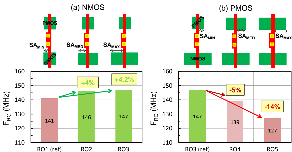
Figure 4-30 : Conception et fréquence d'oscillation des oscillateurs en anneau conçus avec des largeurs SA différentes sur les transistors NMOS (a) ou PMOS uniquement (b)
