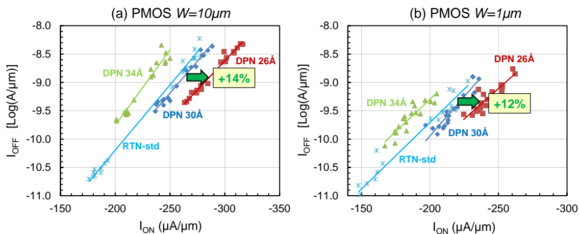
Figure 2-15 : Courbes de mérite I_{OFF}/I_{ON} d'un transistor PMOS de dimension W=10\mu\text{m} (a) et W=1\mu\text{m} (b)
