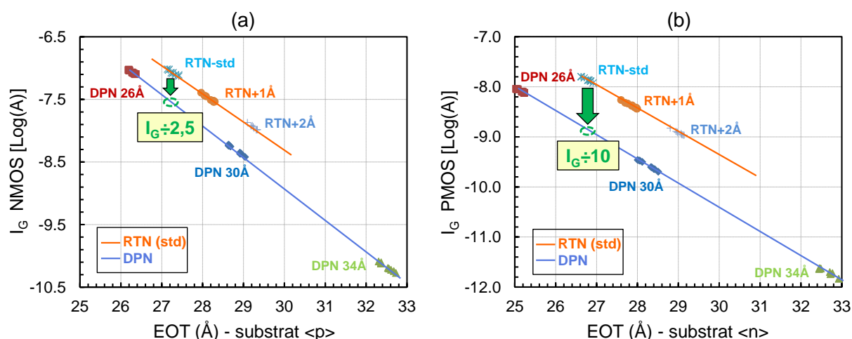
Figure 2-11 : Courant de grille d'un transistor NMOS (a) et d'un transistor PMOS (b) de dimension W=10\mu\text{m} et L=10\mu\text{m} en fonction de l'épaisseur électrique de l'oxyde pour les deux types de nituration RTN et DPN
