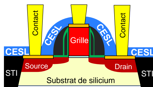
Figure 1-19 : Schéma d'un transistor MOS basse tension recouvert par la couche d'arrêt de gravure des contacts (CESL)
