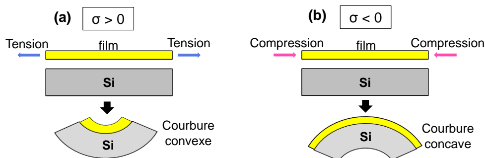
Figure 1-21 : Déformation du substrat de silicium en fonction de la nature de la contrainte mécanique exercée par le film CESL. Une contrainte en tension dans le film donne naissance à une courbure concave (a) et une contrainte en compression donne naissance à une courbure convexe (b)
