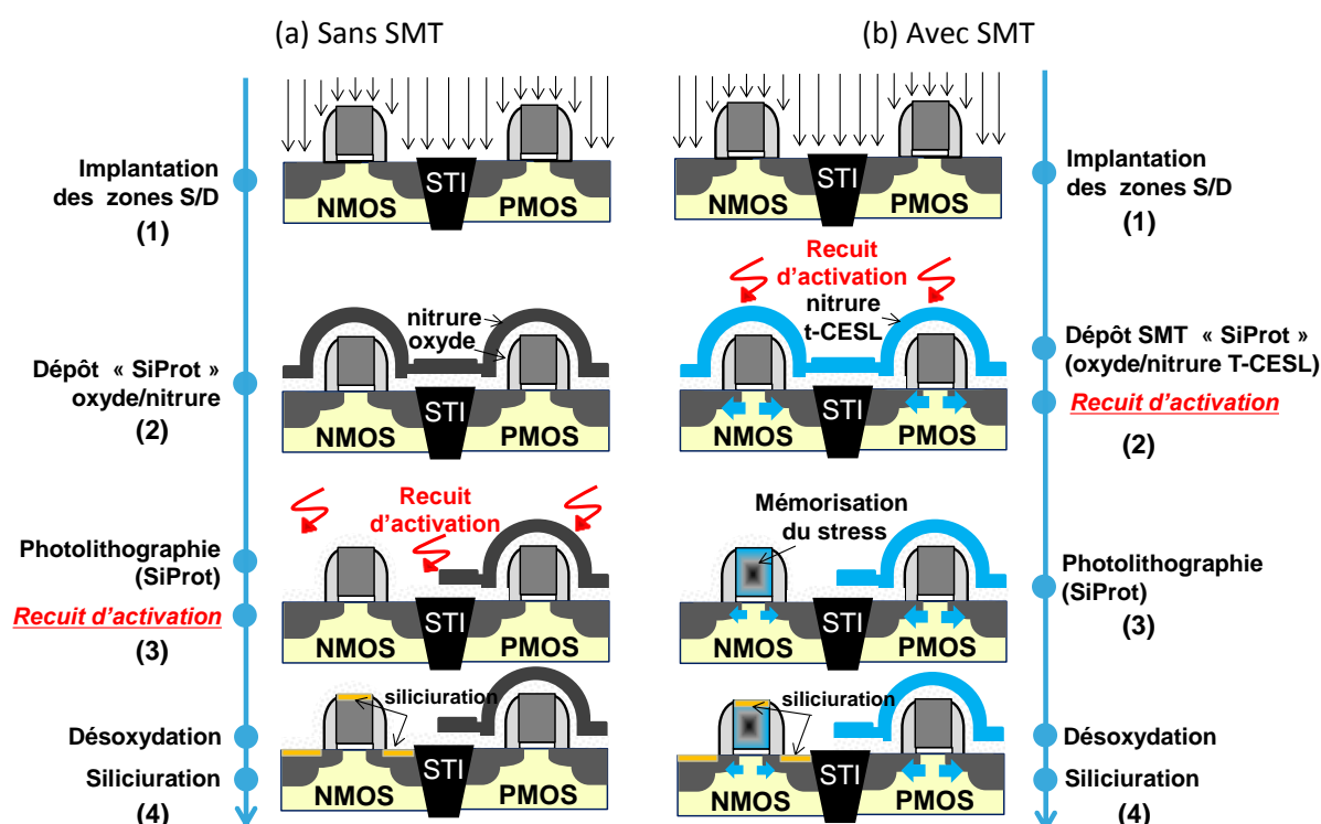
Figure 1-23 : Étapes de fabrication à partir de l'implantation des zones S/D jusqu'à la siliciuration (du transistor NMOS uniquement dans cet exemple) sans (a) et avec l'intégration du procédé SMT (b)
