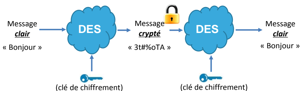
Figure 3-22 : Principe de fonctionnement de la fonction cryptographique du DES
