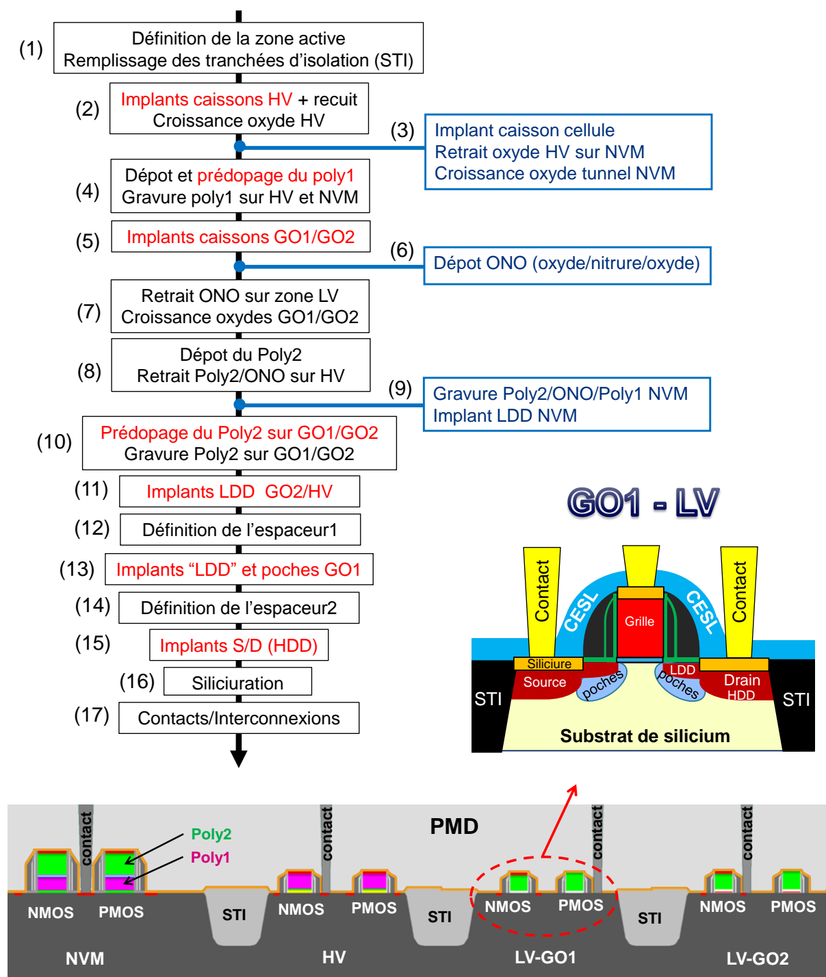
Figure 1-8 : Etapes de fabrication et représentation schématique des transistors MOS (LV, HV) et NVM fabriqués sur une plate-forme technologique e-NVM
