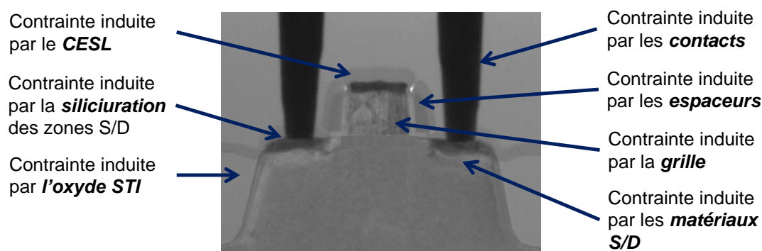
Figure 1-15 : Les principales contraintes induites par les procédés de fabrication lors de la fabrication d'un transistor MOSFET
