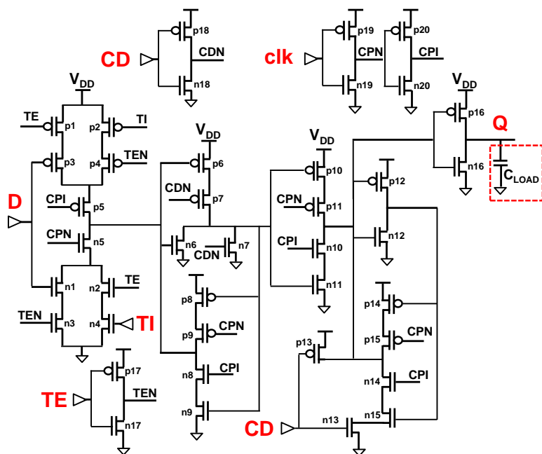
Figure 4-16 : Vue schématique (transistor) de la bascule SCAN choisie dans cette étude
