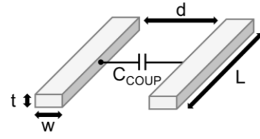
Figure 3-10 : Couplage capacitif entre deux lignes métalliques parallèles
