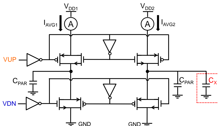
Figure 3-11 : Vue schématique de la structure utilisée pour mesurer la capacité C_{BE}
