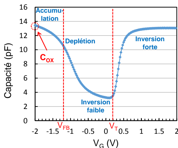
Figure 2-7: Mesure d'une capacité GO1 sur un substrat de type <p> permettant de remonter jusqu'à la valeur de l'épaisseur équivalente d'oxyde T_{ox}
