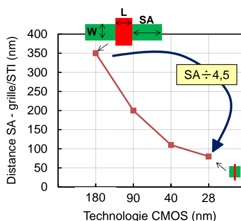
Figure 4-25 : Représentation graphique montrant la réduction de la distance entre la grille et le STI (SA) d'un transistor GO1 fabriqué dans les technologies 180 nm à 28 nm
