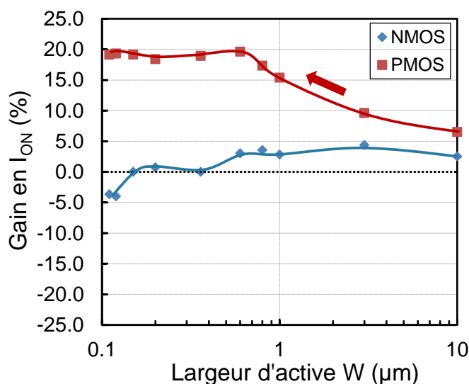
Figure 2-25 : Gain en courant I_{ON} en fonction de la largeur d'active d'un un transistor ayant une orientation cristalline \langle 100 \rangle par rapport à un transistor ayant une orientation cristalline \langle 110 \rangle
