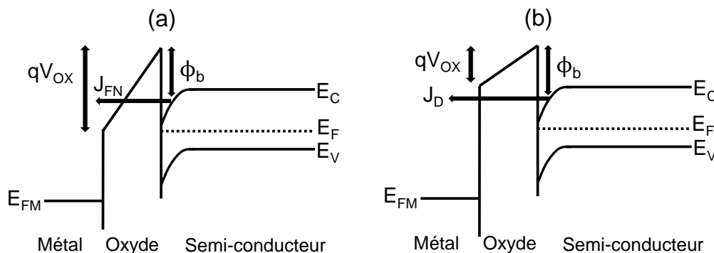
Figure 1-33 : Diagrammes de bandes d'une structure MOS de type <p> en inversion dans le cas d'un courant tunnel de type Fowler-Nordheim (a) et direct (b)
