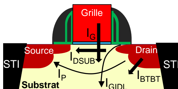
Figure 1-31 : Les principaux courants de fuite d'un transistor MOS
