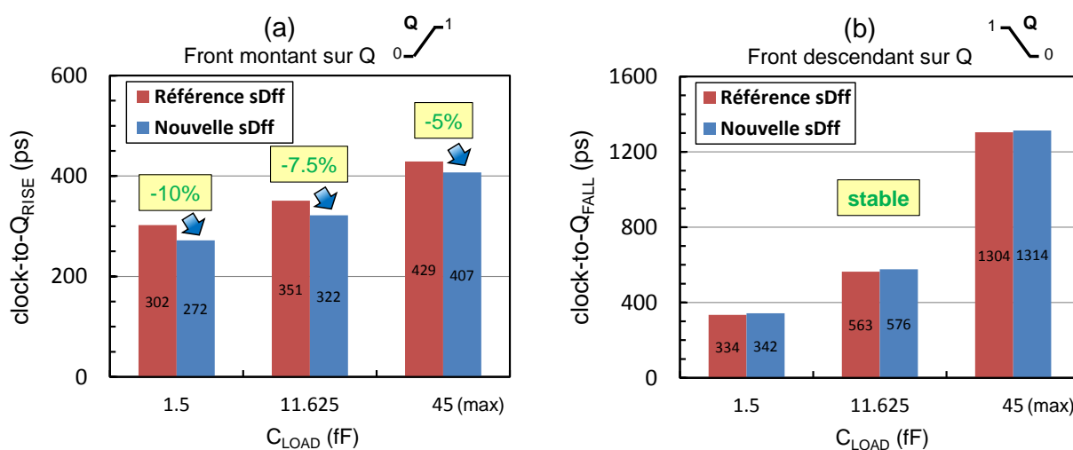
Figure 4-22 : Comparaison du temps de propagation « clock-to-Q » entre les deux bascules D lors d'un front montant (a) et lors d'un front descendant (b) du signal de sortie Q
