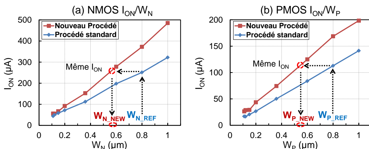
Figure 3-24 : Comparaison entre le courant I_{ON} d'un transistor NMOS (a) et d'un transistor PMOS (b) fabriqués avec le procédé de fabrication standard et le nouveau procédé de fabrication
