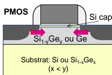
Figure 1-11 : Fabrication d'un substrat s-SiGe ou s-Ge contraint en compression pour augmenter les performances des transistors PMOS
