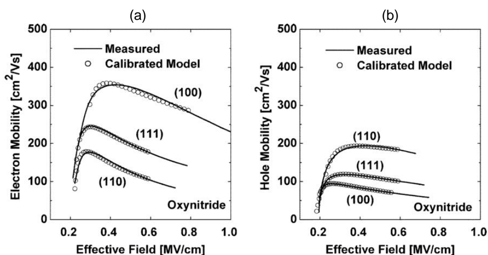
Figure 1-12 : Mobilité des électrons (a) et des trous (b) dans les différents plans cristallins (100), (110) et (111) d'après [Chang'04]
