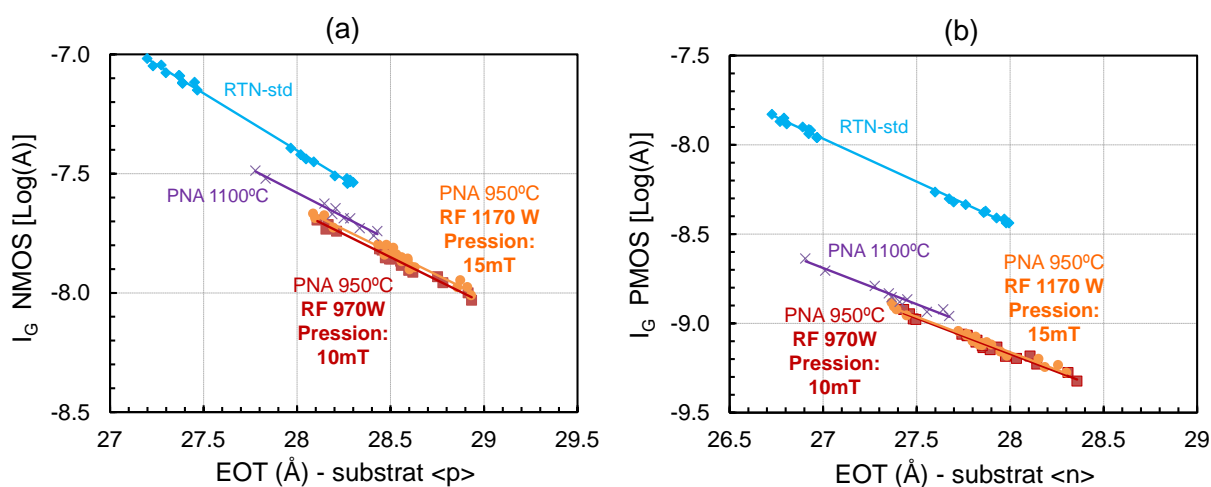
Figure 2-9 : Courant de grille d'un transistor NMOS (a) et d'un transistor PMOS (b) de dimension W=10\mu\text{m} et L=10\mu\text{m} en fonction de l'EOT pour différentes conditions de puissance et de pression dans la chambre DPN
