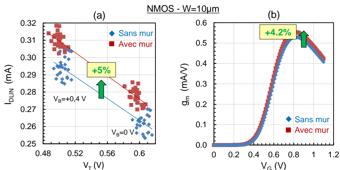
Figure 4-36 : Courbes de mérite I_{DLIN}/V_T (a) et g_m/V_G (b) d'un transistor NMOS dessiné avec et sans le mur en poly-silicium
