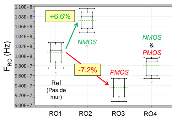
Figure 4-41 : Comparaison entre la fréquence d'oscillation des oscillateurs en anneau conçus avec ou sans le mur en poly-silicium
