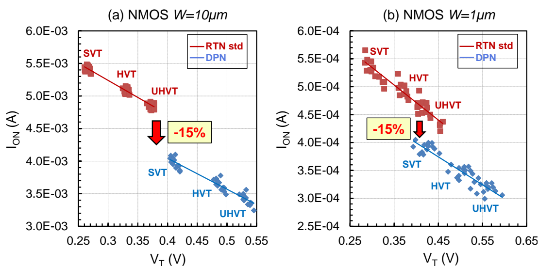
Figure 2-16 : Courbes de mérite I_{ON}/V_T d'un transistor NMOS de dimension W=10\mu\text{m} (a) et W=1\mu\text{m} (b) fabriqués avec le procédé standard RTN ou le procédé DPN
