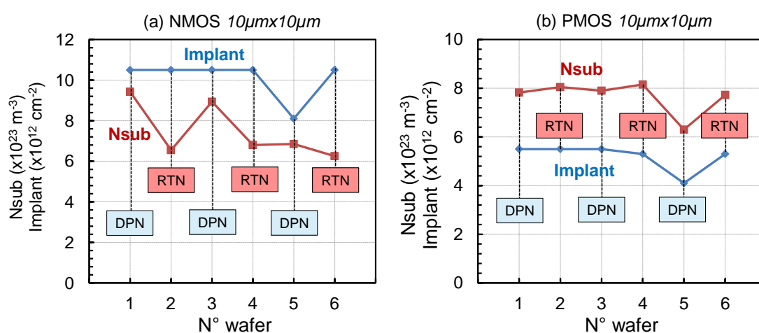
Figure 2-18 : Dopage du substrat de type <n> (a) et du substrat de type <p> (b) pour les plaquettes ayant été fabriquées avec le procédé RTN ou DPN
