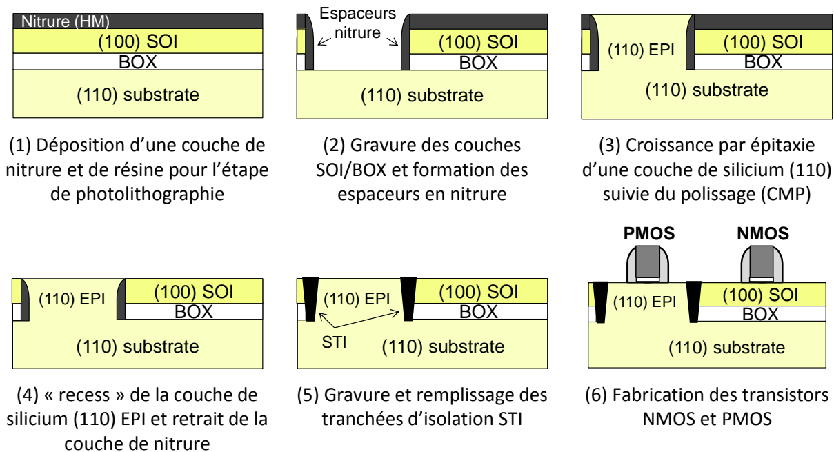
Figure 1-13 : Étapes de fabrication d'une technologie CMOS à orientation hybride (HOT) [Yang'03], [07]
