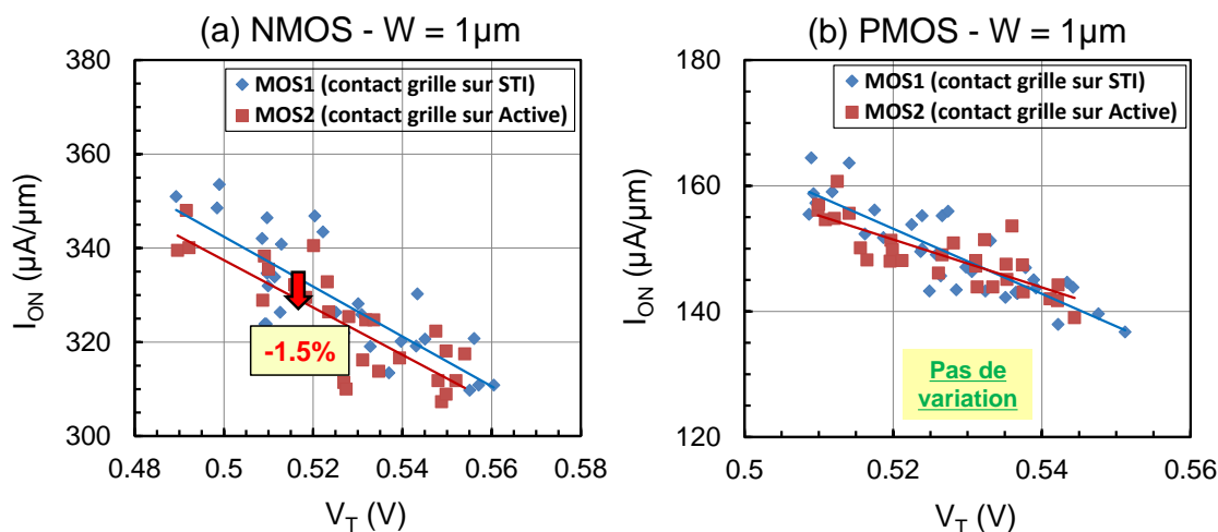
Figure 4-12 : Courbes de mérite I_{ON}/V_T d'un transistor NMOS (a) et d'un transistor PMOS (b) de dimension W_{MIN} fabriqué avec le contact de grille sur STI (MOS1) ou sur active (MOS2)
