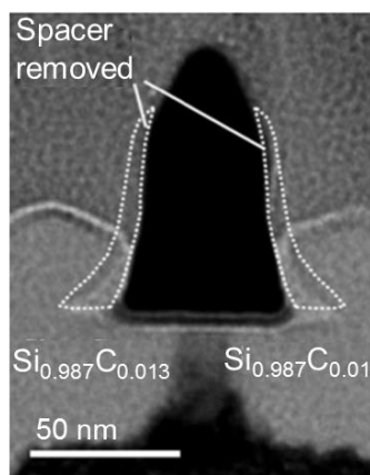
Figure 1-18 : Coupe TEM d'un transistor NMOS fabriqué avec l'intégration du Si:C dans les zones S/D pour augmenter la contrainte mécanique en tension dans le canal [Ang'04], [Chui'07]
