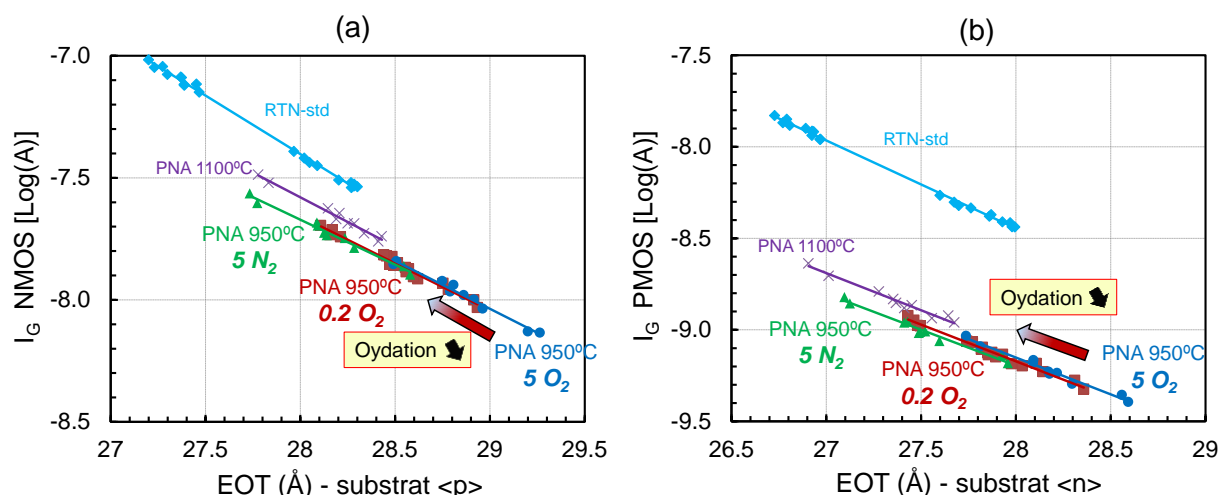
Figure 2-10 : Courant de grille d'un transistor NMOS (a) et d'un transistor PMOS (b) de dimension W=10\mu\text{m} et L=10\mu\text{m} en fonction de l'EOT pour différents types et différentes quantités d'espèces utilisés pendant le recuit PNA
