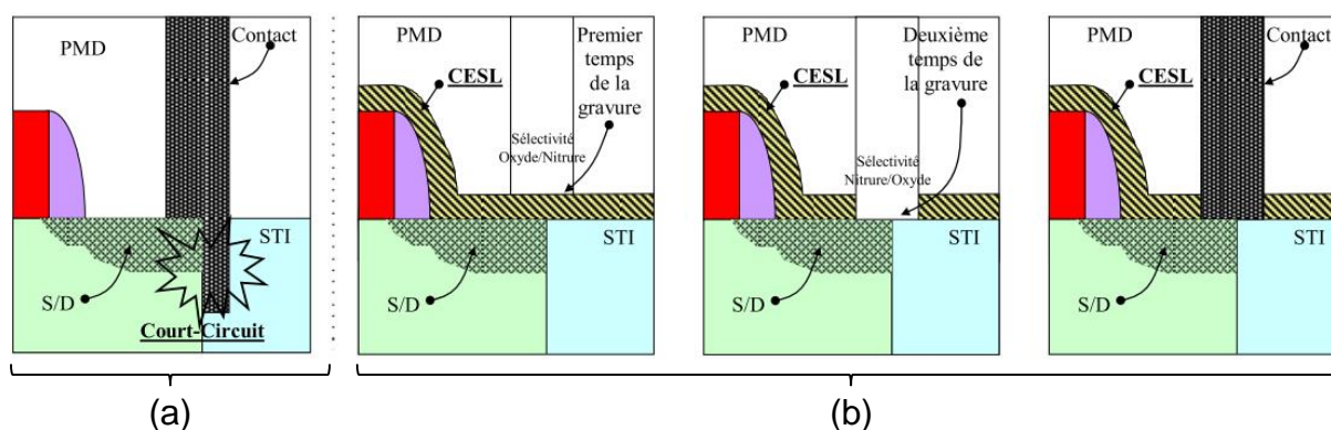
Figure 1-20 : Procédé de gravure des contacts sans le CESL (a) et avec l'introduction du CESL évitant les court-circuits (b)
