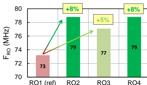
Figure 4-10 : Fréquence d’oscillation des RO conçus avec les inverseurs présentés dans la Figure 4-9
