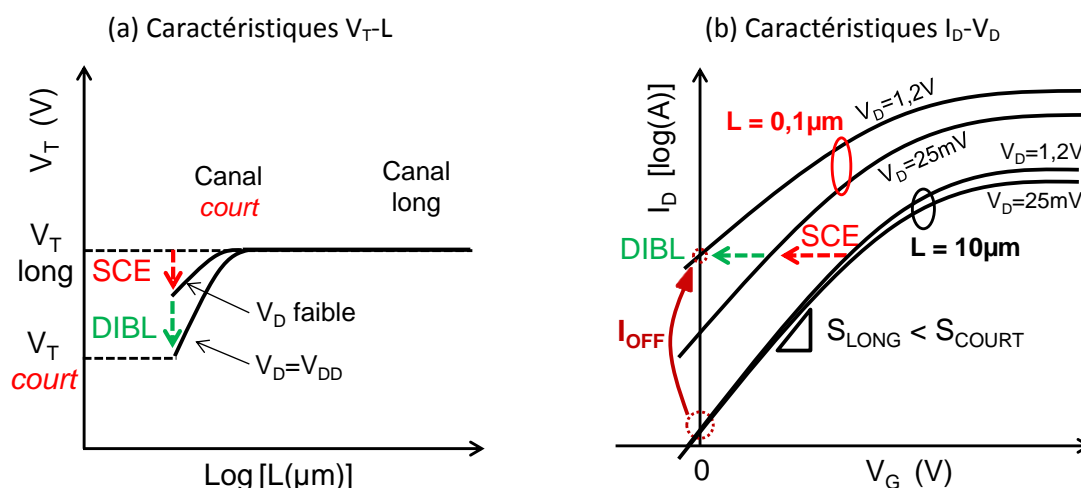
Figure 1-7 : Impact des effets canaux courts SCE et DIBL sur les caractéristiques V_T -L (a) et I_D - V_G (b)
