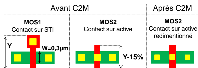
Figure 4-11 : Conception d'un transistor MOS GO1 avec le contact grille sur l'oxyde STI (MOS1) ou sur la zone active du transistor avant et après redimensionnement lors de l'étape de transformation « CAD to Mask » (MOS2)
