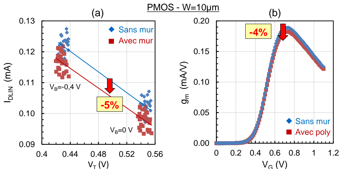
Figure 4-37 : Courbes de mérite I_{\text{DLIN}}/V_T (a) et g_m/V_G (b) d'un transistor PMOS dessiné avec et sans le mur en poly-silicium
