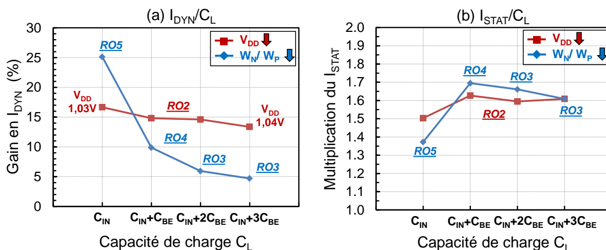
Figure 3-20 : Gains en courant dynamique (a) et multiplication du courant statique (b) obtenus entre le RO fabriqué avec le procédé de référence et le nouveau procédé de fabrication pour une réduction de W_N/W_P ou de V_{DD} et différents rapports entre C_{IN} et C_{BE}
