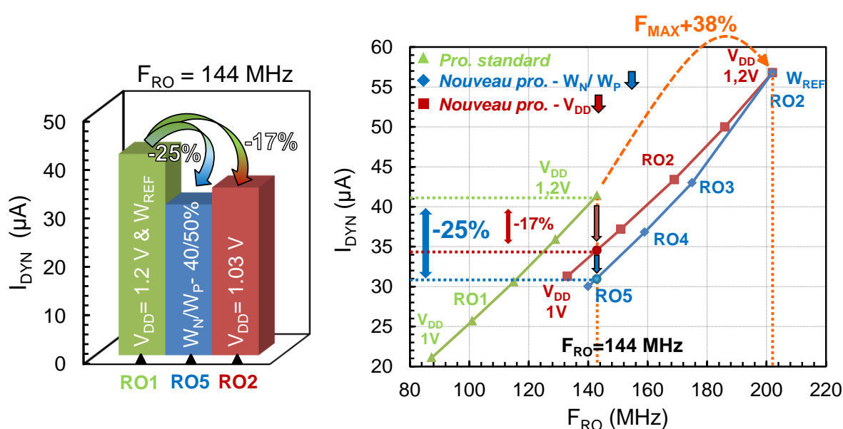
Figure 3-17 : Gains en courant dynamique obtenus entre le procédé de fabrication de référence et le nouveau procédé de fabrication pour une réduction des largeurs d'active W_N/W_P ou de l'alimentation V_{DD} lorsque C_L = C_{IN}
