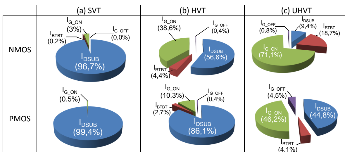
Figure 2-1 : Répartition des différents courants de fuite dans un transistor NMOS et dans un transistor PMOS de type SVT (a) HVT (b) et UHVT (c) de longueur L = 90 nm et de largeur W = 1\mu\text{m}
