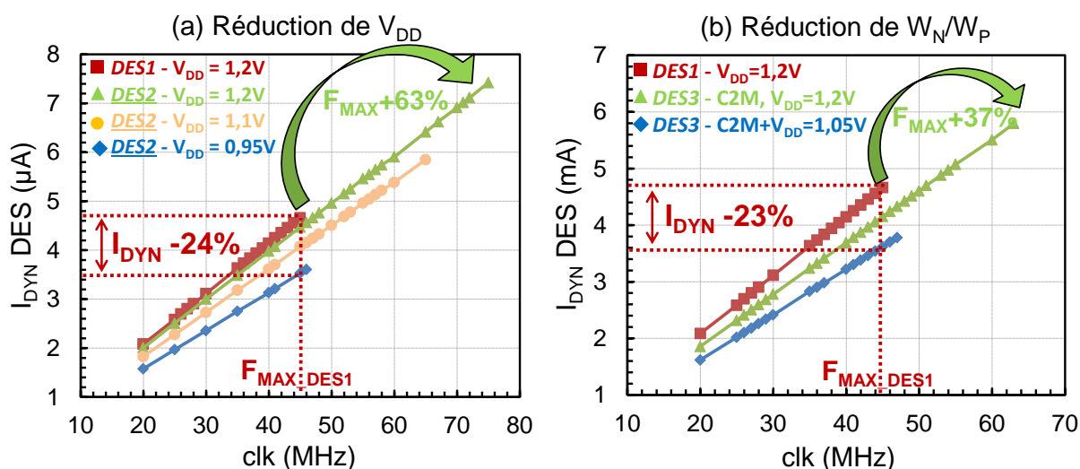
Figure 3-27 : Réduction du courant dynamique consommé par le DES avec l'utilisation du nouveau procédé de fabrication, lors d'une diminution de la tension d'alimentation V_{DD} (a) ou de la largeur des transistors (b)
