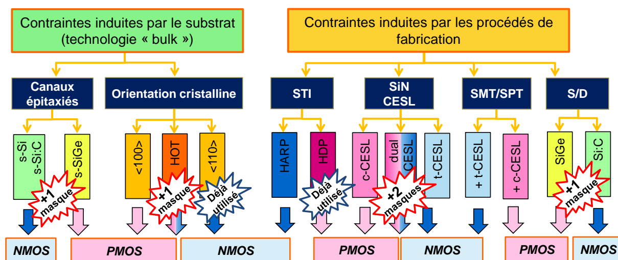
Figure 1-26 : Résumé des solutions technologiques permettant d'introduire des contraintes mécaniques dans le canal et d'augmenter la mobilité des transistors MOS
