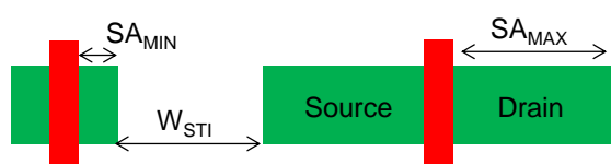
Figure 4-26 : Vue layout d'un transistor dessiné avec une distance grille/STI minimale ( SA_{MIN} ) et une distance grille/STI maximale ( SA_{MAX} )
