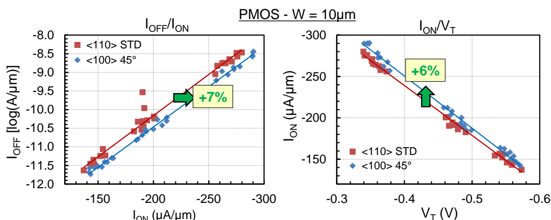
Figure 2-22 : Courbes de mérite I_{OFF}/I_{ON} (a) et I_{ON}/V_T (b) d'un transistor PMOS GO1 de largeur W = 10\ \mu\text{m} fabriqué avec une orientation cristalline standard <110> et une orientation tournée à 45° <100>
