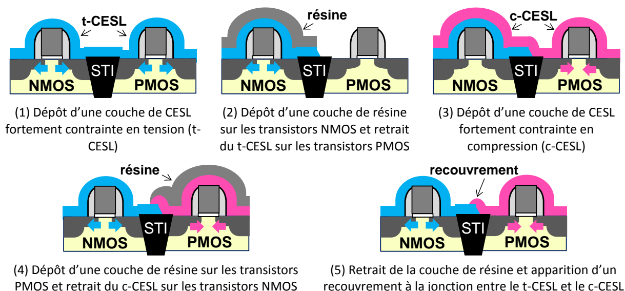
Figure 1-22 : Étapes de fabrication du procédé DSL (Dual CESL) intégrant les deux types de CESL
