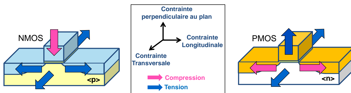
Figure 2-26 : Vue schématique des types de contraintes à appliquer pour augmenter la mobilité des transistors dans les deux orientations cristallines étudiées <100> (standard) et <100> (45°)
