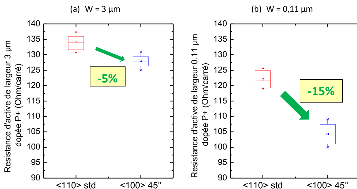
Figure 2-27 : Résistance carrée mesurée sur un barreau d'active P+ non siliciuré de largeur 3 µm (a) et 0,11 µm (b)
