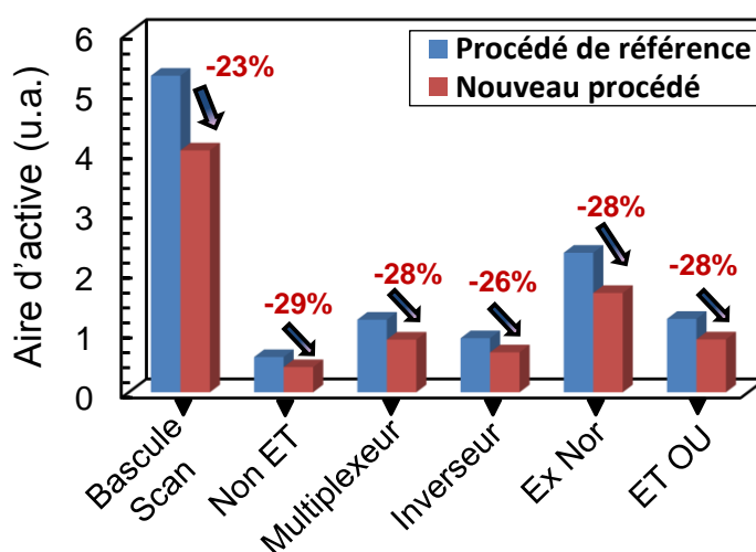
Figure 3-28 : Réduction de la zone active des cellules logiques utilisées dans le circuit DES avec l'utilisation du nouveau procédé de fabrication et du script C2M
