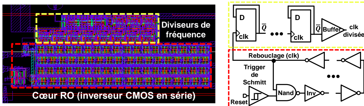
Figure 3-1 : Vue layout et vue schématique de l'oscillateur en anneau utilisé dans cette étude
