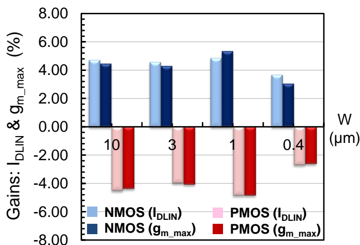
Figure 4-38 : Gains en courant linéaire ( I_{\text{DLIN}} ) et sur la transconductance observés sur des transistors NMOS et PMOS de différentes largeurs
