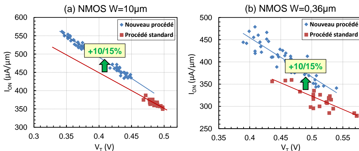
Figure 2-35 : Courbes de mérite I_{ON}/V_T d'un transistor NMOS de dimension W = 10 \mu\text{m} (a) et W = 0,36 \mu\text{m} (b) fabriqués avec le procédé de fabrication standard et le nouveau procédé de fabrication
