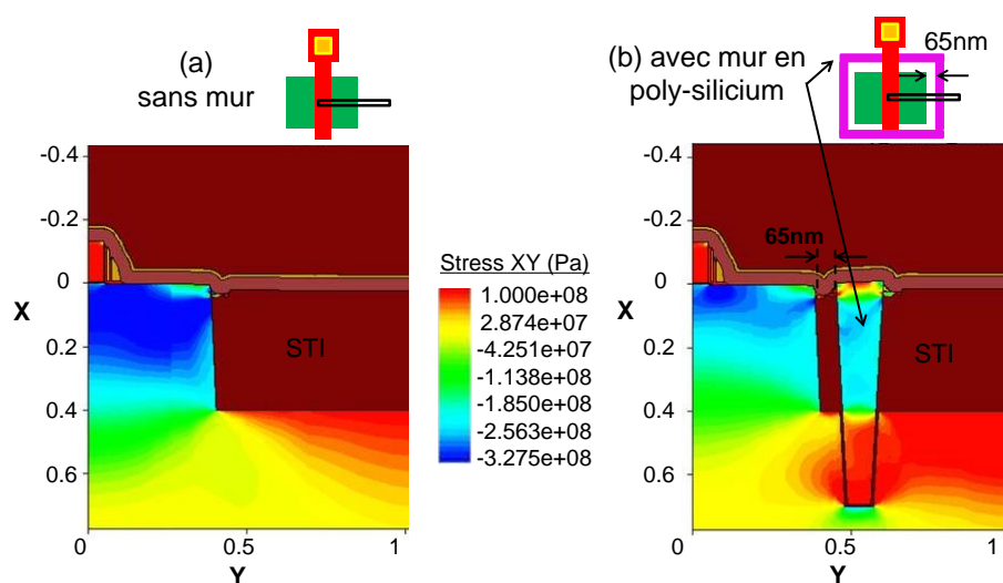
Figure 4-34 : Simulation du stress résiduel dans le canal des transistors sans (a) ou avec l'insertion d'un mur anti-stress conçu avec du poly-silicium (b)
