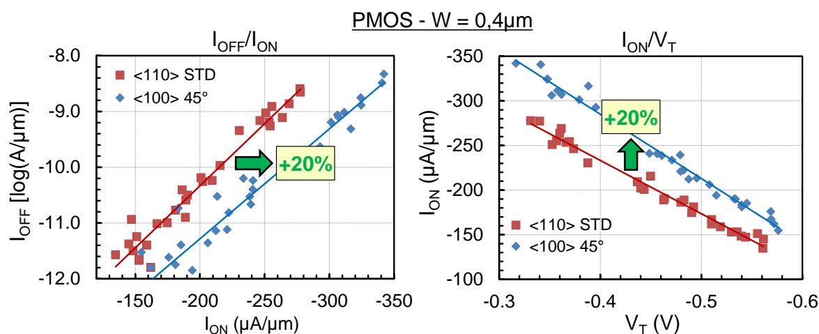
Figure 2-23 : Courbes de mérite I_{\text{OFF}}/I_{\text{ON}} (a) et I_{\text{ON}}/V_T (b) d'un transistor PMOS GO1 de largeur W = 0,4 \mu\text{m} fabriqué avec une orientation cristalline standard \langle 110 \rangle et une orientation tournée à 45^\circ \langle 100 \rangle
