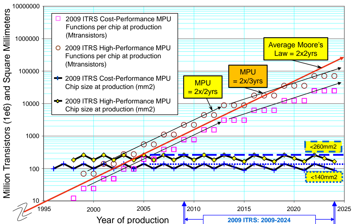
Figure 0-1 : Nombre de transistors fabriqués sur un circuit intégré en fonction de l'année de production en superposition avec la « loi de Moore » [ITRS'10]
