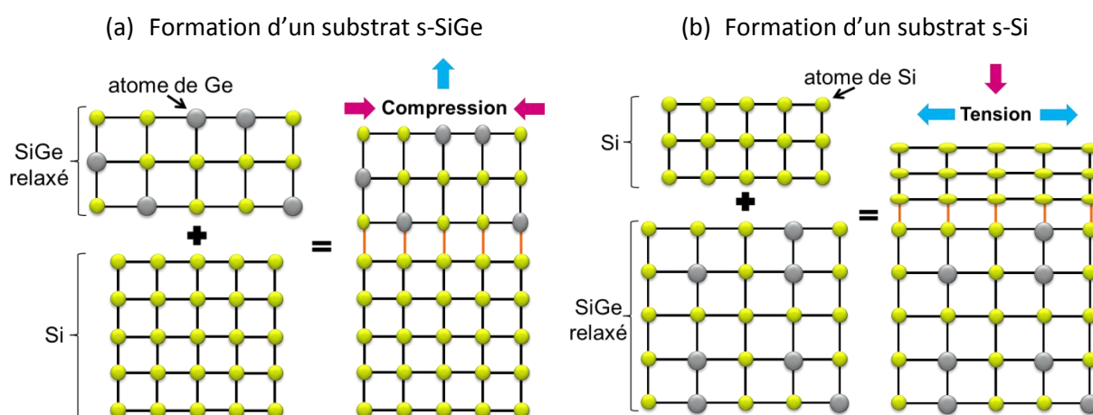
Figure 1-9 : Représentation schématique de l'état de contrainte lors de l'insertion d'une couche de SiGe relaxée sur un substrat de silicium « s-SiGe » (a) ou de l'insertion d'une couche de silicium sur un substrat de SiGe relaxé « s-Si » (b)
