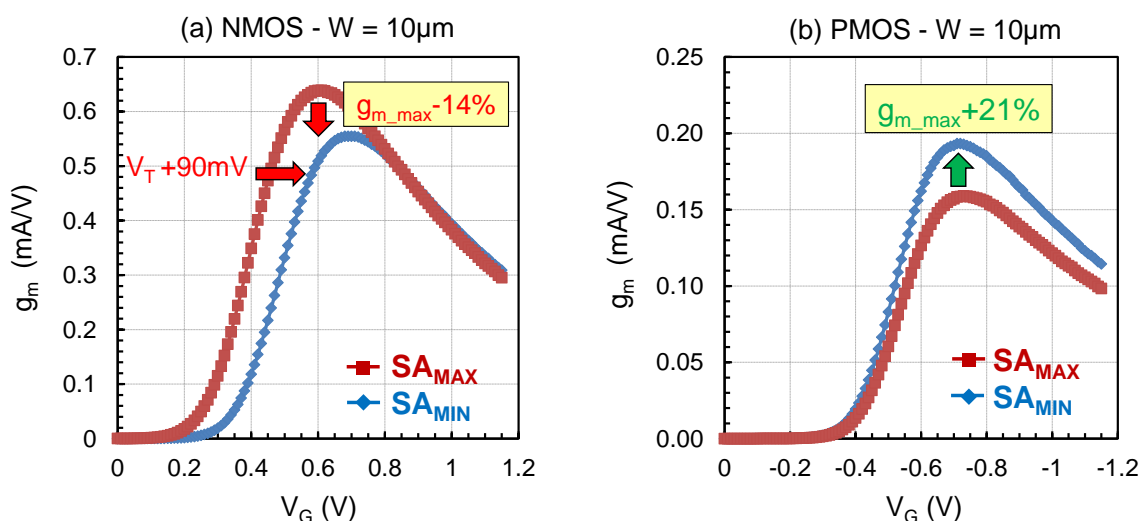
Figure 4-27 : Transconductance g_m en fonction de la tension de grille pour différentes distances entre la grille et le STI (SA) dans le cas d'un transistor NMOS (a) et dans le cas d'un transistor PMOS (b)
