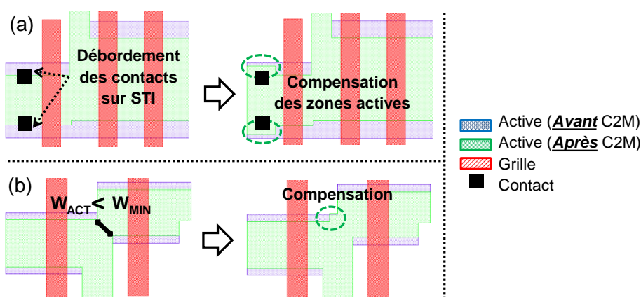
Figure 3-25 : Compensation des zones actives autour des contacts S/D (b) et lorsque la zone active devient inférieure à la largeur minimale ( W_{MIN} ) autorisée par le DRM
