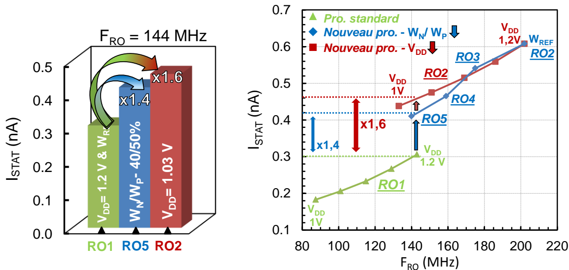
Figure 3-18 : Evolution du courant statique entre le procédé de fabrication de référence (RO1) et le nouveau procédé de fabrication pour une réduction de W_N/W_P (RO5) ou de V_{DD} (RO2) lorsque C_L = C_{IN}
