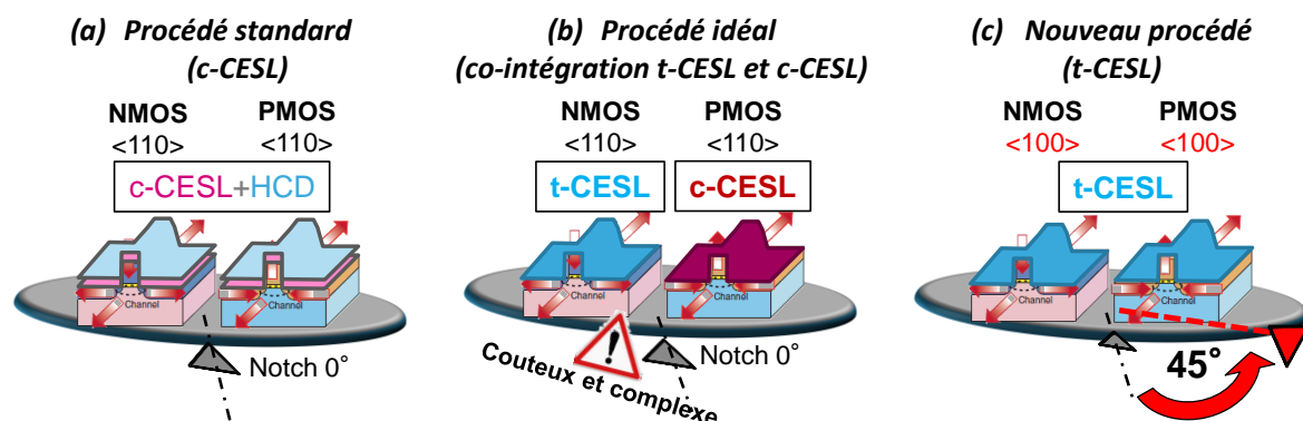
Figure 2-29 : Types de CESL utilisés dans le cas du procédé standard (a), d'une co-intégration DSL (b) et dans le cas du nouveau procédé de fabrication retenu dans ces travaux (c)
