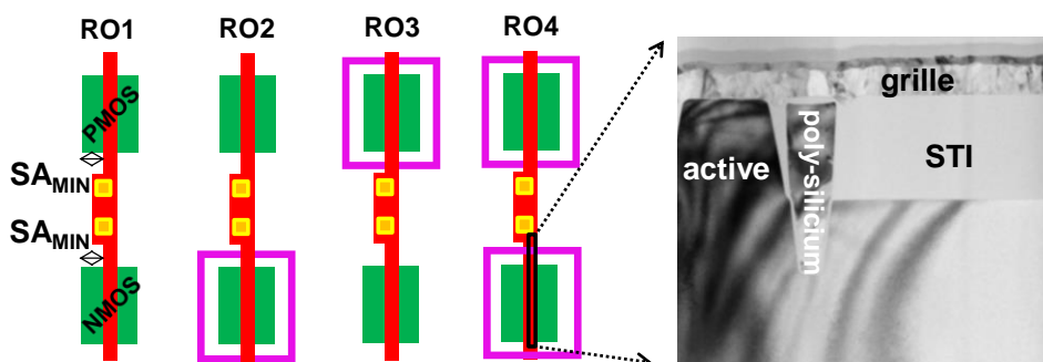
Figure 4-40 : Conception des inverseurs utilisés dans les oscillateurs en anneau pour étudier le comportement dynamique des transistors GO1 avec l'insertion du mur en poly-silicium
