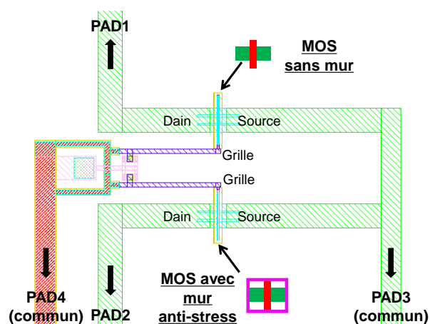
Figure 4-35 : Vue layout de la structure de test permettant de mesurer les paramètres électriques d'un transistor conçu avec ou sans le mur anti-stress
