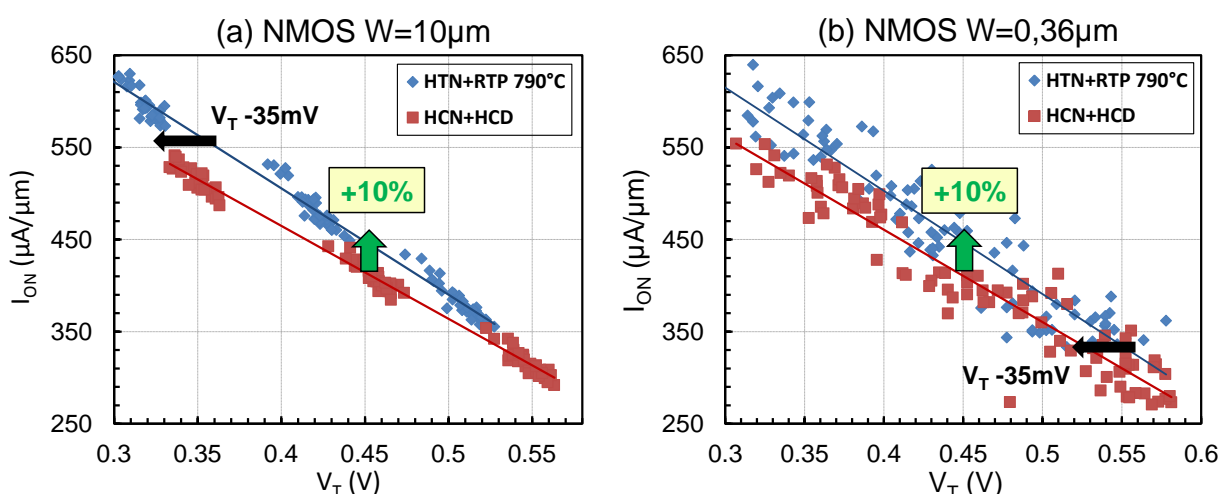
Figure 2-31 : Courbes de mérite I_{ON}/V_T d'un transistor NMOS de dimension W = 10 \mu\text{m} (a) et W = 0,36 \mu\text{m} (b) fabriqués avec un nitrure standard HCN et un nitrure fortement contraint en tension HTN
