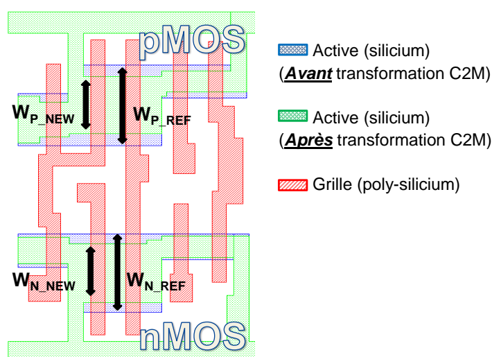
Figure 3-23 : Réduction de la largeur des transistors opérée par le script C2M sur une cellule standard
