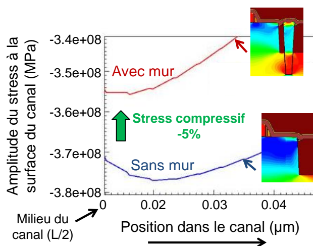
Figure 4-39 : Amplitude du stress résiduel pris au milieu et à la surface du canal dans le cas d'un transistor fabriqué avec ou sans le mur anti-stress en poly-silicium
