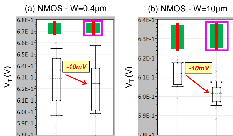
Figure 4-43 : Tension de seuil V_T d'un transistor NMOS de dimension W = 0.4 \mu\text{m} (a) et W = 10 \mu\text{m} (b) dessiné avec ou sans le mur en poly-silicium
