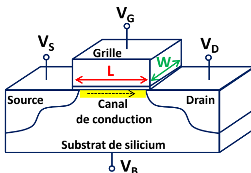
Figure 1-1 : Schéma d'un transistor MOSFET
