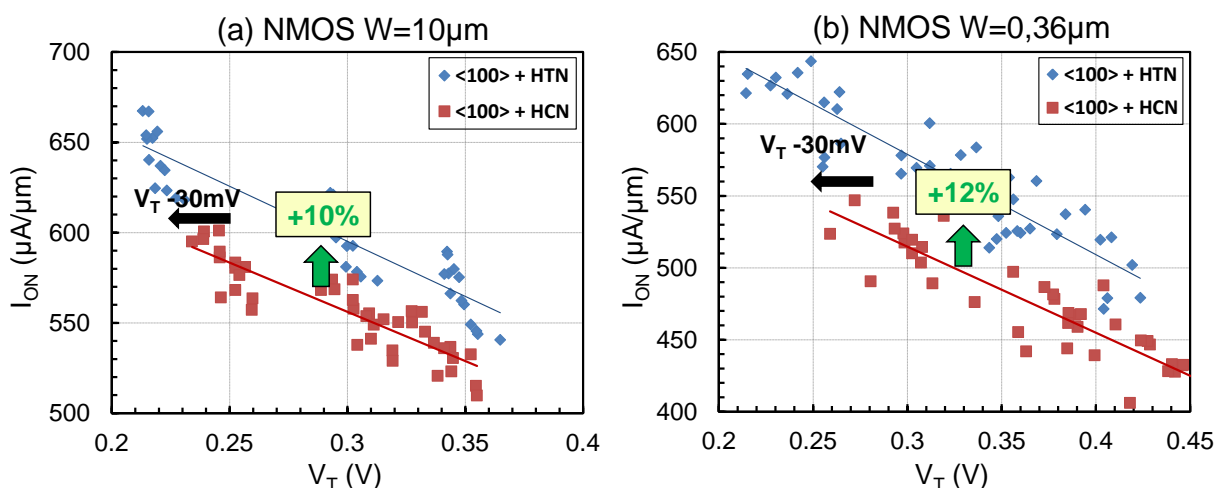
Figure 2-32 : Courbes de mérite I_{ON}/V_T d'un transistor NMOS de dimension W = 10 \mu\text{m} (a) et W = 0,36 \mu\text{m} (b) fabriqués avec un nitrure standard HCN et un nitrure fortement contraint en tension HTN dans l'orientation cristalline \langle 100 \rangle (tournée à 45^\circ )
