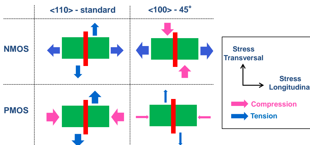
Figure 1-28 : Vue layout des différents types de stress à appliquer sur les deux orientations cristallines \langle 110 \rangle et \langle 100 \rangle afin d'augmenter la mobilité des transistors NMOS et PMOS
