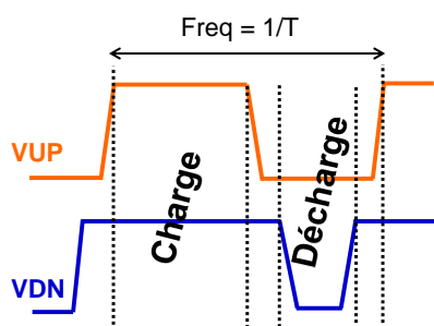
Figure 3-12 : Valeur des signaux permettant la charge ou la décharge de C_X dans la structure CBCM
