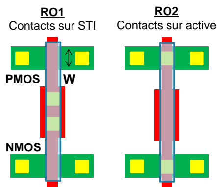
Figure 4-14 : Conception d'un inverseur CMOS avec les contacts de grille des transistors sur STI (RO1) ou sur active (RO2)
