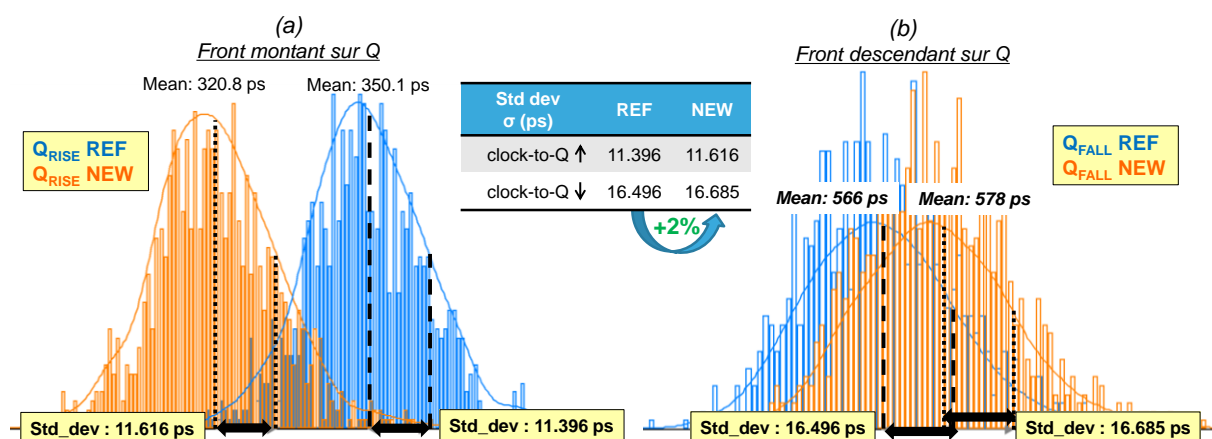
Figure 4-23 : Comparaison de la déviation standard du temps de propagation « clock-to-Q » entre les deux bascules SCAN lors d'un front montant (a) et lors d'un front descendant (b) sur la sortie Q connectée à une capacité C_{LOAD} égale à 11.625 pF
