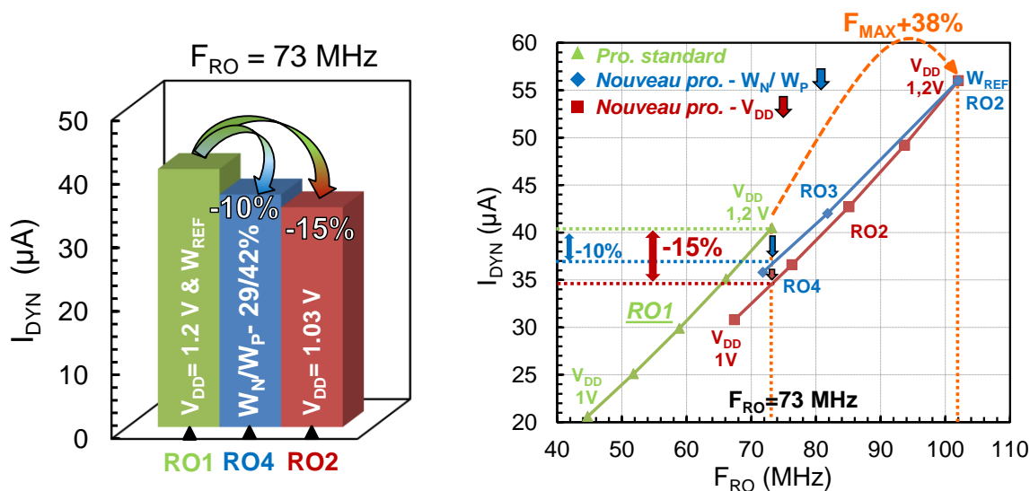
Figure 3-19 : Gains en courant dynamique obtenus entre le procédé de fabrication de référence et le nouveau procédé de fabrication pour une réduction des largeurs d'active W_N/W_P ou de l'alimentation V_{DD} lorsque C_L = C_{BE} + C_{IN}
