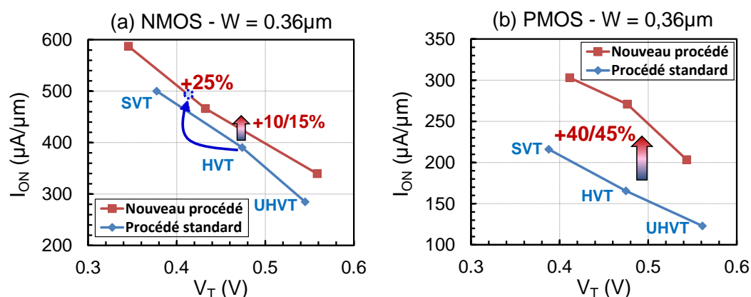
Figure 3-15 : Gain en I_{ON} obtenu avec le nouveau procédé de fabrication pour un transistor NMOS (a) et un transistor PMOS (b) GO1 utilisé dans les cellules standards
