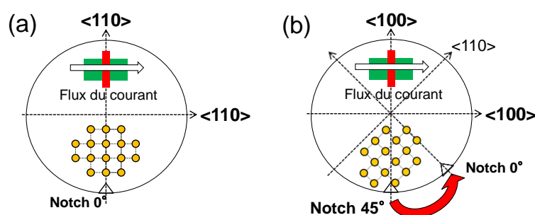
Figure 2-21 : Représentation schématique des deux types de substrats étudiés : l'orientation cristalline standard <110> (a) et l'orientation <100> tournée à 45° (b)
