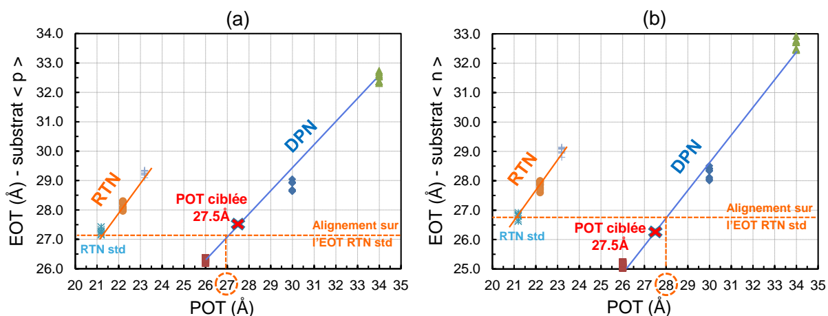
Figure 2-12 : Epaisseur électrique de l'oxyde (EOT) en fonction de l'épaisseur physique (POT) sur un substrat de type <p> (a) et sur un substrat de type <n> (b) entre le procédé de référence RTN et le procédé DPN
