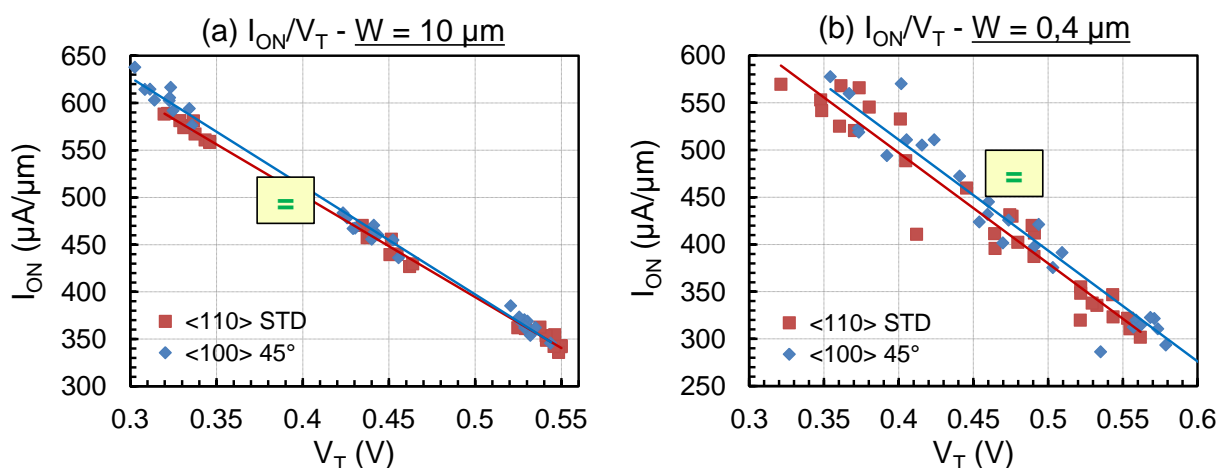
Figure 2-24 : Courbes de mérite I_{ON}/V_T d'un transistor NMOS GO1 de dimension W=10\mu\text{m} (a) et W=0,4\mu\text{m} (b) fabriqué avec une orientation cristalline standard \langle 110 \rangle et tournée à 45^\circ \langle 100 \rangle
