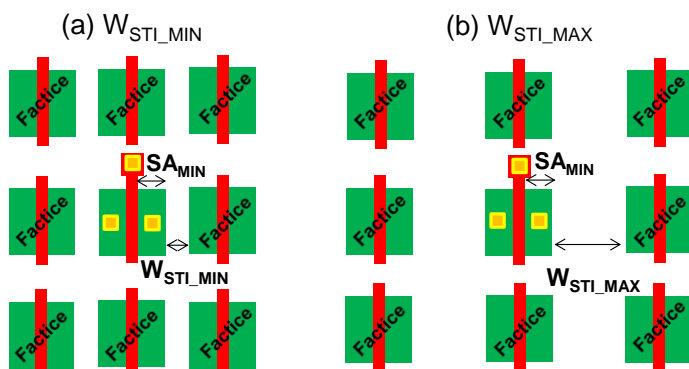
Figure 4-31 : Vue layout d'un transistor MOS dessiné dans un environnement composé de transistors factices séparés par une largeur W_{STI\_MIN} (a) et une largeur W_{STI\_MAX} (b)
