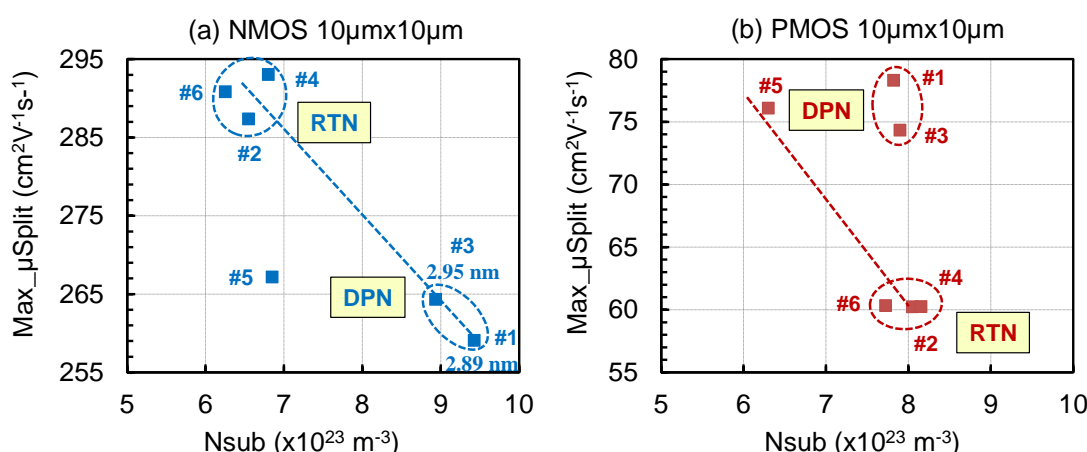
Figure 2-19 : Maximum de la mobilité en fonction du dopage du substrat d'un transistor NMOS (a) et d'un transistor PMOS (b) fabriqués avec le procédé RTN standard et le procédé DPN
