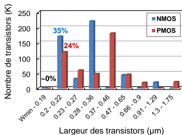
Figure 4-2 : Répartition du nombre de transistors NMOS et PMOS utilisés dans un circuit fabriqué en technologie e-NVM CMOS 80 nm en fonction de leur largeur
