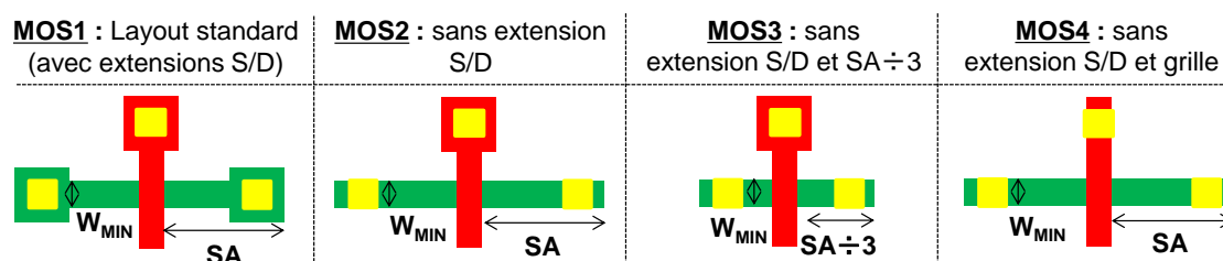
Figure 4-5 : Conception des différents MOS avec ou sans la tête de marteau en active et en poly-silicium
