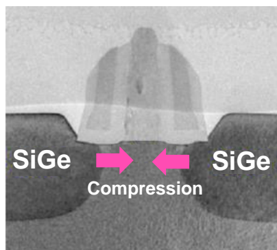
Figure 1-17 : Coupe TEM d'un transistor PMOS fabriqué avec l'intégration du SiGe dans les zones S/D pour augmenter la contrainte mécanique en compression dans le canal [Ghani'03], [Mistry'04]
