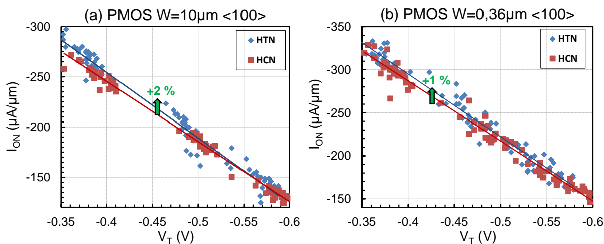
Figure 2-34 : Courbes de mérite I_{ON}/V_T d'un transistor PMOS de dimension W = 10 \mu\text{m} (a) et W = 0,36 \mu\text{m} (b) fabriqués avec un nitrure standard HCN et un nitrure fortement contraint en tension HTN dans l'orientation cristalline \langle 100 \rangle
