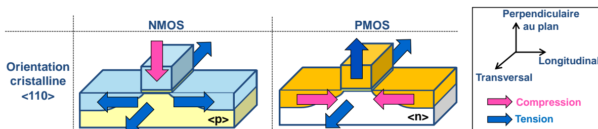
Figure 4-7 : Vue layout des différents types de stress à appliquer afin d'augmenter la mobilité des transistors NMOS et PMOS fabriqués avec une orientation cristalline standard <110>
