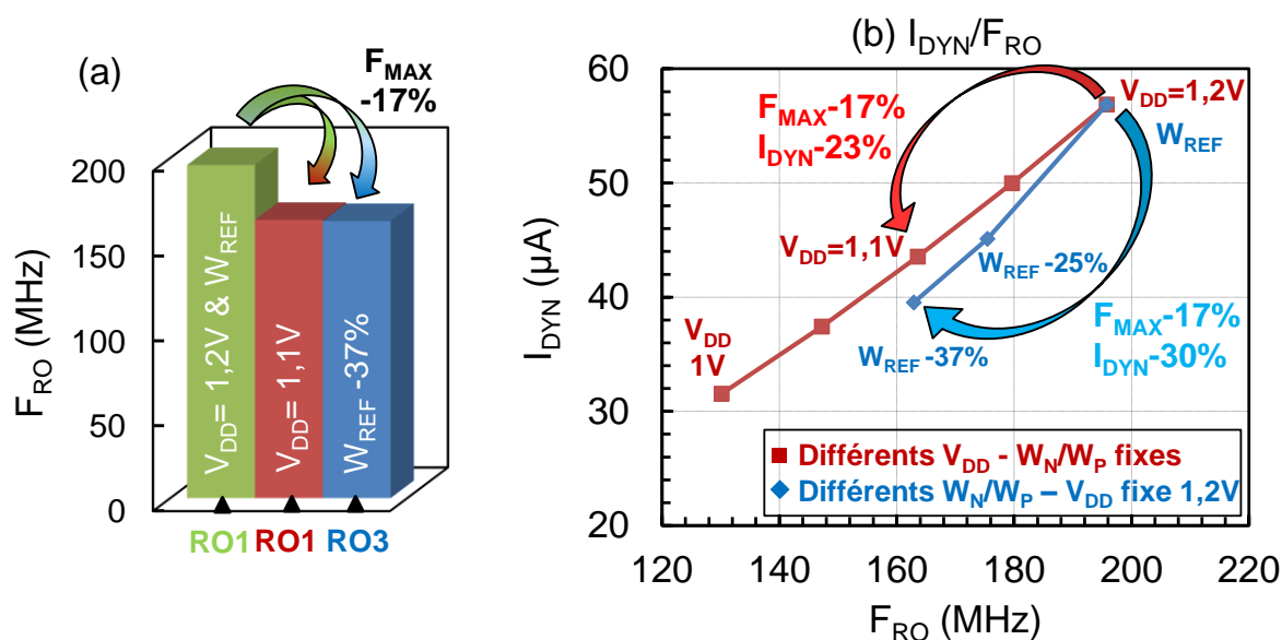
Figure 3-13 : Réduction de la fréquence d'un oscillateur en anneau (a) et du courant dynamique consommé (b) dans le cas d'une réduction de la tension d'alimentation V_{DD} ou d'une réduction de la taille des transistors W_N/W_P
