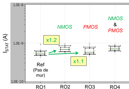
Figure 4-42 : Comparaison du courant statique des oscillateurs en anneau conçus avec ou sans le mur en poly-silicium
