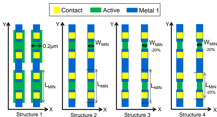
Figure 4-3 : Vue layout des quatre structures permettant de mesurer la résistance des contacts placés sur des barreaux d’actives de différentes largeurs
