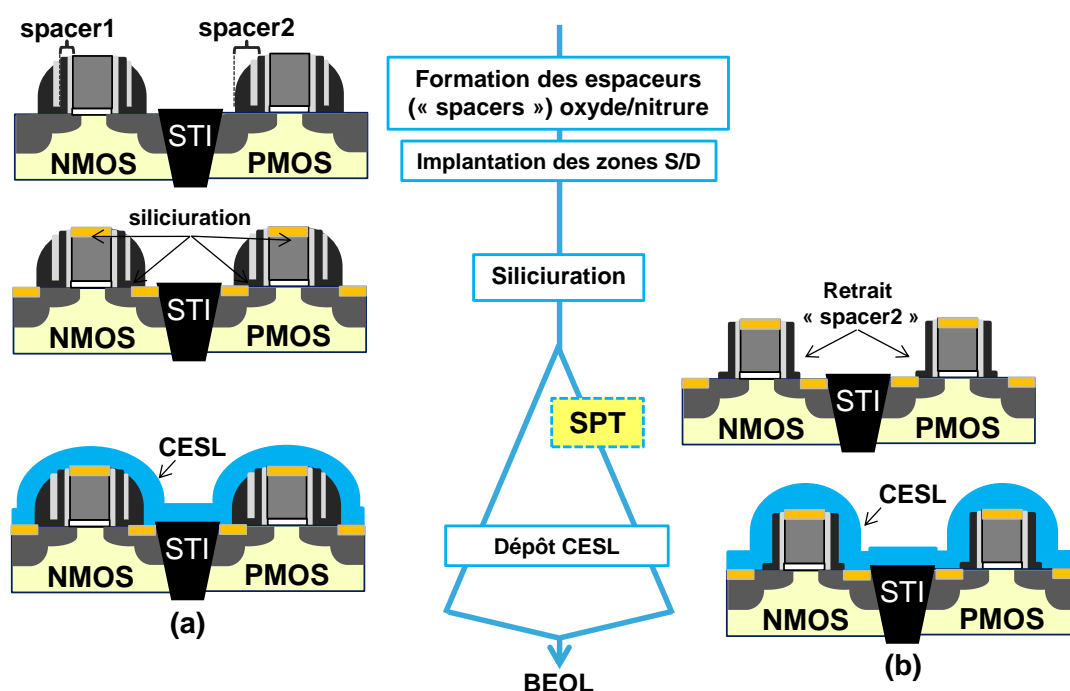
Figure 1-24 : Étapes de fabrication d'un procédé standard à partir de la formation des espaceurs jusqu'au dépôt de la couche de CESL sans (a) et avec l'intégration du procédé SPT (b)
