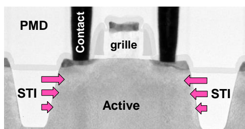
Figure 4-24 : Coupe TEM d'un transistor MOS montrant les tranchées d'isolation STI et la contrainte exercée par l'oxyde STI
