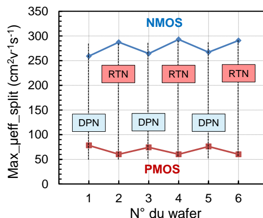
Figure 2-17 : Mobilité des trous et des électrons pour les deux différents procédés RTN et DPN
