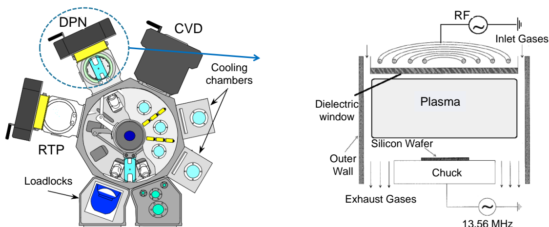
Figure 2-6 : Schéma de la chambre et des conditions utilisées lors de la nitruration par plasma DPN
