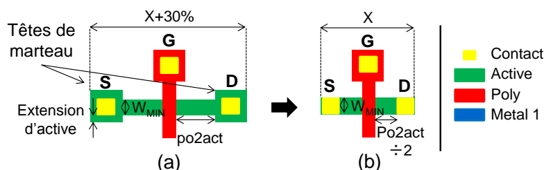
Figure 4-1 : Vue layout d'un transistor MOS dessiné avec (a) ou sans (b) l'extension S/D
