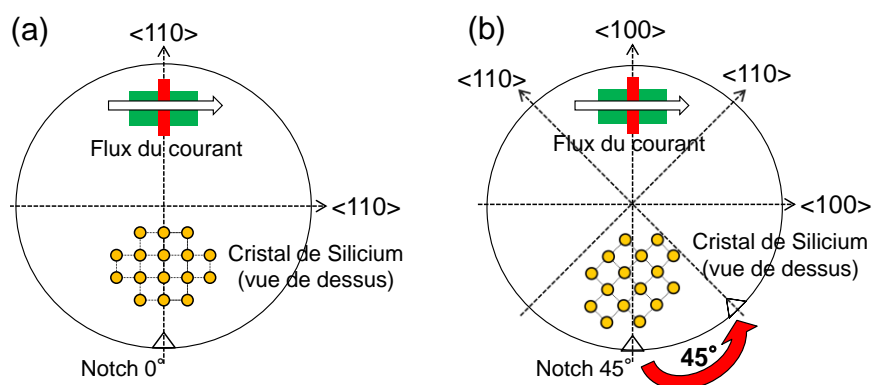
Figure 1-14 : Représentation schématique des deux types de substrat \langle 100 \rangle utilisés dans les circuits CMOS : l'orientation cristalline standard \langle 110 \rangle (a) et l'orientation cristalline tournée à 45^\circ \langle 100 \rangle (b)
