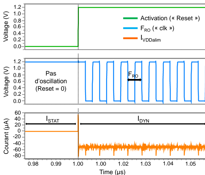
Figure 3-2 : Les différents signaux de l'oscillateur en anneau
