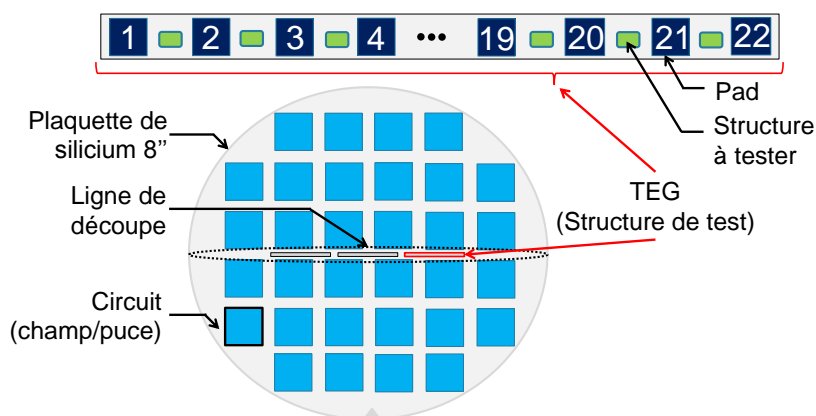
Figure 3-3 : Représentation graphique d'une plaquette de silicium et de l'intégration d'une structure de test (TEG) conçue avec 22 pads
