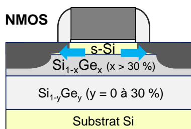
Figure 1-10 : Fabrication d'un substrat s-Si contraint en tension pour augmenter les performances des transistors NMOS
