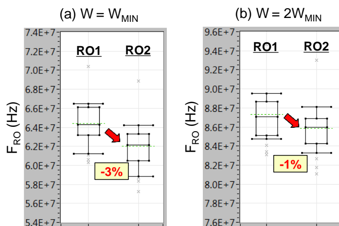
Figure 4-15 : Fréquence d'oscillation des oscillateurs en anneau fabriqués avec des transistors MOS possédant les contacts de grille sur STI (RO1) ou sur active (RO2) de dimension W = W_{MIN} (a) et W = 2W_{MIN} (b)
