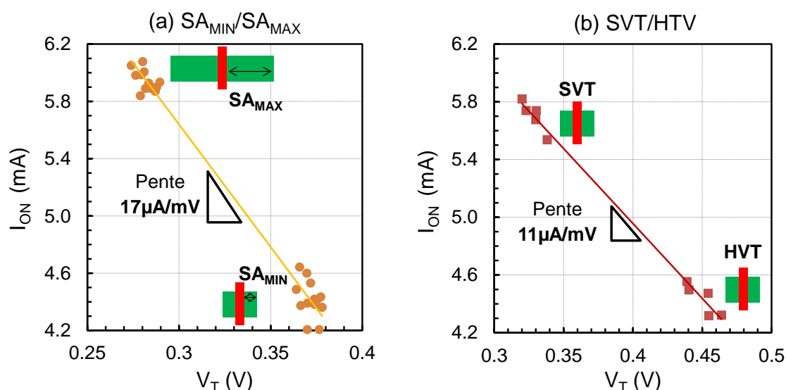
Figure 4-29 : Courbe de mérite I_{ON}/V_T d'un transistor NMOS dessiné avec deux différentes distances grille/STI (a) et d'un transistor NMOS ayant deux différentes tensions de seuil (b)
