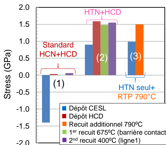
Figure 2-30 : Niveau de stress des 3 procédés de nitruration comparés dans cette étude
