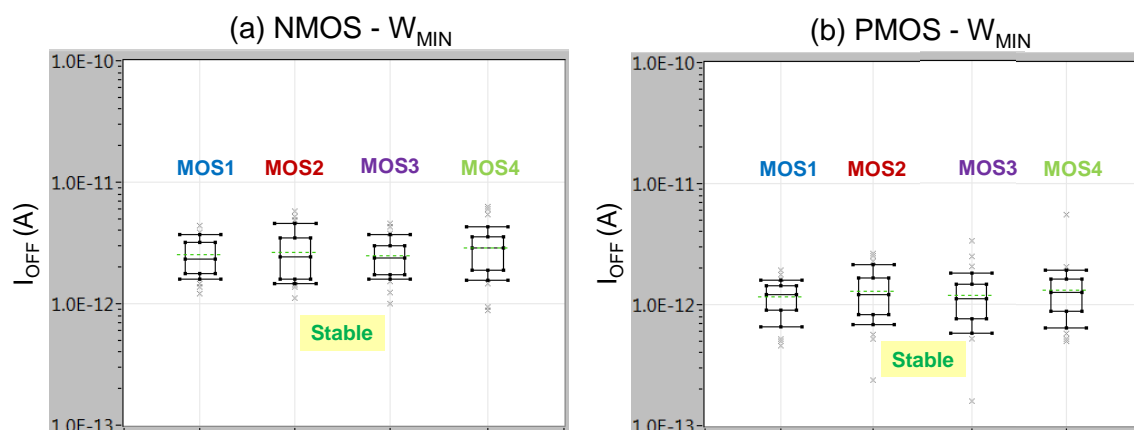
Figure 4-8 : Courant de fuite de drain ( I_{OFF} ) d'un transistor NMOS (a) et d'un transistor PMOS (b) de dimension W_{MIN} dessiné avec ou sans l'extension S/D en active et en poly-silicium
