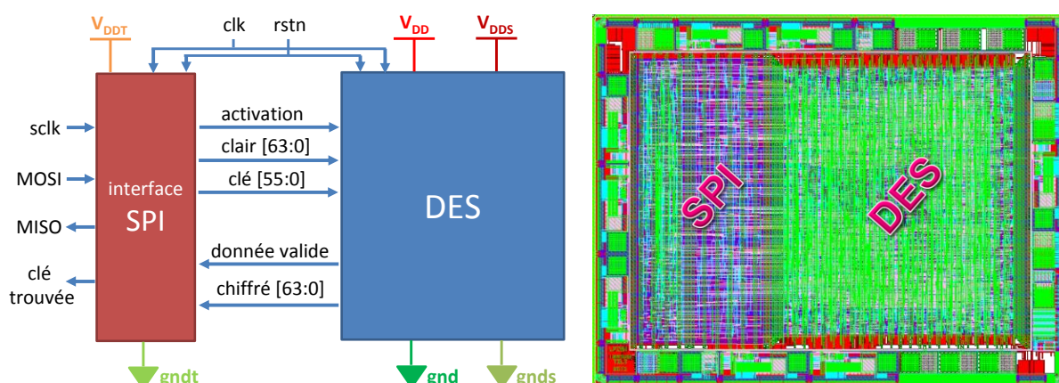
Figure 3-21 : Architecture (a) et vue layout (b) du circuit DES
