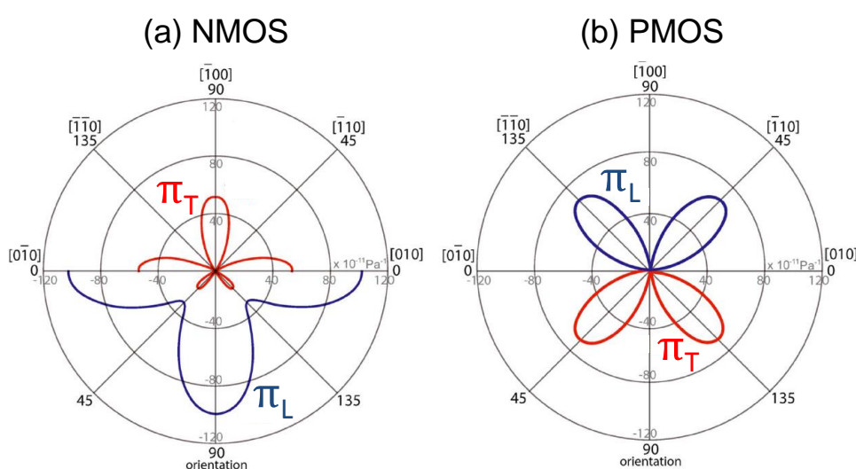
Figure 1-27 : Représentation graphique des coefficients piezorésistifs du transistor NMOS (a) et du transistor PMOS (b) dans le plan cristallin (100) [Kanda'82]
