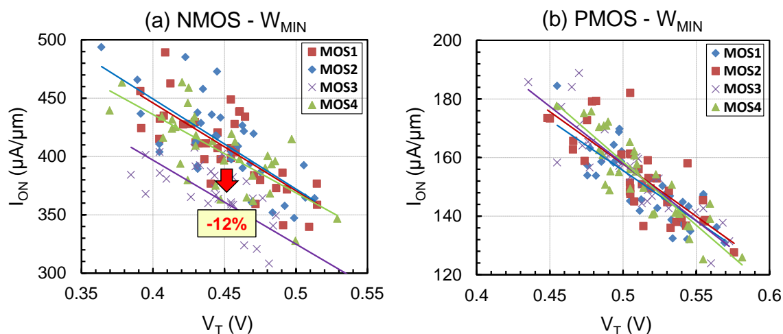
Figure 4-6 : Courbes de mérite I_{ON}/V_T d'un transistor NMOS (a) et d'un transistor PMOS (b) de dimension W_{MIN} dessiné avec ou sans l'extension en active et en poly-silicium
