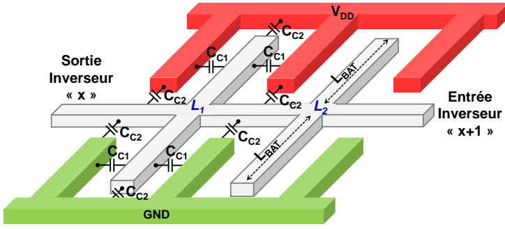
Figure 3-9 : Représentation graphique d'une structure en peigne utilisée pour réaliser la capacité de routage C_{BE}
