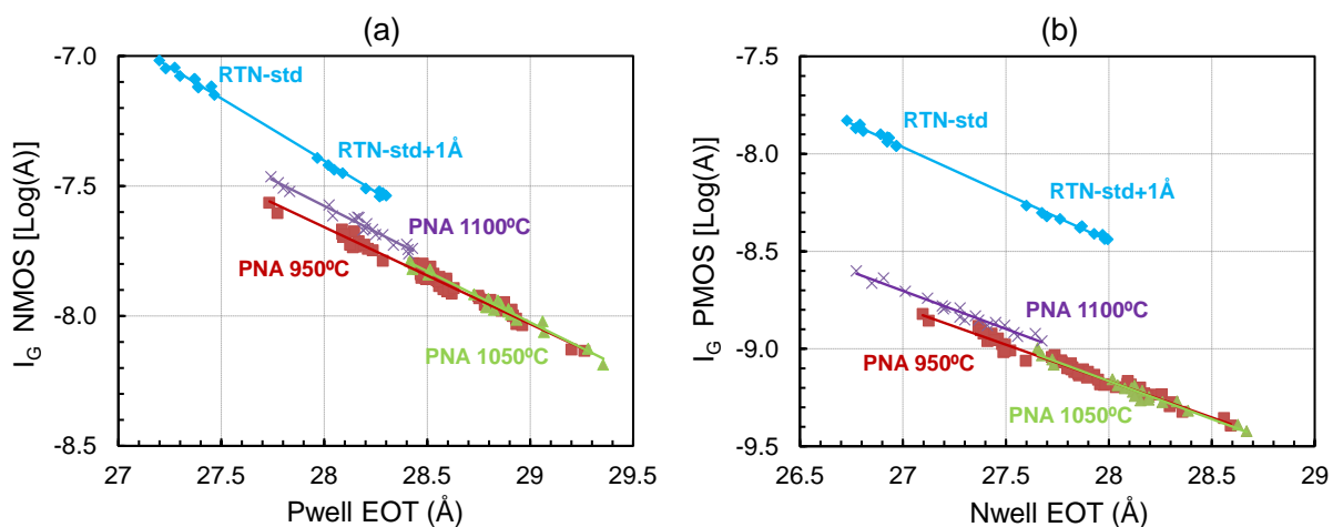
Figure 2-8 : Courant de grille d'un transistor NMOS (a) et d'un transistor PMOS (b) de dimension W=10\mu\text{m} et L=10\mu\text{m} en fonction de l'EOT pour différentes températures du recuit PNA
