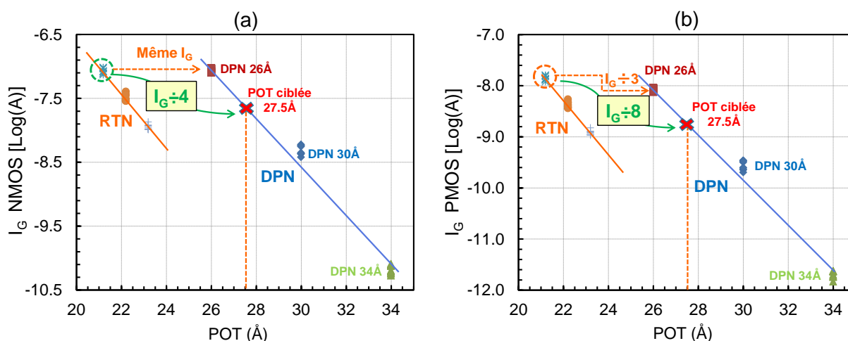
Figure 2-13 : Courant de grille d'un transistor NMOS (a) et d'un transistor PMOS (b) fabriqué avec la nitruration RTN ou DPN en fonction de l'épaisseur physique de l'oxyde
