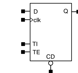
Figure 4-17 : Symbole logique de la bascule D choisie dans cette étude
