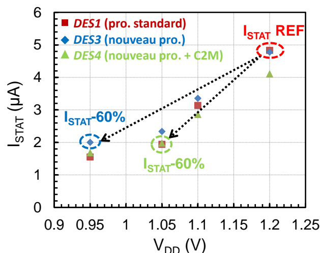
Figure 3-30 : Réduction du courant statique consommé par le DES avec l'utilisation du nouveau procédé de fabrication et lors d'une diminution de la tension d'alimentation V_{DD} et de la taille des transistors W_N/W_P
