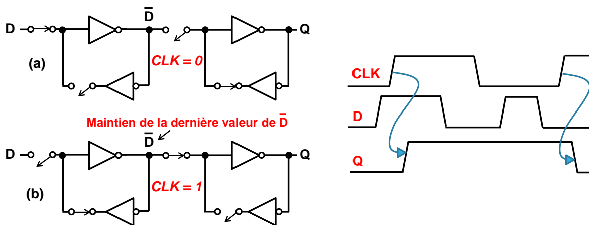
Figure 4-18 : Principe de fonctionnement d'une bascule D lorsque le signal clk est à l'état « 0 » (a) ou à l'état « 1 » (b)
