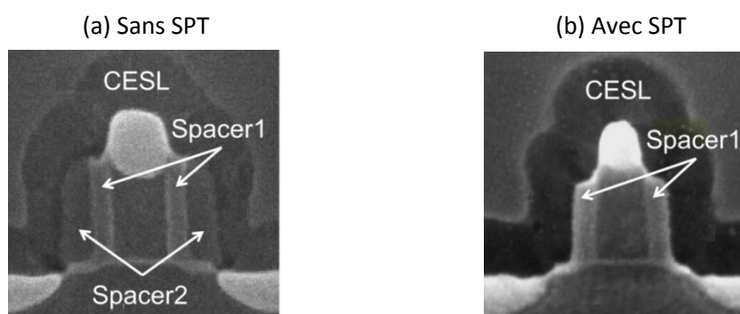
Figure 1-25 : Coupe TEM d'un transistor MOS fabriqué sans (a) ou avec le procédé SPT utilisé pour le retrait du spacer2 (b) [Chen'06], [Fang'06]
