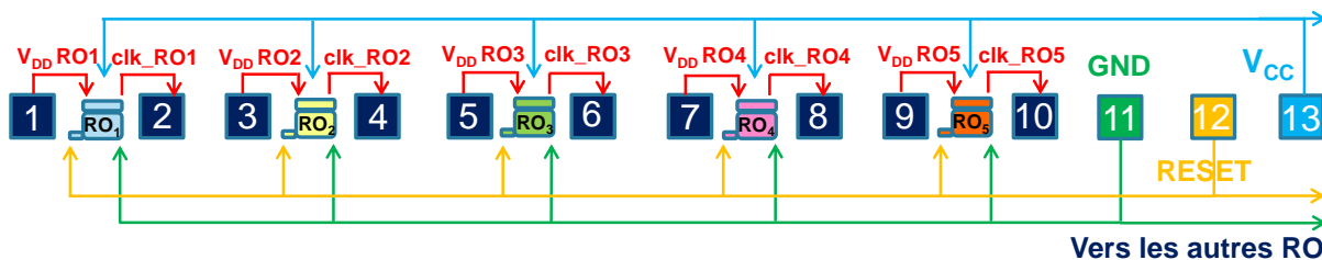
Figure 3-4 : Une partie de la structure de test contenant 9 oscillateurs en anneau
