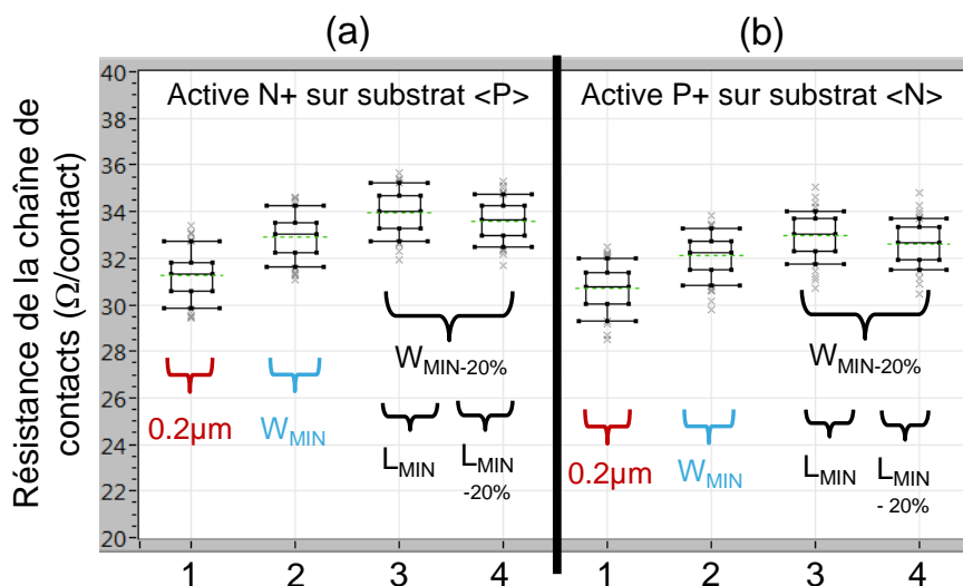
Figure 4-4 : Résistance des chaînes de contacts dessinées avec différentes largeurs d’actives dopées N+ (a), et P+ (b)
