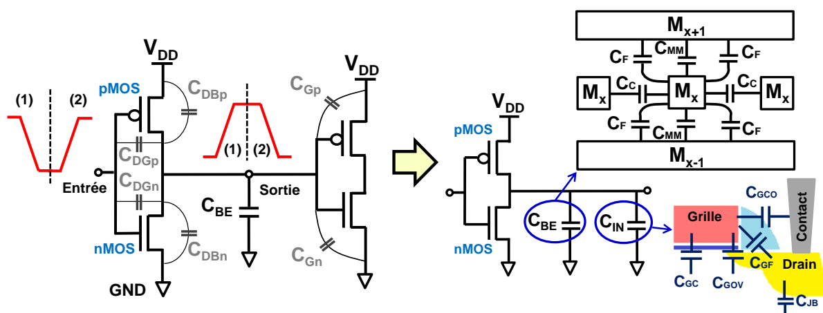
Figure 1-30 : Représentation graphique des capacités parasites C_{BE} et C_{IN} intervenant dans la capacité de charge C_L d'un inverseur CMOS connecté à un autre inverseur
