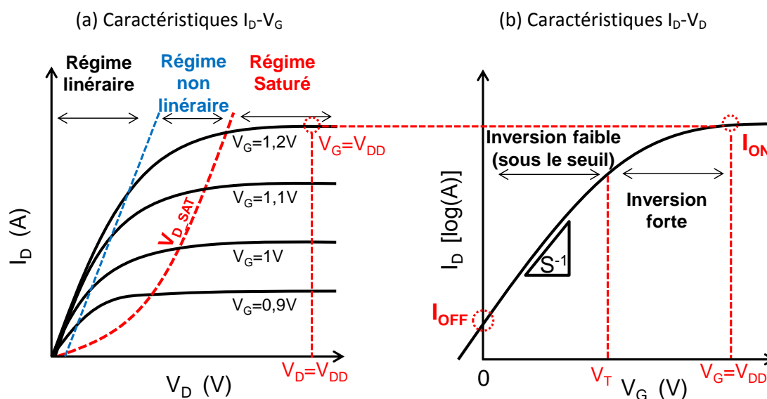
Figure 1-4 : Caractéristiques I_D - V_D (a) et I_D - V_G (b) d'un transistor MOS basse tension fabriqué en technologie e-NVM CMOS 80 nm
