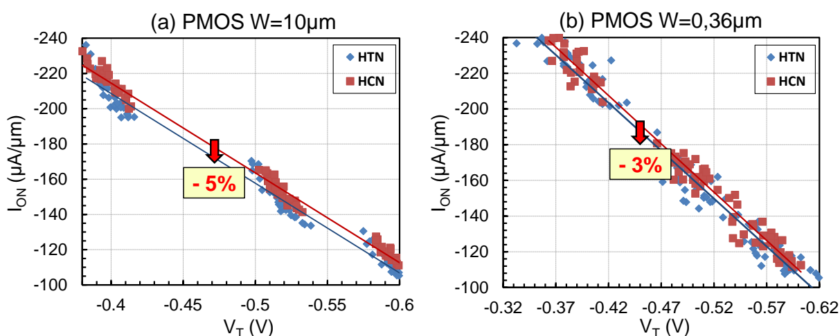
Figure 2-33 : Courbes de mérite I_{ON}/V_T d'un transistor PMOS de dimension W = 10 \mu\text{m} (a) et W = 0,36 \mu\text{m} (b) fabriqués avec un nitrure standard HCN et un nitrure fortement contraint en tension HTN
