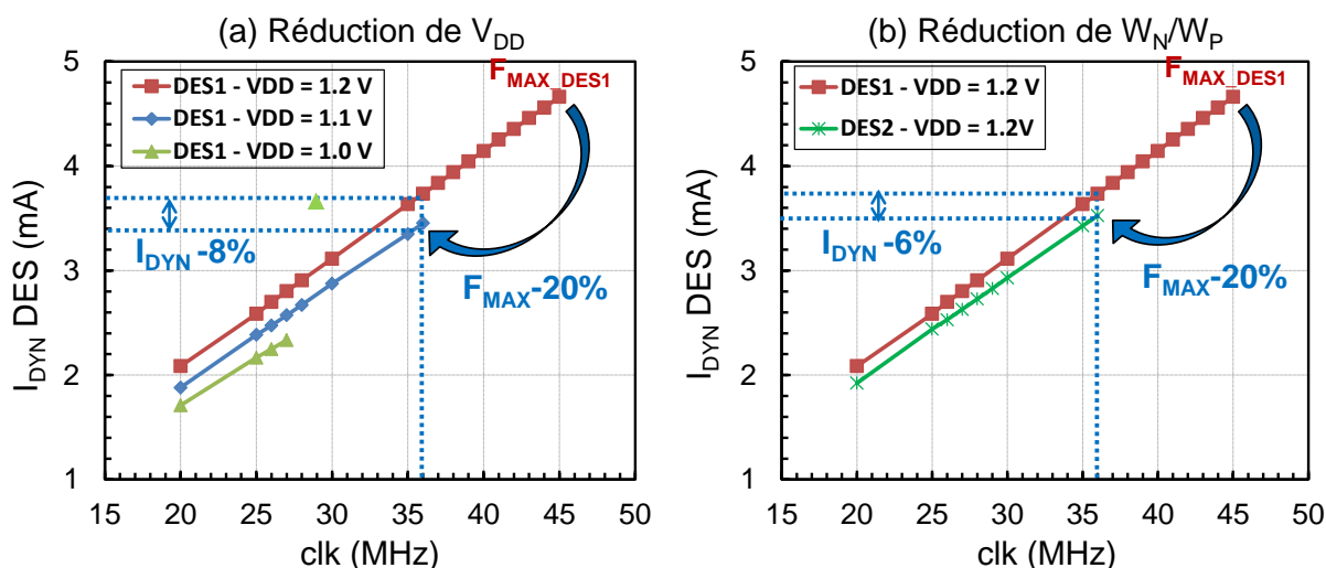
Figure 3-26 : Courant dynamique en fonction de la fréquence de fonctionnement des circuits DES1 et DES2 fabriqués sur le procédé standard lors d'une diminution de la tension d'alimentation V_{DD} (a) ou de la largeur des transistors (b)
