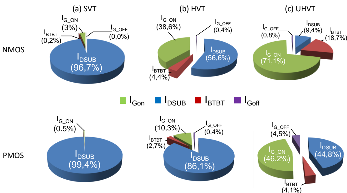
Figure 1-34 : Répartition des différents courants de fuite dans un transistor NMOS et dans un transistor PMOS de type SVT (a) HVT (b) et UHVT (c) de longueur L = 90 \text{ nm} et de largeur W = 1\mu\text{m}
