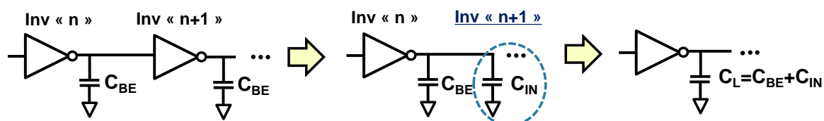
Figure 3-7 : Représentation graphique de la capacité de charge ( C_L ) comme étant la somme de la capacité liée au routage entre les portes ( C_{BE} ) et de la capacité équivalente de la porte attaquée ( C_{IN} )
