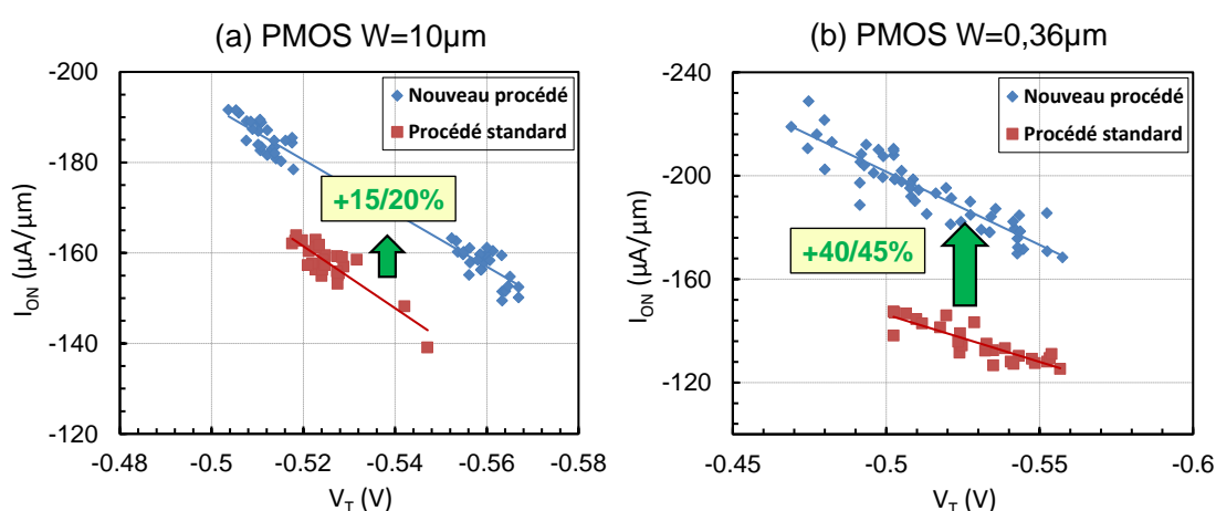
Figure 2-36 : Courbes de mérite I_{ON}/V_T d'un transistor PMOS de dimension W = 10 \mu\text{m} (a) et W = 0,36 \mu\text{m} (b) fabriqués avec le procédé de fabrication standard et le nouveau procédé de fabrication
