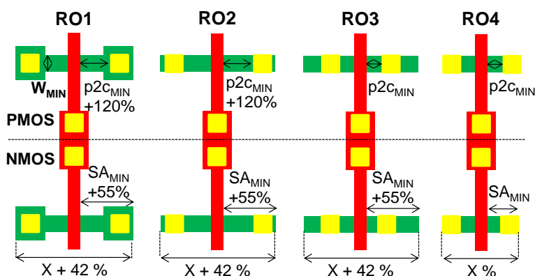
Figure 4-9 : Conception des différents inverseurs utilisés dans les oscillateurs en anneau avec ou sans l’extension S/D
