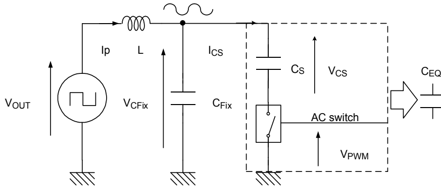
Fig.4 Schéma de principe de systèmes d'accord automatique, qui est basé sur le capacité commutée synchrone.
