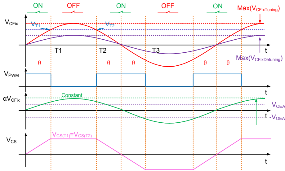
Fig.5 Formes d'ondes théoriques du systèmes d'accord automatique basé sur le capacité commute synchrone
