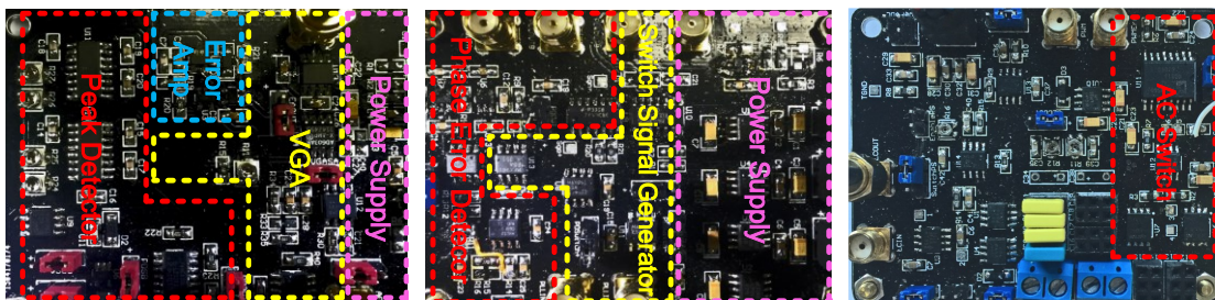
Fig.7 Prototype de l'auto-régulation système en circuit électrique imprimé.
