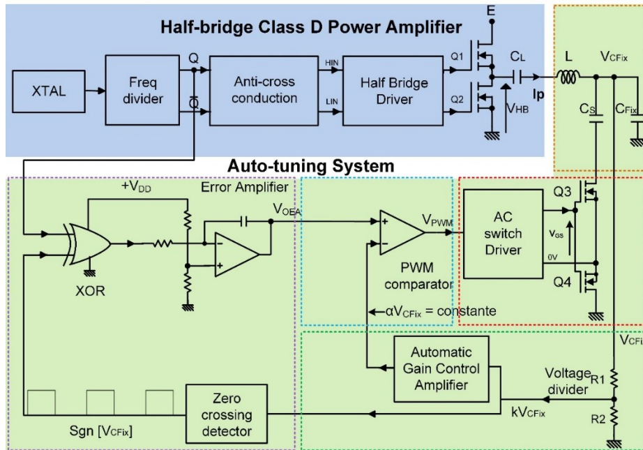
Fig.6 Diagramme de la réalisation d'auto-régulation système basé sur condensateur commuté synchrone.
