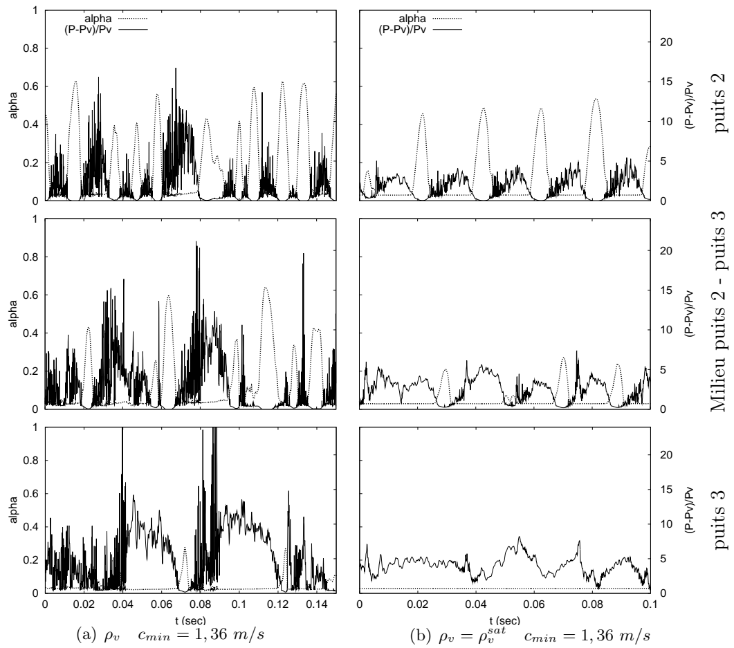
FIGURE 9.26 – Evolutions temporelles de la pression : étude de l'influence de la relaxation thermodynamique en modèle sinusoïdal c_{min} = 1,36 \text{ m/s}
