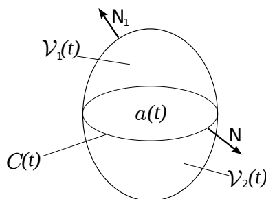
FIGURE 2.1 – Volume de contrôle matériel \mathcal{V}
