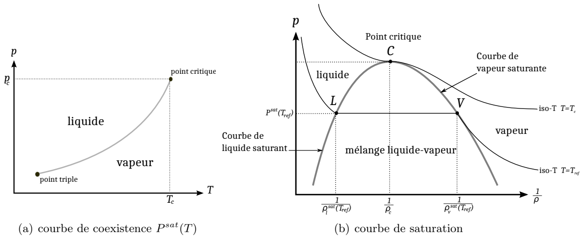
FIGURE 4.1 – Courbes de coexistence et de saturation
