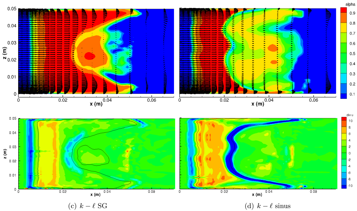
FIGURE 9.40 – Visualisation instantanée des poches de cavitation et de la divergence de la vitesse (avec isocontour de \alpha > 0,85 ) dans le plan horizontal ( y = 6 \text{ mm} ) : comparaison des lois d'état
