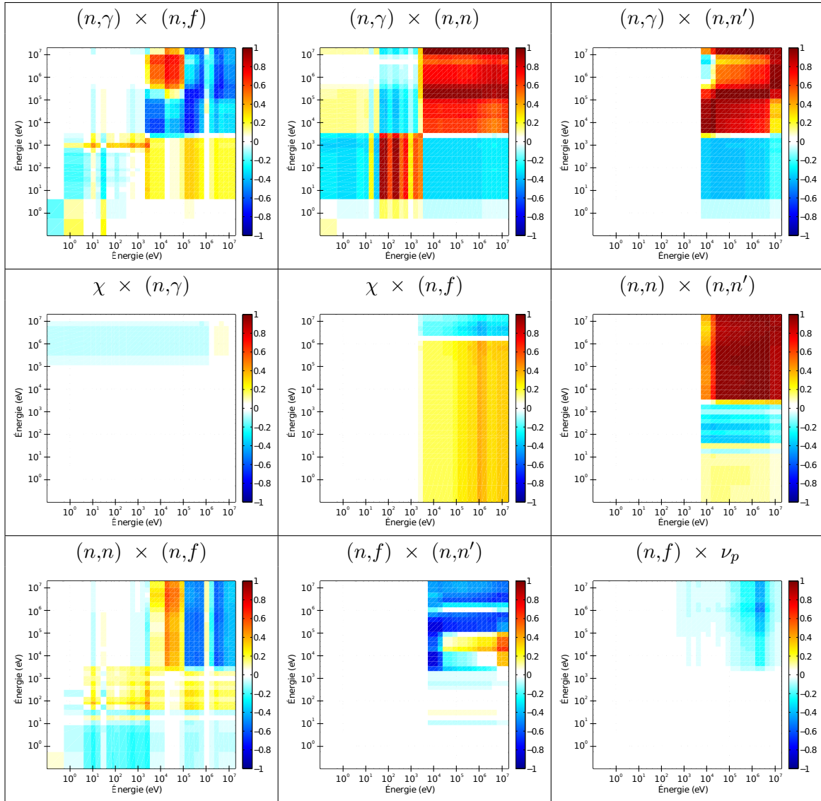
FIGURE 5.17. Matrices des corrélations croisées multigroupes (à 33 groupes en énergie), obtenues à partir de l'assimilation des expériences PROFIL et Jezebel, entre les principales sections efficaces du ^{239}\text{Pu}
