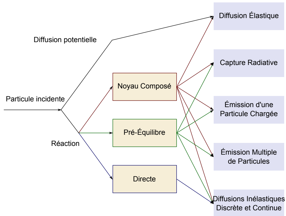
FIGURE 1.5. Schéma décrivant les différents mécanismes de réactions nucléaires à haute énergie
