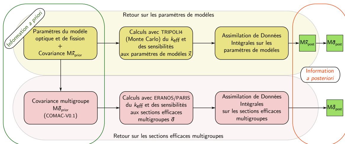
FIGURE 4.7. Schémas utilisés pour comparer les deux méthodes d'assimilation de données intégrales (sur les paramètres et sur les sections multigroupes) pour le ^{239}\text{Pu} en utilisant Jezebel
