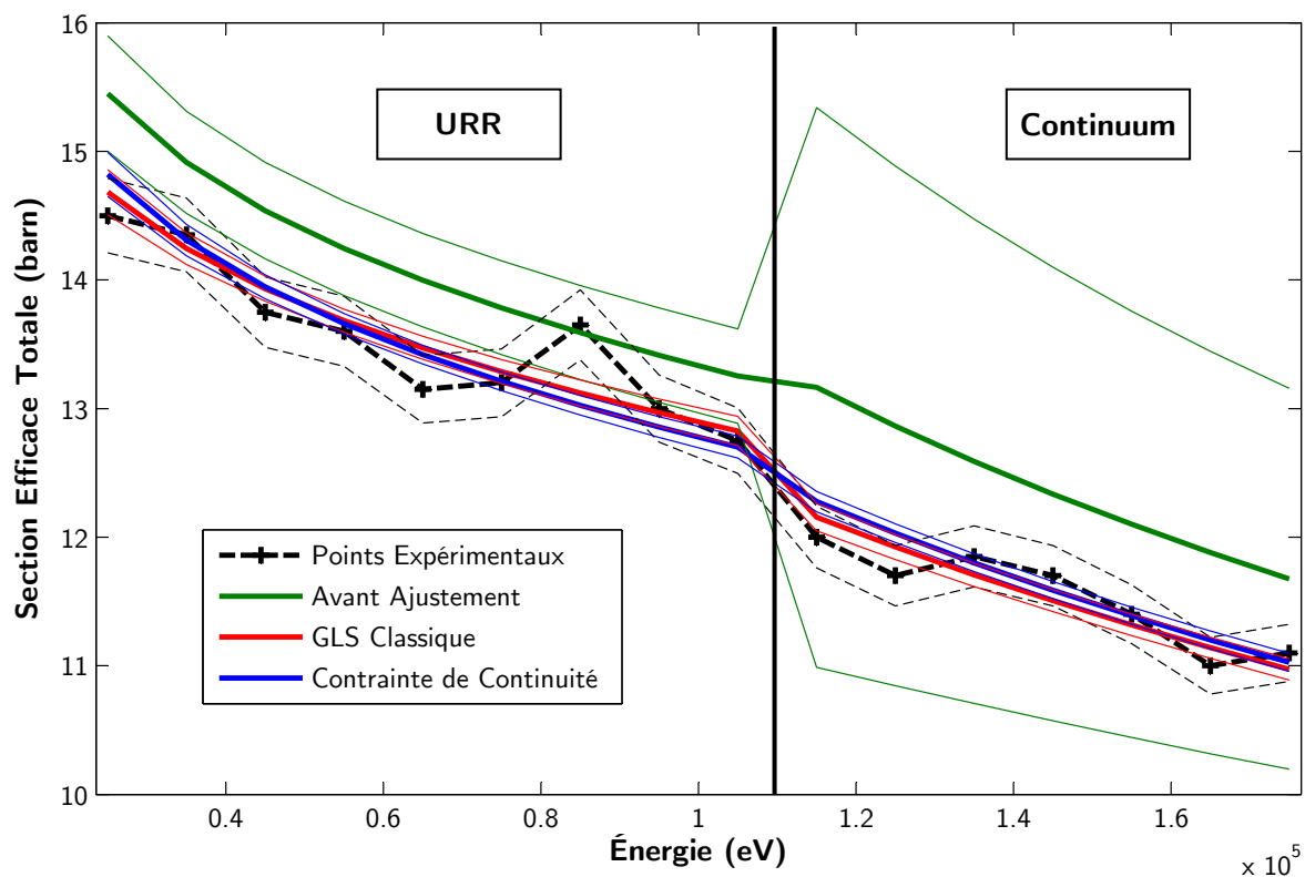
FIGURE 3.14. Résultats obtenus avec/sans prise en compte de la contrainte de continuité sur la section efficace totale de l'^{238}\text{U} (URR pour les énergies inférieures à 105\text{ keV} et modèle optique pour les énergies supérieures)
