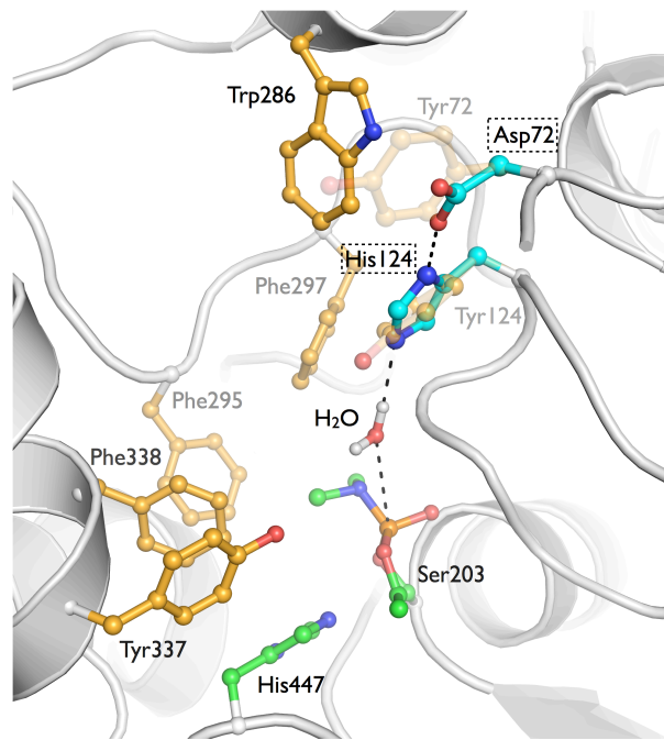
Figure 45. Modèle du mutant Y72D/Y124H phosphorylé par le tabun. Les résidus mutés (cyan) permettraient de stabiliser une molécule d'eau dans une position propice à la déphosphoramidation de la sérine par un mécanisme en ligne.
