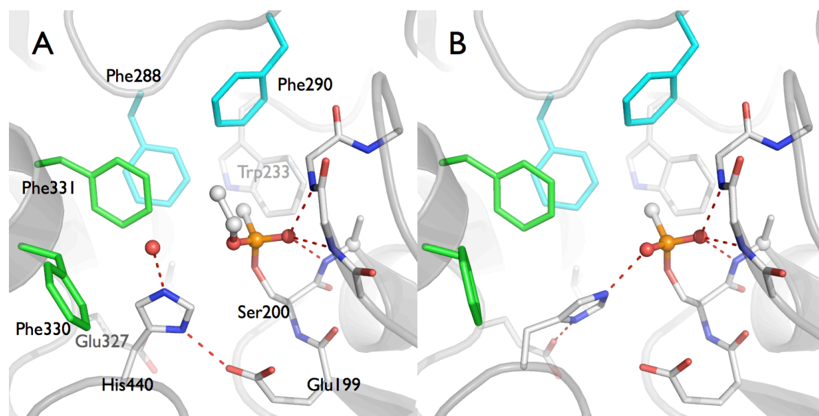
Figure 28. Sites actifs de la TcAChE inhibée par le VX, avant (A ; 1vxr ; 2.2 Å) et après vieillissement (B ; 1vxo ; 2.4 Å). Les résidus de la poche acyle sont en cyan. Avant vieillissement, His440 forme des liaisons H avec une molécule d'eau et Glu199. Elle forme une liaison H avec Glu327 et un pont salin avec l'oxyanion du phosphonate après vieillissement.
