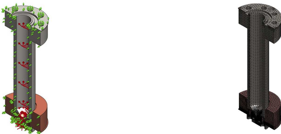
FIGURE B.1 – A gauche : Conditions limites imposées à la cellule pour le calcul par éléments finis. A droite : Maillage utilisé lors des calculs par éléments finis
