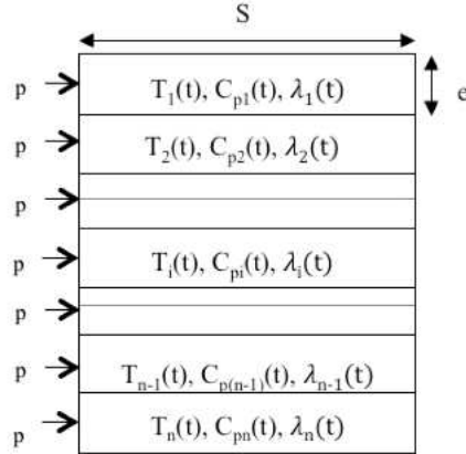
FIGURE 2.22 – Représentation d'une pièce pour un système de régulation
