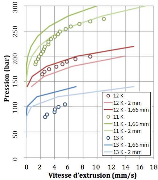
FIGURE 4.9 – Résultats obtenus avec le modèle dédié pour une buse d'une section équivalente à 1 \times 10^{-6} \text{ m}^2 .
