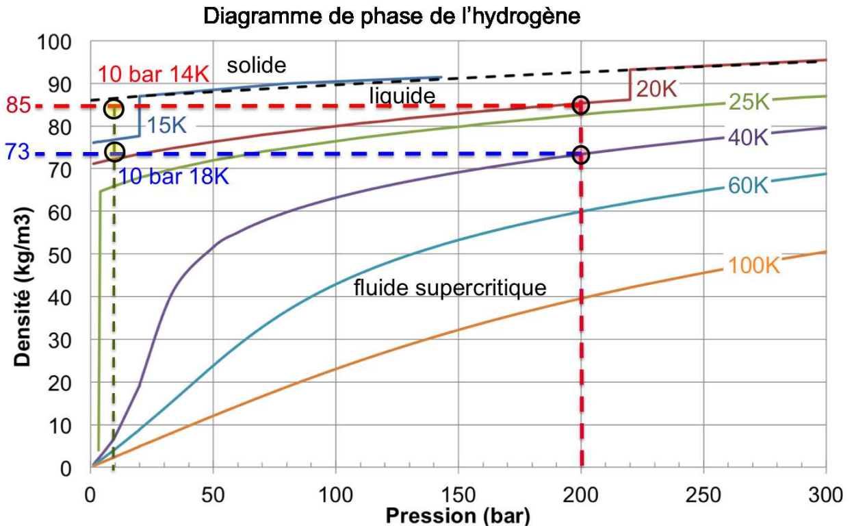
FIGURE 2.4 – Diagramme de phase de l'hydrogène. En pointillés rouges et trait plein noir : ligne d'iso-densité à 87 g/l et 76 g/l, pour des conditions de remplissage initiales représentés respectivement par les points verts. Points rouges : points d'un fonctionnement à 200 bar
