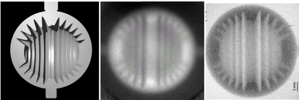
FIGURE 1.4 – Radiographie gamma. De gauche à droite : CAO de la pièce de référence, radiographie réalisée par une source de 400 \mu\text{m} , radiographie obtenue avec une source de 50 \mu\text{m} . Source : [18]
