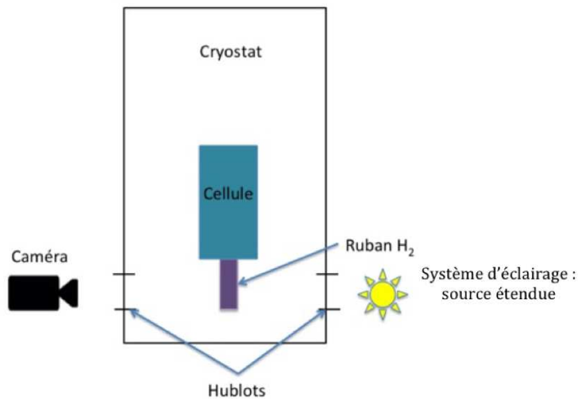
FIGURE 3.1 – Schéma du système de visualisation des rubans d'hydrogène solide en configuration ELISE
