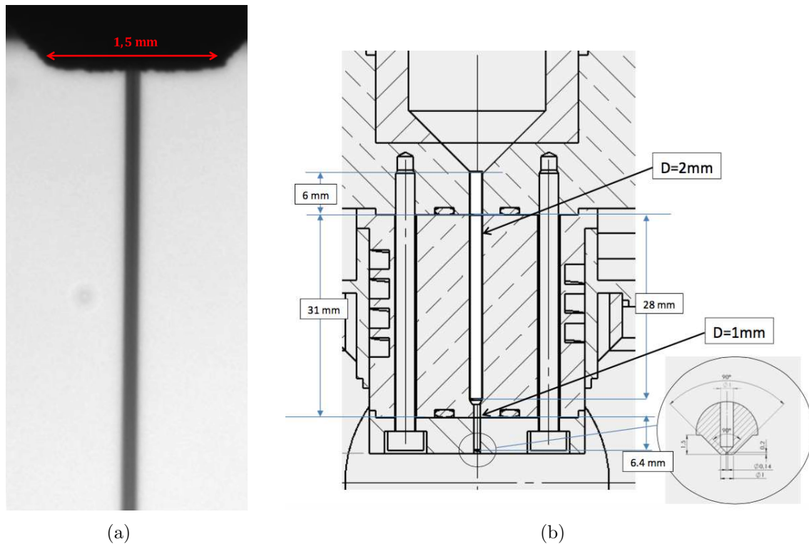
FIGURE 3.18 – (a) cylindre d’hydrogène de 90 \mu\text{m} de diamètre (mesure) obtenu par extrusion (b) géométrie du canal d’extrusion. La buse est en laiton et mesure 140 \mu\text{m} de diamètre uniquement sur une hauteur de 200 \mu\text{m} . Vidéo réalisée avec la caméra PIKE et l’objectif sigma f8 mirror à une distance de travail de 1,5 m et une résolution de 22 \mu\text{m} .
