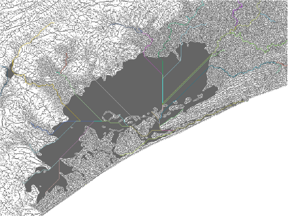
Slope Lenght
