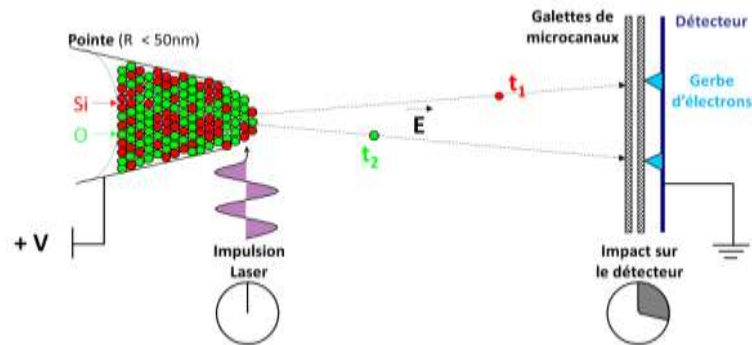
Figure II.4 Principe de fonctionnement d'une sonde atomique Laser. Les atomes de l'échantillon sont ionisés à l'aide d'un potentiel positif et d'impulsions laser et accélérés vers un détecteur aDLD sensible en position. Le temps de vol d'un ion est mesuré entre l'impulsion laser et l'impact sur le détecteur [3].
