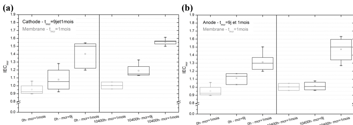
Figure 22. Comparaison des valeurs d'IEC membrane après 1 mois de macération à celles de la (a) GDCathode et (b) GDAnode après 9 j et 1 mois de macération pour les AME neufs et vieillis.
