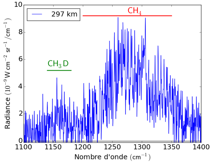
FIGURE 2.7 – Exemple de spectres CIRS obtenus après co-addition mesurés à 35^{\circ}\text{S} ( L_S = 29^{\circ} ) par FP4, acquis à 297 km d'altitude (1.3 hPa). Ce spectre a une résolution spectrale de 0.25\text{ cm}^{-1} .
