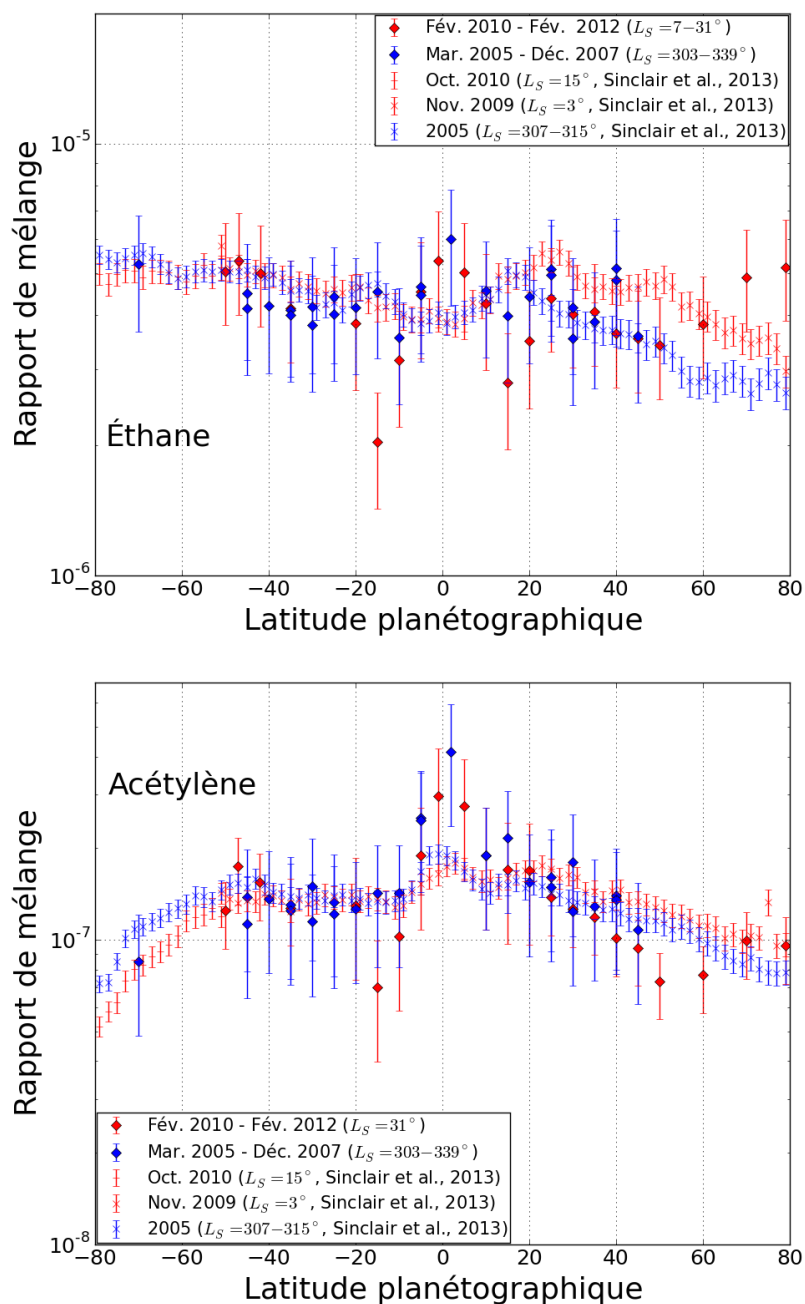
FIGURE 4.10 – Comparaison des mesures CIRS au limbe (losanges) des abondances de C 2 H 6 et de C 2 H 2 avec celles au nadir (croix et tirets) de Sinclair et al. (2013). Les points rouges représentent les mesures effectuées au printemps de l'hémisphère nord. Celles effectuées en hiver sont représentées en bleu.
