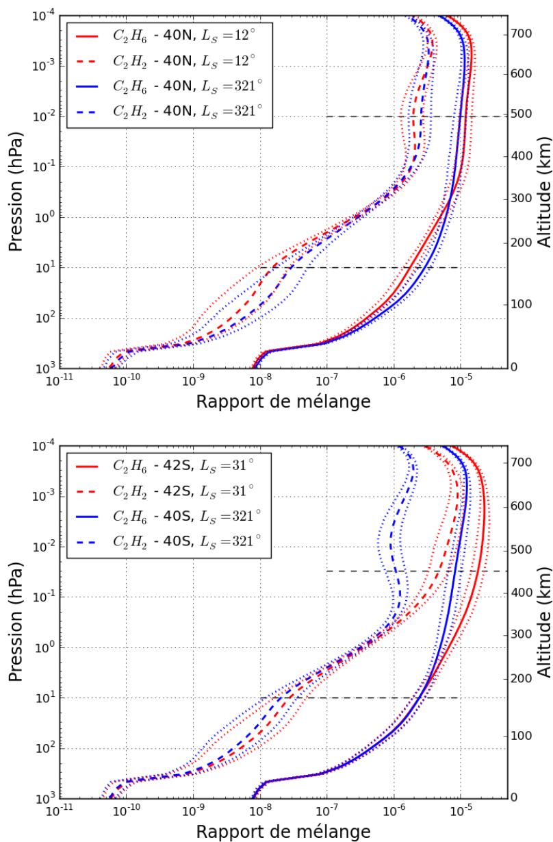
FIGURE 4.5 – Profils d’abondance d’éthane (trait plein) et d’acétylène (tirets), mesurés à 40^{\circ}N (en haut) et 42^{\circ}S (en bas). Le rouge correspond aux données acquises au printemps boréal et le bleu à celles de l’hiver boréal (Guerlet et al. 2009). Les pointillés représentent l’enveloppe d’erreur des profils. Les tirets noirs représentent les limites de sensibilité des données.
