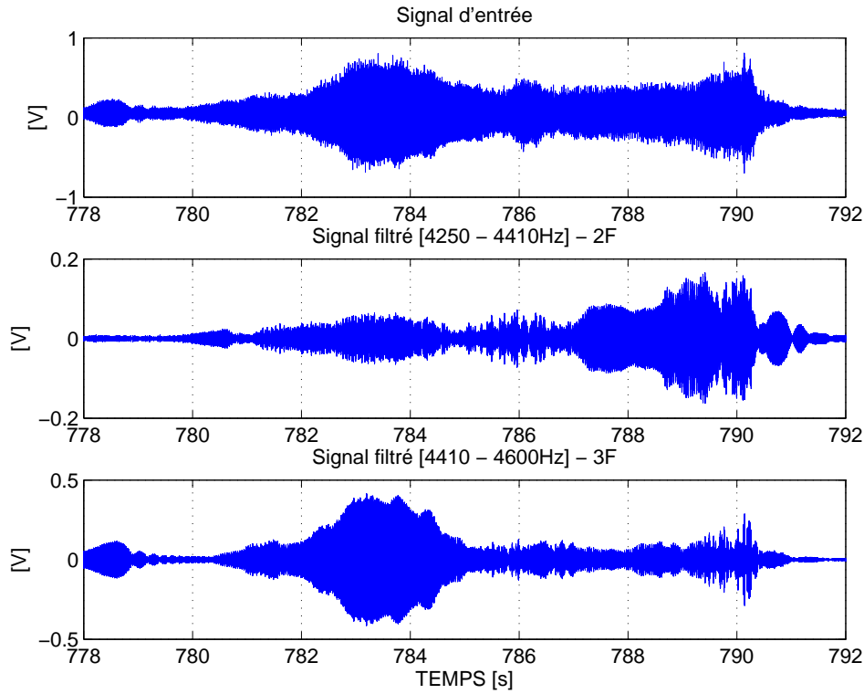
FIGURE 4.34 – Contributions modales lors de la septième bouffée
