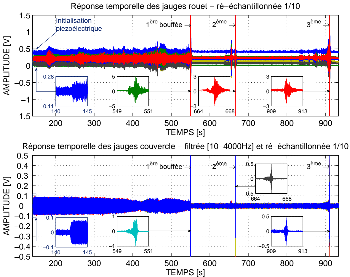
FIGURE 4.3 – Réponse dynamique du rouet et du couvercle lors des essais de la configuration 1
