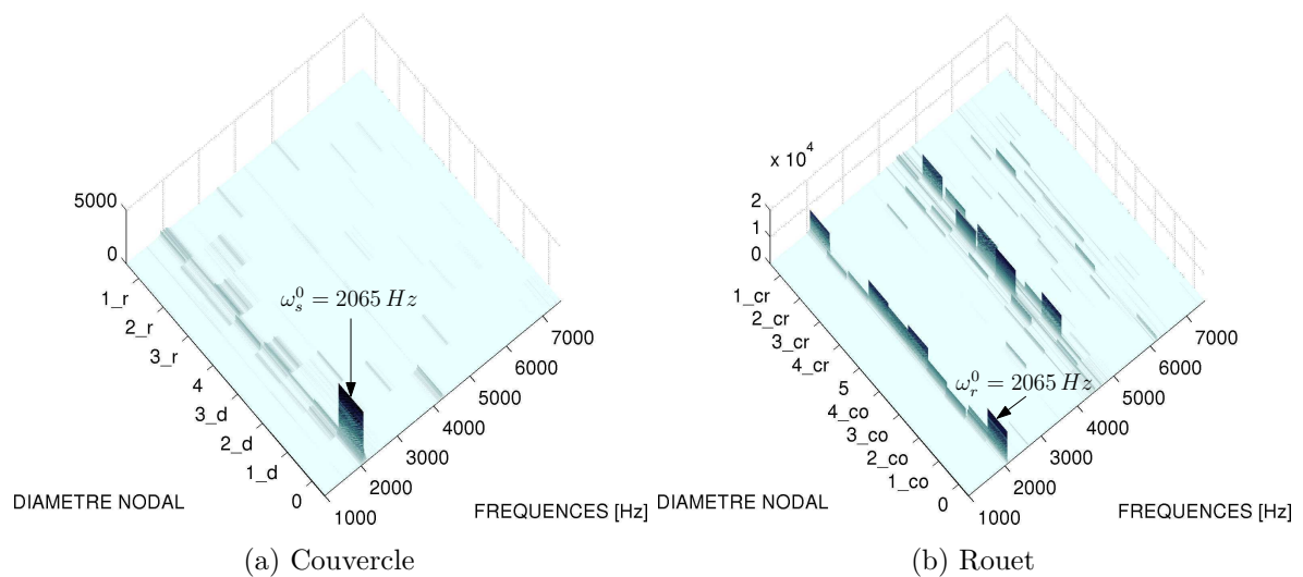
FIGURE 4.30 – Diagramme fréquences - diamètres nodaux : quatrième bouffée
