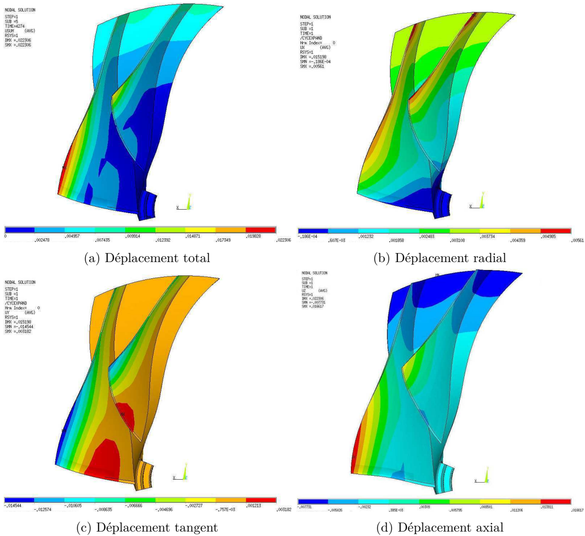
FIGURE 2.6 – Champs de déplacement [mm] sous chargement centrifuge du rouet encasté sur deux alésages
