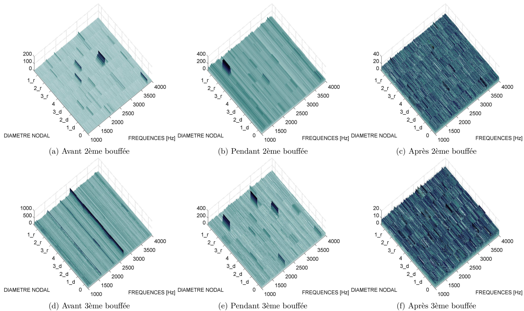
FIGURE 4.21 – Diagramme fréquences - diamètres nodaux du couvercle : Deuxième et troisième buffée
