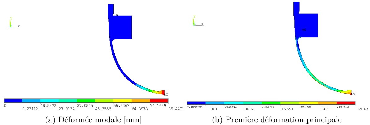
FIGURE 2.29 – Cartes d'intensité normalisées par rapport à la matrice de masse du déplacement total et de la première déformation principale du mode à 2 diamètres
