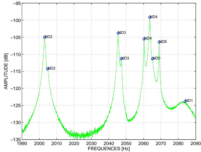
FIGURE 3.3 – Somme des modules des FRF mm/s/V obtenues avec les jauges d’extensométrie installées en bord d’attaque des pales principale du rouet à l’arrêt monté sur l’arbre. Mesure réalisée à P = 30 mbar et T_{amb} .
