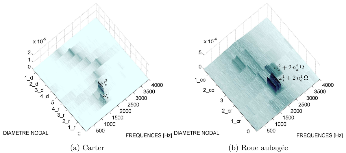
FIGURE 6.18 – Diagramme fréquences - diamètres nodaux à t > 2.78 s
