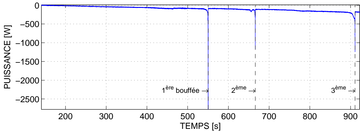
FIGURE 4.15 – Puissance développée à l'arbre lors du contact
