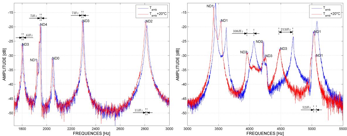
(a) FRFs de la première famille des modes de flexion (b) FRFs de la deuxième famille des modes de flexion
