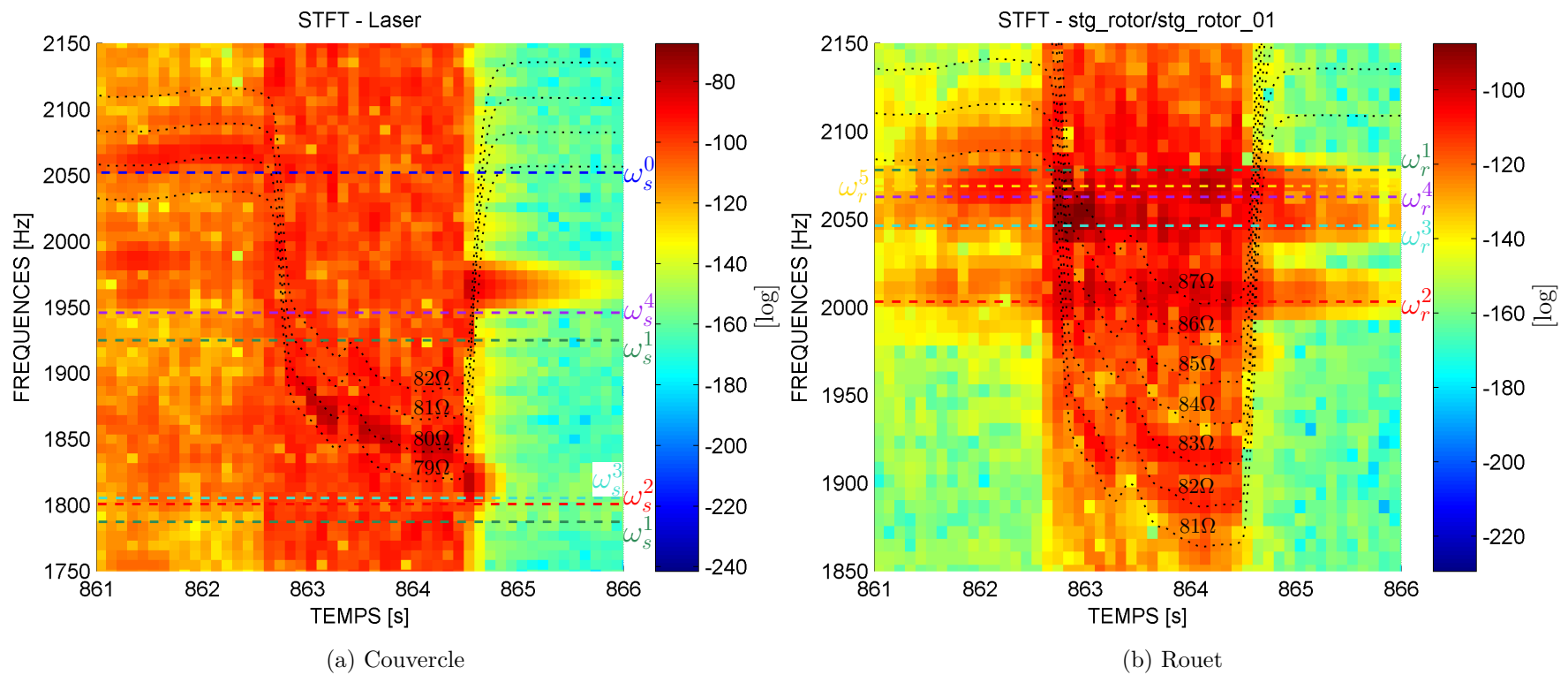
FIGURE 4.36 – STFT focalisée sur la huitième bouffée
