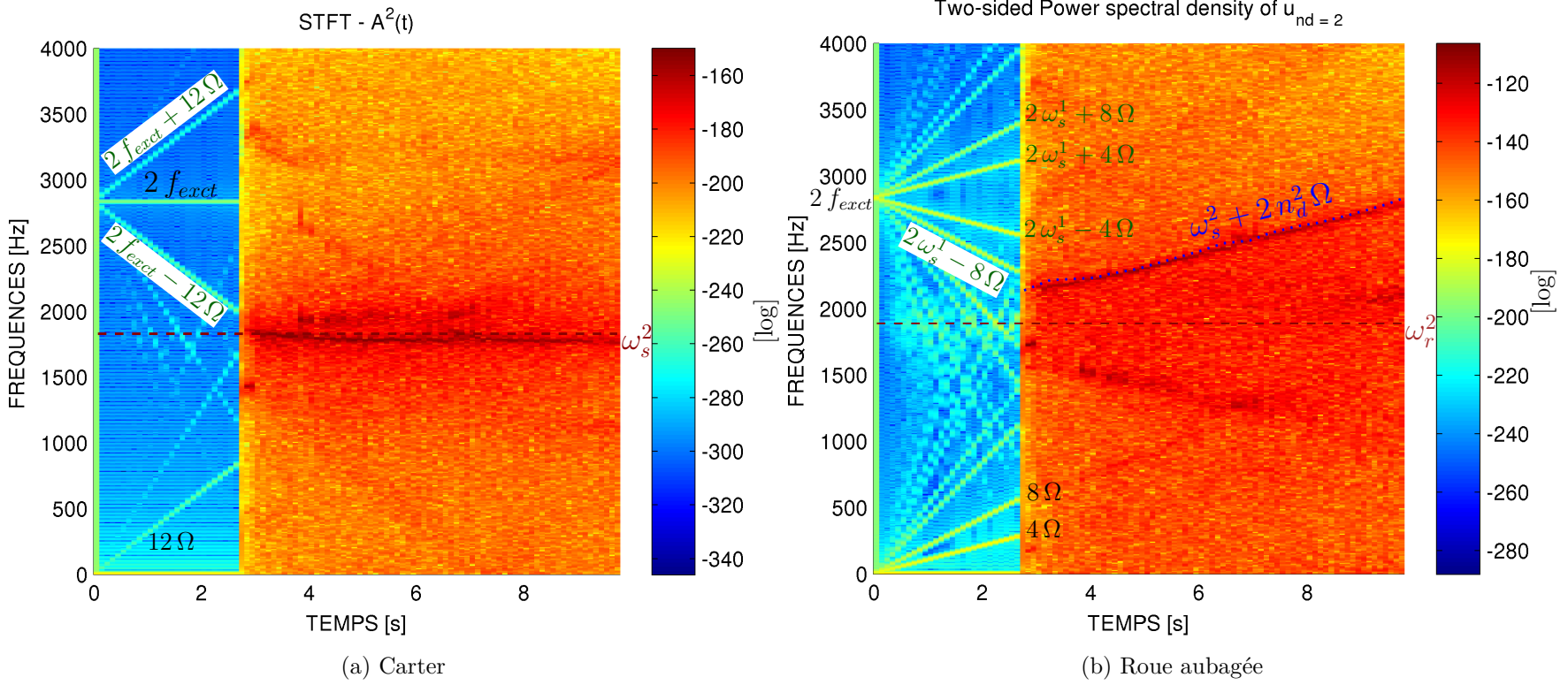
FIGURE 6.20 – STFT filtrée spatialement au diamètre deux
