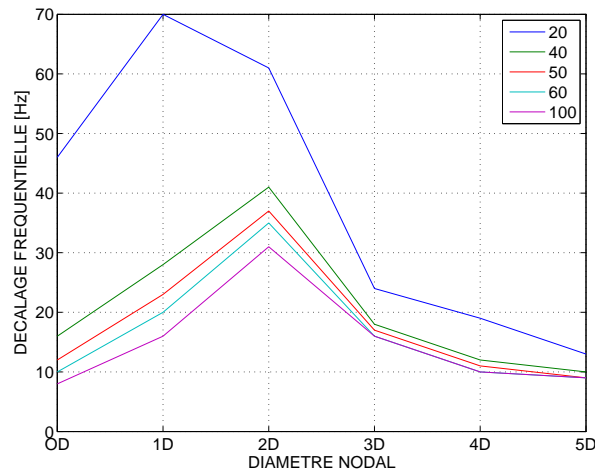
FIGURE 2.18 – Décalage en fréquence lié à l'ajout de l'enceinte à vide
