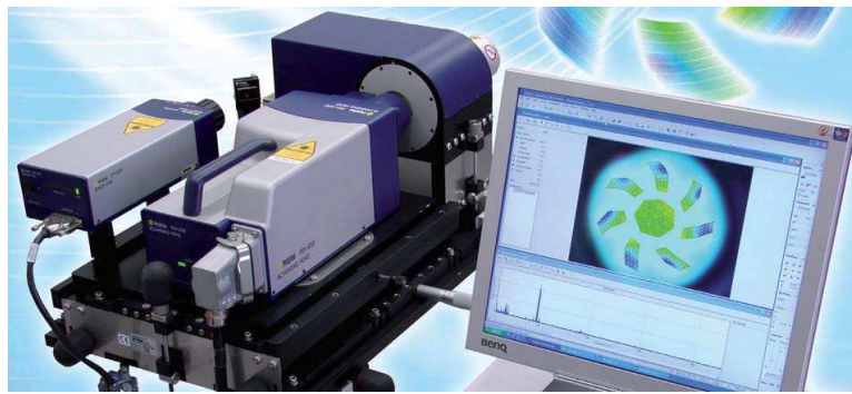
FIGURE 2.2 – Vibromètre PSV-400 associé au derotator [78]
