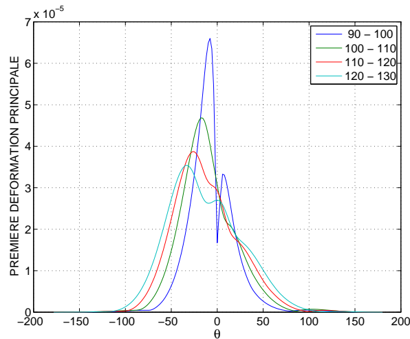
FIGURE 2.25 – Répartition circconférentielle de la première déformation principale en fonction de la position axiale du point d'application de l'effort
