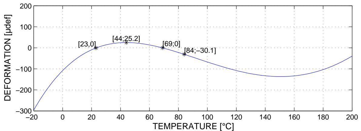
FIGURE 4.10 – Déformation apparente des jauges couvercle (données fournisseur)
