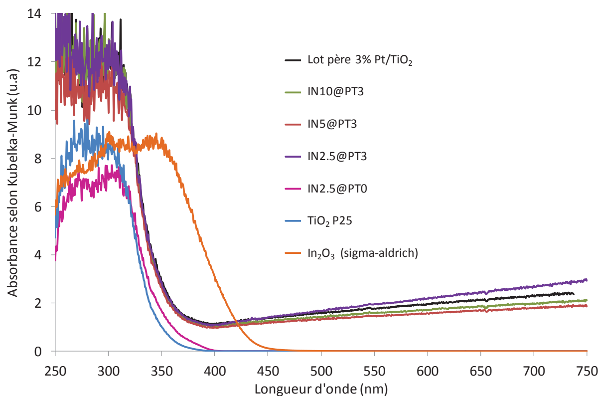
Figure 49 : Spectres d'absorption mesurés en SRD des différents composites IN_x@PT_3 et des références In_2O_3 , 3% Pt/TiO_2 et TiO_2 P25
