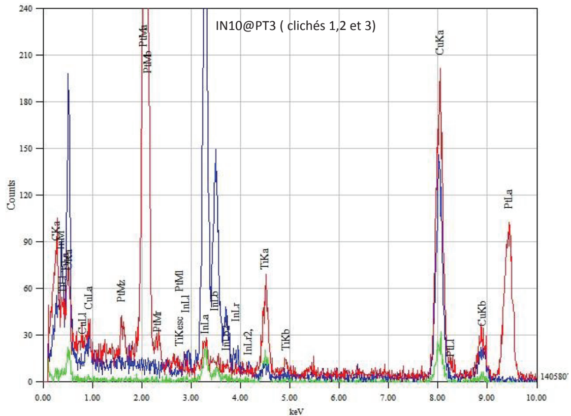
Figure 31 : Analyses EDX correspondant aux zones indiquées par des cercles rouge, bleu et vert sur les clichés 1, 2 et 3 du composite IN10@PT3
