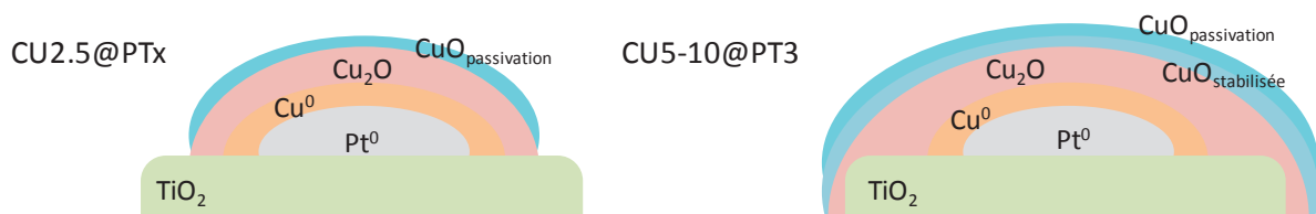
Figure 66 : Schéma descriptif simplifié des différents composites \text{Cu}_2\text{O}@Pt/\text{TiO}_2
