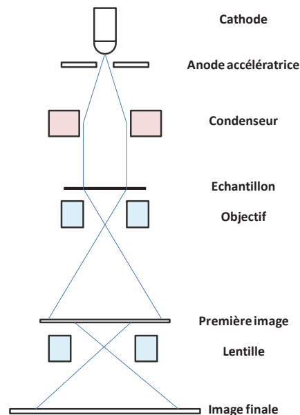
Figure 2 : Optique simplifiée d'un microscope électronique en transmission
