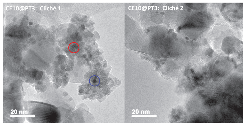
Figure 18 : Clichés de MET représentatifs des particules de Ce déposées en surface de TiO 2 pour le composite CE10@PT3 (les cercles de couleur correspondent aux zones analysées en EDX)
