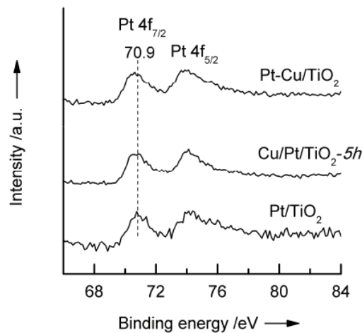
Figure 34 : Spectres XPS du Pt4f réalisés par Zhai et al. 23
