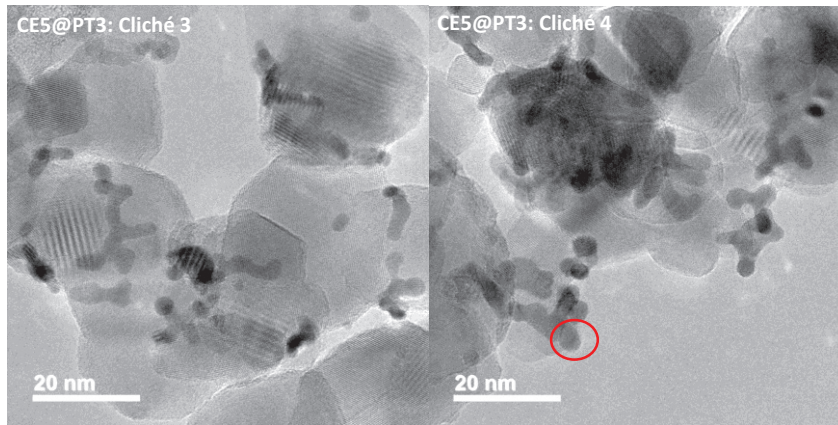
Figure 16 : Clichés de MET représentatifs des particules de Pt déposées en surface de TiO 2 pour le composite CE5@PT3 (le cercle rouge correspond à une zone analysée en EDX)
