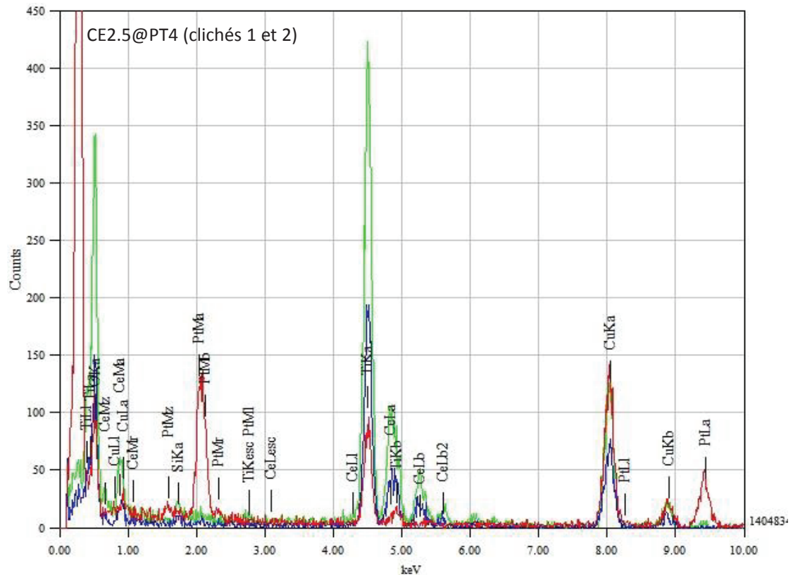
Figure 13 : Analyses EDX correspondant aux zones indiquées par des cercles rouge, bleu et vert sur les clichés 1 et 2 du composite CE2.5@PT4
