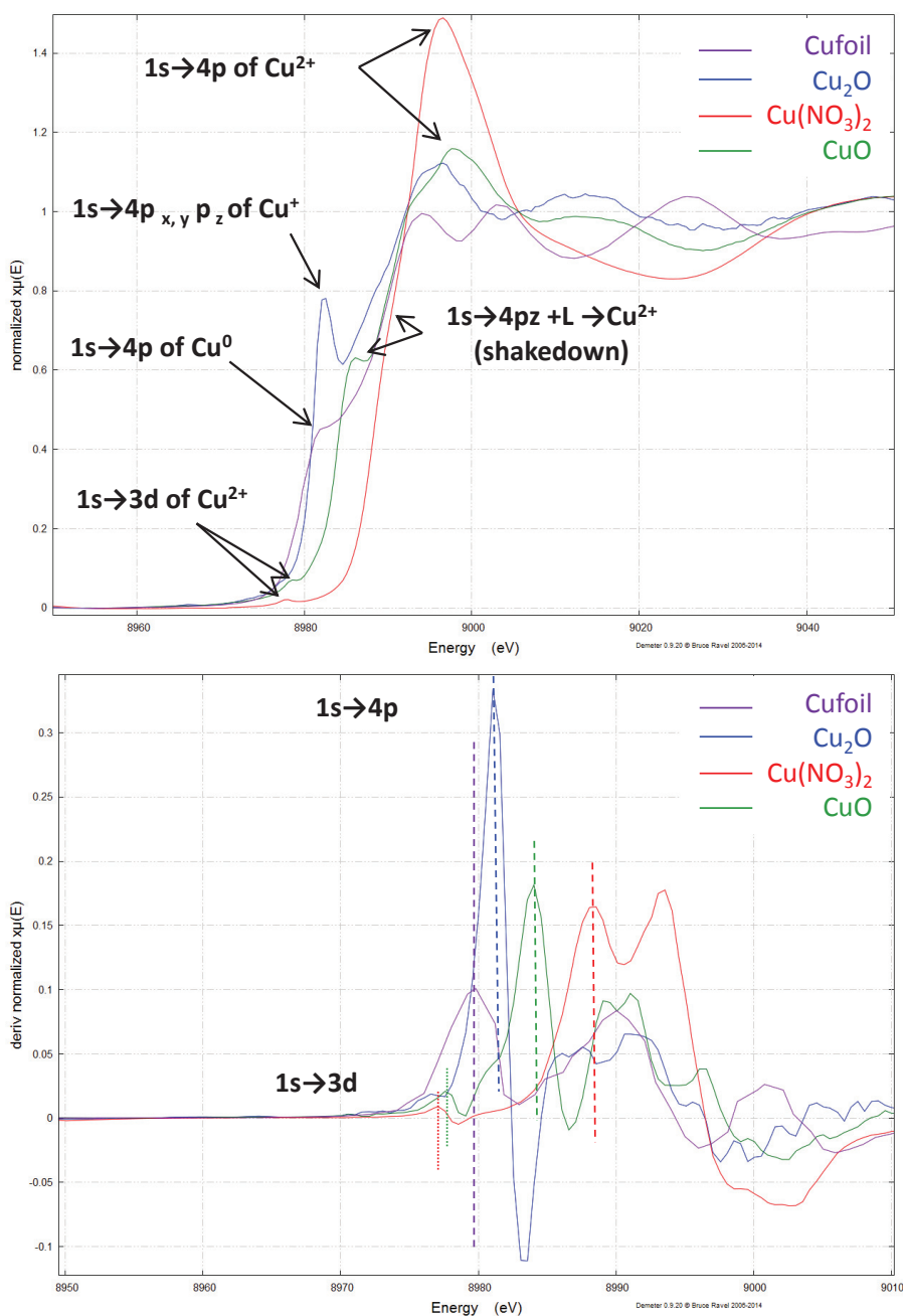
Figure 42 : Spectres XANES des références Cu, Cu 2 O, Cu(NO 3 ) 2 , et CuO (en haut) et les dérivées premières associées (en bas)
