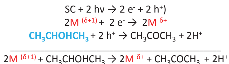
Figure 20 : Réactions mises en jeu lors du dépôt de \text{M}_x\text{O}_y par photoréduction (issu de la précipitation de \text{M}^{\delta+} )
