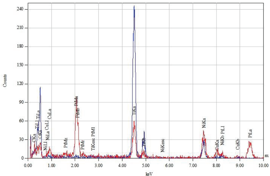
Figure 26 : Analyses EDX correspondants aux zones indiquées par les cercles rouge et bleu sur le cliché 1 du composite CU2.5@PT3
