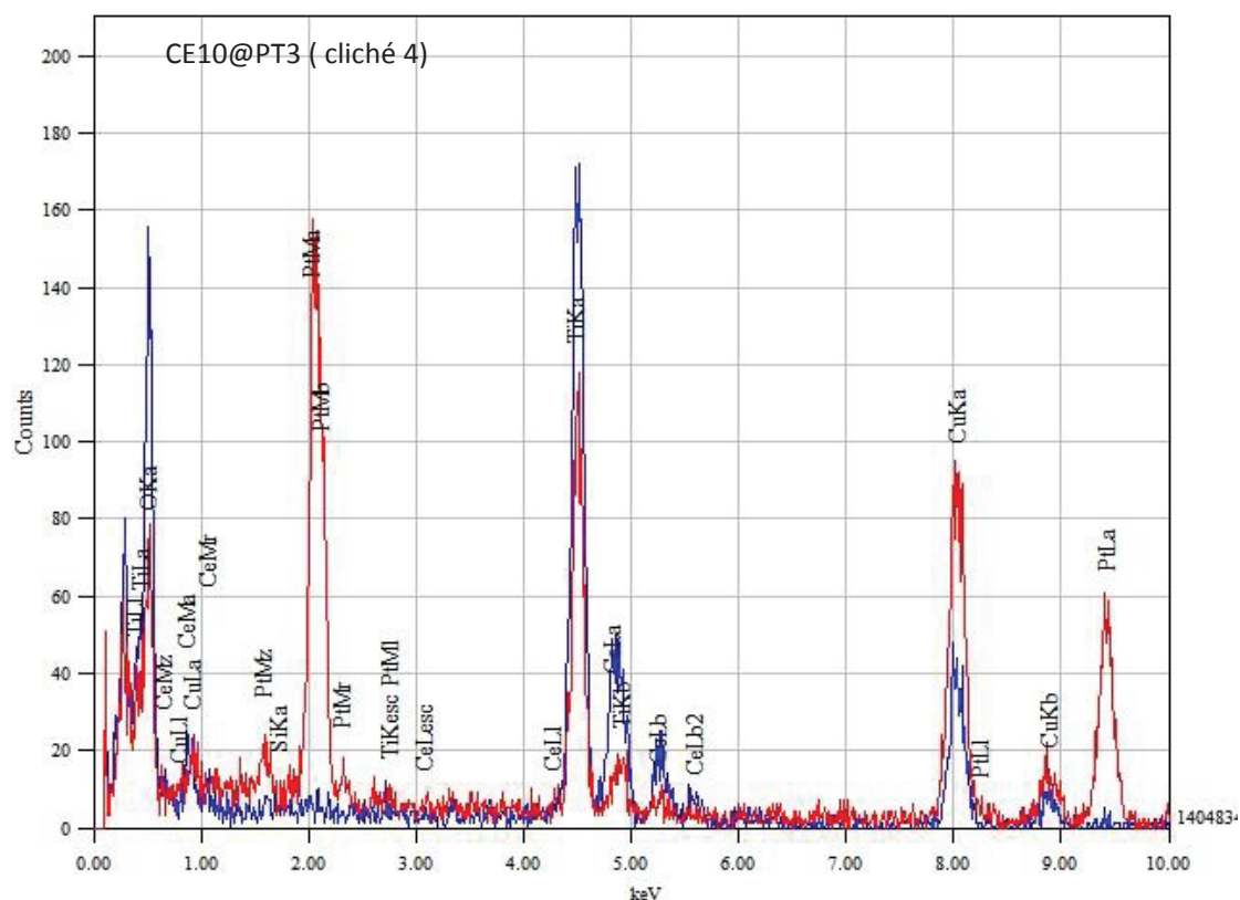
Figure 21 : Analyses EDX correspondant aux zones indiquées par des cercles rouge et bleu sur le cliché 4 du composite CE10@PT3
