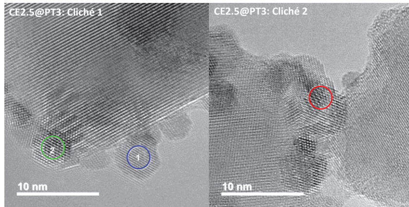
Figure 8 : Clichés de MET représentatifs des particules à base de Ce déposées en surface de TiO 2 pour le composite CE2.5@PT3 (les cercles de couleur correspondent aux zones analysées en EDX)
