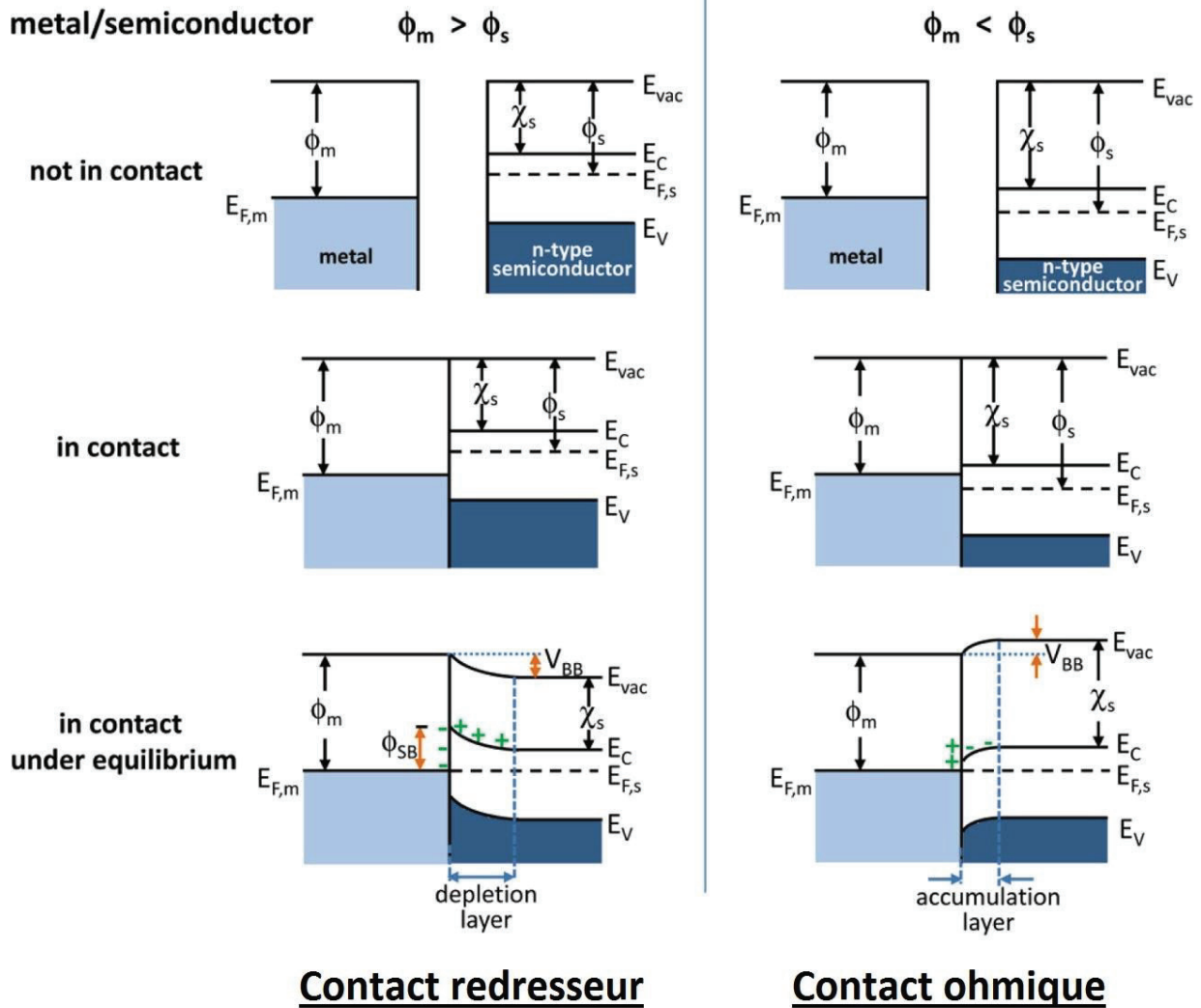
Figure 10 : Représentation schématique des différents cas de figure rencontrés lors d'un contact métal-semiconducteur de type n ( E_{vac} : énergie du niveau de vide, E_C : énergie minimum de la bande de conduction, E_V : énergie maximale de la bande de valence, \phi_m : fonction de travail du métal, \phi_s : fonction de travail du semiconducteur et \chi_s : affinité électronique du semiconducteur) 25
