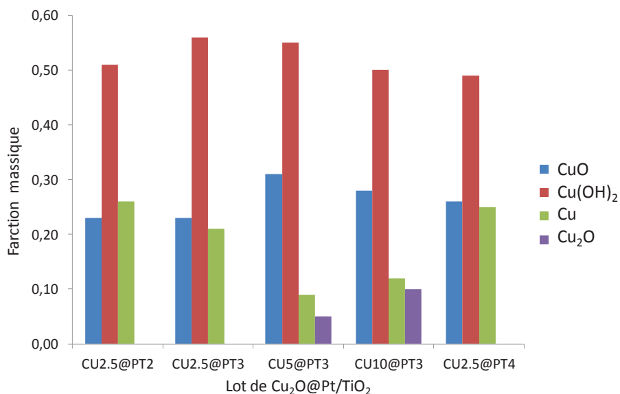
Figure 45 : Composition des lots CU y @Pt x obtenus par combinaison linéaire XANES
