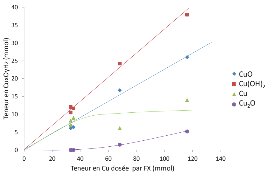
Figure 46 : Teneurs molaires en différents composés Cu x O y H z en fonction de la teneur molaire en cuivre totale dosée par FX
