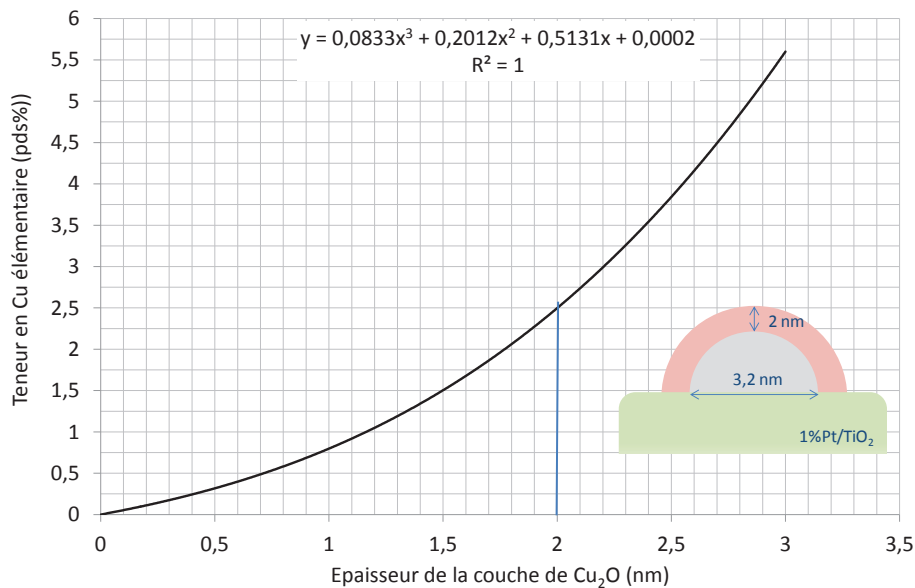
Figure 28 : Teneur en Cu en fonction de l'épaisseur de la couche de \text{Cu}_2\text{O} pour 1\% \text{Pt}/\text{TiO}_2
