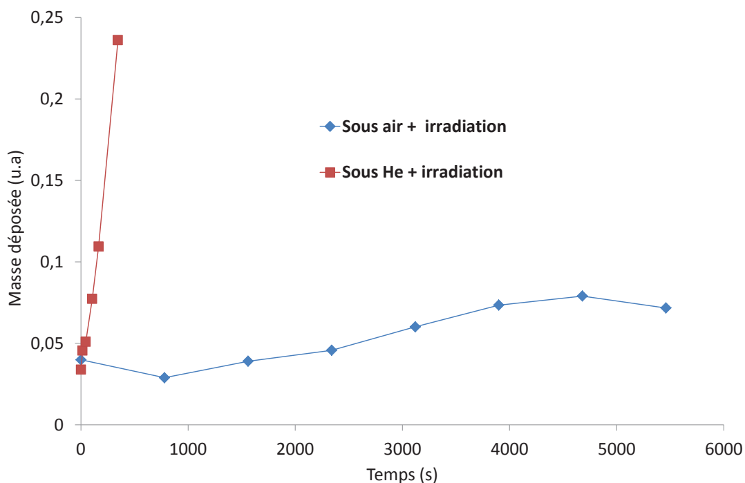
Figure 51 : Etude du dépôt de cuivre sur TiO 2 en fonction de l'atmosphère du milieu
