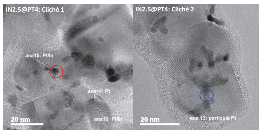
Figure 26 : Clichés de MET représentatifs du composites IN2.5@PT4 (les cercles de couleur correspondent aux zones analysées en EDX)
