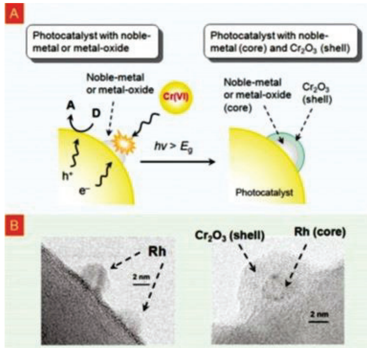
Figure 14 : A. Représentation schématique du processus de dépôt de Cr 2 O 3 par réduction photocatalysée des ions Cr VI . B. Clichés HR-MET de GaN :ZnO enrichi en particules de Rh avant (gauche) et après (droite) le recouvrement de celles-ci par la coquille de Cr 2 O 3 26
