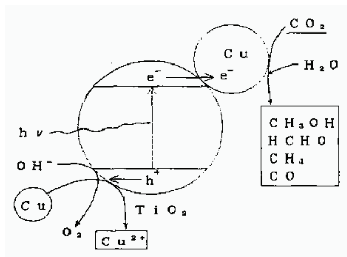
Figure 16: Schéma du fonctionnement supposé de la réduction du \text{CO}_2 photocatalysée par un mélange de poudres de \text{TiO}_2 et \text{Cu} en suspension 68
