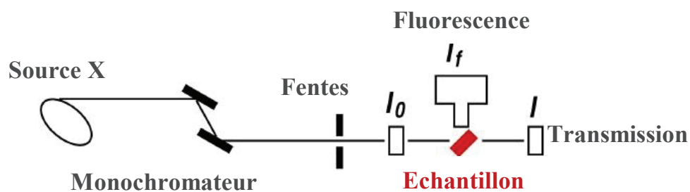
Figure 5 : Schéma décrivant les différents principes de détections utilisés en XAS
