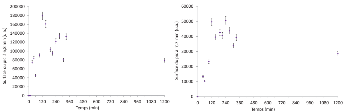
Figure 13 : Surface des pics à 6,8 min (à gauche) et 7,7 min (à droite) au cours du test de réduction photocatalytique des carbonates pour le photocatalyseur CU2.5@PT1
