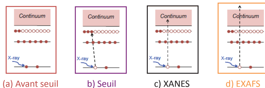
Figure 4 : Description des différents phénomènes mis en jeu lors de l'acquisition d'un spectre d'absorption X 7
