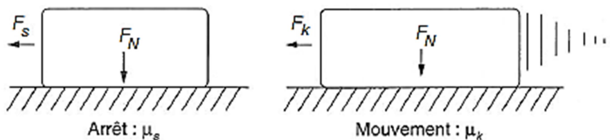
Figure 2 : Coefficients de frottement statique et dynamique
