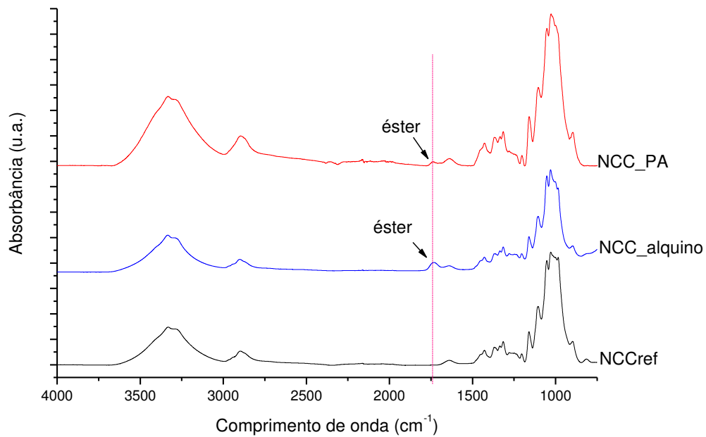
Figura 5.34 Espectros de FTIR do NCC de partida (NCCref), do NCC modificado com radical alquino (NCC_alquino) e após a reação de click chemistry (NCC_PA).
