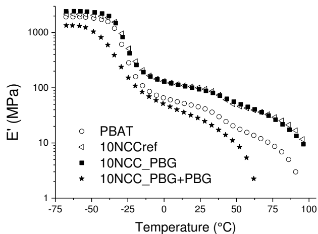
Figura 5.25 Curvas do módulo de armazenamento versus temperatura.
