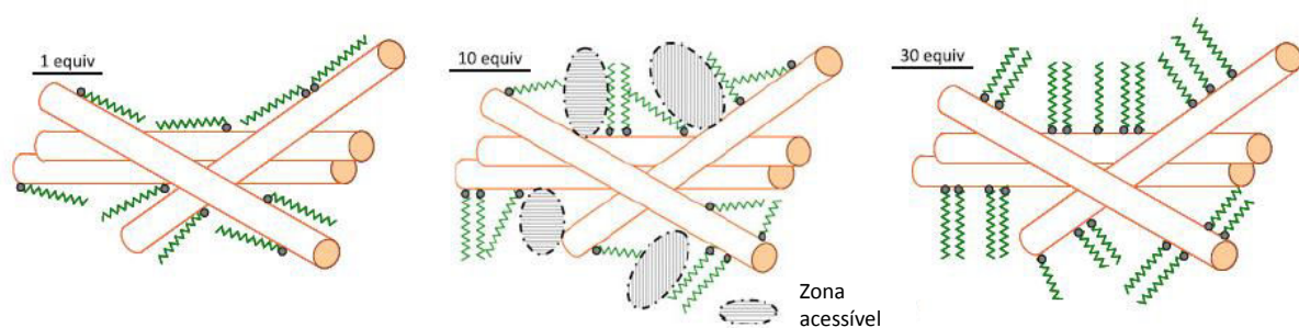
Figura 3.22 Representação esquemática da distribuição das longas cadeias alifáticas de octadecil isocianato na superfície das microfibrilas de celulose.
