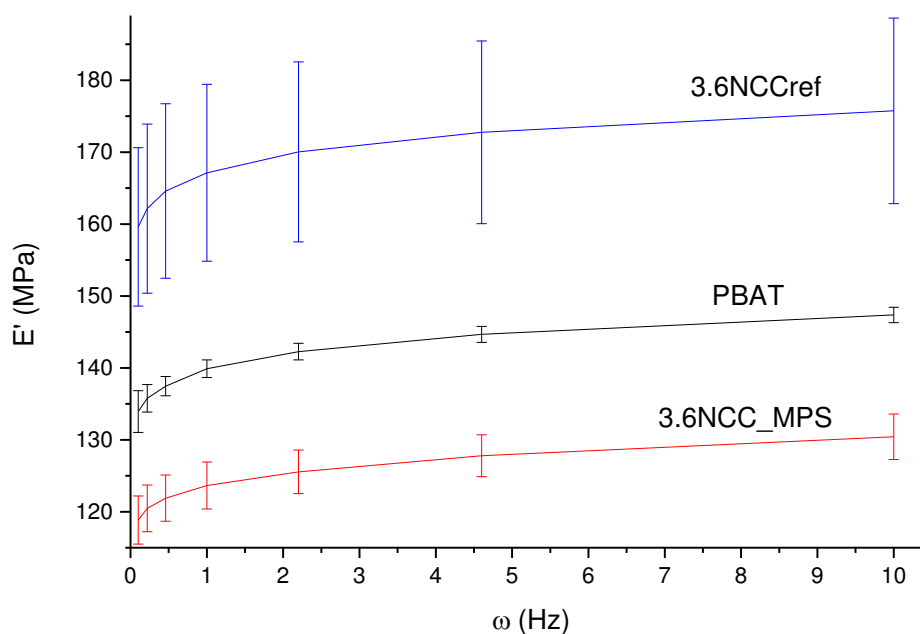
Figure 5 Variation des modules élastiques de conservation ( E' ) en fonction des fréquences de sollicitation de l'échantillon ( \omega ).
