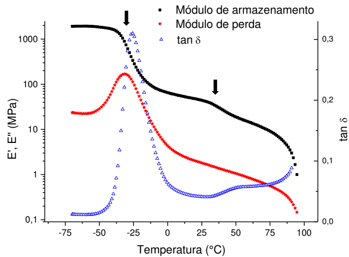
Figura 5.24 Curvas do módulo de armazenamento ( E' ), do módulo de perda ( E'' ) e de \tan \delta em função da temperatura, para o PBAT extrudado puro. As setas indicam as transições térmicas discutidas.
