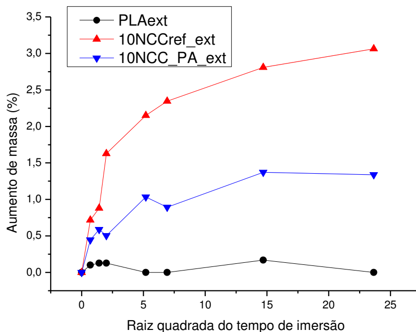
Figura 5.46 Evolução do aumento de massa dos compósitos causado pela absorção de água em função do tempo de imersão (5 semanas).
