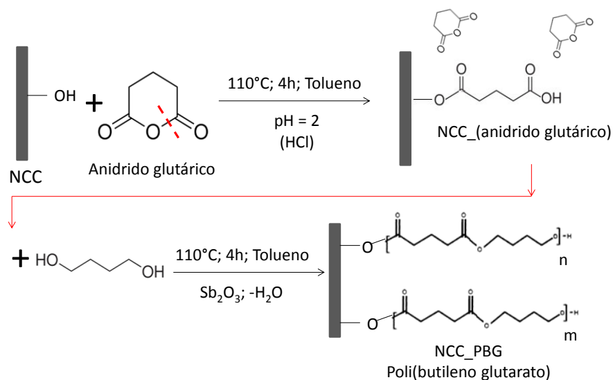
Figura 4.7 Esquema da reação enxertia de NCC com PBG por polimerização in situ .
