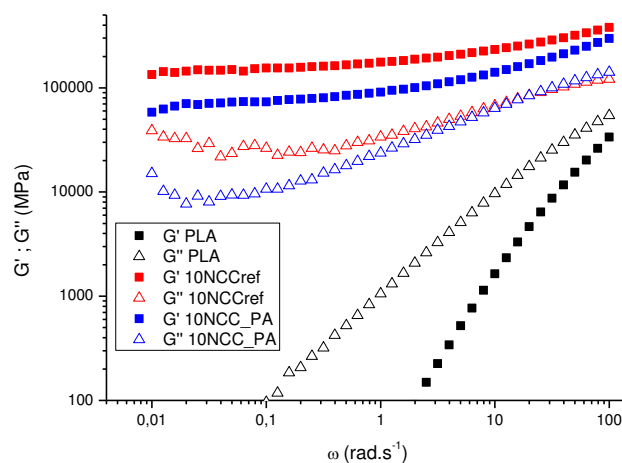
Figura 5.44 Módulo de armazenamento ( G' ; pontos preenchidos) e módulo de perda ( G'' ; pontos não preenchidos) em função da frequência.
