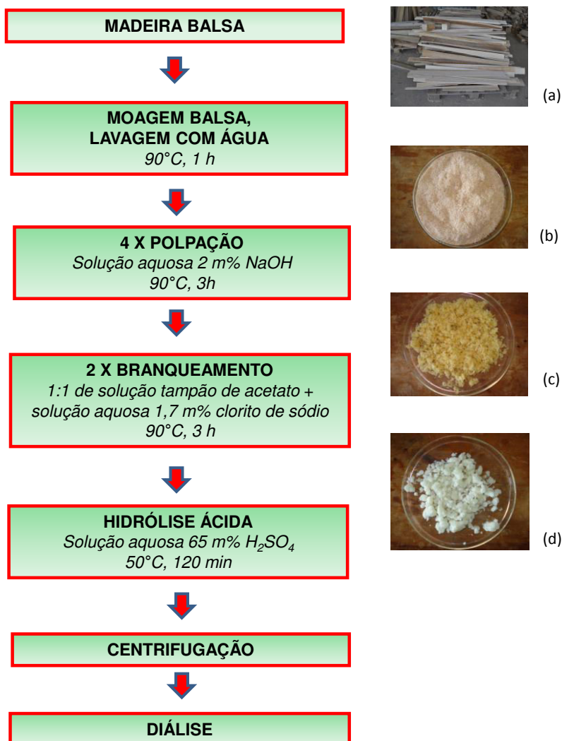
Figura 4.3 Etapas do processo de obtenção de NCC a partir da madeira balsa. As fotos representam as ripas de madeira balsa (a); e o estado da balsa após a moagem (b); após as quatro etapas de polpação (c) e após as duas etapas de branqueamento (d).
