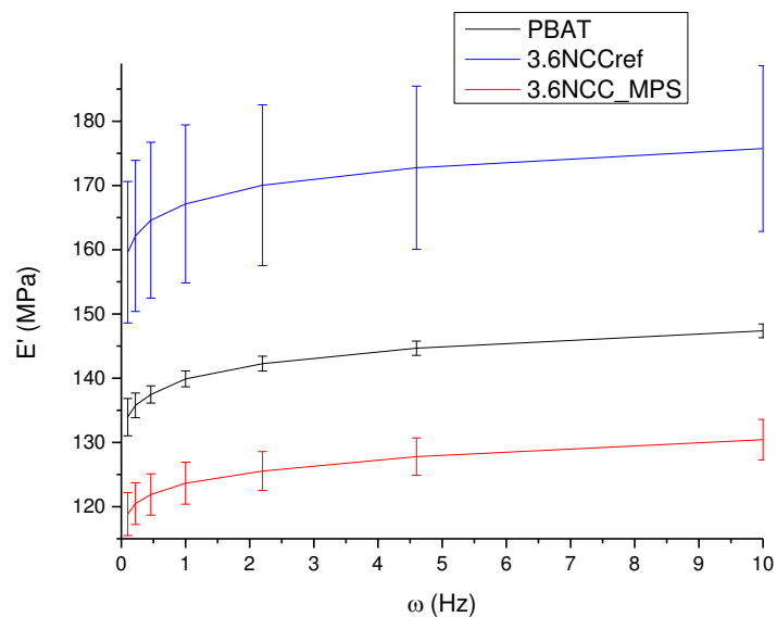
Figura 5.31 Curvas E' x \omega para as três distintas amostras, com os desvios padrão correspondentes.
