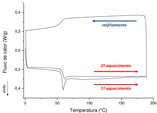
Figura 5.39 Curva do compósito 10NCCref_ext representando o comportamento típico em DSC de todas as amostras de PLA, com ou sem NCC.
