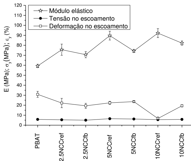
Figura 5.17 Módulo elástico (E), tensão no escoamento ( \sigma_y ) e deformação no escoamento ( \epsilon_y ) dos filmes obtidos por extrusão e termoprensagem.
