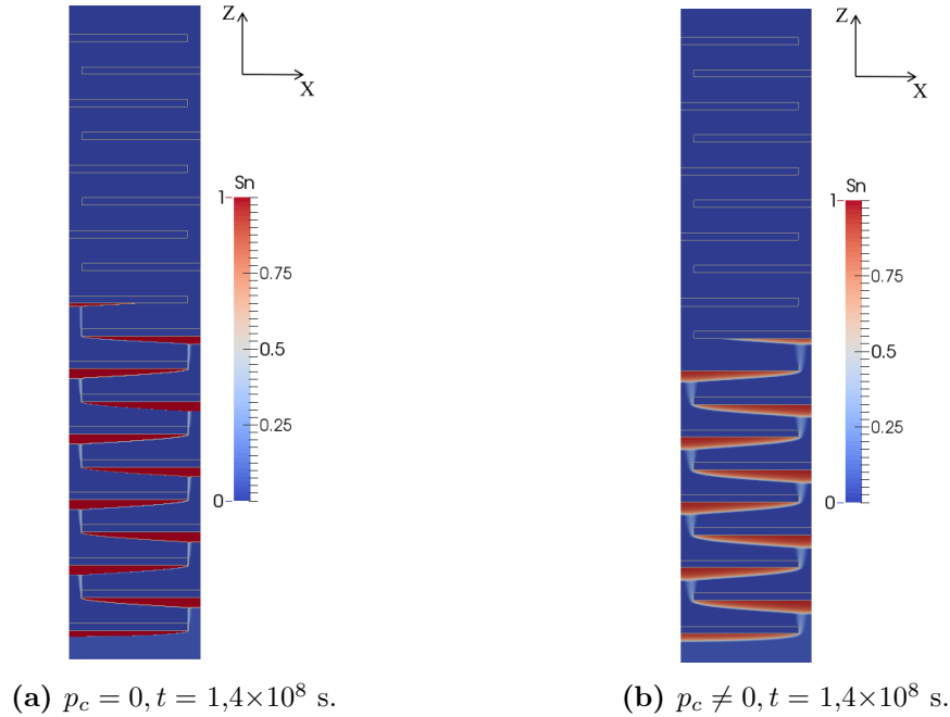
Figure 4.25 – Inclusions imperméables : évolution du \text{CO}_2 dans la colonne bi-dimensionnelle pour une saturation imposée S_i = 0,05 dans les cas sans capillarité (à gauche) et avec capillarité (à droite). Les interfaces entre la matrice et les inclusions sont représentés par les traits continus.
