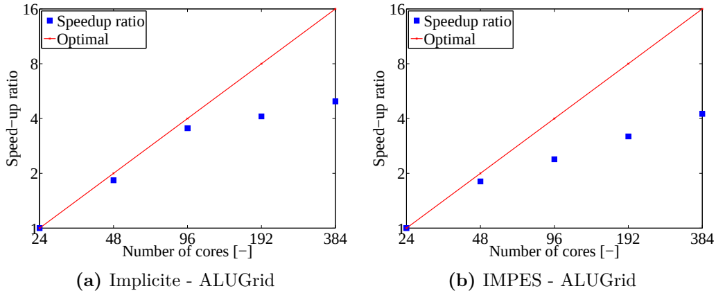
Figure 5.4 – Représentation log-log de l'accélération pour le cas implicite - ALUGrid(a) et IMPES - ALUGrid (b).
