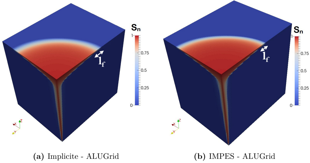
Figure 5.3 – Carte de saturation de CO 2 après 20 ans d’injection pour les simulations utilisant le schéma implicite (a) et IMPES (b). La direction Z est multipliée par un facteur de 50.
