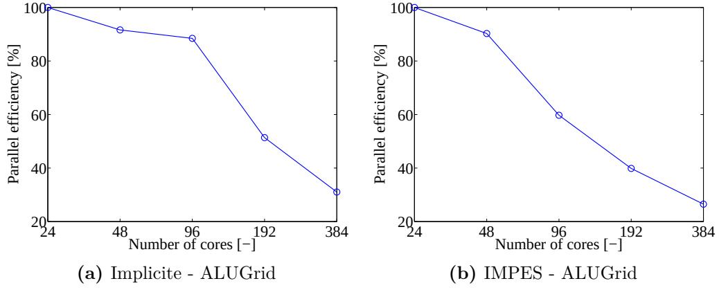
Figure 5.5 – Efficacité parallèle pour le cas implicite - ALUGrid(a) et IMPES - ALUGrid (b).
