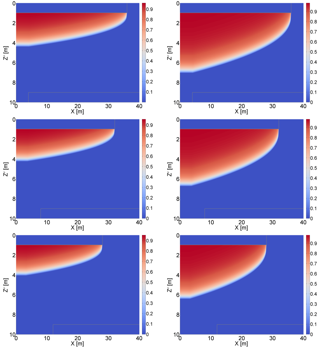
Figure 4.20 – Cas avec capillarité - Inclusions imperméables : reconstruction de la solution du problème local à petite échelle obtenue par l'approche de courant de gravité : 2L = 72 [m] (haut), 2L = 64 [m] (milieu) et 2L = 56 [m] (bas) pour la saturation imposée S_i = 0,05 (à gauche) et S_i = 0,10 (à droite) . Les traits en gris représentent les interfaces entre la matrice et les inclusions.
