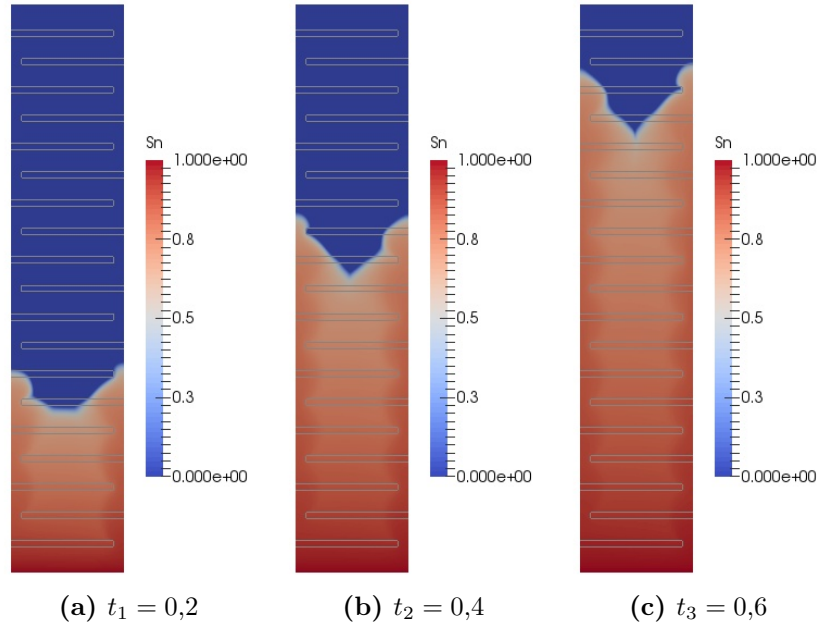
Figure A.3 – Carte de saturation du CO 2 dans la colonne bi-dimensionnelle à différents temps pour N_g = 0,1 . Les interfaces entre la matrice et les inclusions sont représentées par les rectangles. Le temps est adimensionné (équation (A.1)).
