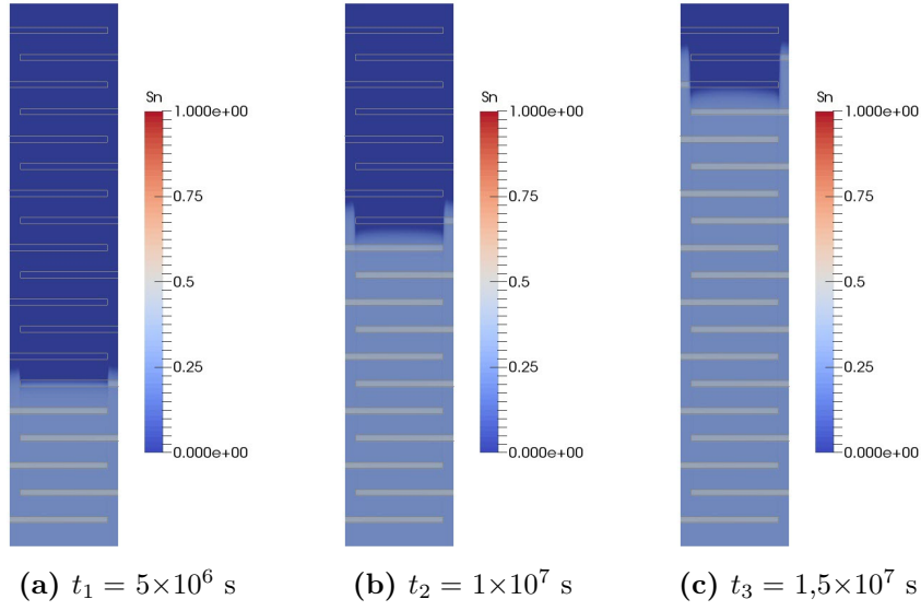
Figure B.3 – Carte de saturation du \text{CO}_2 dans la colonne bi-dimensionnelle aux différents temps pour S_i = 0,25 < S_{li}^m . Ici, le temps est le temps réel non-adimensionné.
