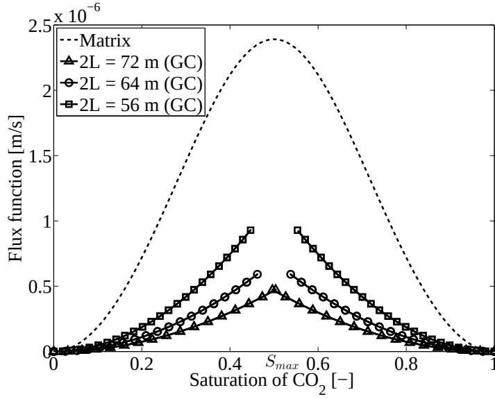
Figure 4.15 – Cas sans capillarité - Inclusions imperméables : flux gravitaire effectif en fonction de la saturation moyenne de \text{CO}_2 . La ligne discontinue présente le flux dans la matrice homogène. Les lignes continues avec symboles montrent le flux gravitaire mis à l'échelle et calculé par l'approche de courant de gravité, pour différentes valeurs de la longueur de l'inclusion.
