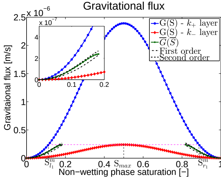
Figure 4.17 – Flux gravitaire dans la matrice (en bleu), dans l'inclusion (en rouge) et celui mis à l'échelle calculé numériquement (en vert) avec, ses approximations au premier et second ordre. La fenêtre rectangulaire en haut à gauche présente un zoom pour la partie de faible saturation.
