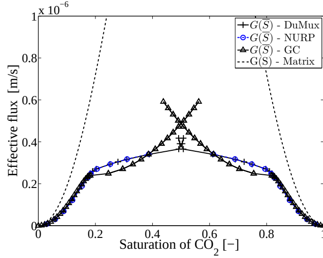
Figure 4.35 – Cas sans capillarité - Inclusions perméables : flux effectif mis à l'échelle obtenu à partir des simulations diphasiques pour le cas L_0 = 40m et H_c = 10m .
