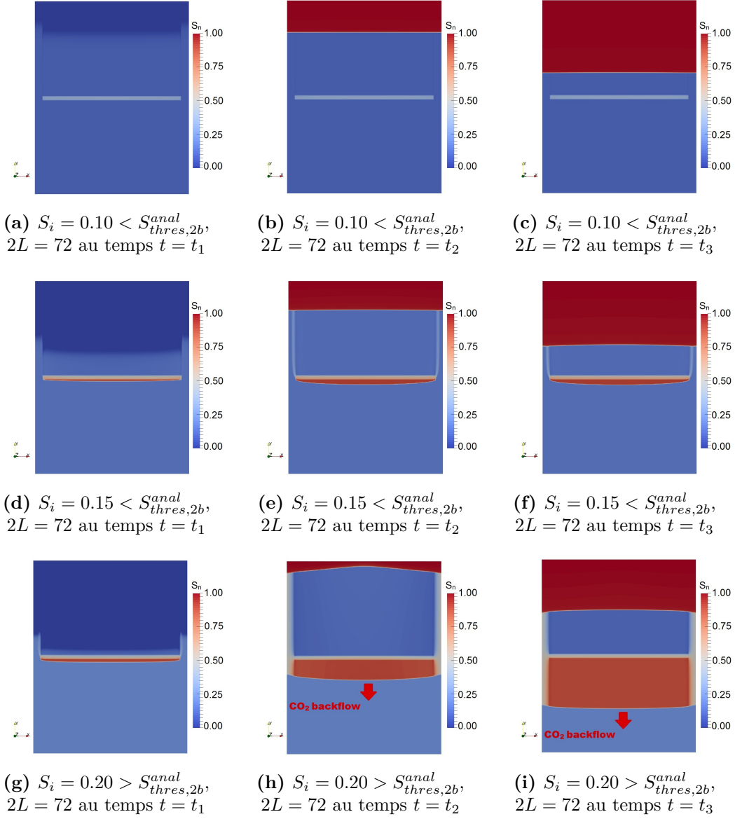
Figure 4.7 – Cas 3b - Cas sans capillarité - Inclusion semi-pérmeable : distribution du CO_2 à un temps court t_1 (a,d,g) quand le front de CO_2 arrive à la barrière semi-pérmeable, à un temps intermédiaire t_2 (b,e,h) et à un temps relativement long t_3 (c,f,i) pour 2L = 72 [m].
