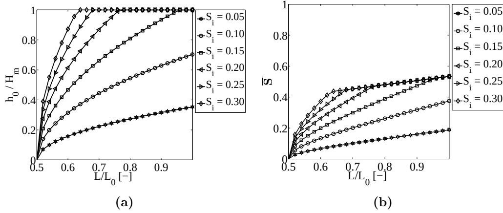
Figure 4.13 – Influence de la longueur de l'inclusion sur la hauteur maximale du courant de gravité et sur la saturation moyenne \bar{S} dans le cas L_0 = 40m .
