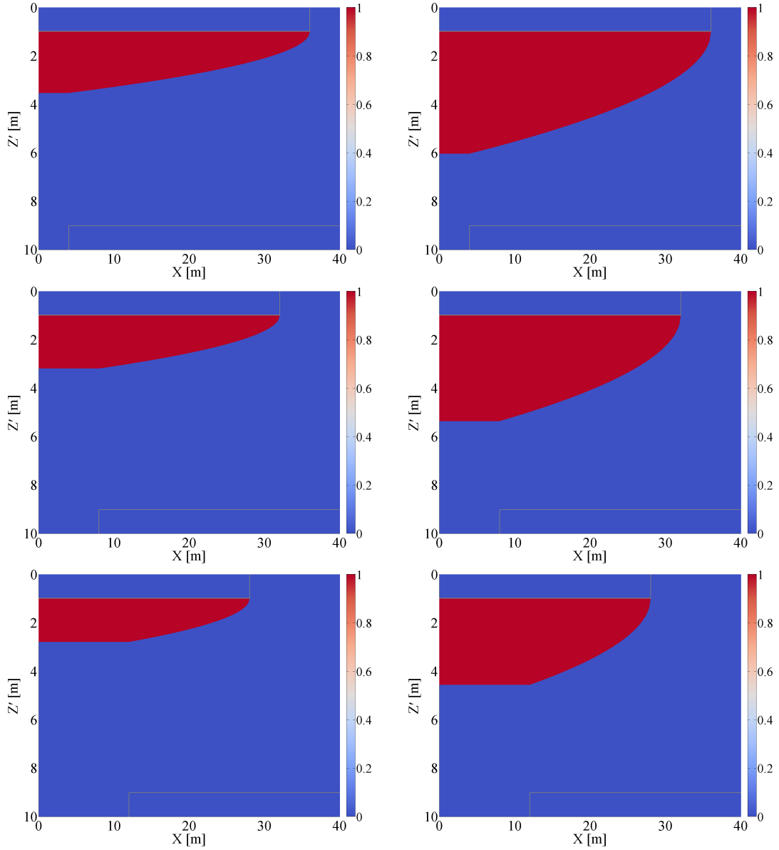
Figure 4.12 – Cas sans capillarité - Inclusions imperméables : reconstruction de la solution du problème local à petite échelle obtenue par l’approche des courants de gravité : 2L = 72 [m] (haut), 2L = 64 [m] (milieu) et 2L = 56 [m] (bas) pour la saturation imposée S_i = 0,05 (à gauche) et S_i = 0,10 (à droite) . Les traits en gris représentent les interfaces entre la matrice et les inclusions.
