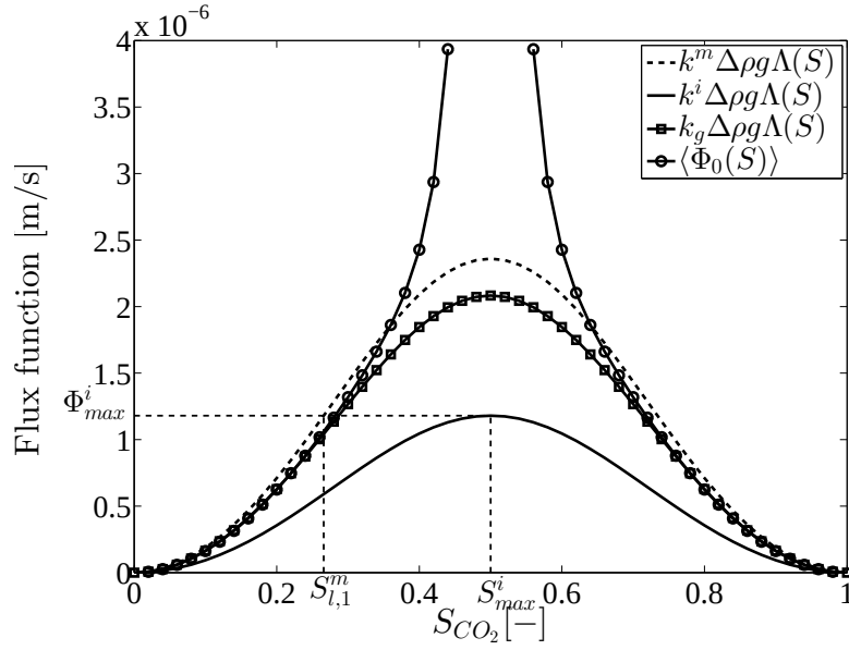
Figure B.2 – Flux gravitaire effectif en fonction de la saturation S_{CO_2} pour le cas k^i/k^m = 0,50 ( k^m = 3 \times 10^{-12} \text{ m}^2 et k^i = 1,5 \times 10^{-12} \text{ m}^2 ). La saturation pour G^i(S) maximal est S_{max}^i = 0,50 et la saturation S_{l_1}^m pour que G^m(S_{l_1}^m) soit égal au flux gravitaire maximal dans l'inclusion \Phi_{max}^i est égale à 0,265.
