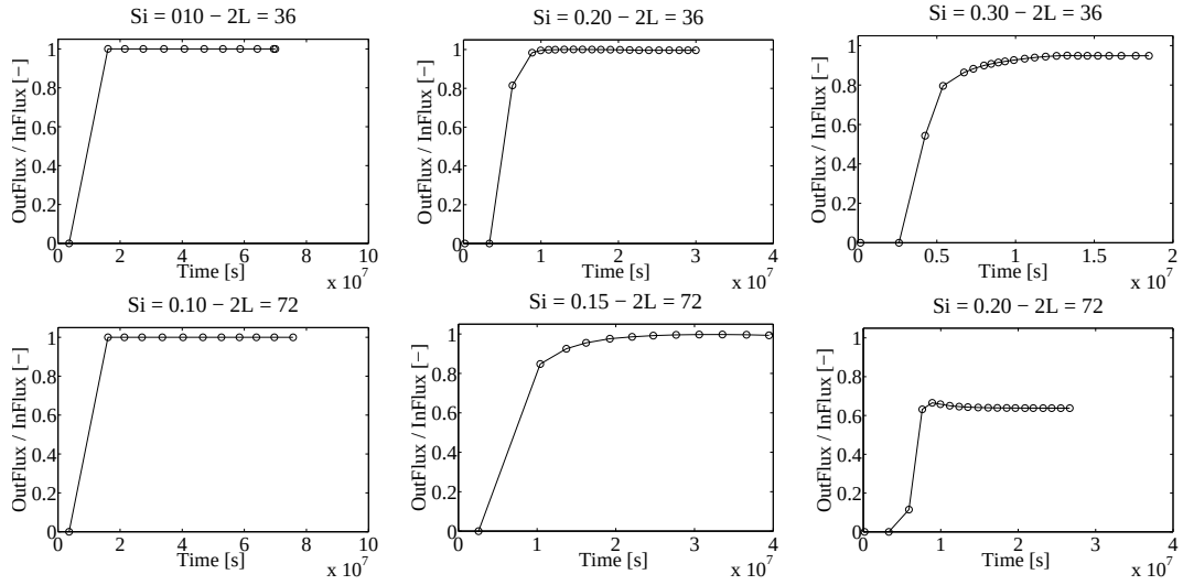
Figure 4.8 – Cas 3b - Cas sans capillarité - Inclusion semi-pérmeable : Comparaison entre le flux sortant à travers les intervalles et le flux entrant en bas de la colonne au cas où 2L = 36 [m] (haut) et 2L = 72 [m] (bas), en se basant sur les résultats des simulations numériques à l'aide du code DuMu x .
