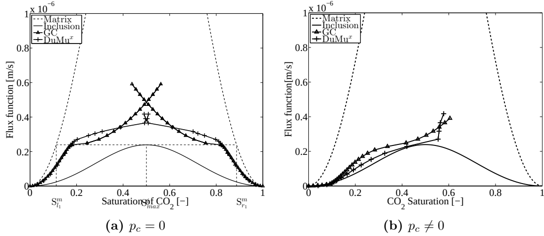
Figure 4.28 – Inclusions perméables : flux total effectif pour le cas sans capillarité (à gauche) et avec capillarité (à droite). La longueur des inclusions est fixée à 2L = 72m .
