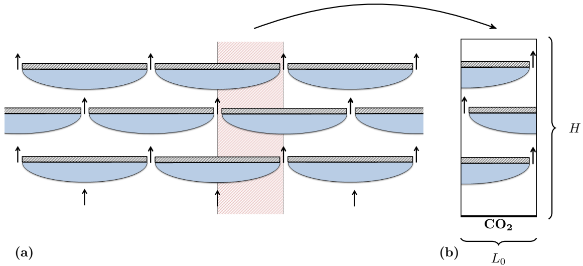
Figure 4.1 – Schéma d'écoulement du \text{CO}_2 dans un milieu bidimensionnel stratifié périodique (a). Le problème se simplifie en un écoulement dans une colonne verticale (b) sous réserve que les conditions initiales et aux limites soient également périodiques.
