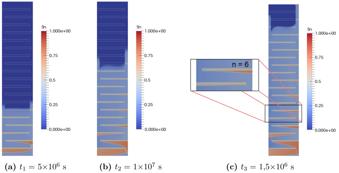
Figure B.4 – Carte de saturation de \text{CO}_2 dans la colonne bi-dimensionnelle aux différentes temps pour S_i = 0,30 > S_{li}^m . Le temps n'est pas adimensionné.
