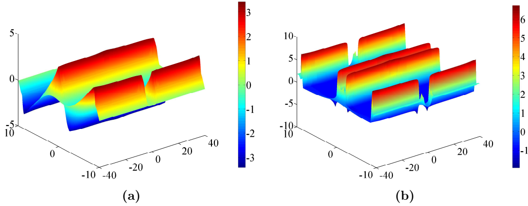
Figure A.2 – Fonction \psi_3 (a) et le gradient \partial\psi_3/\partial Y_3 (b) dans la cellule pour le rapport k^i/k^m = 0,10 .
