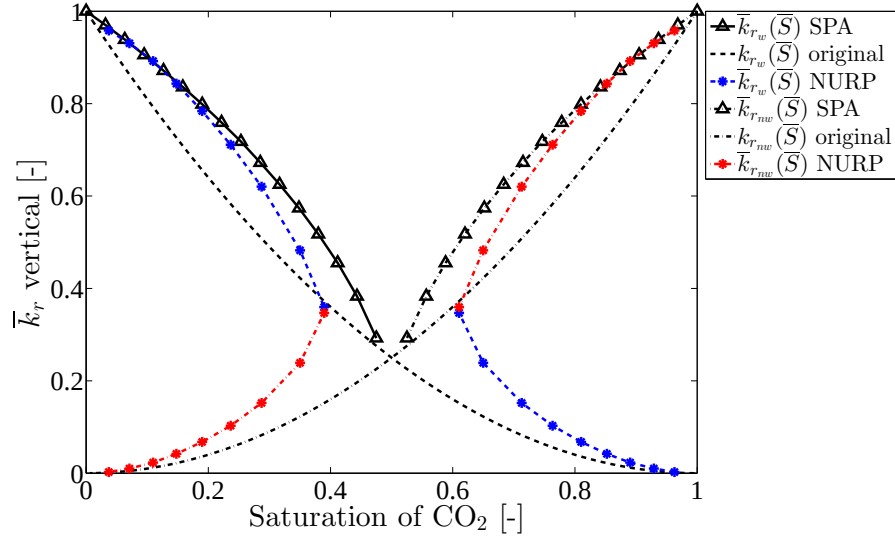
Figure 4.31 – Cas sans capillarité - Inclusions imperméables : perméabilités relatives effectives de la saumure (ligne discontinue bleue avec étoiles) et du \text{CO}_2 (ligne discontinue-pointillée rouge avec étoiles), obtenues avec les méthodes SPA et NURP dans le cas 2L = 72m , L_0 = 40m et H_c = 10m .
