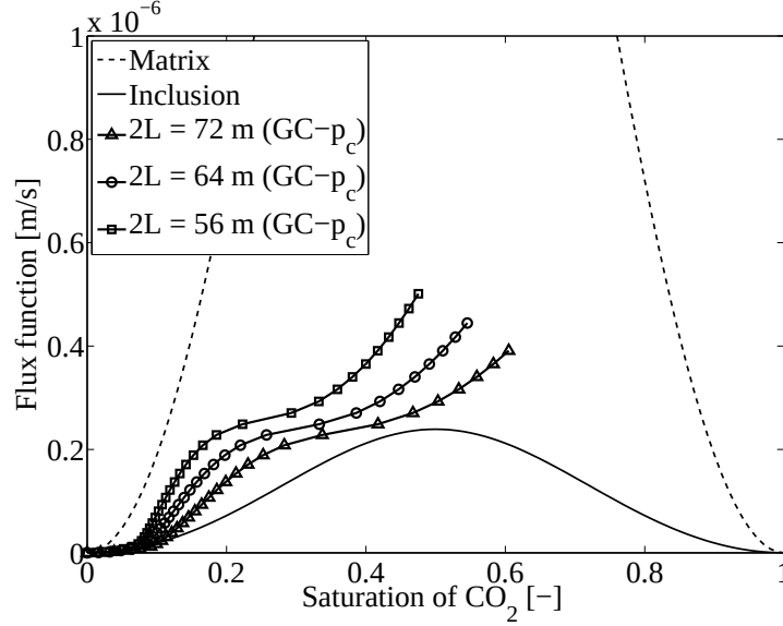
Figure 4.24 – Cas avec capillarité - Inclusions perméables : Flux total mis à l'échelle calculé numériquement pour des inclusions semi-perméables de 2L = 56 [m], 2L = 64 [m] et 2L = 72 [m] de longueur.
