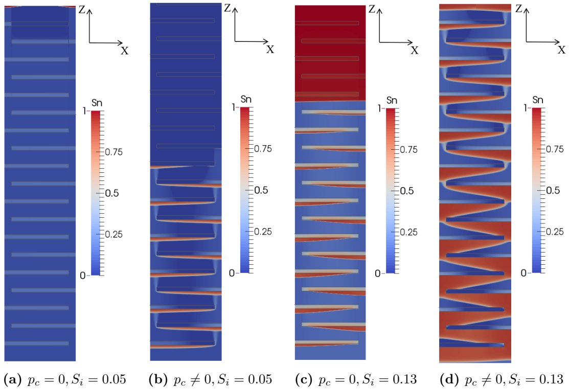
Figure 4.27 — Inclusions perméables : carte de saturation du \text{CO}_2 dans la colonne bi-dimensionnelle au temps t = 1,0 \times 10^8 s pour les cas sans capillarité (a,c) et avec capillarité (b,d).
