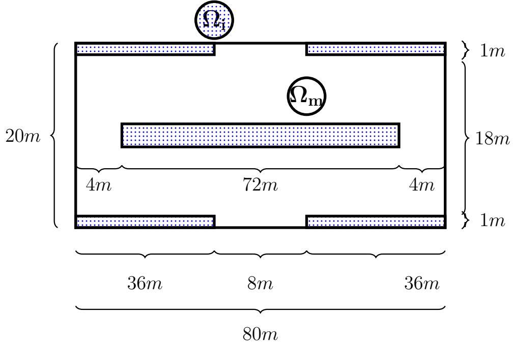
Figure A.1 – Dimensions d'une cellule.
