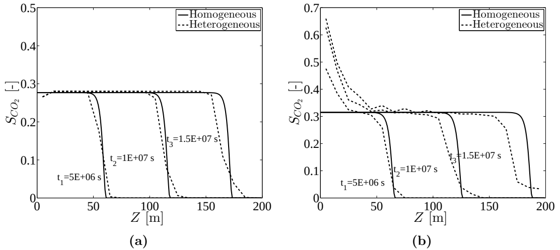
Figure B.6 – Profil de saturation de \text{CO}_2 analytique dans un milieu homogène équivalent (continu) et numérique dans le milieu hétérogène (discontinu) pour les cas S_i = 0,25 (a) et S_i = 0,30 (b).
