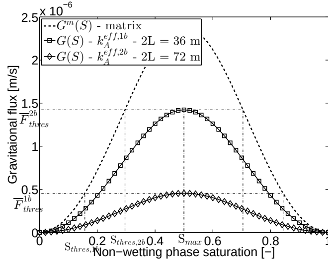
Figure 4.9 – Flux gravitaire de la zone équivalente pour 2L = 36 [m] et 2L = 72 [m]
