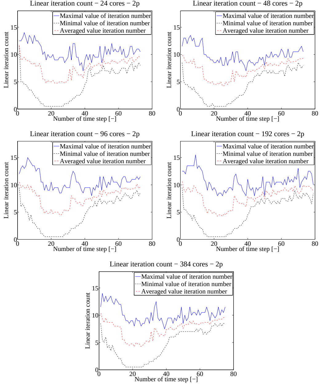
Figure 5.14 – Le nombre d'itération maximal, minimal et moyen pour chaque pas de temps des simulations du cas Implicite - ALUGrid. Ces courbes restent quasiment inchangées quand le nombre de processeur augmente.
