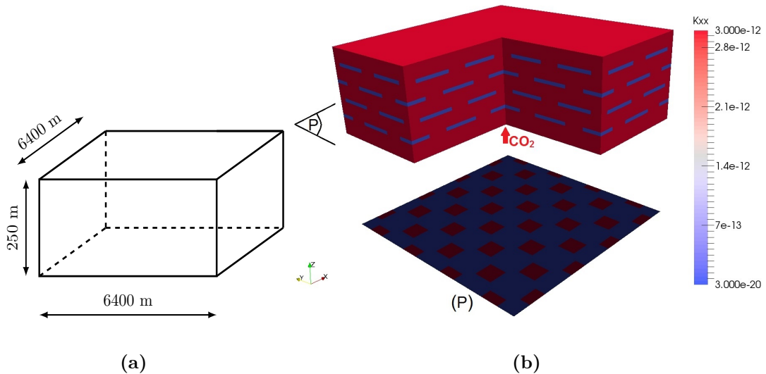
Figure 5.8 – Milieu à strates périodiques : Dimension (a) et champs de perméabilité (b). La hauteur du milieu dans la Figure (b) est multiplié par un facteur 10. La surface (P) montre la forme d'une strate typique.
