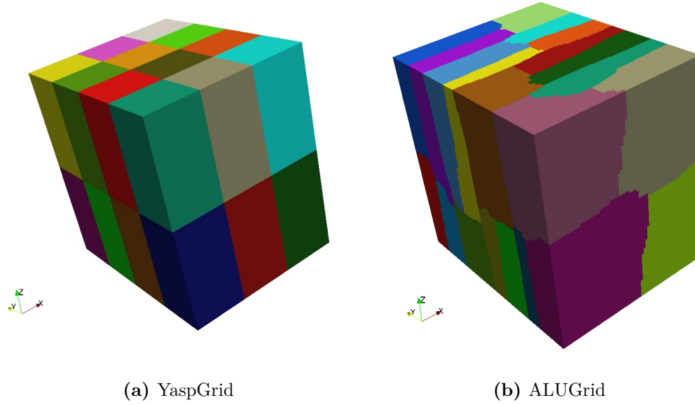
Figure 5.6 – Décomposition de domaines pour la simulation sur 24 cœurs avec YaspGrid (a) et ALUGrid (b).
