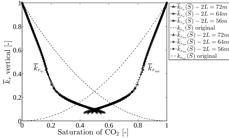
Figure 4.33 – Cas sans capillarité - Inclusions perméables : perméabilité relative mise à l'échelle obtenue à partir des simulations des écoulements monophasiques dans le cas L_0 = 40m et H_c = 10m pour trois géométries de VER.
