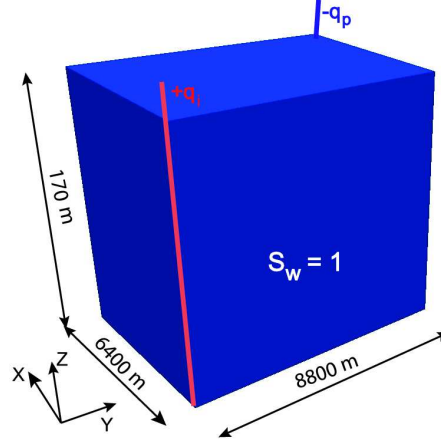
Figure 5.2 – Configuration du cas de test de performance : milieu 3D homogène avec un puits d'injection et un autre puits de production en deux coins opposés du domaine. Chaque puits s'étend verticalement à travers tout le réservoir. La dimension suivant l'axe Z est multipliée par un facteur de 50.
