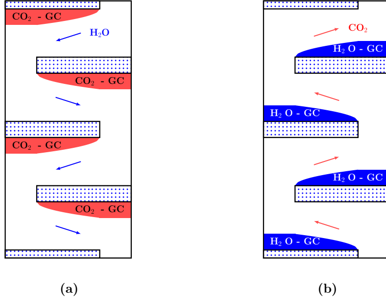
Figure 4.29 – Cas sans capillarité : sketch des courants de gravité dans une colonne bidimensionnelle pour la montée du CO_2 (a) et pour la migration descendante de la saumure (b).
