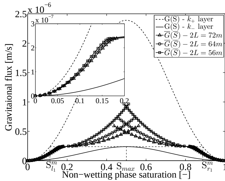
Figure 4.19 – Cas sans capillarité - Inclusions perméables : Flux gravitaire mis à l'échelle pour différentes géométries des inclusions perméables. La fenêtre rectangulaire en haut à gauche présente un zoom sur les faibles saturations.
