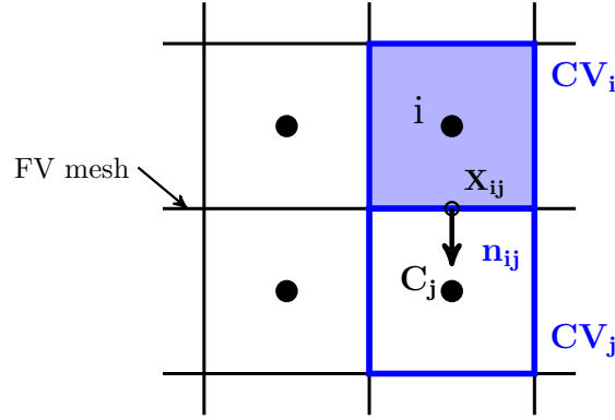
Figure 5.1 – Discrétisation de la méthode CCFV.
