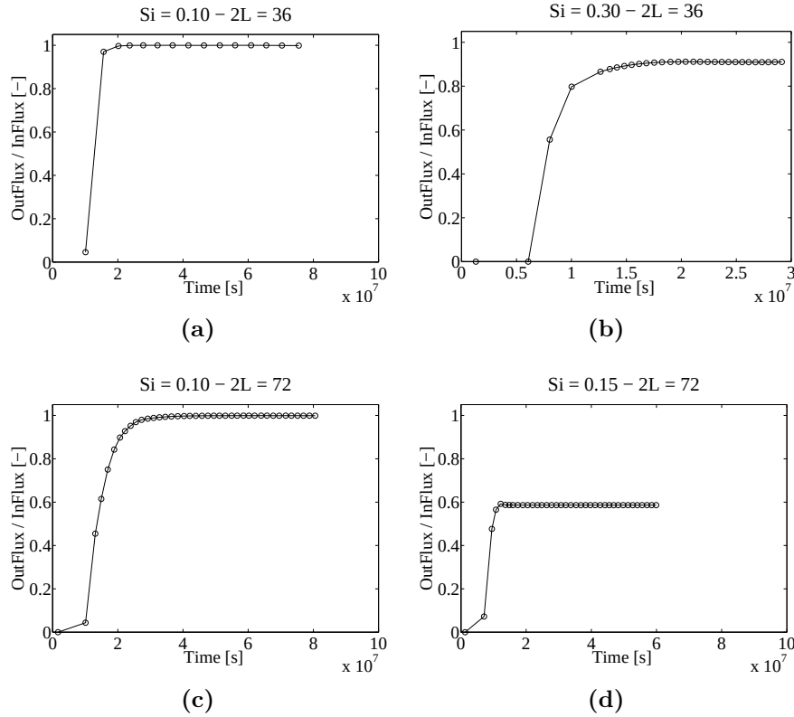
Figure 4.4 – Cas sans capillarité - Inclusion imperméable : rapport entre le flux sortant à travers les intervalles et le flux entrant en bas de la colonne dans le cas où 2L = 36 [m] (haut) et 2L = 72 [m] (bas). Résultats issus des simulations numériques à l'aide du code DuMu x .
