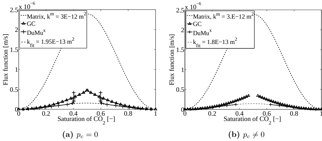
Figure 4.26 – Inclusions imperméables : flux total effectif pour le cas sans capillarité (à gauche) et avec capillarité (à droite). La longueur des inclusions est fixée à 2L = 72 \text{ m} .
