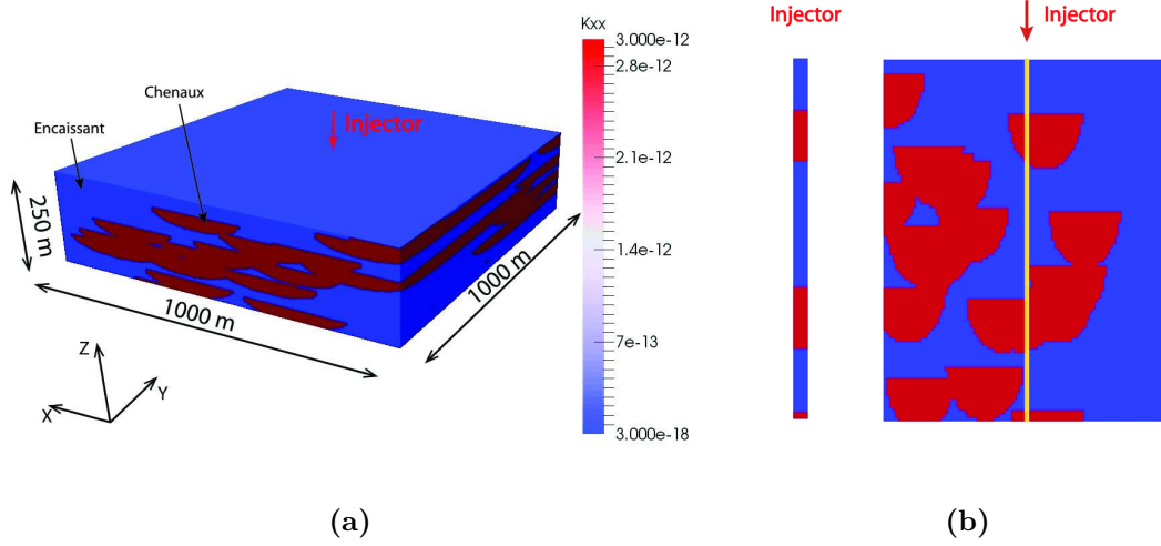
Figure 5.10 – Milieu fluvatile 3D : La dimension du milieu (a) et une coupe à la surface Y = 500 m passant à travers le puits injecteur (b).
