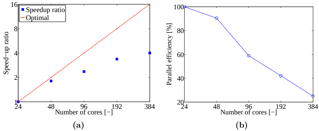
Figure 5.7 – Réprésentation log-log de l'accélération (a) et efficacité parallèle (b) pour le cas Implicite - YaspGrid.
