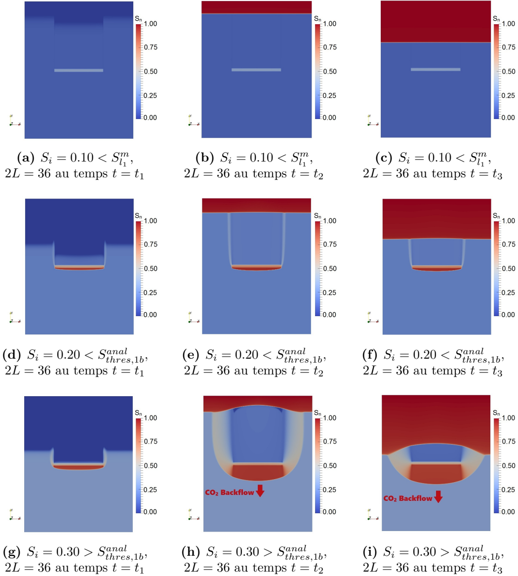
Figure 4.6 – Cas 3b - Cas sans capillarité - Inclusion semi-perméable : distribution du \text{CO}_2 à un temps court t_1 (a,d,g) quand le front \text{CO}_2 arrive à la barrière semi-perméable, à un temps intermédiaire t_2 (b,e,h) et à un temps relativement long t_3 (c,f,i) pour 2L = 36 [m].
