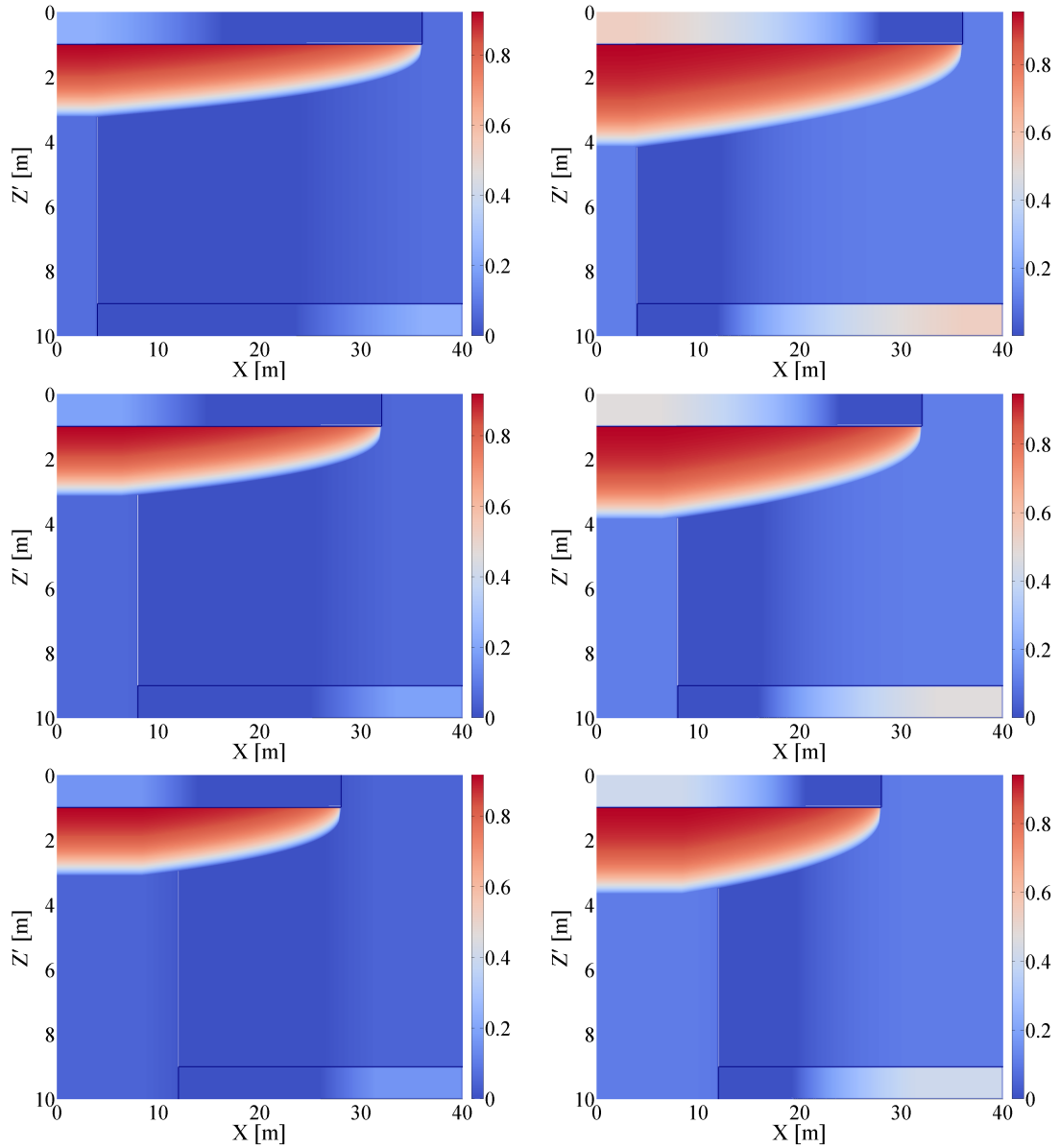
Figure 4.23 – Cas avec capillarité - Inclusions perméables : reconstruction de la solution du problème local à petite échelle obtenue par l’approche de courant de gravité : 2L = 72 [m] (haut), 2L = 64 [m] (milieu) et 2L = 56 [m] (bas) pour la saturation imposée S_i = 0,05 (à gauche) et S_i = 0,10 (à droite). Les inclusions sont délimitées par les traits continus.
