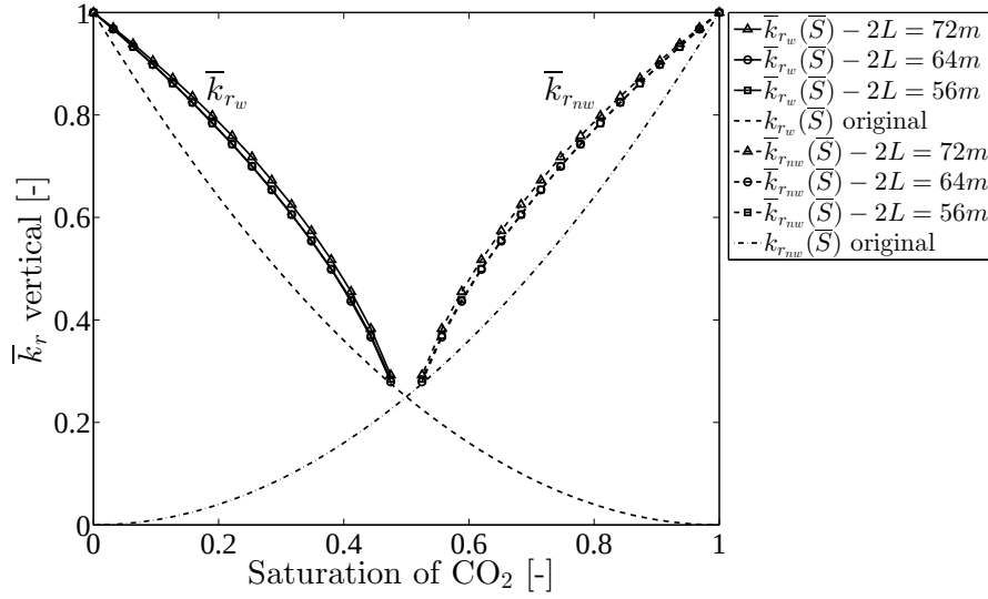
Figure 4.30 – Cas sans capillarité - Inclusions imperméables : perméabilité relative mise à l'échelle obtenue par l'approche SPA dans le cas L_0 = 40m et H_c = 10m .
