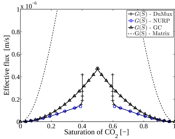
Figure 4.32 – Cas sans capillarité - Inclusions imperméables : flux effectif mis à l'échelle obtenu à partir des simulations diphasiques pour le cas L_0 = 40m et H_c = 10m .
