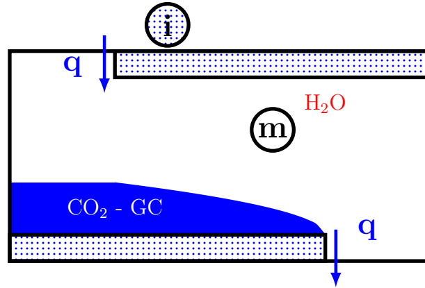
Figure 4.14 – Sketch de la migration descendante de H_2O dans une cellule.
