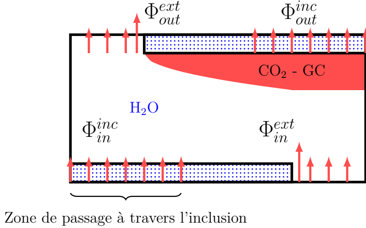
Figure 4.22 – Schéma de la montée du \text{CO}_2 dans le cas avec capillarité et inclusion perméable. Les flux distribués sont représentés par de petites flèches, les flux ponctuels par des flèches plus grandes.
