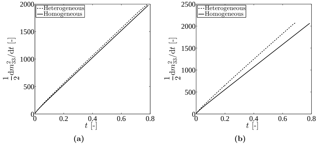
Figure A.6 – Dérivée temporelle du second moment centré pour les milieux périodique et homogène pour N_g = 0,10 (a) et N_g = 0,50 (b). La différence entre ces courbes souligne l'effet de l'hétérogénéité.
