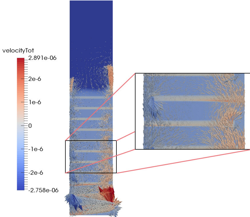
Figure B.5 – Champ de vitesse total pour le cas S_i = 0,30 avec un zoom au niveau des inclusions numéro n = 5 et n = 6 .
