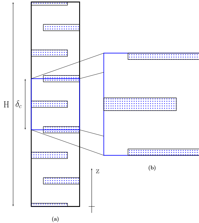
Figure 4.10 – La colonne périodique étudiée (a) et la zoom qui représente une cellule élémentaire de la colonne (b).
