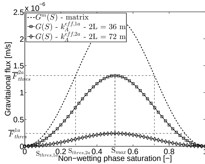
Figure 4.5 – Flux gravitaire de la zone équivalente pour 2L = 36 [m] et 2L = 72 [m]
