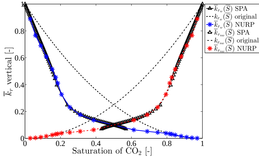
Figure 4.34 – Cas sans capillarité - Inclusions perméables : perméabilités relatives effectives de la saumure (ligne discontinue bleue avec étoiles) et du \text{CO}_2 (ligne discontinue-pointillée rouge avec étoiles), obtenues avec les méthodes SPA et NURP dans le cas 2L = 72m , L_0 = 40m et H_c = 10m .
