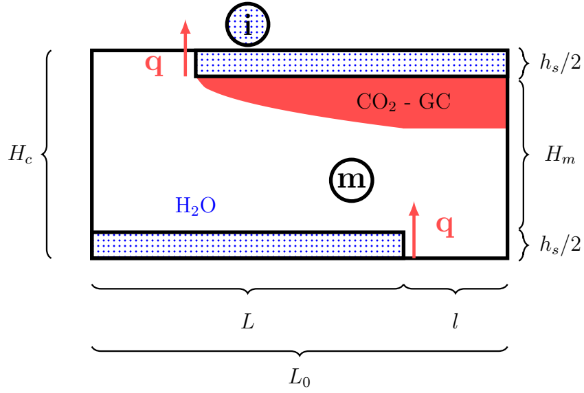
Figure 4.11 – Cellule d'un milieu stratifié périodique constitué d'inclusions imperméables. Les caractères i, m désignent l'inclusion et la matrice. h_s est l'épaisseur de l'inclusion, H_c la hauteur de la cellule et H_m représente l'écart vertical entre deux inclusions consécutives. 2L et L_0 représentent respectivement la largeur des inclusions et de la colonne étudiée. l = L_0 - L est une moitié de l'écart horizontal entre deux inclusions avoisinantes.
