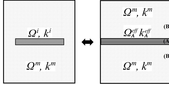
Figure 4.2 – Schéma du milieu initial, inclusion isolée (a), et décomposition en un milieu équivalent (b). k^i , k^m sont respectivement la perméabilité absolue de l'inclusion \Omega^i et de la matrice \Omega^m .
