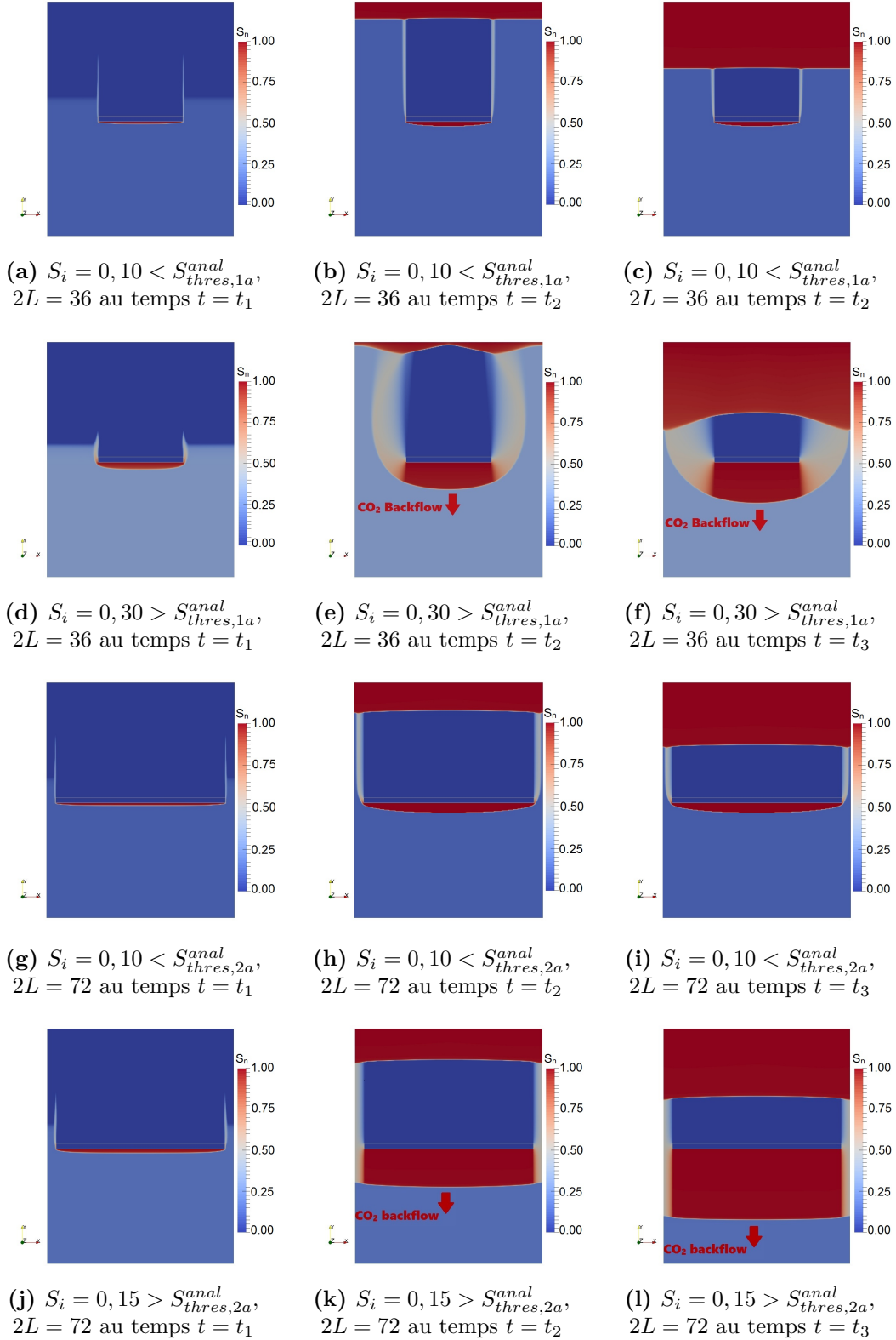
Figure 4.3 – Cas sans capillarité - Inclusion imperméable : distribution du CO_2 à un temps court t_1 (a,d,g,j) quand le front de CO_2 arrive à la barrière imperméable, à un temps intermédiaire t_2 (b,e,h,k) et à un temps relativement long t_3 (c,f,i,l). Dans chaque figure, le rectangle au centre du domaine indique les bords de l'inclusion.
