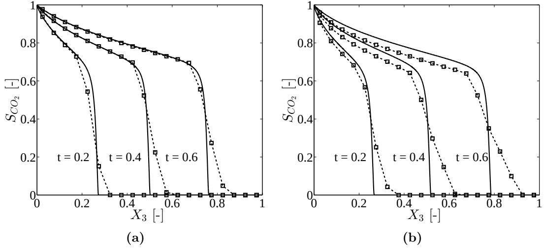
Figure A.5 – Profils de saturation de CO 2 en fonction de la coordonnée verticale pour le cas N_g = 0,10 (a) et N_g = 0,50 (b). Les courbes continues sont les solutions dans le milieu homogène équivalent en négligeant la dispersion, tandis que les courbes discontinues représente profil de saturation moyenné dans la cellule à partir de simulation numérique avec DuMu x dans le milieu hétérogène.
