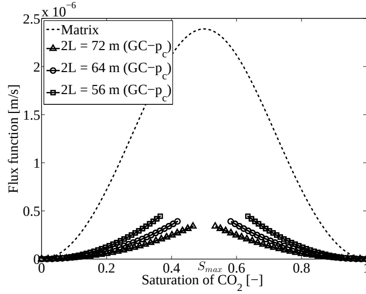
Figure 4.21 – Cas avec capillarité - Inclusions imperméables : flux gravitaire de la matrice homogène (lignes discontinues) et flux gravitaires mis à l'échelle calculés par l'approche des courants de gravité pour différentes valeurs de la longueur de l'inclusion (lignes continues avec symboles).
