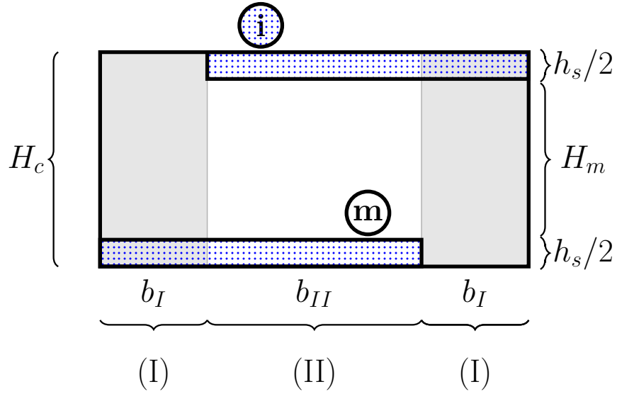
Figure 4.16 – Décomposition du domaine en multiples colonnes quasi-unidimensionnelles.
