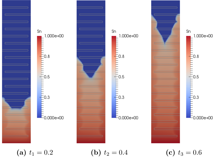
Figure A.4 – Carte de saturation du \text{CO}_2 dans la colonne bi-dimensionnelle à différents temps pour N_g = 0,5 . Les interfaces entre la matrice et les inclusions sont représentées par les rectangles. Le temps est adimensionné (équation (A.1)).
