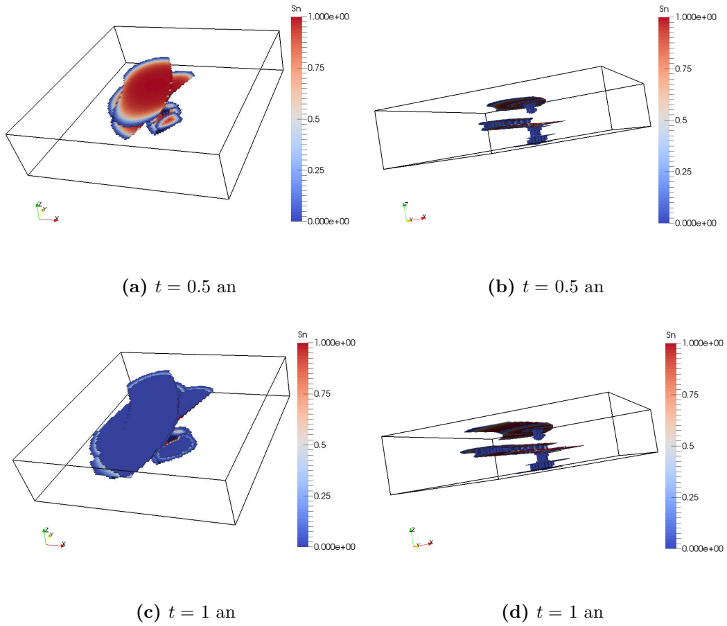
Figure 5.11 – Évolution du panache de CO_2 dans le milieu fluvial 3D vu de dessus (à gauche) et de dessous (à droite).
