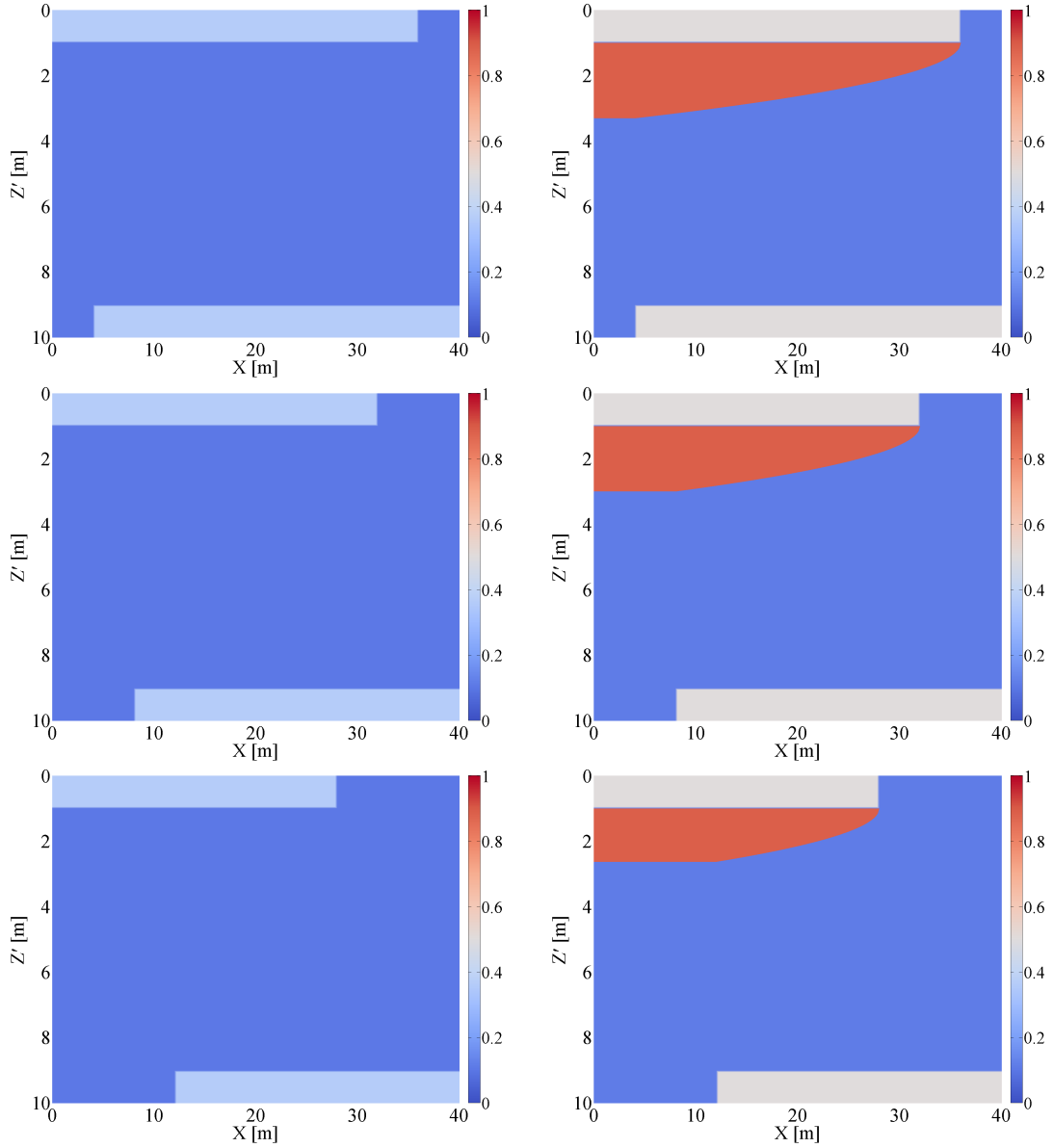
Figure 4.18 – Cas sans capillarité - Inclusions perméables : Reconstruction de la solution du problème local à petite échelle obtenue par l'approche de courant de gravité : 2L = 72 [m] (haut), 2L = 64 [m] (milieu) et 2L = 56 [m] (bas) pour la saturation imposée S_i = 0,05 (à gauche) et S_i = 0,10 (à droite). Le rapport entre la perméabilité des inclusions et celle de la matrice est égal à 0,10 qui conduit à S_{l_1}^m = 0,1127 . Les traits en gris représentent les interfaces entre la matrice et les inclusions.
