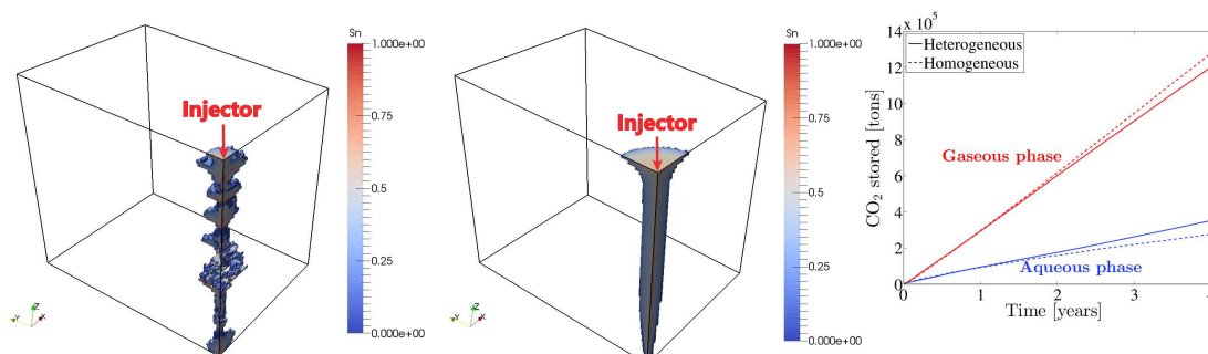
Figure 5.13 – Le panache de CO 2 après 5 ans d’injection dans le milieu réservoir SPE 10 hétérogène (à gauche) et dans le milieu homogène équivalent (au milieu). La sous-figure à droite montre l’évolution temporelle du CO 2 piégé sous forme gazeuse (CO 2 supercritique) et aqueuse (CO 2 dissout dans la saumure). La direction Z est multipliée par un facteur de 50.
