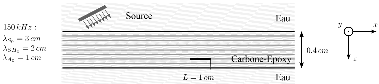
FIGURE 3.11 – Schéma de la plaque de carbone-époxy endommagée par une fissure horizontale. La fissure est centrée en (x_c, z_c = z_6) = (10, 0.3 cm).
