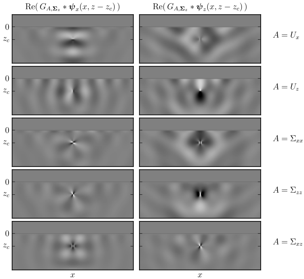
FIGURE 3.7 – Champ rayonné par un potentiel de double couche de forme \psi_x (figures de gauche) ou \psi_z (figures de droite) situé près d’une interface vide/aluminium, pour le paramètre de Laplace s = 1.0 + 13.5i \text{ rad MHz} . Au travers de la source le champ de déplacement est discontinu et le champ de contrainte normale \Sigma_z varie fortement tout en ayant une partie principale continue. Un potentiel de double couche intervient dans une condition aux limites de Neumann.
