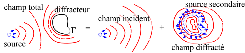
FIGURE 3.1 – Principe de Huygens-Fresnel : un défaut est remplacé par une distribution de potentiels de simple couche \mathbf{f}_s et de double couche \mathbf{f}_d rayonnant dans le milieu sans défaut.
