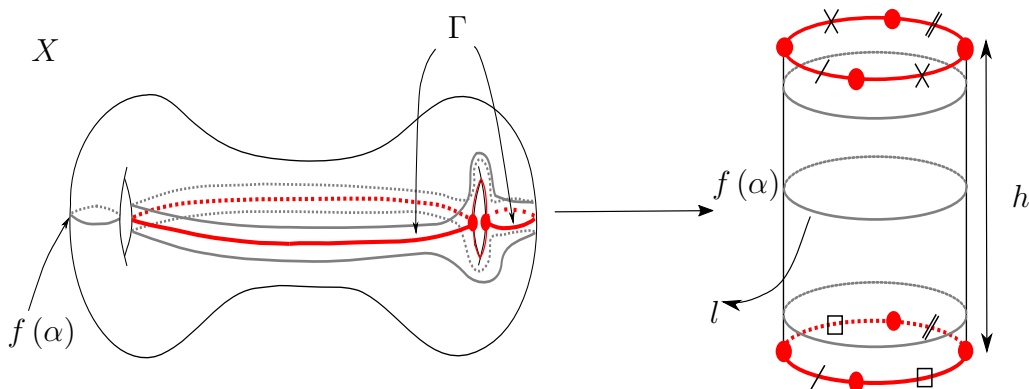
FIGURE 1 – Une manière grossière de voir le cylindre qui réalise l’infimum dans la définition 2.12 de la longueur extrême de \alpha \in \mathcal{S} sur x = [X, f] \in \mathcal{T}(X_0) . Le graphe rouge \Gamma représente le graphe critique du feuilletage associé à f(\alpha) et donc X \setminus \Gamma est biholomorphe à un cylindre euclidien de module \frac{h}{l} .
